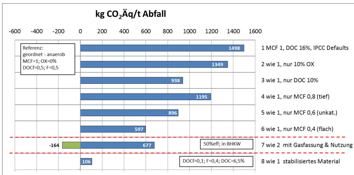
Abbildung 36: Varianten Deponierung
