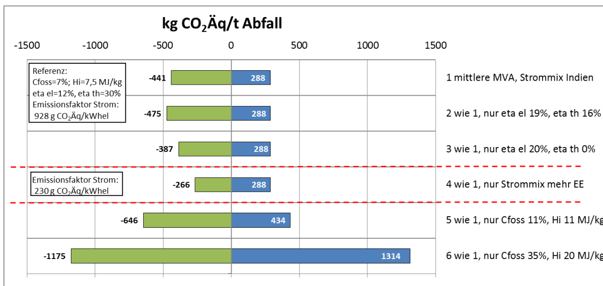
Abbildung 37: Varianten Abfallverbrennung
