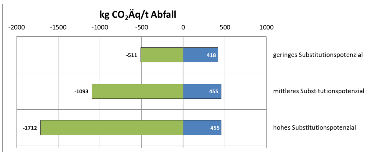
Abbildung 40: Varianten Kunststoffrecycling
