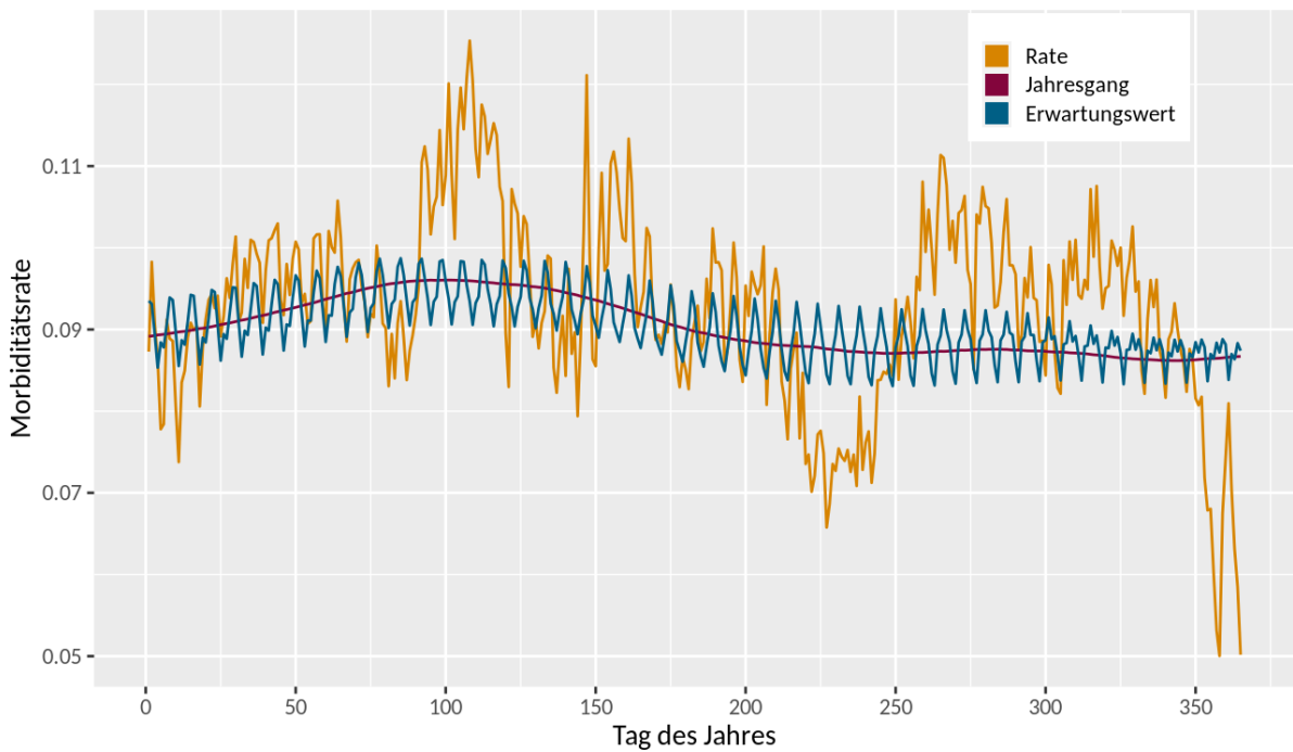
Abbildung A 3: Jahresverlauf der Mortalitätsrate aufgrund Asthma bronchiale und Status asthmaticus (J45 – J46) in Deutschland gemittelt über die Jahre 2001 – 2015 und den dazu berechneten Erwartungswert und geglättetem Jahresgang.
