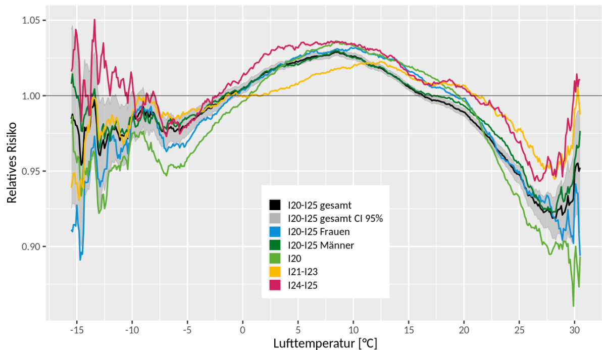
Abbildung 31: Zusammenhang zwischen dem Tagesmittelwert der Lufttemperatur und dem Relativen Risiko der Morbidität aufgrund von ischämischen Herzerkrankungen unterteilt in verschiedene ICD-Gruppen in den Jahren 2001 - 2015 in Deutschland.
