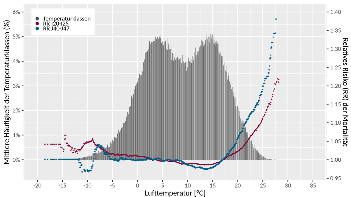
Abbildung 16: Häufigkeitsverteilung der Lufttemperaturklassen [%] der Ensembledaten des Referenzzeitraumes 1981 – 2010 und das Relative Risiko (RR) der Mortalität aufgrund von chronischen unteren Atemwegserkrankungen (J40 – J47) und ischämischen Herzerkrankungen (I20 – I25) pro Lufttemperaturklasse für Deutschland.
