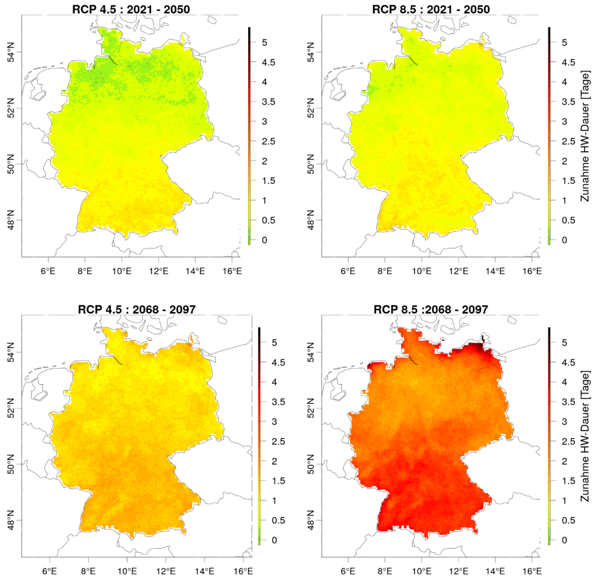
Abbildung 46: Änderung der mittleren Dauer von Hitzewellen im RCP4.5-Szenario für den Zeitraum 2021 – 2050 (links oben) und 2068 – 2097 (links unten) und im RCP8.5-Szenario für dieselben Zeiträume (rechts oben und unten).
