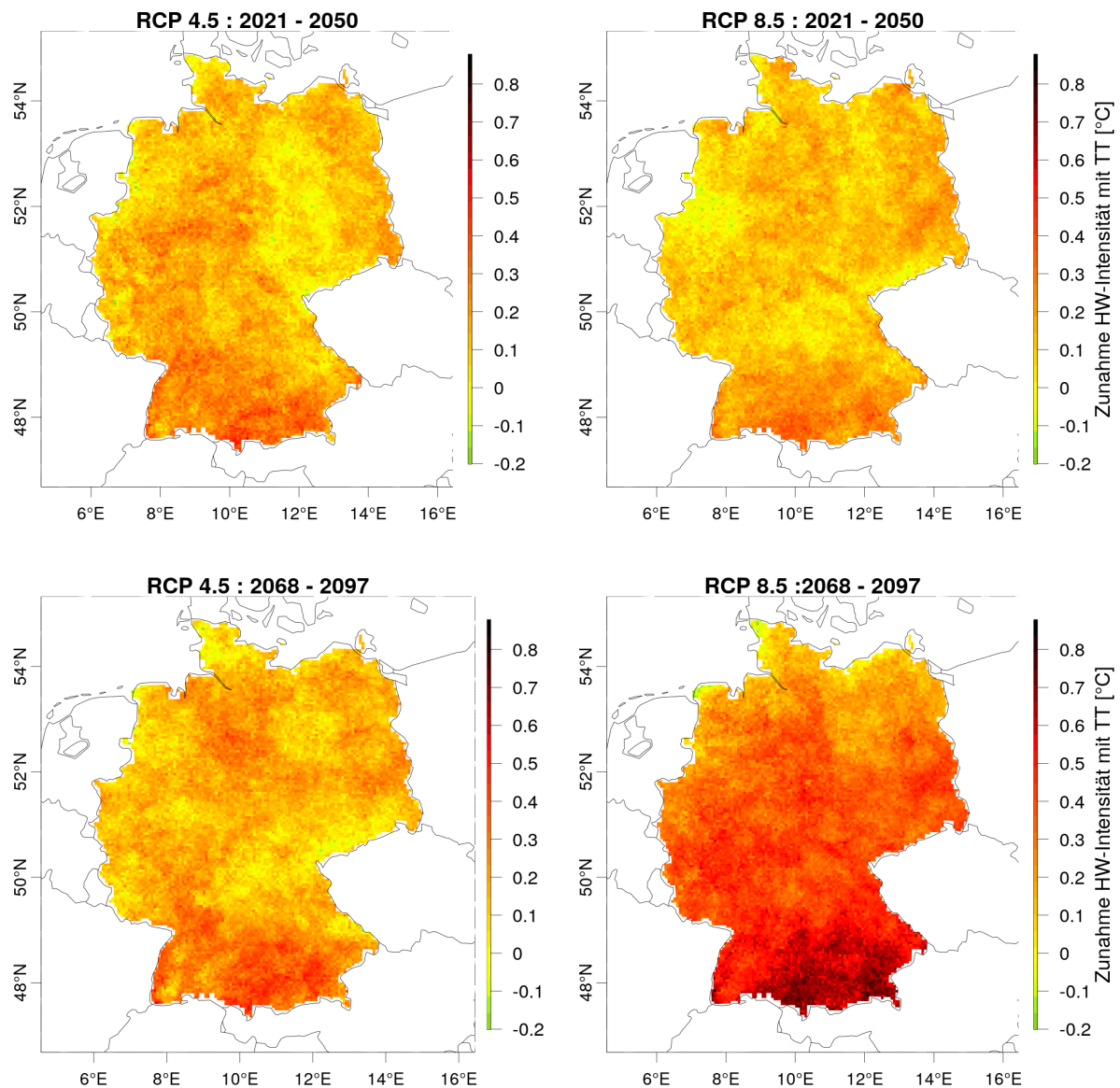
Abbildung 47: Änderung der mittleren Lufttemperatur während Hitzewellen im RCP4.5-Szenario für den Zeitraum 2021 – 2050 (links oben) und 2068 – 2097 (links unten) und im RCP8.5-Szenario für dieselben Zeiträume (rechts oben und unten).
