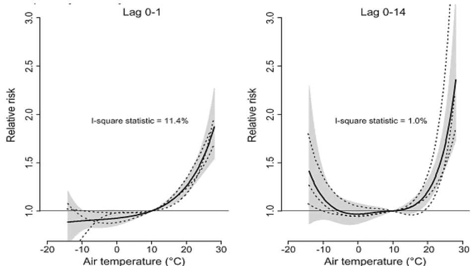
Abbildung 4: Vergleich des zeitlichen Wirkungsbereiches von Kälte und Hitze auf die Mortalität von Atemwegserkrankungen in Deutschland von 1990 bis 2006.
