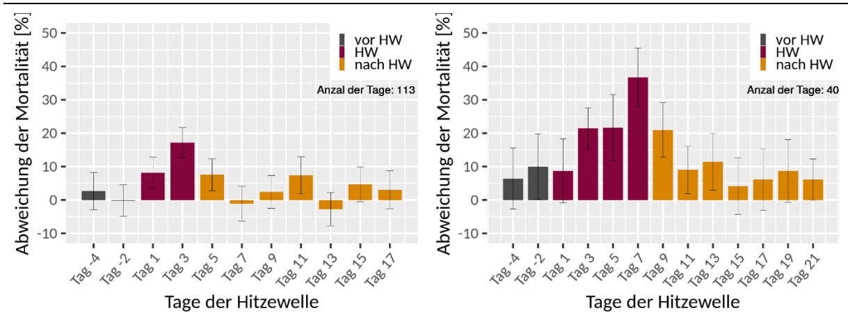
Abbildung 35: Prozentuale Abweichung der Mortalität aufgrund von chronischen Erkrankungen der unteren Atemwege (J40 – J47) im Verlauf von 4-tägigen (links) bzw. 8-tägigen Hitzewellen (rechts) mit Tagen vor, während und nach den Hitzewellen.
