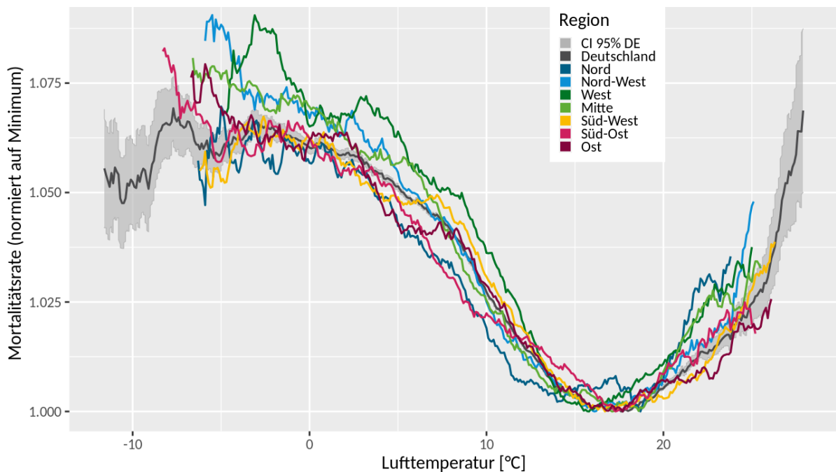
Abbildung 19: Zusammenhang zwischen dem Zweitagesmittelwert der Lufttemperatur und der 2-tägigem Mortalitätsrate aufgrund von chronischen Erkrankungen der unteren Atemwege (J40 – J47) in den Jahren 2001 - 2015 für sieben Großregionen und den Deutschlandmittelwert. *
