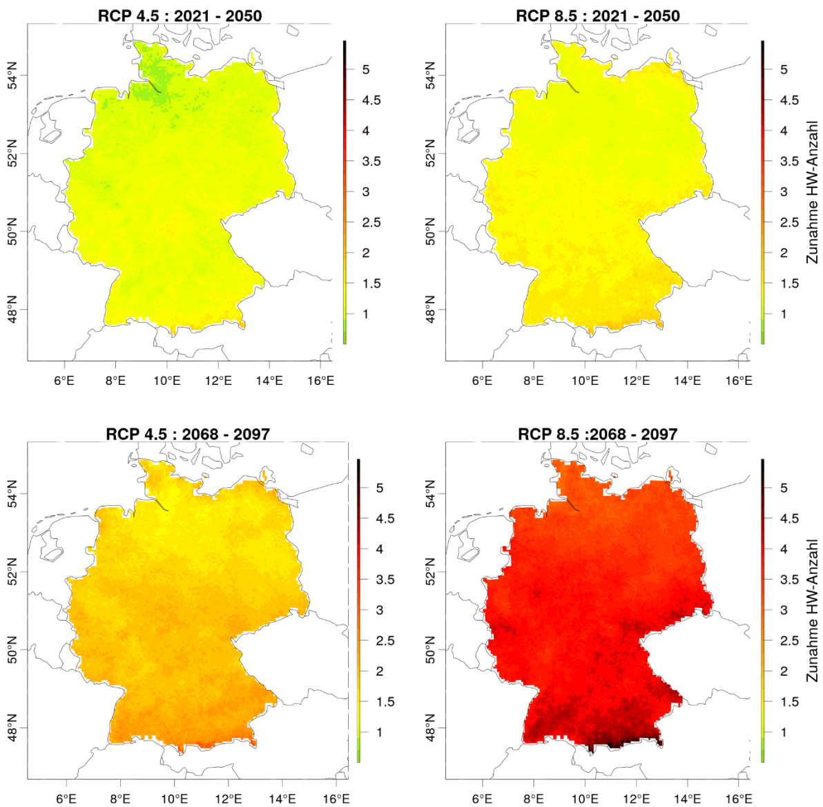
Abbildung 45: Änderung der mittleren Anzahl der Hitzewellen im RCP4.5-Szenario für den Zeitraum 2021 – 2050 (links oben) und 2068 – 2097 (links unten) und im RCP8.5-Szenario für dieselben Zeiträume (rechts oben und unten).
