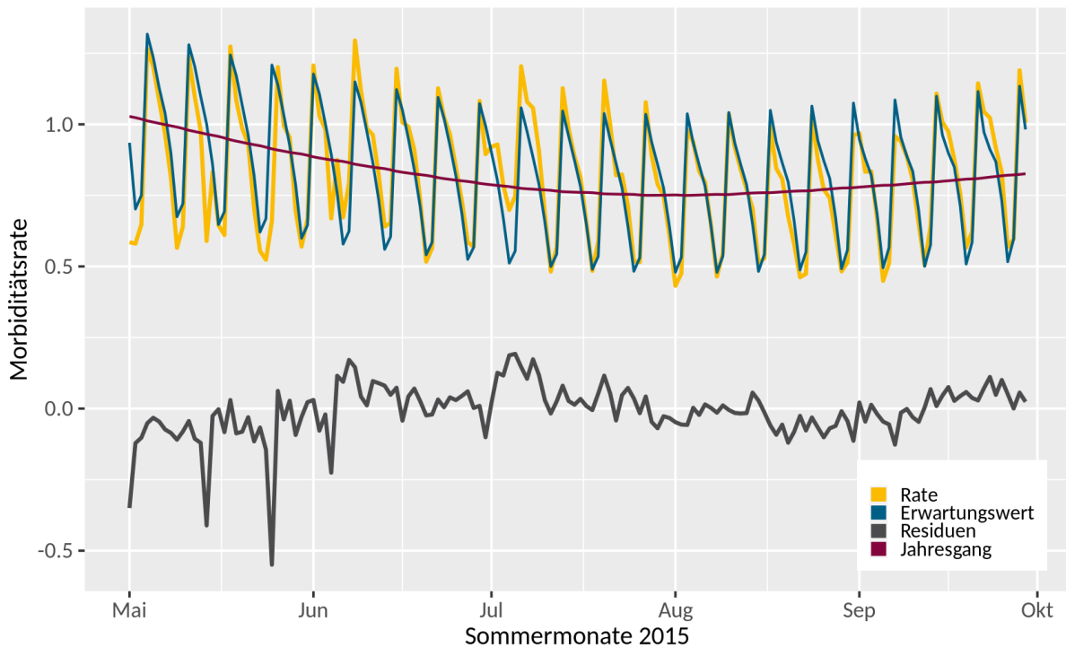
Abbildung 15: Morbiditätsrate, Jahresgang, Erwartungswert und Abweichungen vom Erwartungswert (Residuen) von COPD (J44) für den Zeitraum vom 01. Mai bis 30. September 2015.
