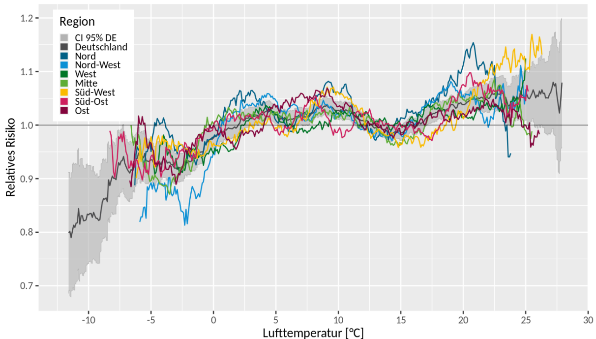
Abbildung 32: Zusammenhang zwischen dem Zweitagesmittelwert der Lufttemperatur und dem Relativen Risiko von Suiziden der Jahre 2001 – 2015 für sieben Großregionen und den Deutschlandmittelwert.
