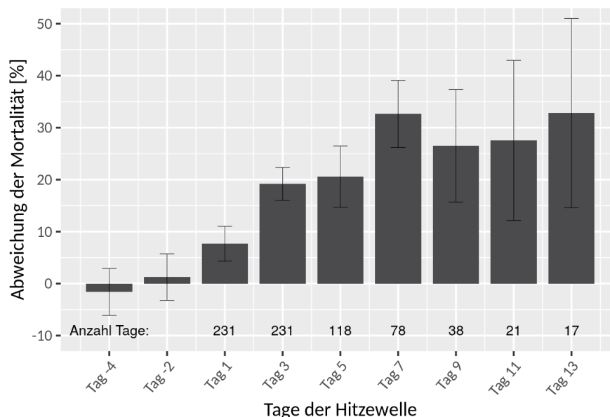
Abbildung 34: Prozentuale Abweichung der Mortalität aufgrund von chronischen Erkrankungen der unteren Atemwege (J40 – J47) während Hitzewellen gemittelt über die Jahre 2001 – 2015 in Deutschland.
