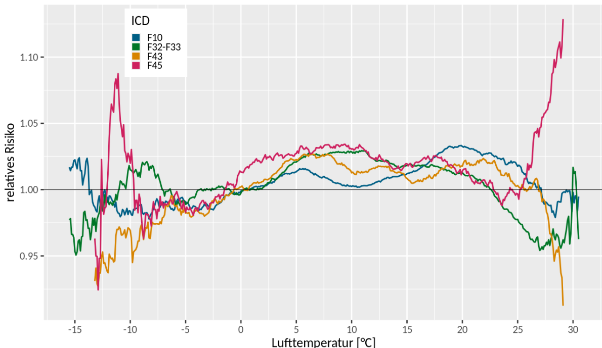
Abbildung 33: Zusammenhang zwischen dem Tagesmittelwert der Lufttemperatur und dem Relativen Risiko der Morbidität aufgrund von verschiedenen psychischen und Verhaltensstörungen in den Jahren 2001 - 2015 in Deutschland.
