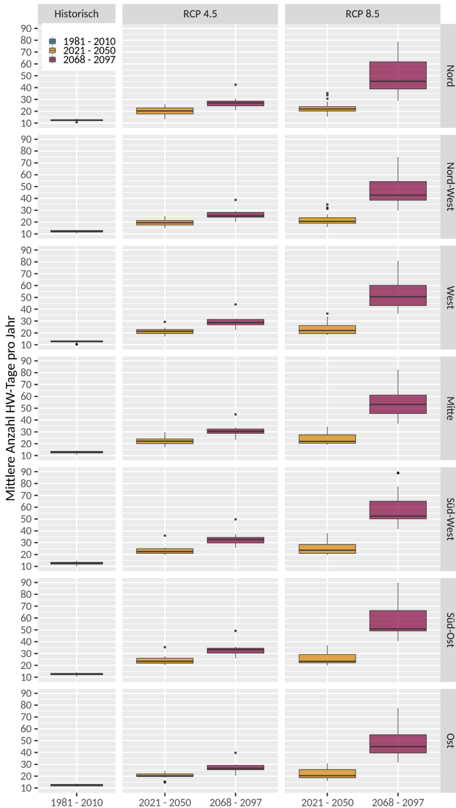
Abbildung A 5: Mittlere Anzahl der Hitzewellen-Tage pro Jahr im Referenzzeitraum 1981 – 2010 und die Veränderung der Anzahl in der Zukunft (2021 – 2050 und 2068 – 2097) anhand der RCP-Szenarien 4.5 und 8.5 in sieben Regionen in Deutschland.
