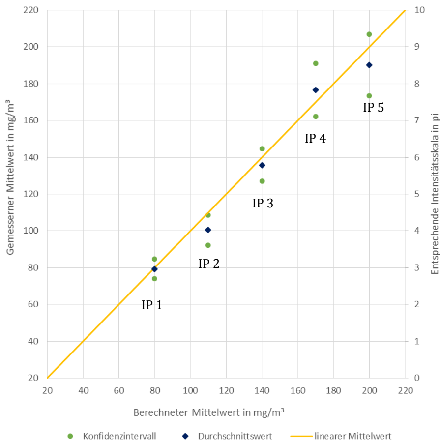
Abbildung 64: Ergebnisse der Mittenversuche – Phase 1 [Quelle: eigene Darstellung, HTW Berlin]
