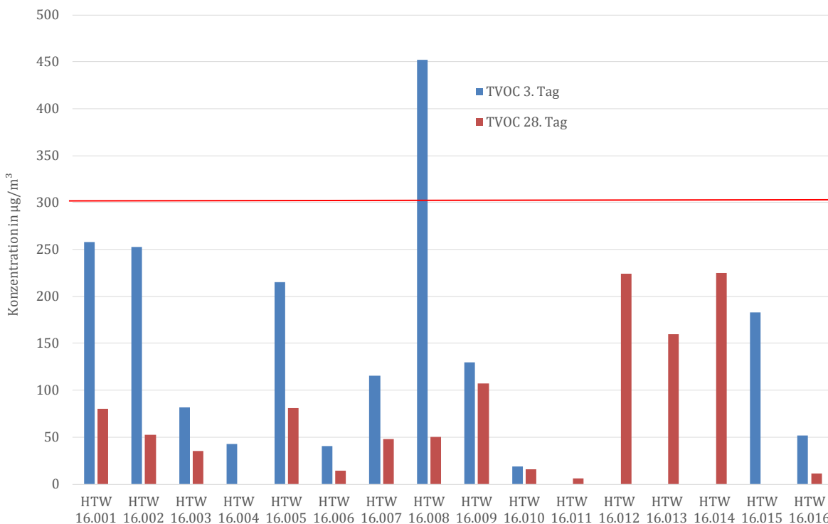
Abbildung Z5: TVOC-Werte der AgBB-Auswertung der elastischen Bodenbeläge am 3. und 28. Tag (rote Linie: Grenzwert UZ 120 = 300 µg/m³) [Quelle: eigene Darstellung, BAM]
