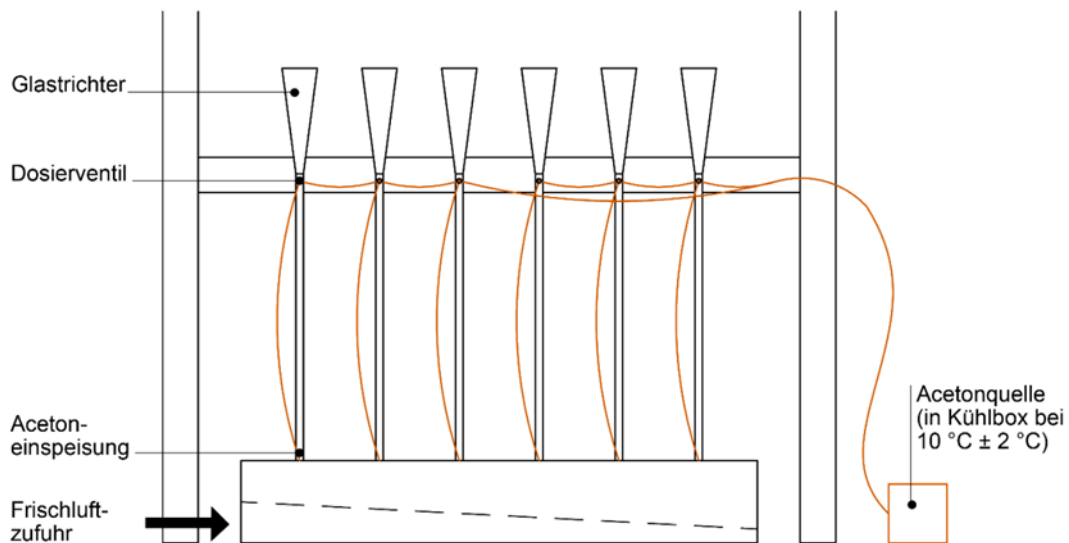
Abbildung 1: Konstruktionsprinzip des Vergleichsmaßstabs [Quelle: eigene Darstellung, HTW Berlin]
