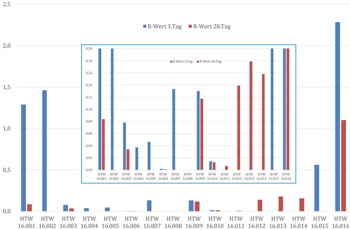
Abbildung 53: R-Werte der AgBB-Auswertung der elastischen Bodenbeläge am 3. und 28. Tag, das Inset zeigt die gleichen Daten nur mit einer vergrößerten Achsenskalierung [Quelle: eigene Darstellung, BAM]
