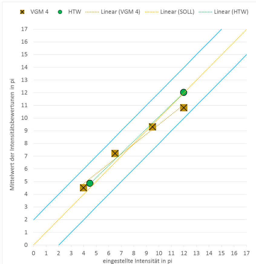
Abbildung 60: Mittelwerte der dargebotenen Acetonkonzentration (Vergleichsmaßstab 4) [Quelle: eigene Darstellung, HTW Berlin]
