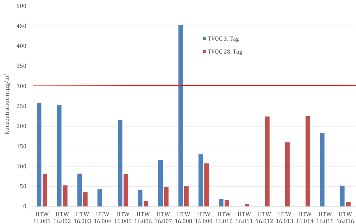
Abbildung 52: TVOC-Werte der AgBB-Auswertung der elastischen Bodenbeläge am 3. und 28. Tag (rote Linie: Grenzwert UZ 120 = 300 µg/m 3 ) [Quelle: eigene Darstellung, BAM]
