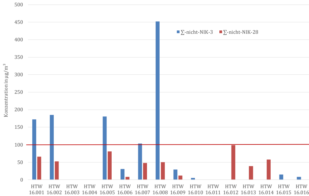
Abbildung 54: \Sigma -nicht-NIK-Werte der AgBB-Auswertung der elastischen Bodenbeläge am 3. und 28. Tag (Grenzwert UZ 120: 100 \mu\text{g}/\text{m}^3 am 28. Tag, rote Linie) [Quelle: eigene Darstellung, BAM]
