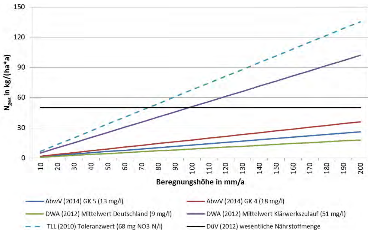
Abbildung 28: Potenzielle Stickstofffrachten ( N_{ges} ) in Abhängigkeit von der Beregnungshöhe bei Einhaltung der Anforderungen an Stickstoff für Kläranlagen der Größenklassen 4 und 5, der Einhaltung der Empfehlung des Bundeslands Thüringen, der mittleren Stickstoff-Ablaufkonzentration deutscher Klärwerke, der mittleren Zulaufkonzentration sowie die Definition „wesentliche Nährstoffmenge“ für die Stickstofffracht
