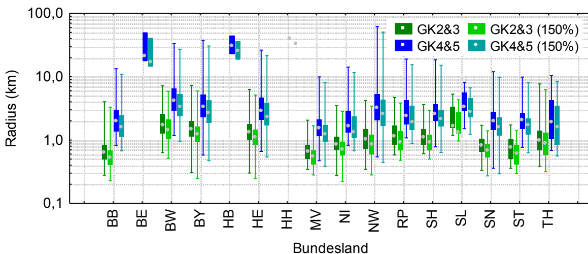
Abbildung 20: Radien der mit der vorhandenen Abwassermenge bewässerbaren Ackerfläche um die Kläranlagen (Größenklassen 2 und 3, Größenklassen 4 und 5) für die aktuelle und zukünftige (150 %) Beregnungshöhe in Abhängigkeit vom Bundesland
