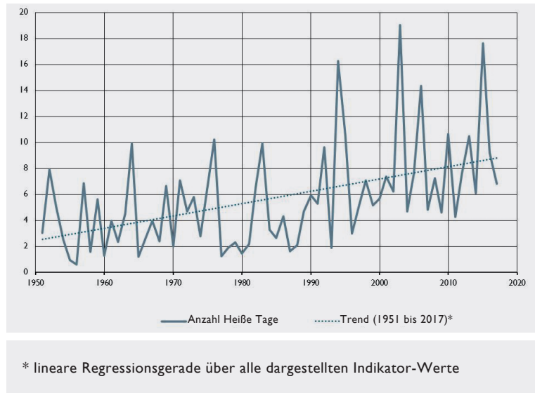
ABBILDUNG 1 Anzahl heißer Tage mit einem Maximum der Lufttemperatur von mindestens 30°C („Heißer Tag“) im Flächenmittel für Deutschland. Quelle: UBA 2018.
