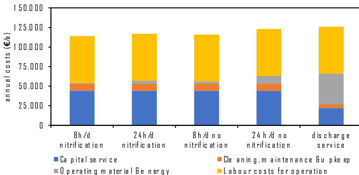
Abbildung 110: Vergleich des Jahreskosten der einzelnen MBR Betriebsmodi bei einem Betrieb von 250 d/a.
