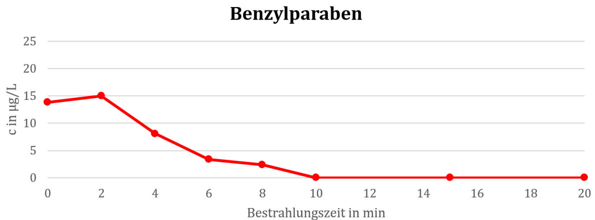
Abbildung 44: UV-unterstützter Abbau von Benzylparaben.
