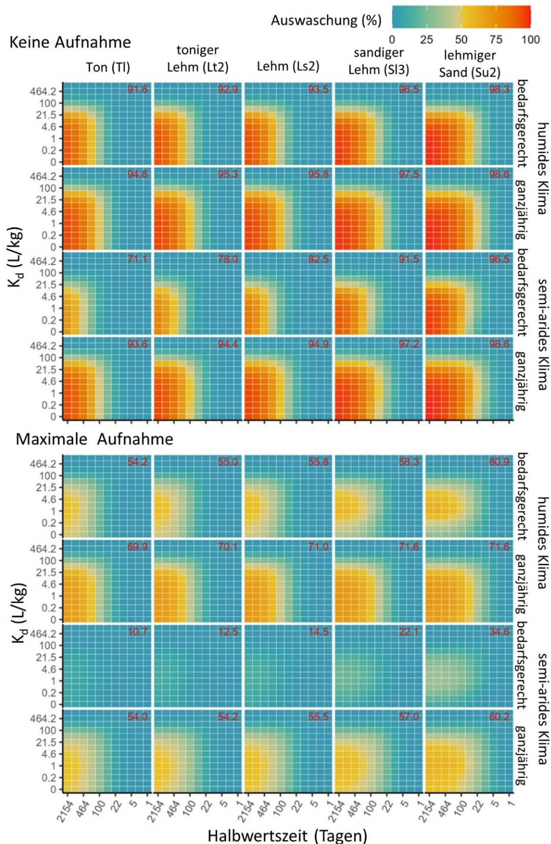
Abbildung 101: „Heatmap“ zur Auswaschung aller H1D Simulations-Szenarien.
