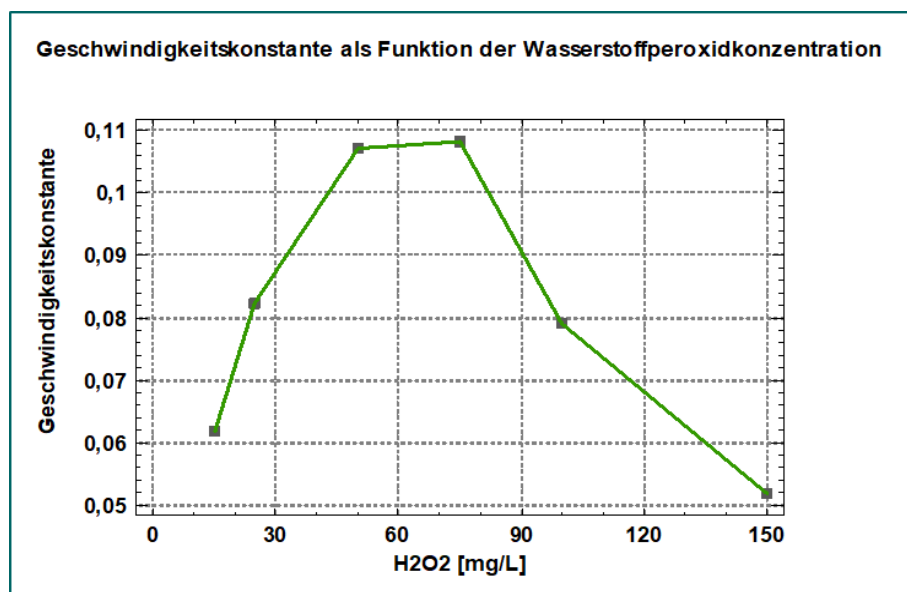
Abbildung 54: Abhängigkeit der Reaktionsgeschwindigkeit von der Wasserstoffperoxidkonzentration.
