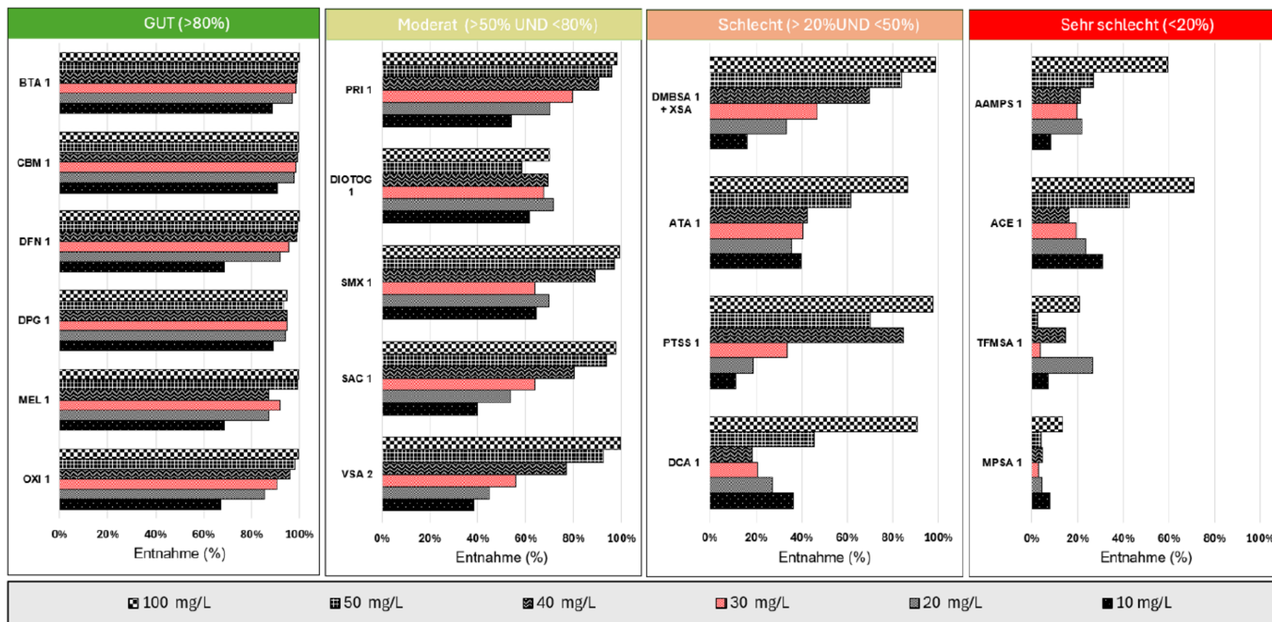
Abbildung 32: Klassifizierung der Pulveraktivkohle SAE SUPER anhand der Reduktionsraten bei 30 mg/L PAK (in Rot) und 24 Stunden Kontaktzeit (negative Eliminationsraten wurden auf 0 % gesetzt).
