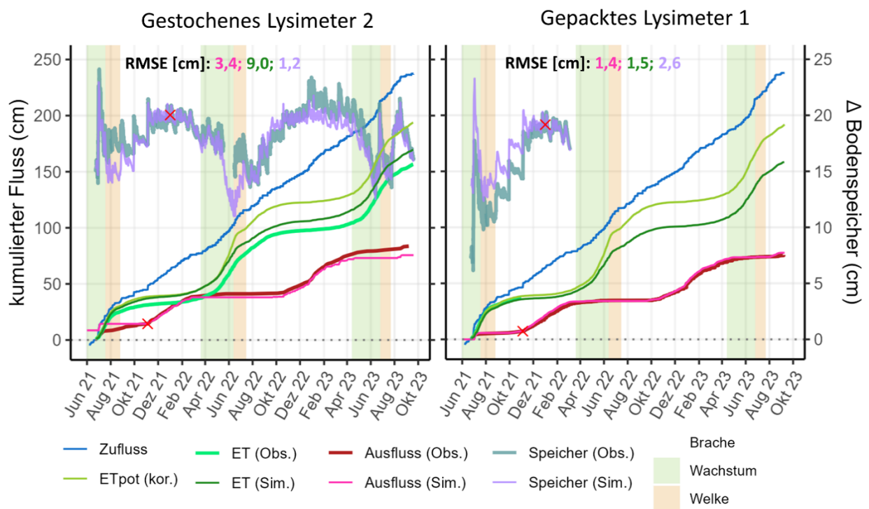
Abbildung 90: Vergleich der simulierten zu beobachteten Wasserhaushaltsgrößen für 2 Lysimeter.
