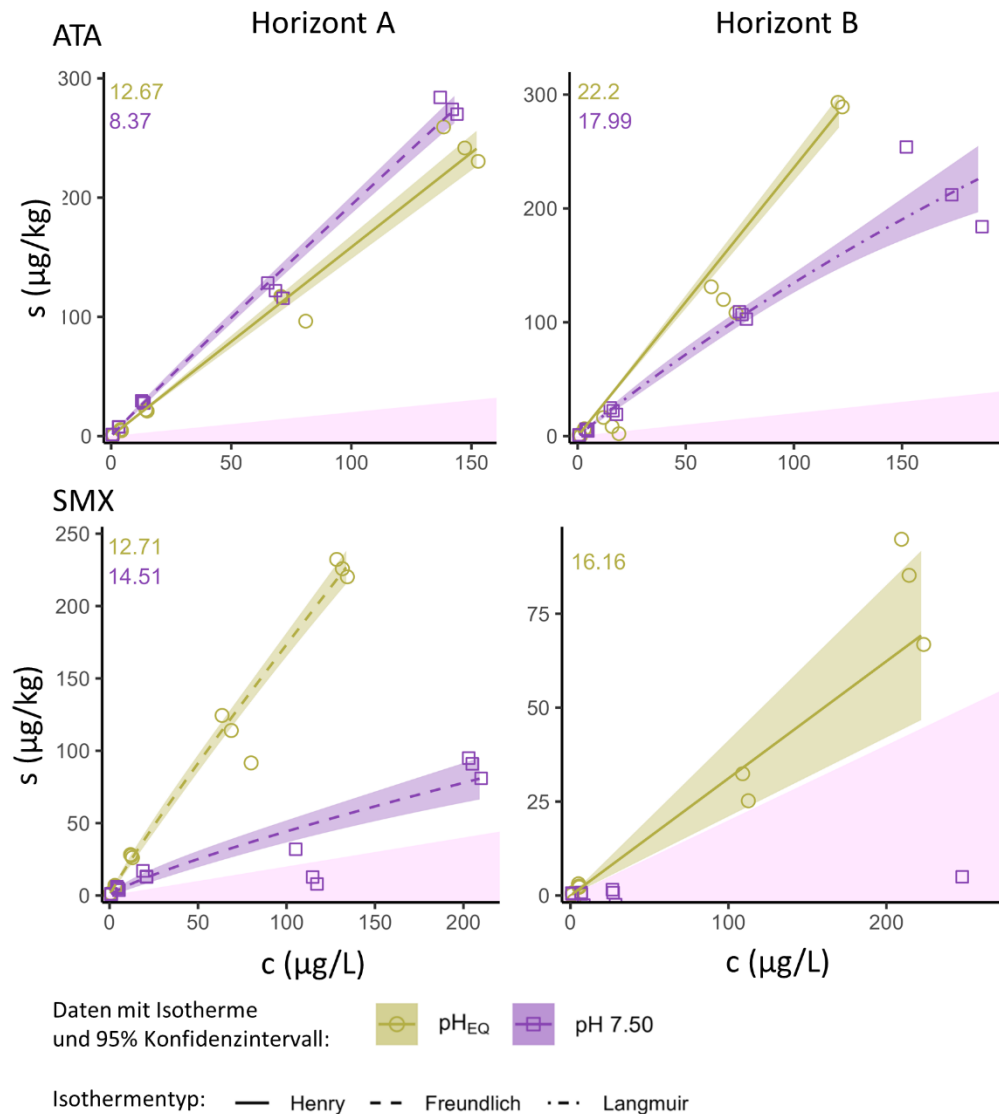
Abbildung 72: Einfluss des pH-Wertes auf die Sorption von ATA und SMX.
