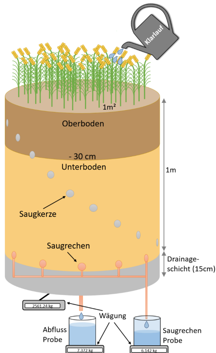
Abbildung 78: Schematische Zeichnung des Lysimeterversuchs mit der der zugehörigen Instrumentierung durch Saugkerzen, Saugrächen und Wäge- und Drainagesystem.
