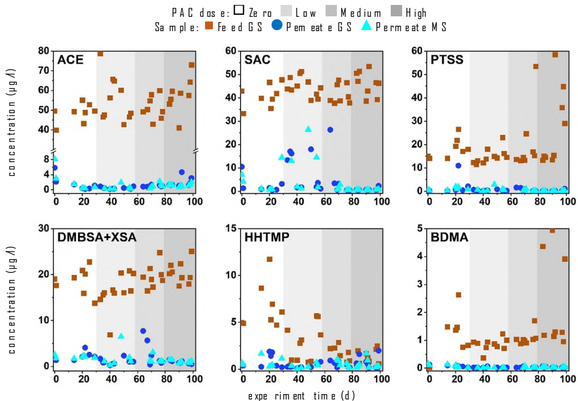
Abbildung 36: Feed- und Permeatkonzentrationen biologisch abbaubarer organischer Spurenstoffe (weißer Hintergrund für Betrieb ohne PAK, hellgrau für niedrige, grau für mittlere und dunkelgrau für hohe PAK-Dosen).
