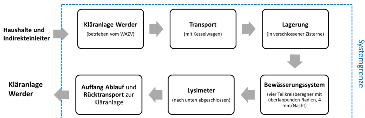
Abbildung 117: Prozessschema des Bewässerungsversuchs mit Klarlauf.
