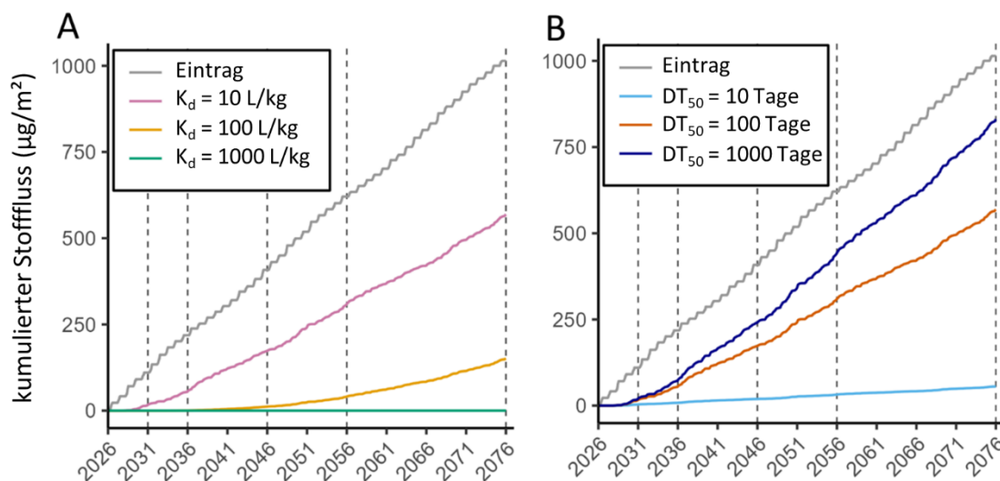
Abbildung 100: Herleitung der Auswaschungs-Werte.
