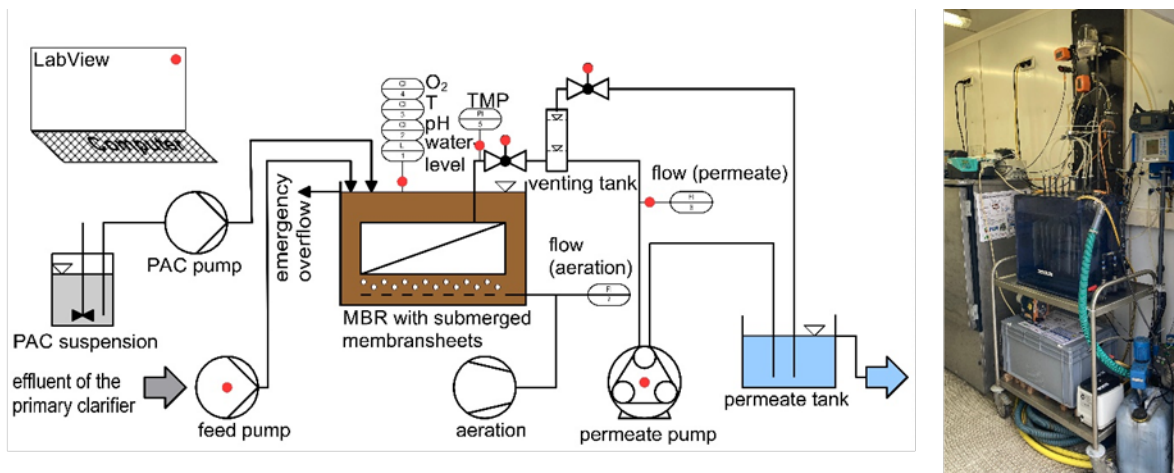
Abbildung 9: Prozessschema (links) und Foto des MBR (rechts); die im Prozessschema mit roten Punkten markierten Geräte sind mit dem Prozessleitsystem verbunden.
