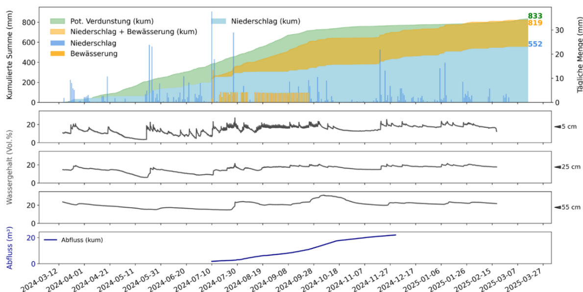
Abbildung 118: Darstellung der Eingangsgrößen zur klimatischen Wasserbilanz für das hydrologische Jahr März 2024 - März 2025. Die eingegangenen Niederschlagsdaten entstammen der Wetterstation Großkreutz-Krielow, die der Verdunstung der Station Potsdam. Darunter ist der volumetrische Bodenwassergehalt jeweils für die Tiefen 5, 25 und 75 cm für eine Messsonde des Klarlauf-Lysimeters dargestellt. Die Abflussmenge des Klarlauf-Lysimeters ist unten dargestellt.
