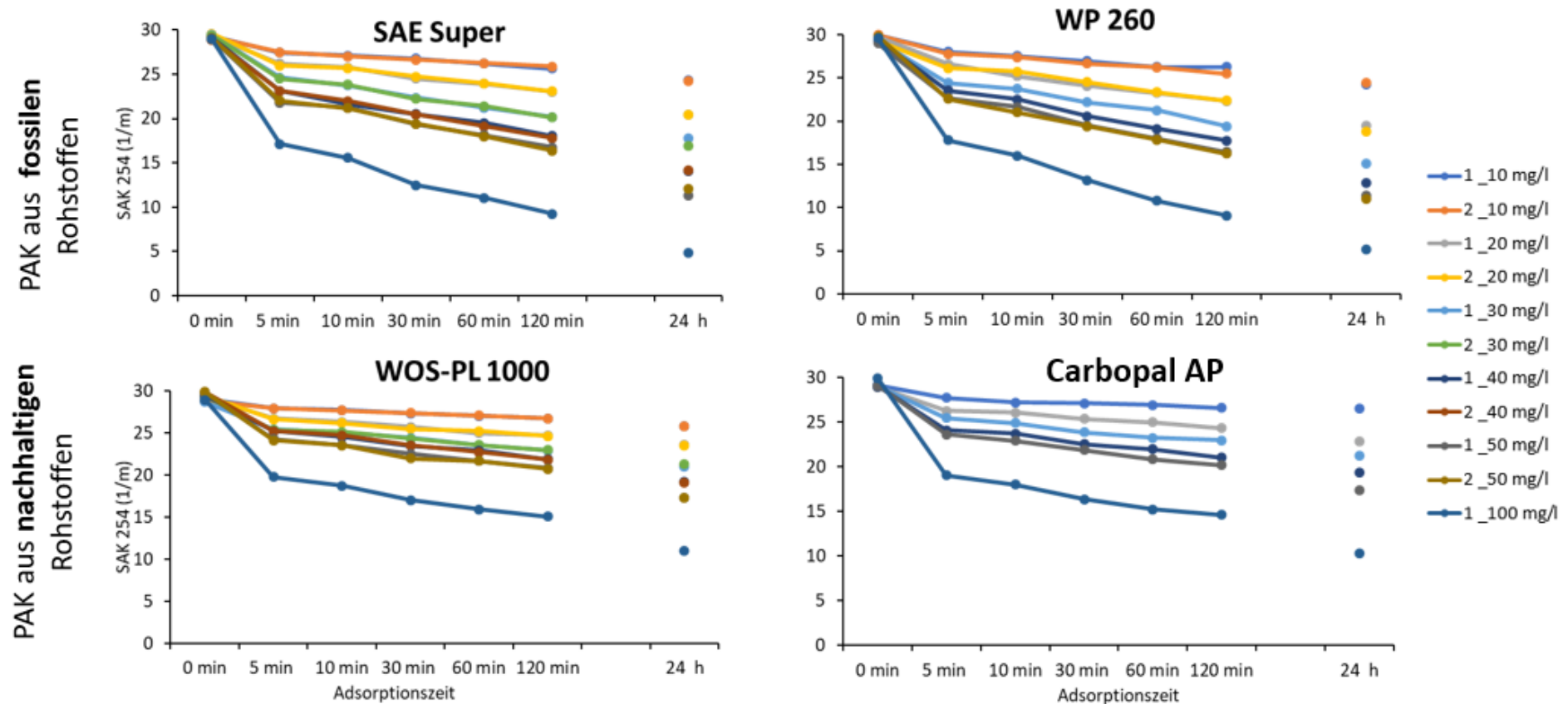
Abbildung 29: Eliminationsleistung der untersuchten PAK-Produkte anhand des UV 254
