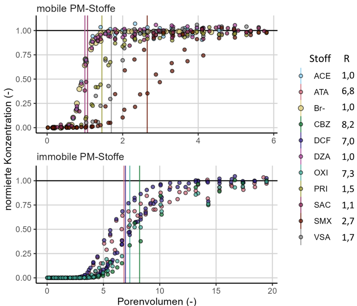
Abbildung 77: Durchbruchkurven von Bromid und 10 PM-Stoffen in den gepackten Säulen.
