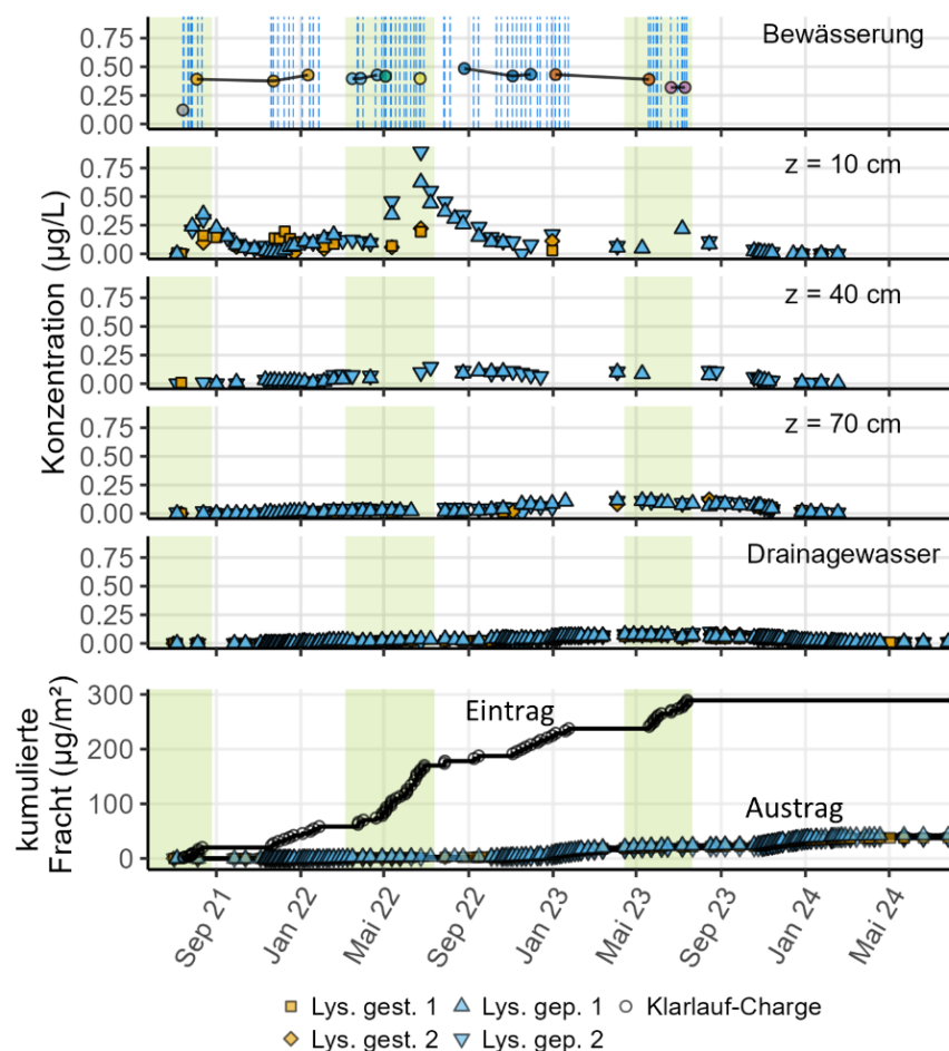
Abbildung 84: Zeitreihen der PRI -Konzentration verschiedener Tiefen und der kumulierten Grenzfrachten.
