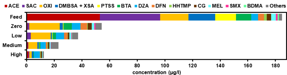
Abbildung 35: Kumulierte Konzentrationen organischer Spurenstoffe mit individuellen mittleren Konzentrationen > 1 \mu\text{g}/\text{L} sowie weiteren organischen Spurenstoffen (kumulierte Konzentration aller Parameter mit individuellen Konzentrationen < 1 \mu\text{g}/\text{L} im MBR-Feed).
