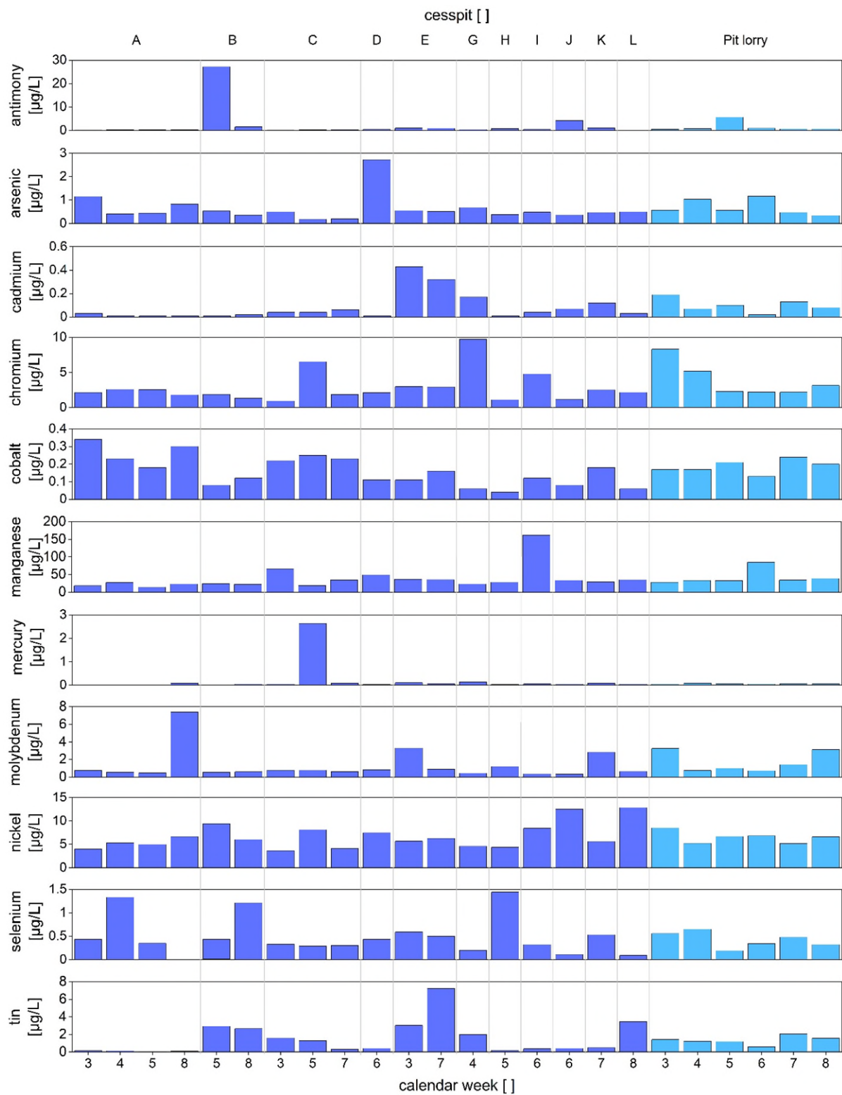
Abbildung 6: Schwermetallkonzentrationen in den Gruben- (A bis L) und Saugwagenproben.
