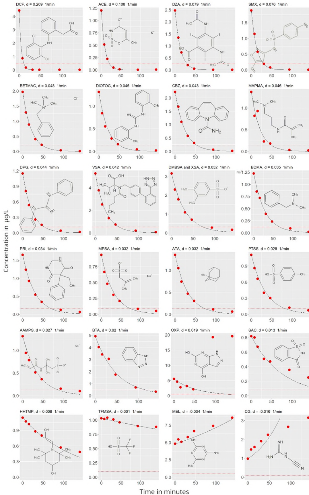
Abbildung 56: Abbaukonstanten für 24 Spurenstoffe mit 100 mL/s Rezirkulation, 20 mg/L H 2 O 2 , 185 & 254 nm Strahler, in Kläranlagenablauf. Die rote Linie zeigt 10 % von c 0 an.
