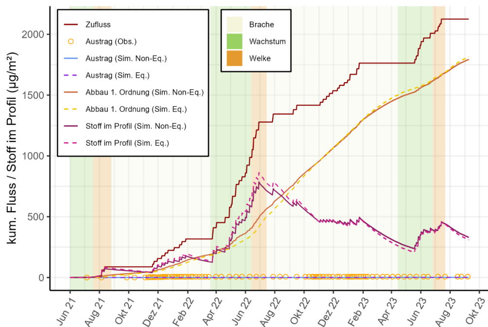
Abbildung 94: Simulierte und beobachtete Stoffflüsse von DCF im gepackten Lysimeter 1.
