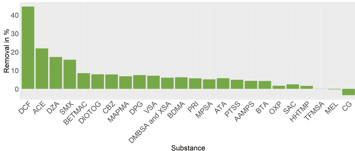
Abbildung 57: Spurenstoffentfernung nach berechnetem einmaligem UV-Reaktor-Durchgang bei 100 mL/s, 20 mg/L Wasserstoffperoxid, 254 nm Strahler, in UF-Permeat.
