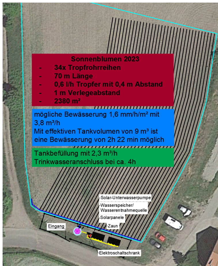
Abbildung 113: Installationsaufbau zur Bewässerung von Sonnenblumen (2023).
