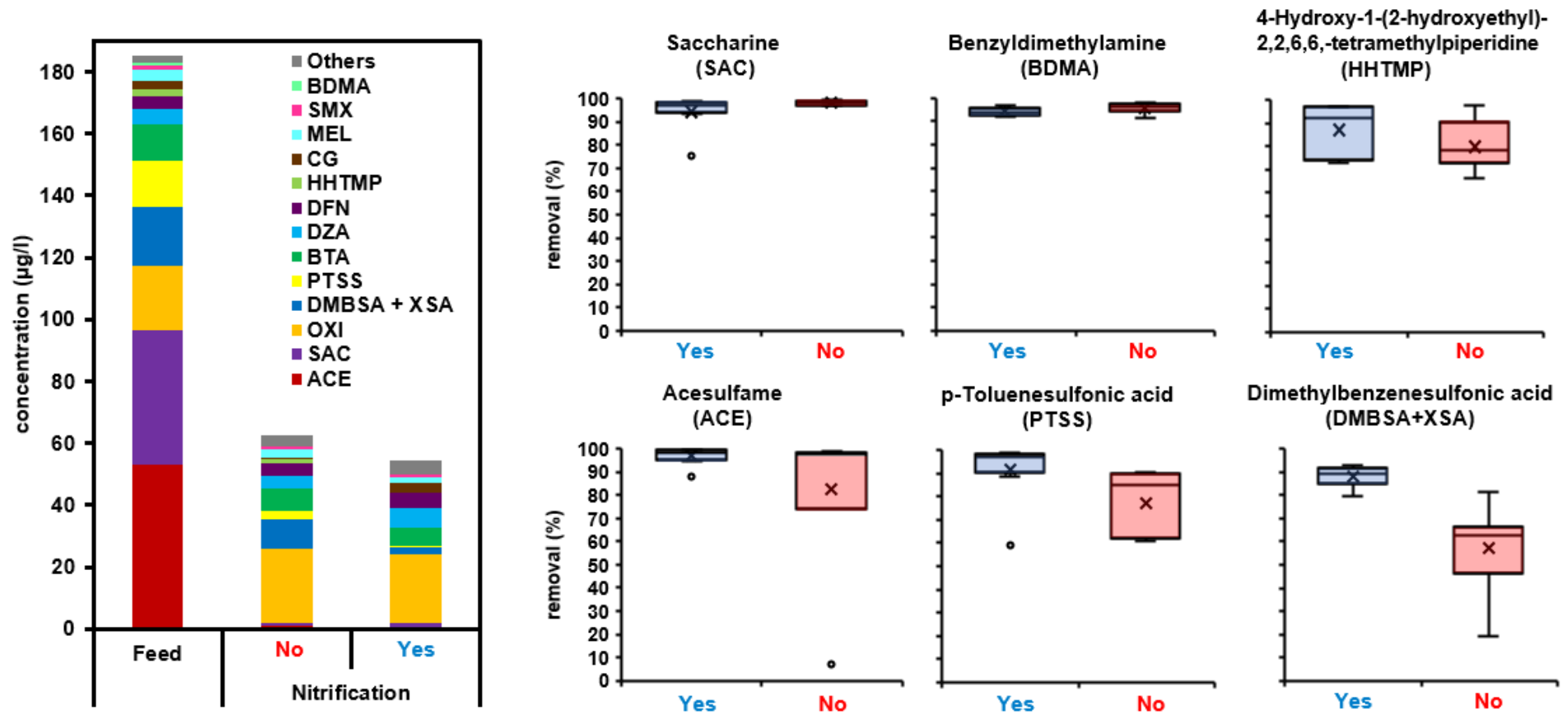
Abbildung 20: Elimination von 24 organischen Spurenstoffen beim MBR-Betrieb mit Nitrifikation bzw. ausschließlicher Kohlenstoffelimination (links; Spurenstoffe < 1 µg/l sind in der Kategorie „Others“ zusammengefasst) und Vergleich von sechs biologisch gut abbaubaren Spurenstoffen beim Betrieb mit und ohne Nitrifikation (rechts).
