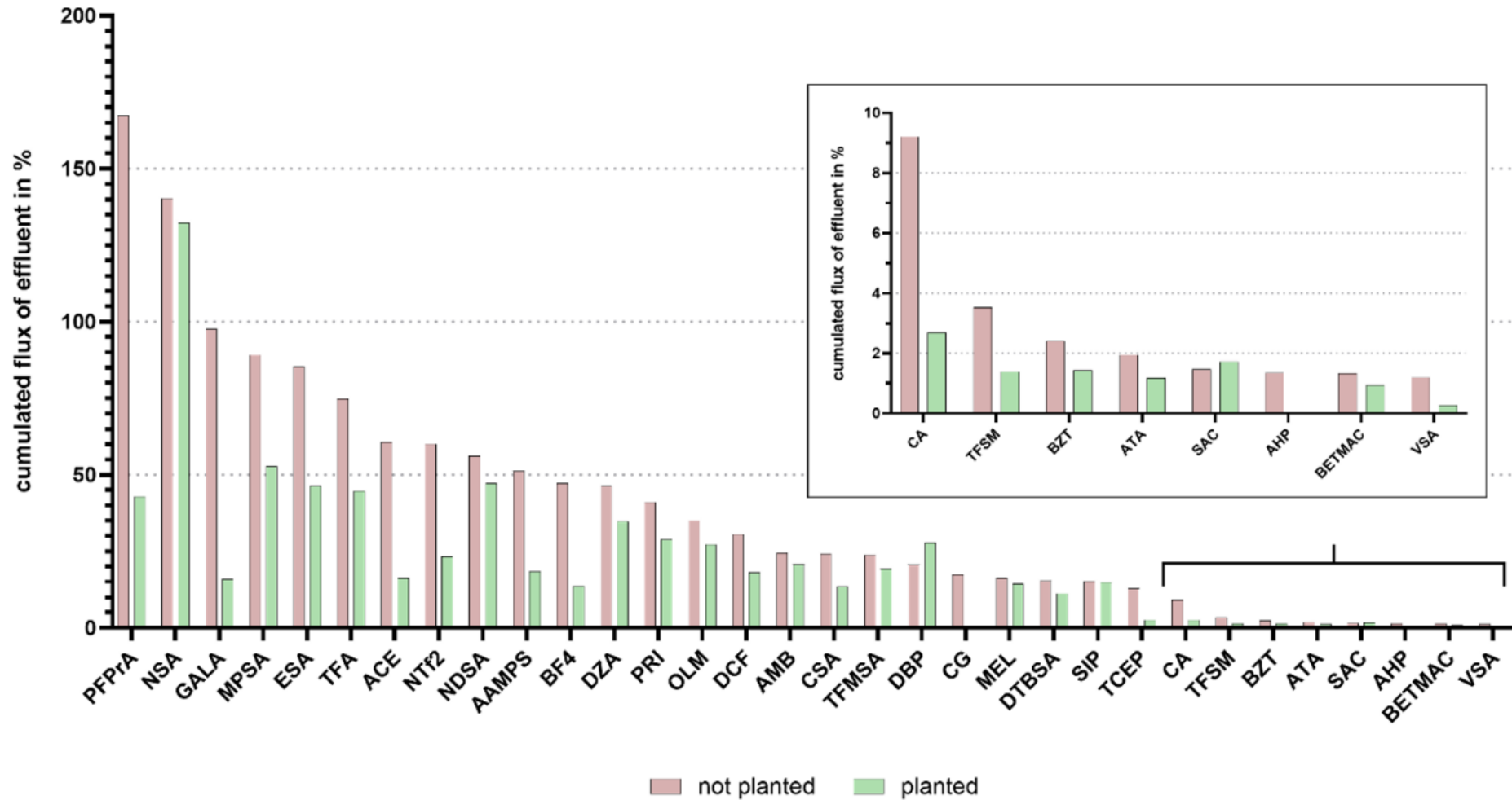
Abbildung 2: Kumulierte Fracht an PM-Stoffen im Ablauf der Lysimeter (60 cm) über die Betriebszeit von 9 Monaten bezogen auf die kumulierte Fracht im Zulauf in %, für bepflanzte (grün) und nicht-bepflanzte (rot) Lysimeter.
