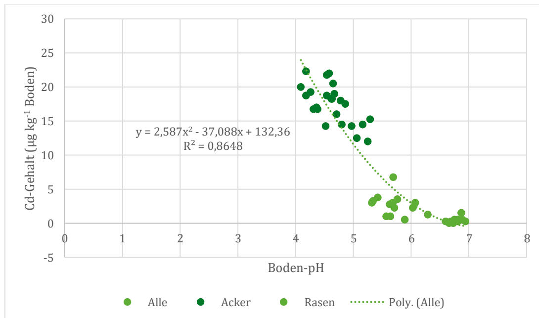
Abbildung 60: Einfluss des Boden-pH-Wertes auf die Gehalte an \text{NH}_4\text{NO}_3 -löslichem Cd im Boden; die Symbole stellen die Messwerte der Gefäße mit Ackerboden (Acker) und Rasentragschicht (Rasen) dar.
