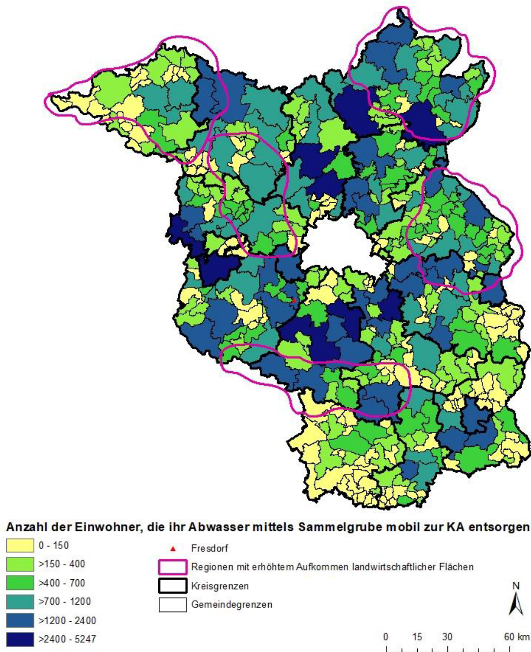
Abbildung 106: Anzahl der Einwohner mit abflusslosen Sammelgruben (2019) und Regionen viel landwirtschaftlich genutzter Fläche (2018).
