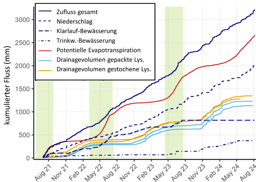
Abbildung 80: Kumulative Flüsse an der oberen und unteren Grenze der Lysimeter.
