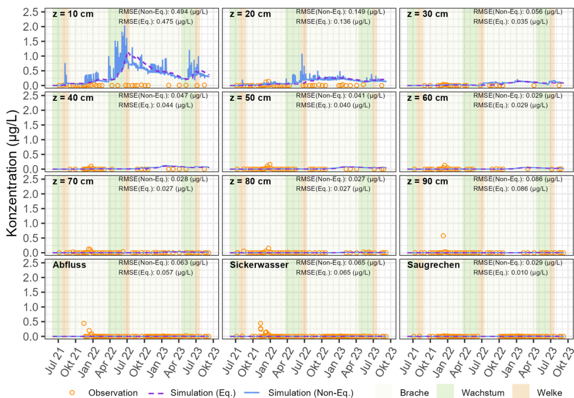
Abbildung 93: Vergleich des observierten und simulierten Transports von DCF im gepackten Lysimeter 1.
