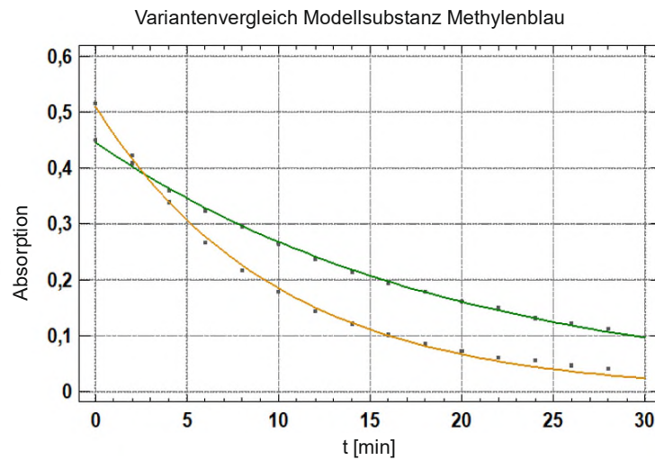
Abbildung 41: Abbaugeschwindigkeiten zur Prozessbeschreibung am Beispiel der Verwendung eines Photokatalysators (mit Katalysator orange, ohne Katalysator grün).
