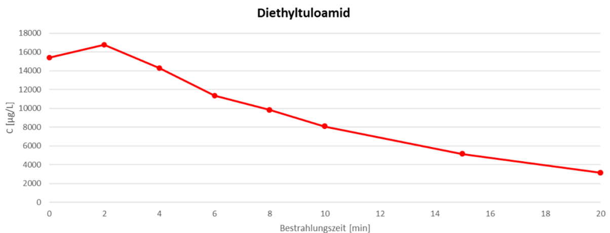
Abbildung 45: UV-unterstützter Abbau von Diethyltuloamid.
