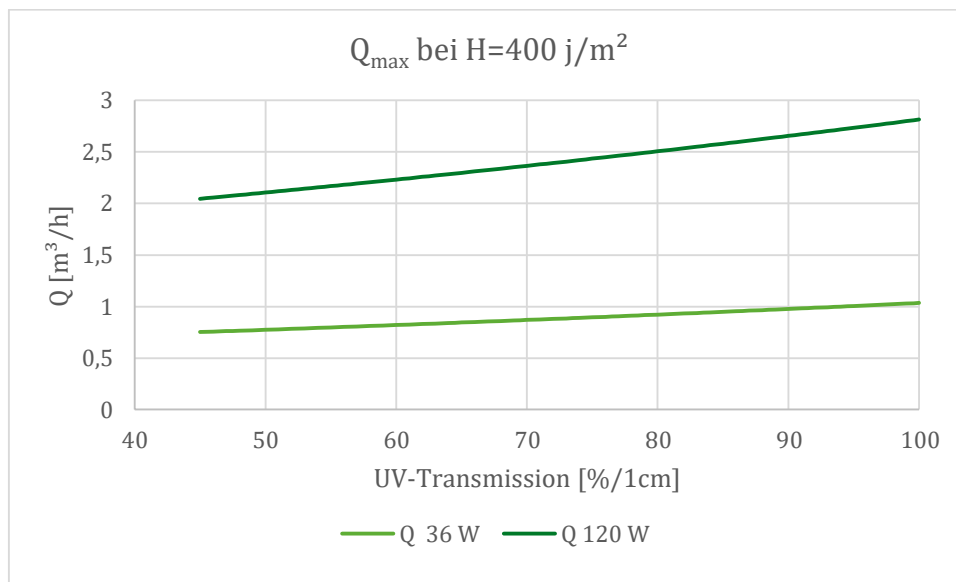
Abbildung 51: Maximale Volumenströme für unterschiedliche Strahlungsquellen in Abhängigkeit von der Transmission bei einer Keimreduzierung um 4-log-Stufen H=400 \text{ J/m}^2 .
