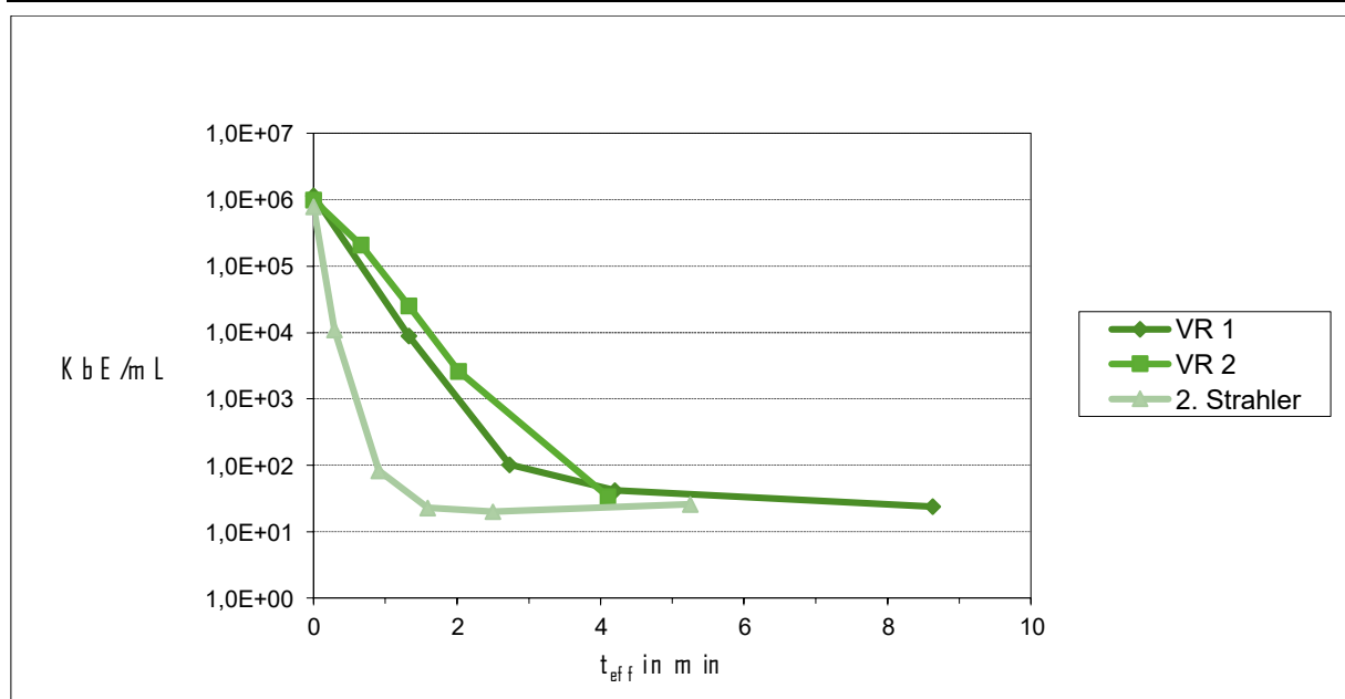
Abbildung 28: Vergleich unterschiedlicher Strahler hinsichtlich ihrer Effizienz bei der Keimreduzierung in Abhängigkeit von der Verweilzeit im Reaktor.
