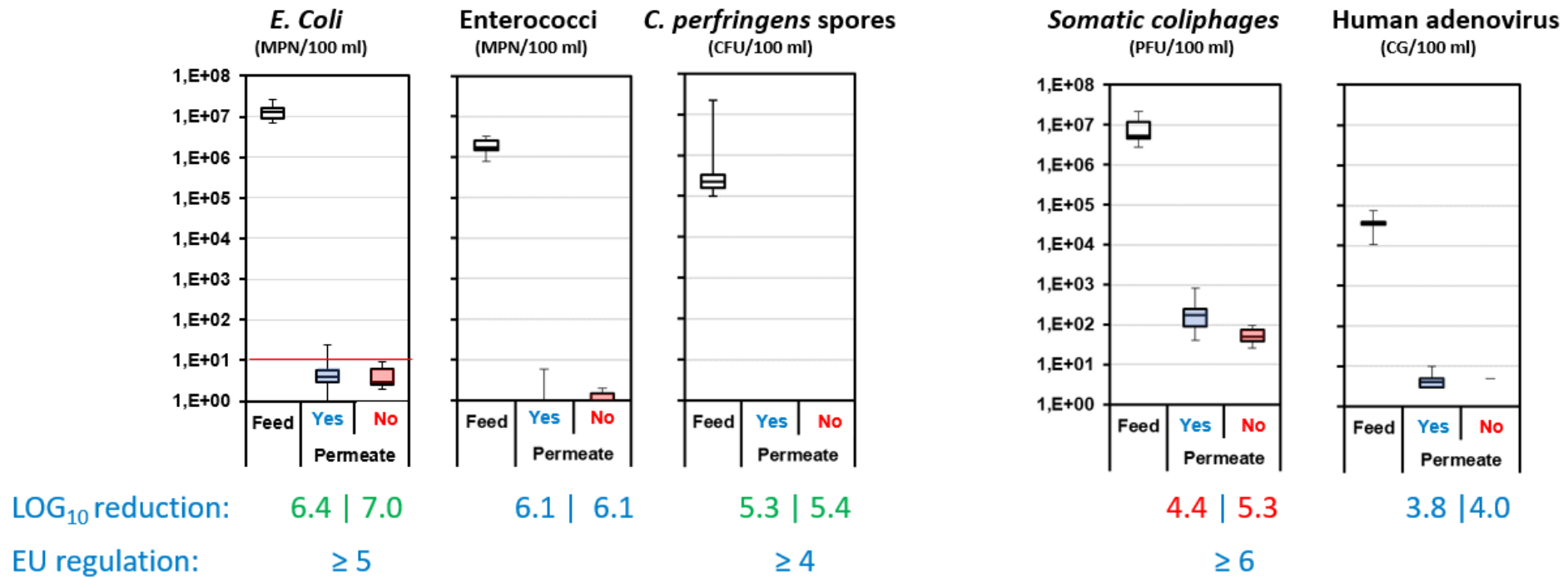
Abbildung 22: Konzentrationen von E. Coli (MPN/100 mL), Enterokokken (MPN/100 mL), C.-perfringens -Sporen (KBE/100 mL), somatischen Coliphagen (PFU/100 mL) und humanen Adenoviren (GC/10 mL) im MBR-Zulauf und Permeat beim Betrieb des kleinen Pilot-MBR mit Nitrifikation („Yes“) oder ausschließlicher Kohlenstoffelimination („No“).
