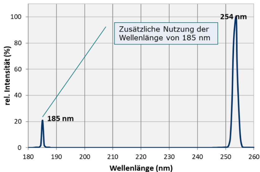
Abbildung 55: UV-Spektrum des UV-Strahlers mit 185 nm und 254 nm.
