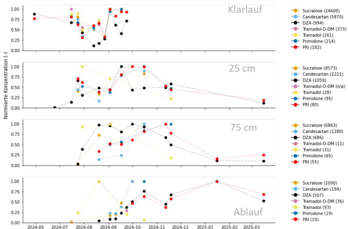
Abbildung 120: Transportdynamik ausgewählter Stoffe, die im Ablauf des Klarlauf-Lysimeters gemessen wurden. Die Ergebnisse wurden auf die im Versuchszeitraum maximale Konzentration der jeweiligen Probenahmestellen (Klarlauf, 25 cm, 75 cm, Ablauf) normiert, sodass der dargestellte Maximalwert 1 ist. Proben der Tiefen 25 und 75 cm wurden für einen Zeitpunkt gemittelt.
