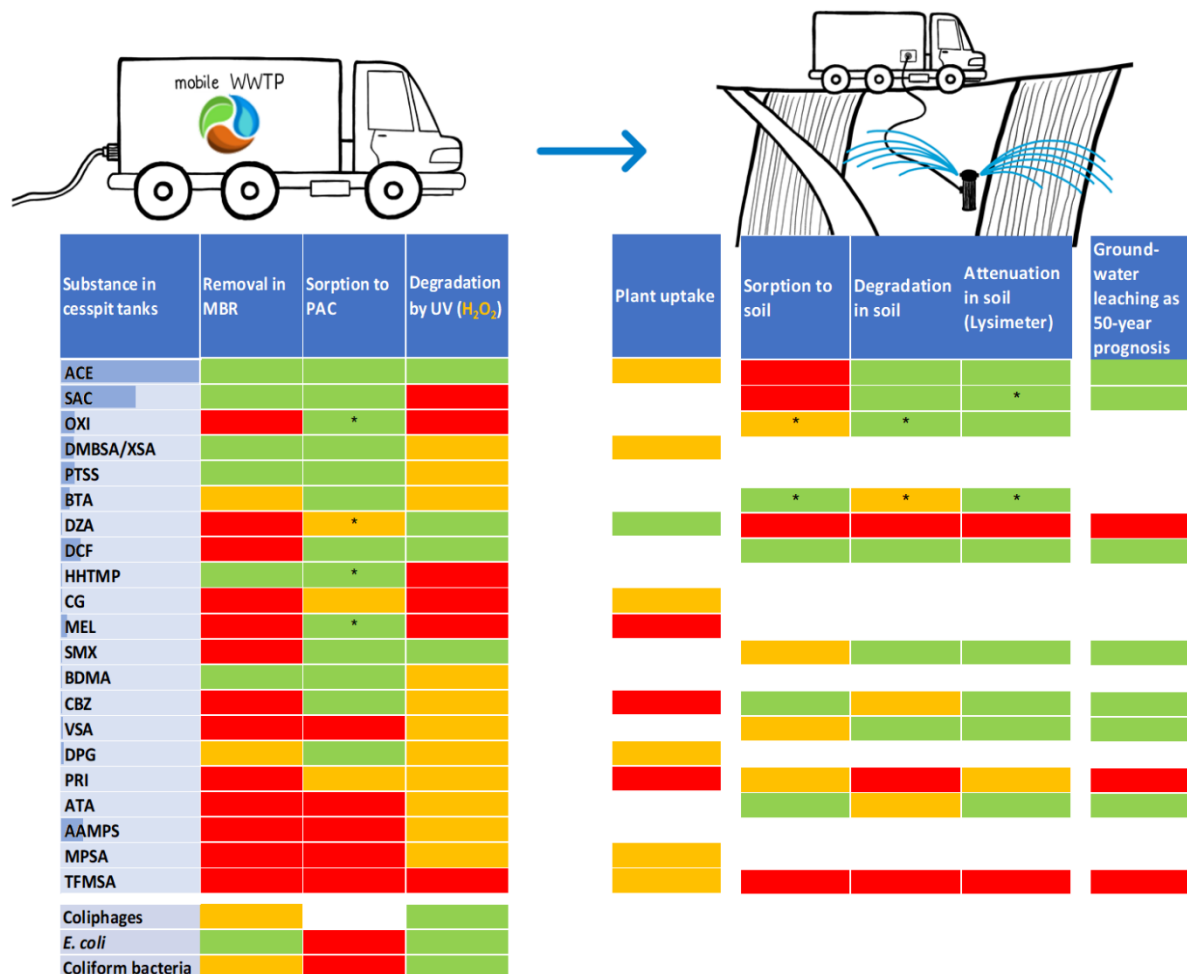
Abbildung 3: Multibarrieren-Prinzip für die PU 2 R-Prozesskette von der Abwasseraufbereitung über die Pfade Boden-Pflanze und Boden-Grundwasser. Qualitative Rückhalte der organischen Spurenstoffe und Mikroorganismen sind farbig kodiert (grün = gut, orange = mäßig, rot = schlecht). Balken in der ersten Spalte repräsentieren semi-quantitativ die Konzentration der Substanz, wie sie in den abflusslosen Sammelgruben detektiert wurden. Substanzen die nur durch Zugabe von H 2 O 2 mittels UV entfernt werden können sind gelb markiert. Bei der Pflanzenaufnahme steht rot für eine starke Aufnahme und grün für eine schwache Aufnahme.
