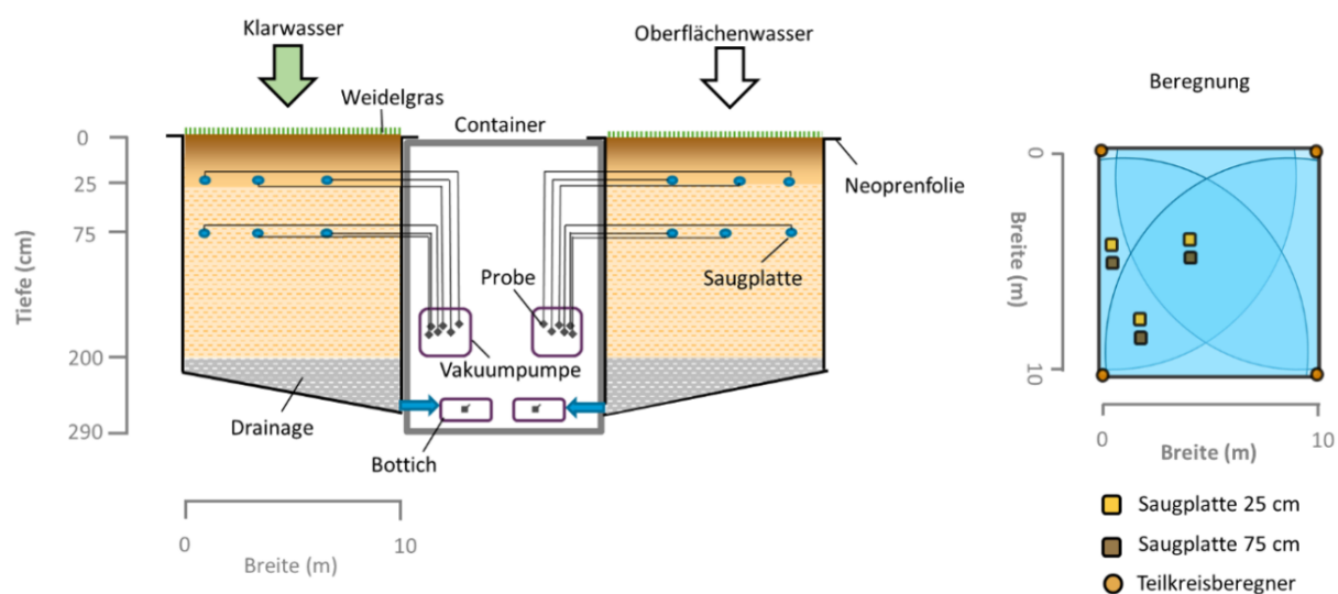
Abbildung 116: Skizze der zwei Versuchsanlage inklusive Probenahmestellen und Anordnung der Teilkreisberegner.
