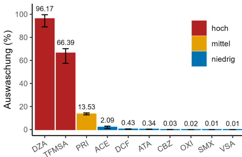
Abbildung 81: Auswaschung der 10 untersuchten PM-Stoffen.
