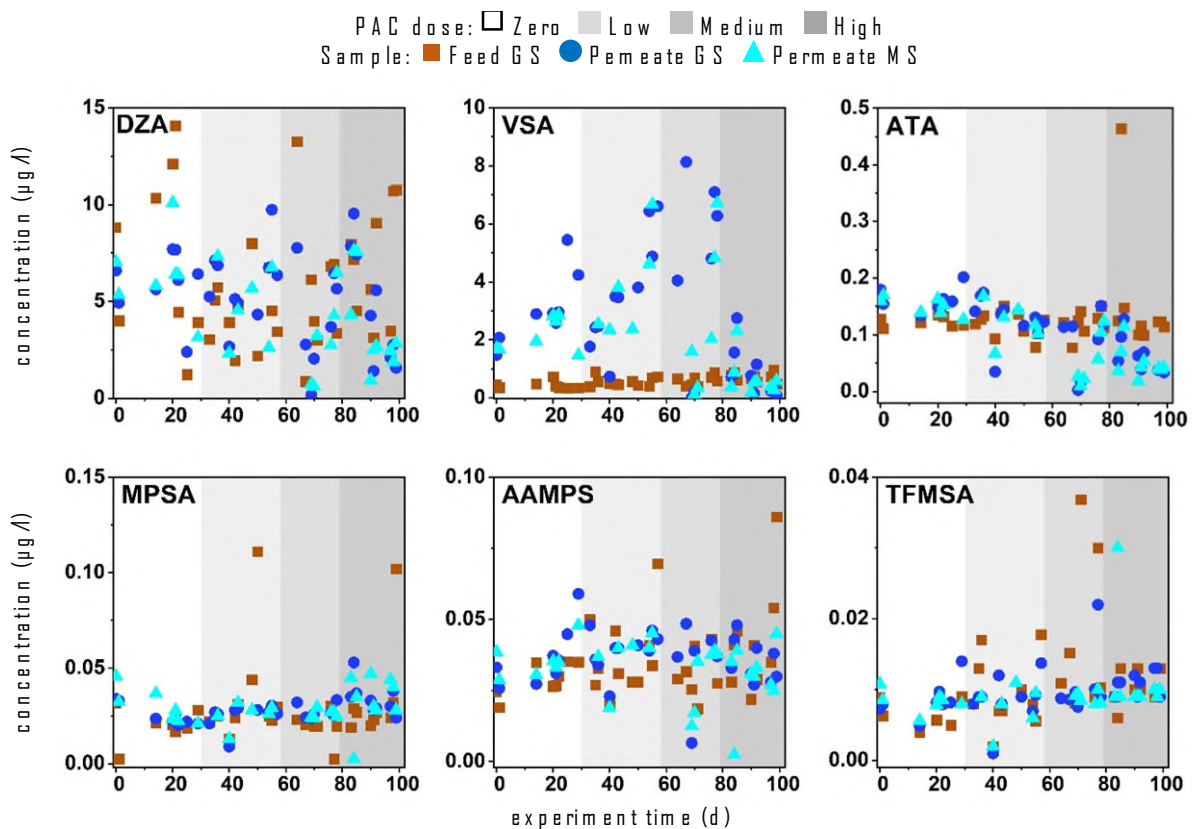
Abbildung 38: Feed- und Permeatkonzentrationen persistenter organischer Spurenstoffe (weißer Hintergrund für Betrieb ohne PAK, hellgrau für niedrige, grau für mittlere und dunkelgrau für hohe PAK-Dosen).
