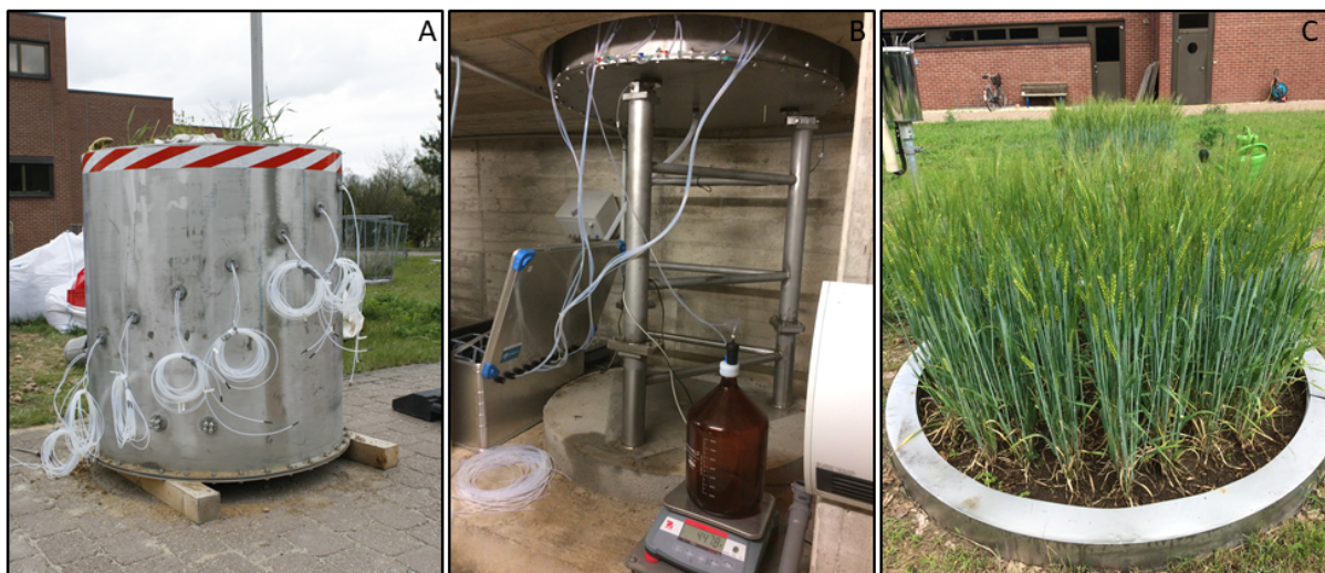
Abbildung 79: Fotosequenz zum Lysimeterversuch.
