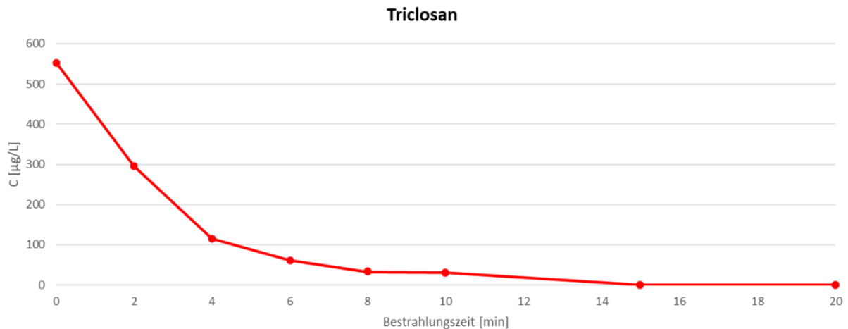
Abbildung 43: UV-unterstützter Abbau von Triclosan.
