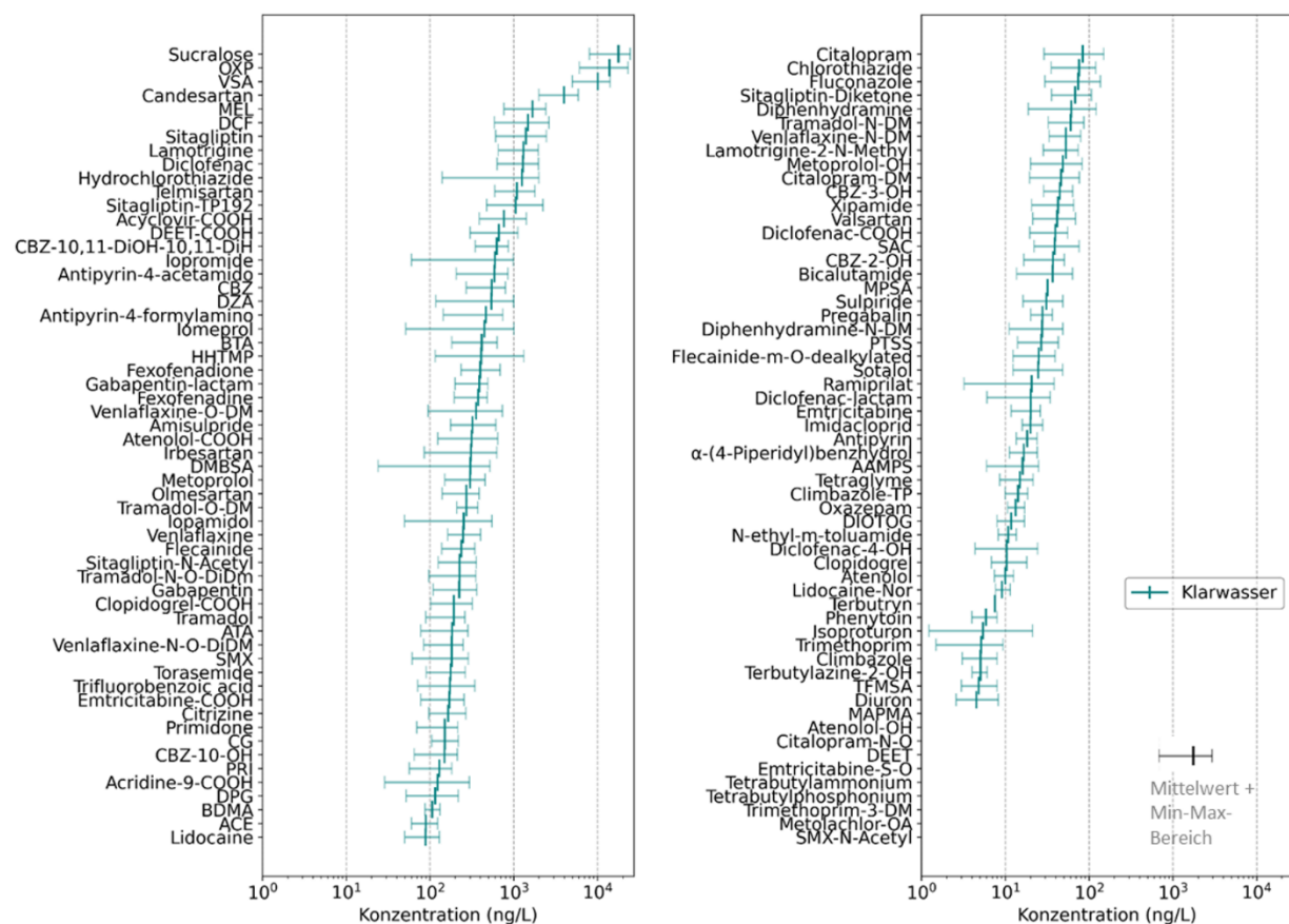
Abbildung 119: Darstellung der mittleren sowie minimalen und maximalen Konzentrationen der Target-Analyten im Klarlauf bezogen auf den Versuchszeitraum.
