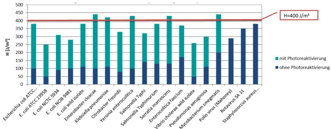
Abbildung 25: Untersuchungen zur Sicherheit des technischen Einsatzes von UV-Strahlern zur Trinkwasserdesinfektion. Aus Abschlussbericht 1994, Forschungsvorhaben gefördert durch das Bundesministerium für Forschung und Technologie 02• WT 9078.
