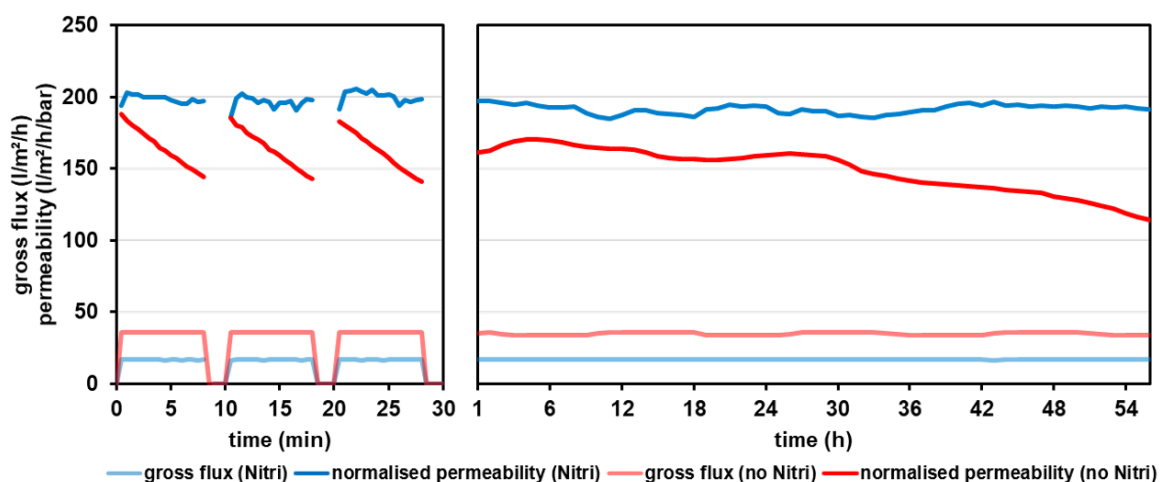
Abbildung 18: Brutto-Flux und Membranpermeabilität beim MBR-Betrieb mit Nitrifikation („Nitri“) bzw. ausschließlicher Kohlenstoffelimination („no Nitri“).
