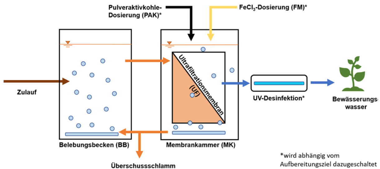
Abbildung 10: Verfahrensschema der großen MBR-Pilotanlage.
