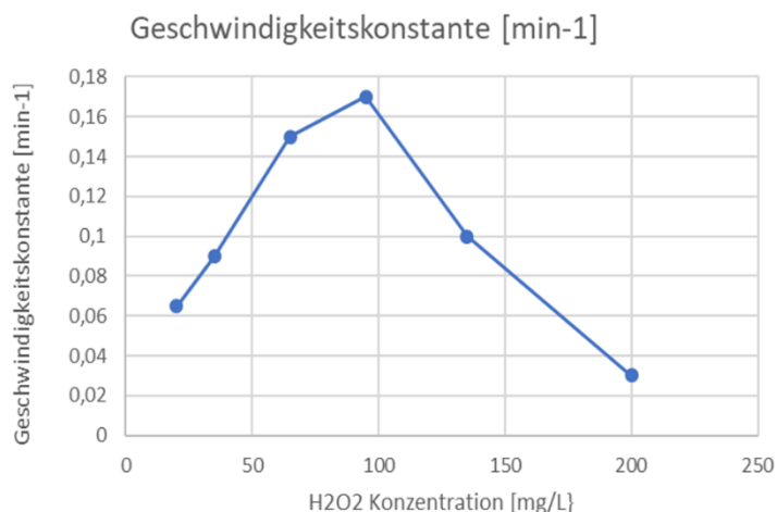
Abbildung 46: Abhängigkeit der Geschwindigkeitskonstanten von der Wasserstoffperoxidkonzentration für den Abbau eines Farbstoffs.
