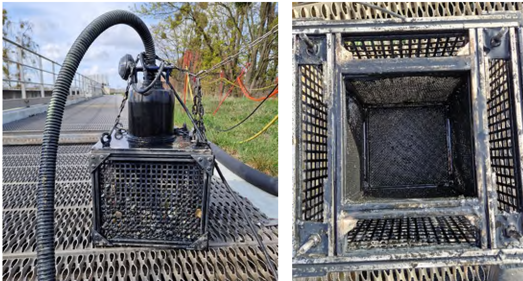
Abbildung 11: Feinsiebung des Zulaufs des großen Pilot-MBR an der Zulaufentnahmepumpe.
