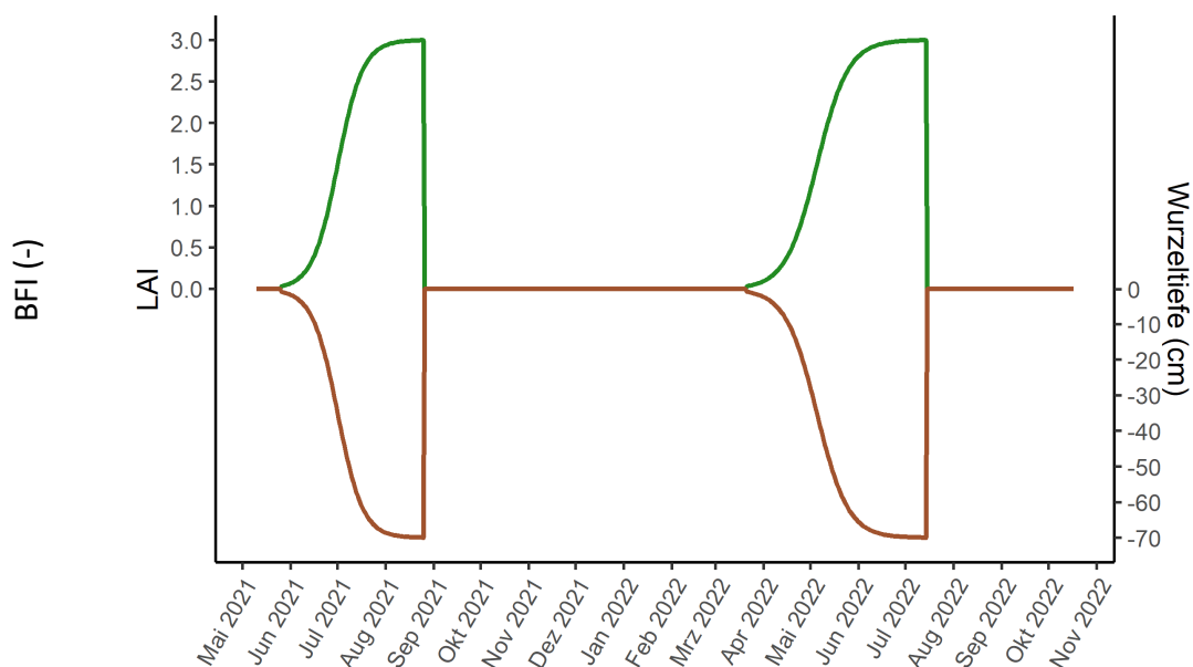
Abbildung 88: Zeitlicher Verlauf des BFI und der Wurzeltiefe für Sommerbraugerste in 2021 und 2022.
