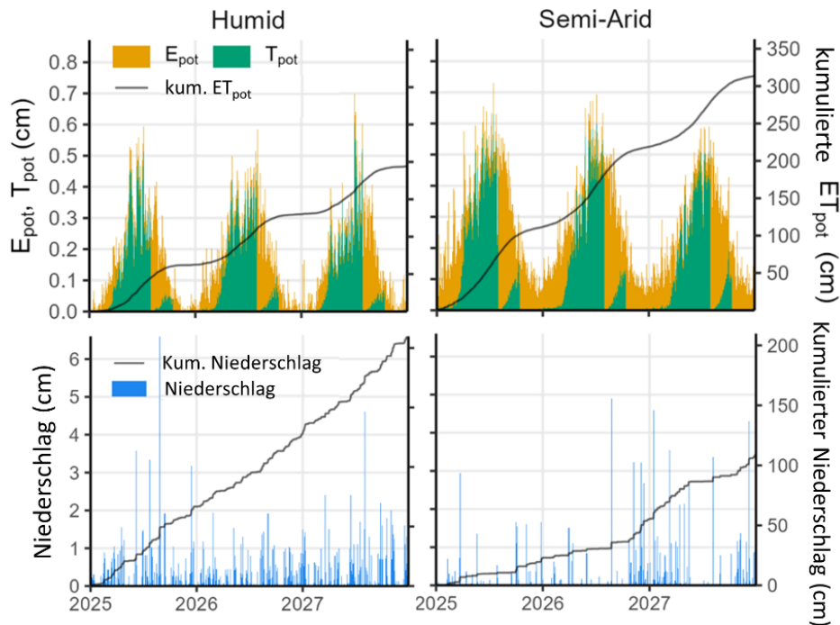
Abbildung 98: Tägliche (Balken) und kumulative (schwarze Linien) Werte für ET_{pot} und Niederschlag für die ersten drei Simulationsjahre für humides bzw. semi-arides Klima.
