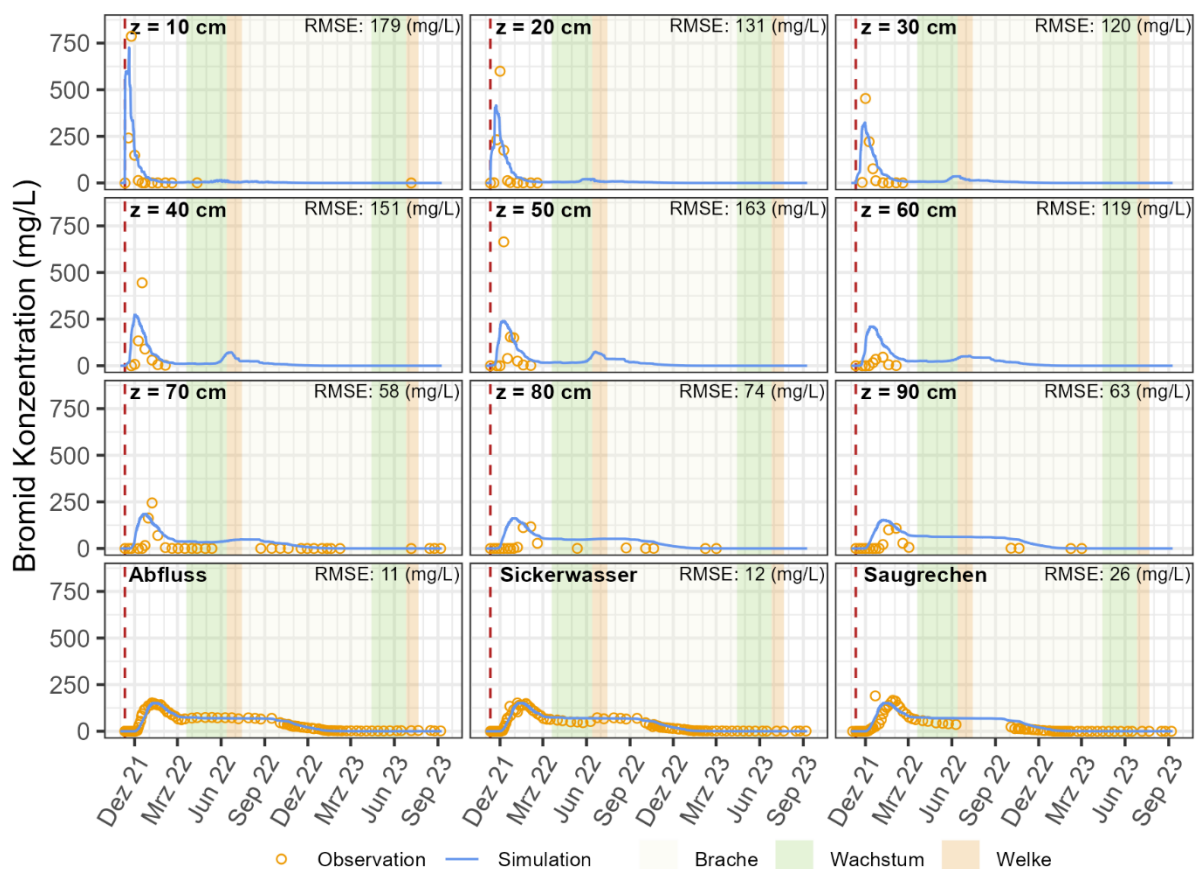
Abbildung 89: Vergleich der simulierten (blaue Linie) und beobachteten (orange Kreise) Bromid-Konzentrationen im gepackten Lysimeter 1.
