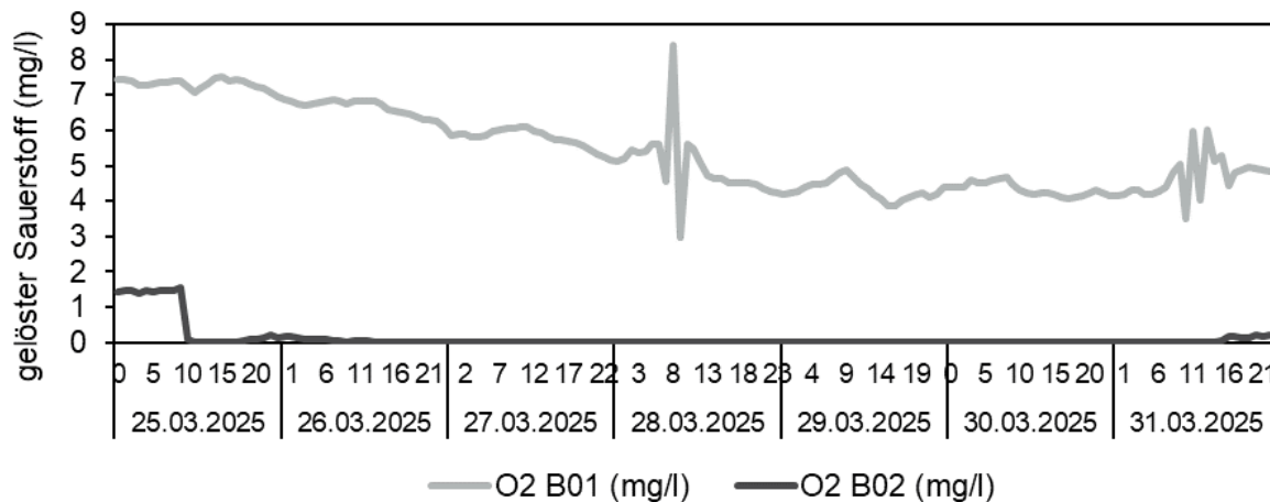
Abbildung 17: Sauerstoffkonzentration in der Membrankammer (B01) und im Belebungsbecken (B02) des großen Pilot-MBR.
