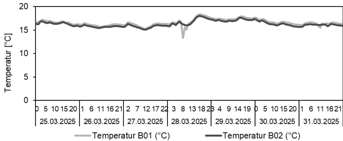
Abbildung 16: Temperatur in der Membrankammer (B01) und im Belebungsbecken (B02) des großen Pilot-MBR.
