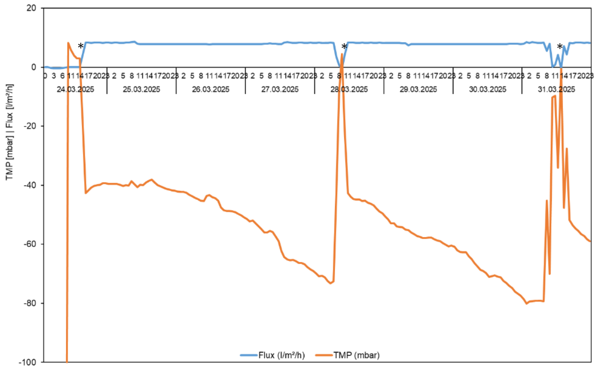
Abbildung 15: Transmembrandruck und Flux beim Betrieb des großen Pilot-MBR mit Denitrifikation (*: chemische Zwischenreinigungen).
