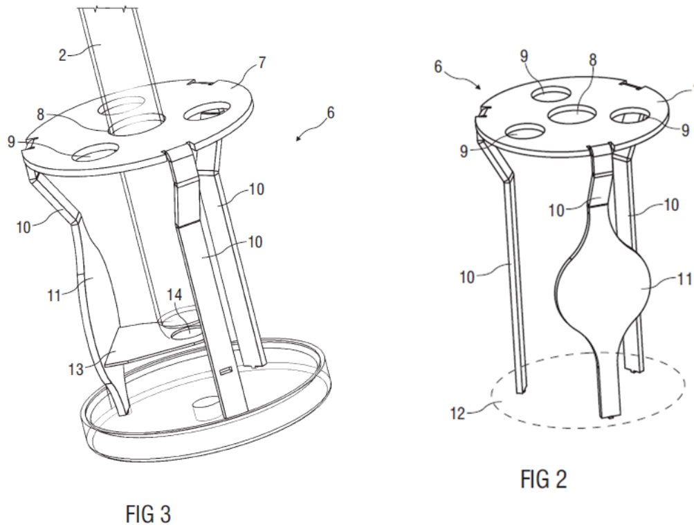
Abbildung 52: Gebrauchsmuster DE 20 2023 100 378 zur Gestaltung einer Lichtfalle im UV-Reaktor.
