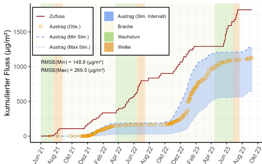
Abbildung 92: Kumulierter Zufluss von DZA und Vergleich des simulierten und beobachteten kumulativen Austrags mit dem Sickerwasser für das gepackte Lysimeter 1.
