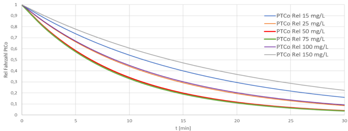
Abbildung 53: Vergleich der Reaktionsgeschwindigkeiten für unterschiedliche Wasserstoffperoxidkonzentrationen.
