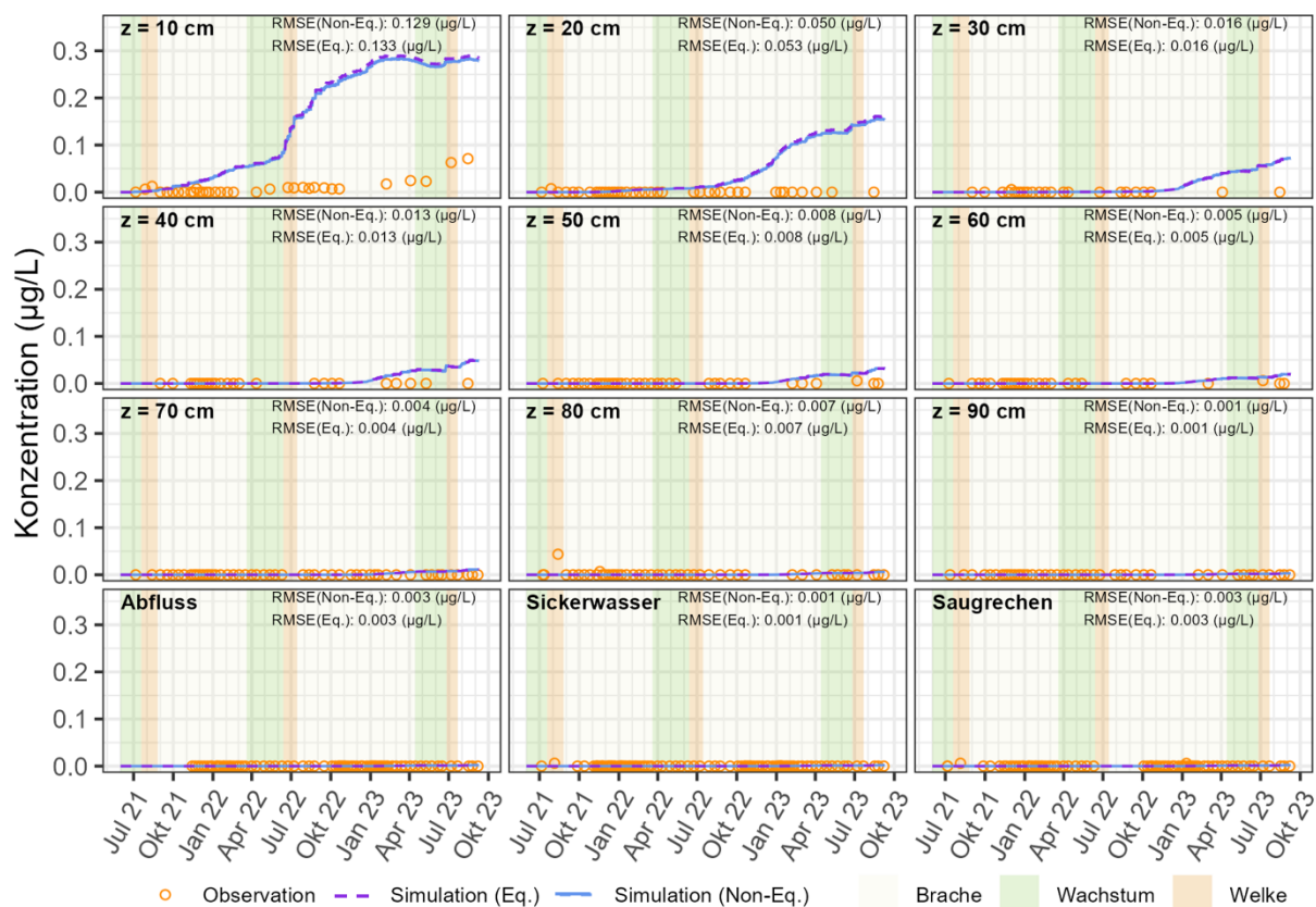
Abbildung 95: Vergleich des observierten und simulierten Transports von CBZ im gepackten Lysimeter 1.
