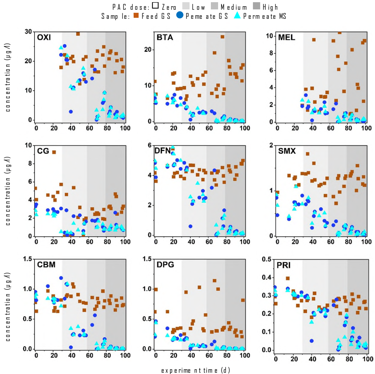
Abbildung 37: Feed- und Permeatkonzentrationen adsorbierbarer organischer Spurenstoffe (weißer Hintergrund für Betrieb ohne PAK, hellgrau für niedrige, grau für mittlere und dunkelgrau für hohe PAK-Dosen).
