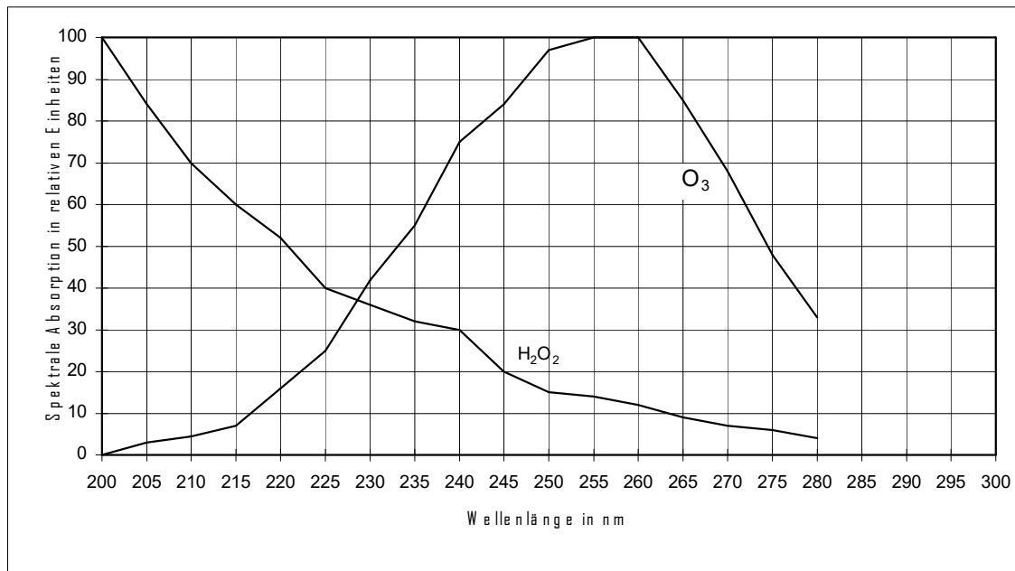
Abbildung 39: Normierte Absorptionsspektren von Wasserstoffperoxid und Ozon.
