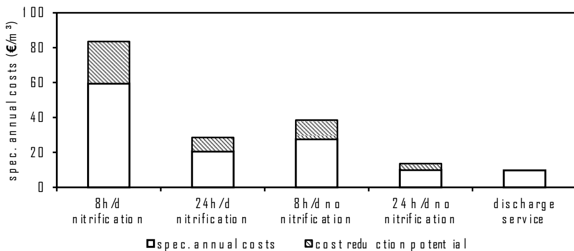
Abbildung 111: Vergleich der spezifischen Jahreskosten bezogen auf die gereinigte Abwassermenge (Die potenzielle Kostenreduktionen resultieren aus der Optimierung des Betriebs von 250 d/a zu 354 d/a)
