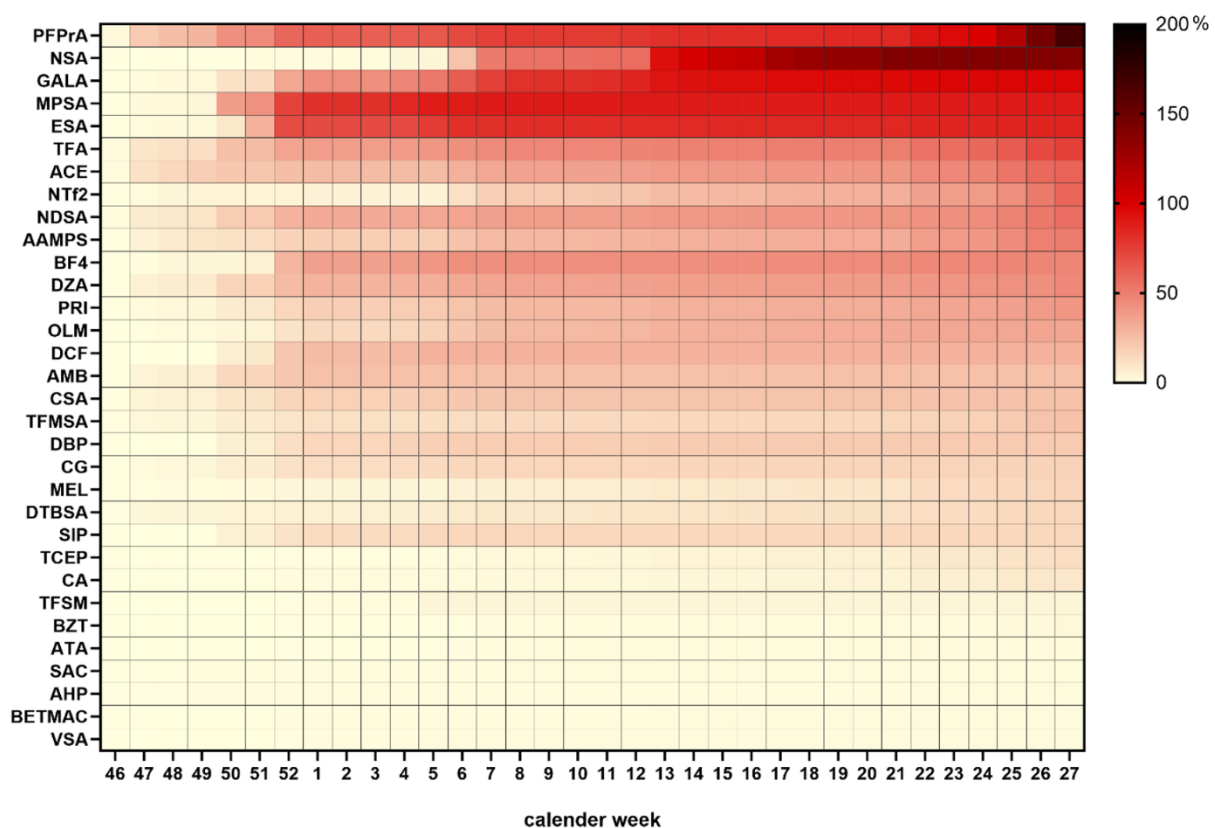
Abbildung 65: Kumulierter Fluss an PM-Stoffen im Ablauf der Testsäulen (60 cm) über den Betriebszeitraum. PM-Stoffe mit einem gesamten prozentualen Anteil von < 1% sind aus der Grafik ausgenommen. Die Abkürzungen der PM-Stoffe können dem Abkürzungsverzeichnis entnommen werden.
