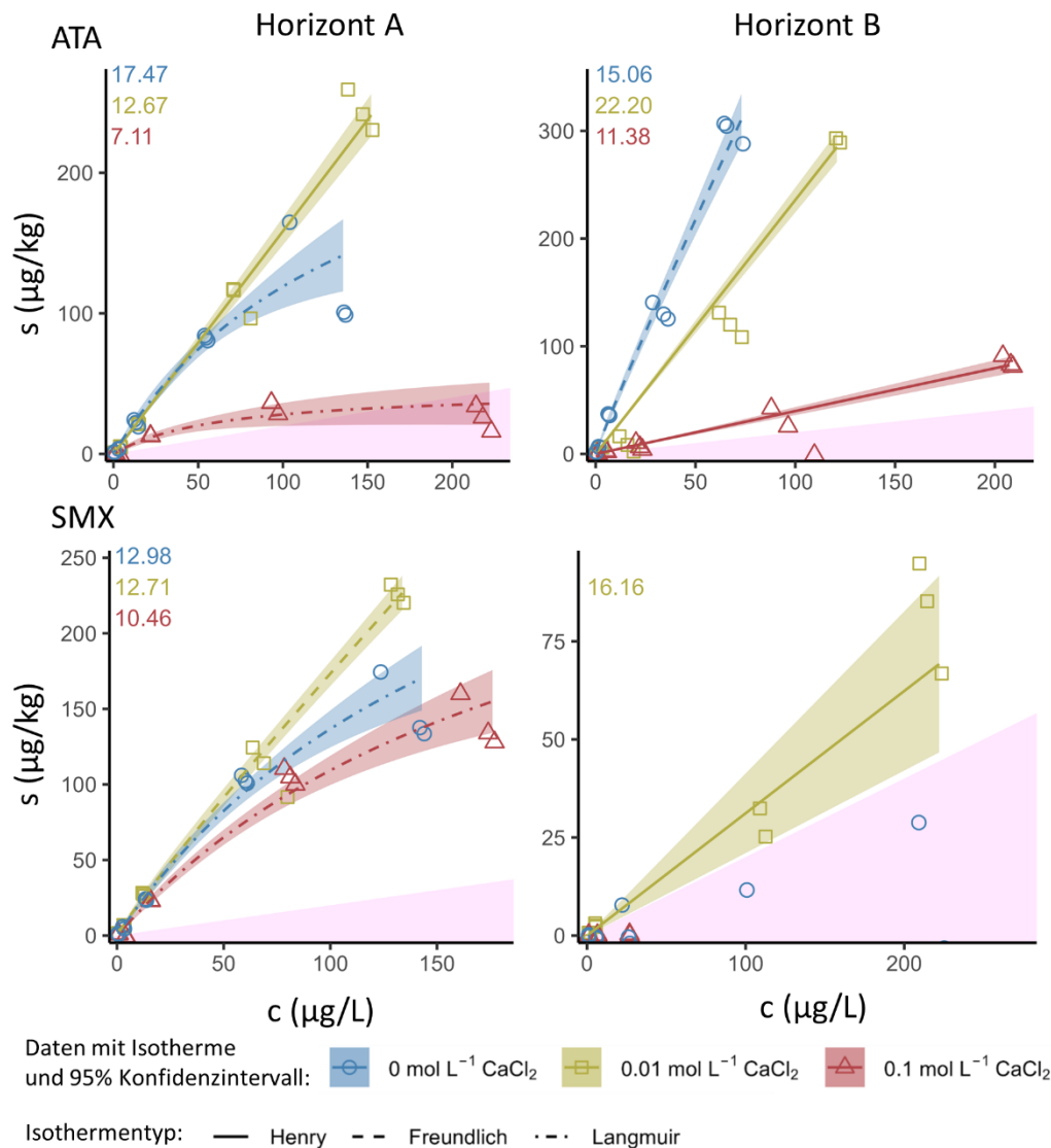
Abbildung 70: Einfluss der Ionenstärke auf die ATA- und SMX-Sorption.
