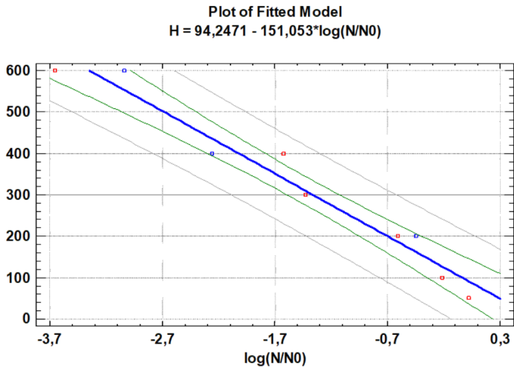
Abbildung 26: Kalibrierkurve für Sporen von Bacillus subtilis unter UV-Bestrahlung bei 253,7 nm.
