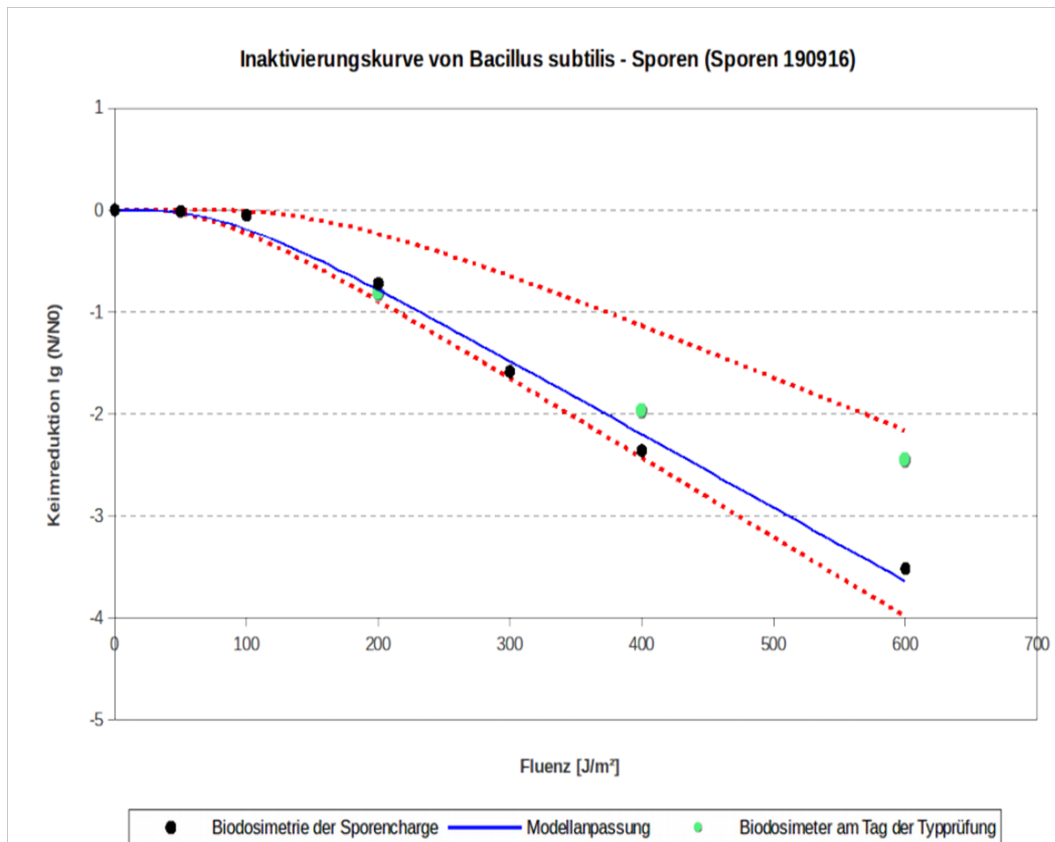
Abbildung 27: Abhängigkeit der möglichen Keimreduktion von der Fluenz.
