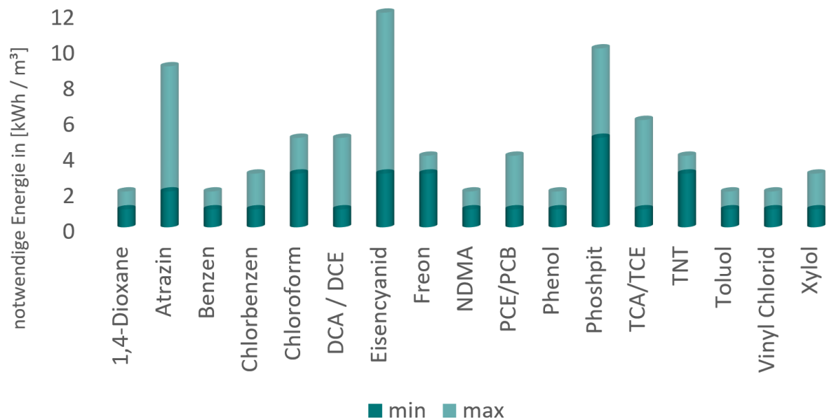
Abbildung 40: Beispiele für die notwendige elektrische Energie in KWh je m³ für 90 % Reduzierung (abhängig von der Ausgangskonzentration).
