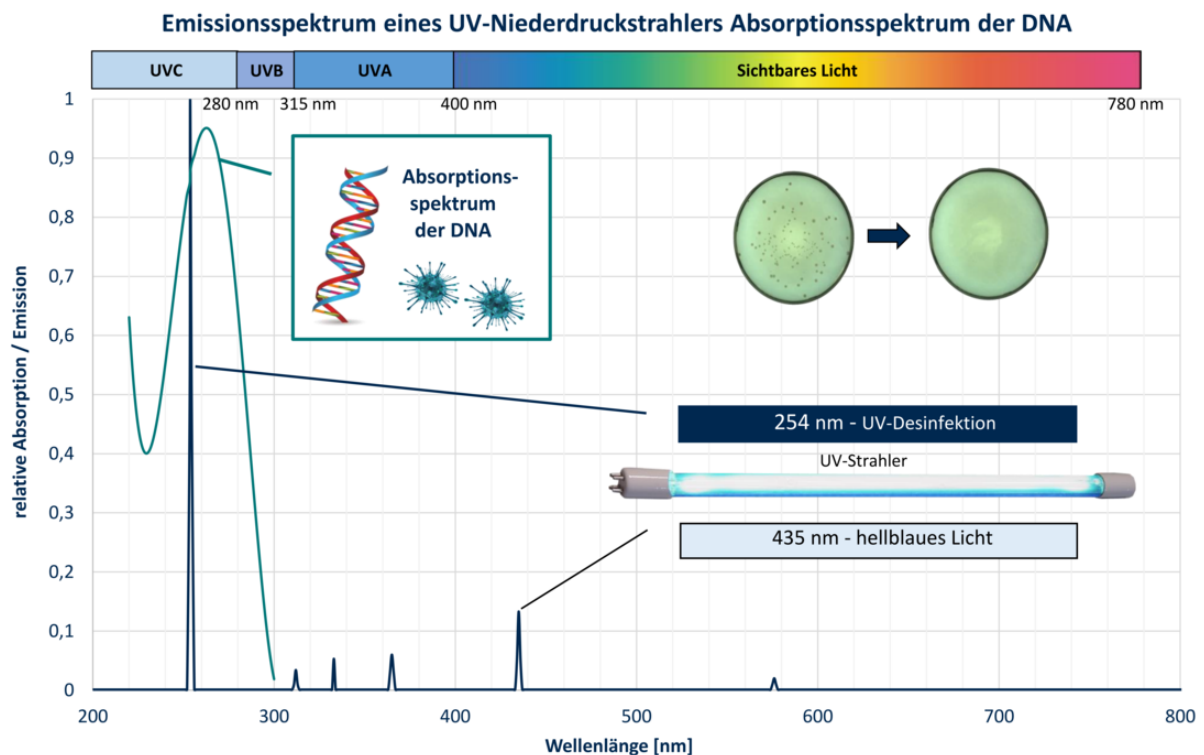
Abbildung 24: Emissions- und Absorptionsspektren für die Zellinaktivierung.
