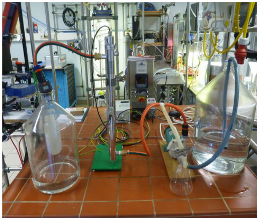
Abbildung 49: Laboraufbau mit Kreislauf zur Untersuchung des UV-unterstützten Abbaus von organischen Problemstoffen und zur biosimetrischen Untersuchung.
