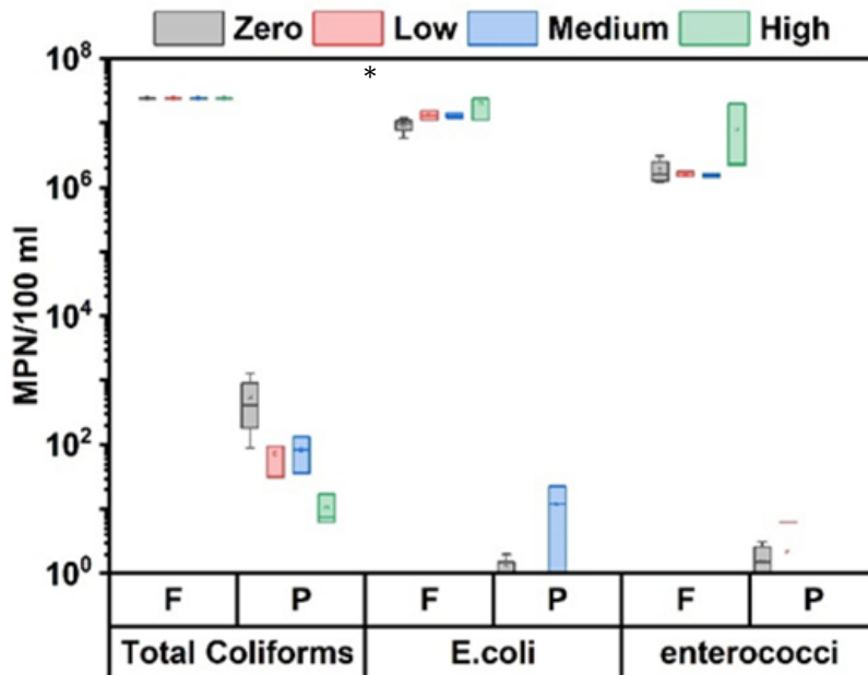
Abbildung 23: Konzentrationen von gesamtcoliformen Bakterien, E. coli und Enterokokken im MBR-Zulauf (F) und Permeat (P) ohne und mit Zugabe von Pulveraktivkohle (*: Messwerte über der oberen Bestimmungsgrenze 2,4 \cdot 10^7 MPN/100 mL).
