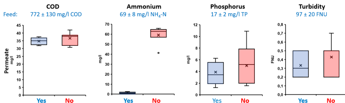
Abbildung 19: Permeatqualität beim MBR-Betrieb mit Nitrifikation („Yes“) bzw. ausschließlicher Kohlenstoffelimination („No“).
