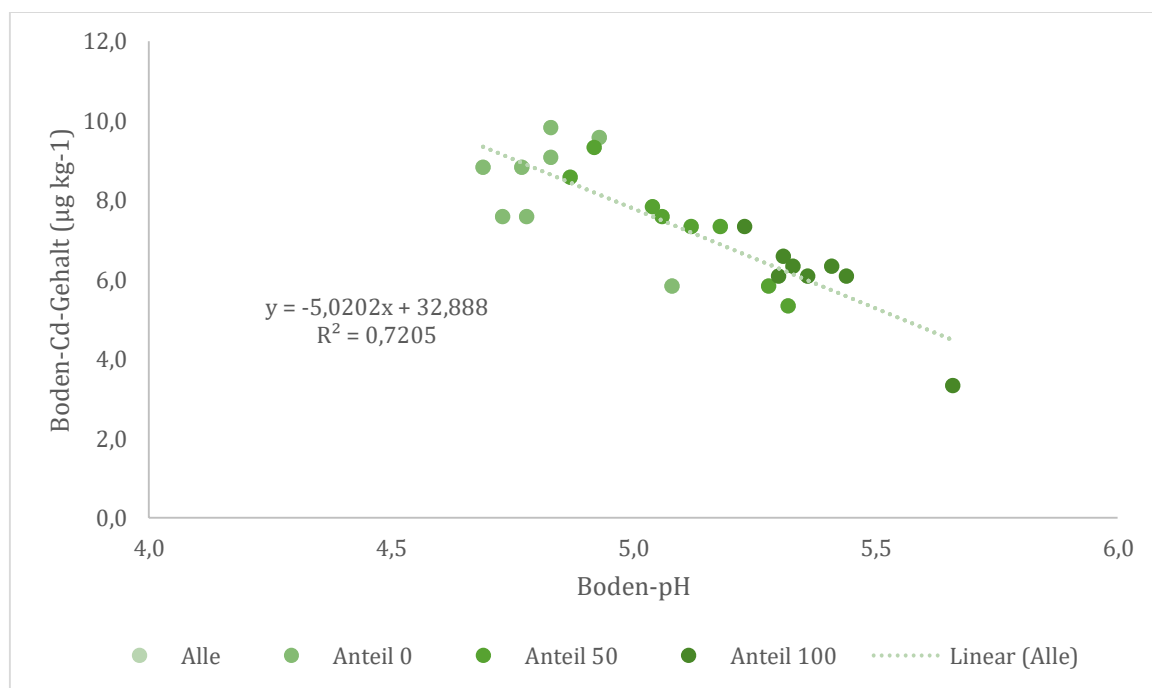
Abbildung 59: Beziehung zwischen dem pH-Wert und dem Gehalt an \text{NH}_4\text{NO}_3 -löslichen Cd im Boden bei Rucola; die Symbole stellen die Messwerte der 24 Gefäße mit Ackerboden (3 Klarwasseranteile x 2 Bewässerungsarten x 4 Wiederholungen) dar.
