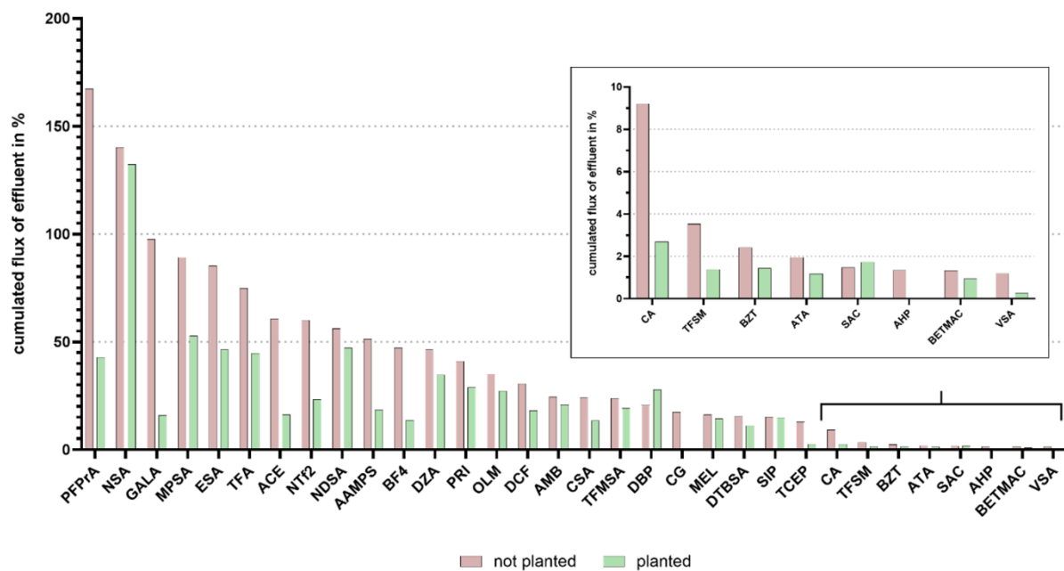
Abbildung 66: Kumulierte Fracht an PM-Stoffen im Ablauf der Lysimeter (60 cm) über die Betriebszeit von 9 Monaten bezogen auf die kumulierte Fracht im Zulauf in %, für bepflanzte (grün) und nicht-bepflanzte (rot) Lysimeter.
