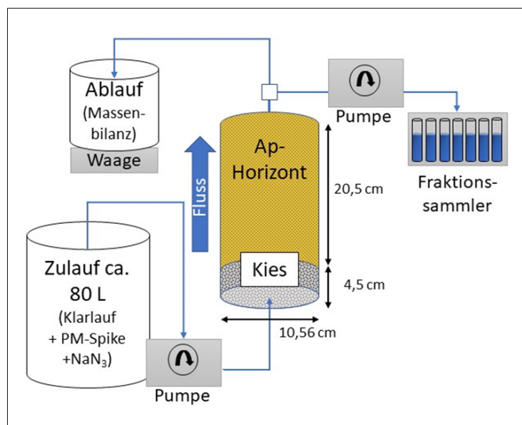
Abbildung 76: Schematischer Aufbau der Säulen und des Versuchsstands.
