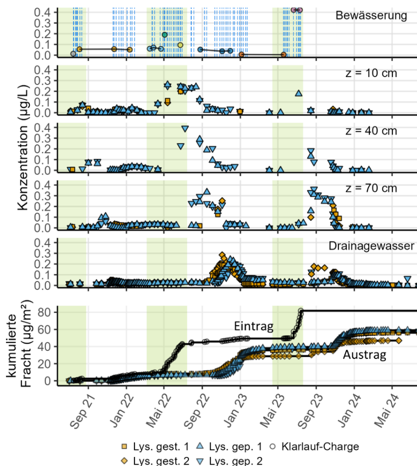
Abbildung 83: Zeitreihen der TFMSA -Konzentration verschiedener Tiefen und der kumulierten Grenzfrachten.
