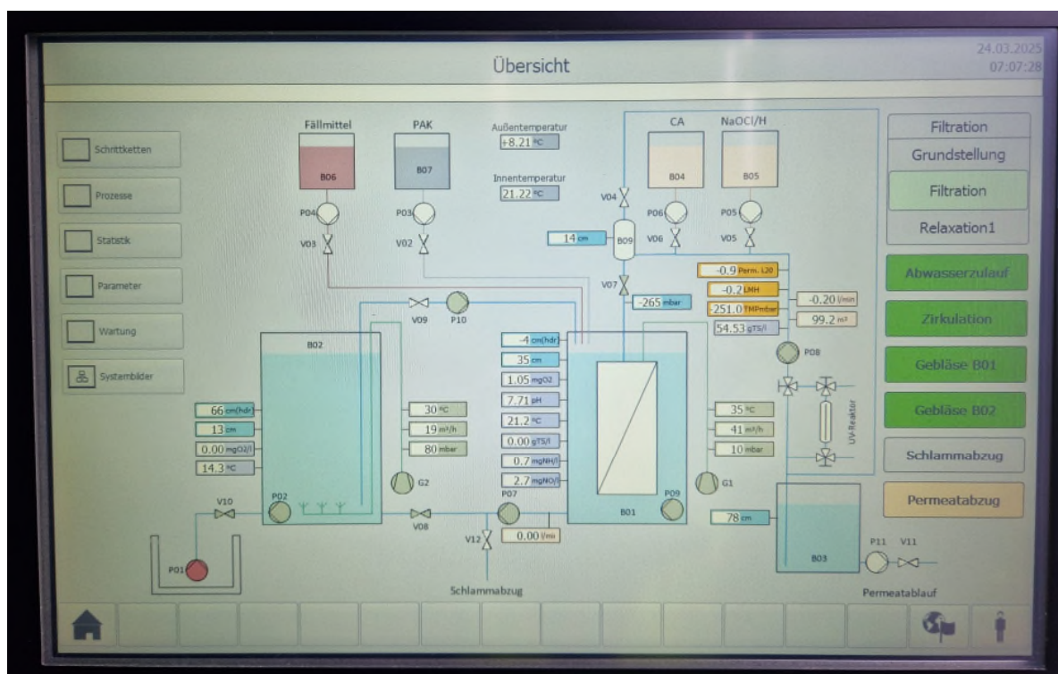
Abbildung 12: Frontpanel der Bedienoberfläche des großen Pilot-MBR.
