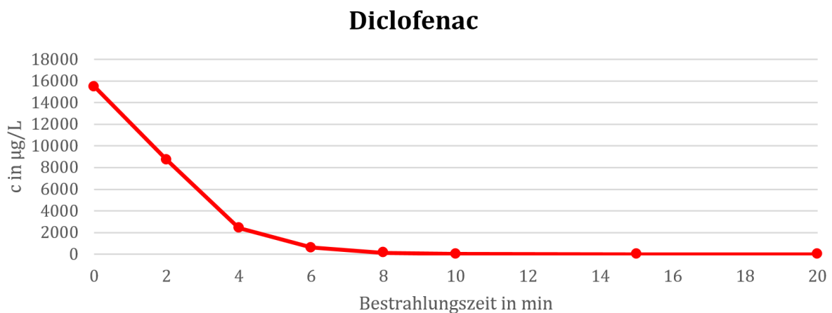
Abbildung 42: UV-unterstützter Abbau von Diclofenac.
