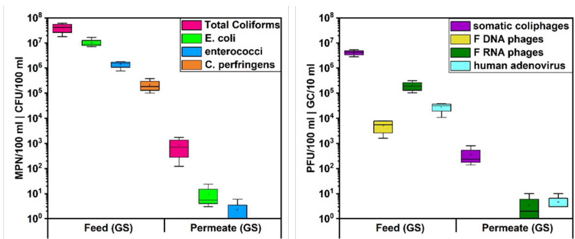
Abbildung 21: Konzentrationen von gesamtcoliformen Bakterien (MPN/100 mL), E. coli (MPN/100 mL), Enterokokken (MPN/100 mL), C.-perfringens -Sporen (KBE/100 mL), somatischen Coliphagen (PFU/100 mL), F-spezifischen DNA-Bakteriophagen (PFU/100 mL), F-spezifischen RNA-Bakteriophagen (PFU/100 mL) und humanen Adenoviren (GC/10 mL) im Zulauf und Permeat des kleinen Pilot-MBR ohne PAK (n = 4)
