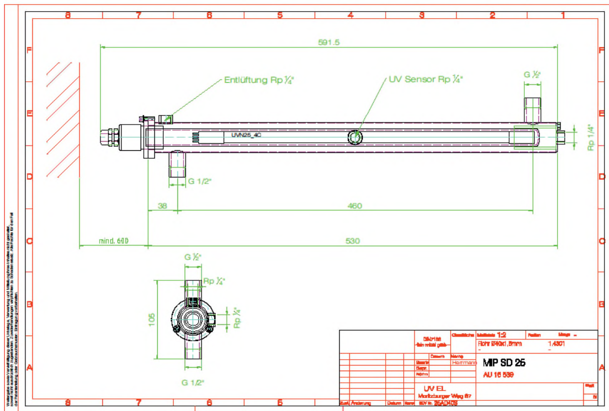
Abbildung 48: Skizze des verwendeten UV-Reaktors für die Laborversuche.
