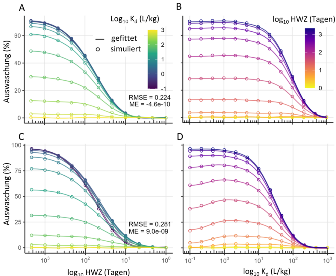
Abbildung 102: Die simulierte Auswaschung als Funktion von Halbwertszeit und K_d .
