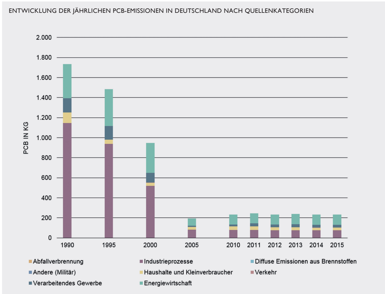
ABBILDUNG 2 Entwicklung der jährlichen PCB-Emissionen in Deutschland nach Quellkategorien. Quelle: UBA 2017.
