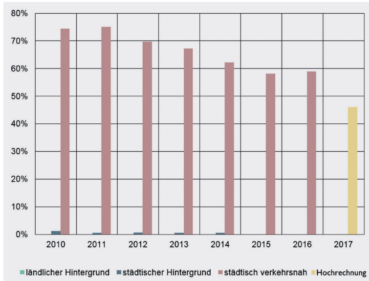
ABBILDUNG 3 Messstationen mit Überschreitung des Grenzwertes für das NO 2 -Jahresmittel im jeweiligen Belastungs- regime. Quelle: UBA 2018.
