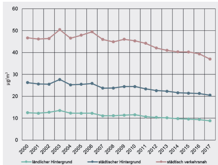
ABBILDUNG 5 Entwicklung der \text{NO}_2 -Jahresmittelwerte im Mittel über ausgewählte Messstationen im jeweiligen Belastungsregime. Quelle: UBA 2018.
