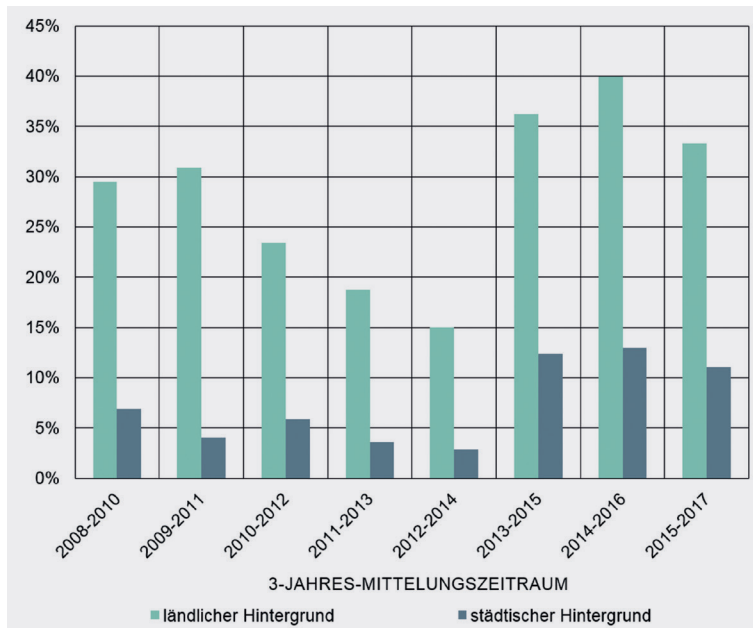
ABBILDUNG 6 Messstationen mit Überschreitung des Ozon-Zielwertes für den Schutz der Gesundheit. Quelle: UBA 2018.
