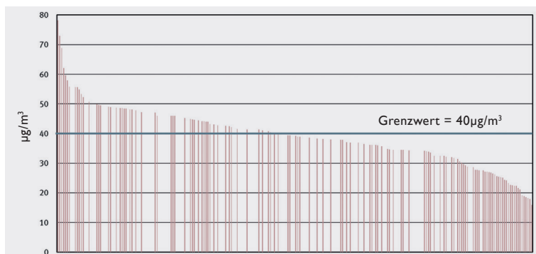
ABBILDUNG 4 NO 2 -Jahresmittelwerte 2017 aller verkehrsnahen Messstationen. Quelle: UBA 2018.
