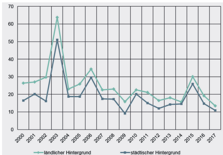
ABBILDUNG 7 Überschreitungstage des langfristigen Ozon-Zieles (höchster täglicher 8-Stunden-Mittelwert: 120 µg/m³). Mittelwert über ausgewählte Stationen. Quelle: UBA 2018.
