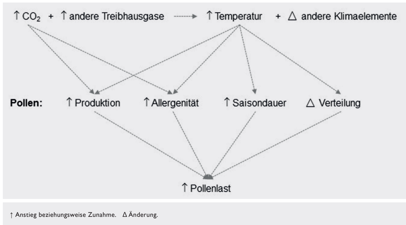
ABBILDUNG 2 Möglicher Einfluss von erhöhter CO 2 -Konzentration und erhöhter Temperatur auf das Pollen-System. Modifiziert nach Beggs (2004) und Behrendt, Ring (2012), siehe auch Höflich (2014).
