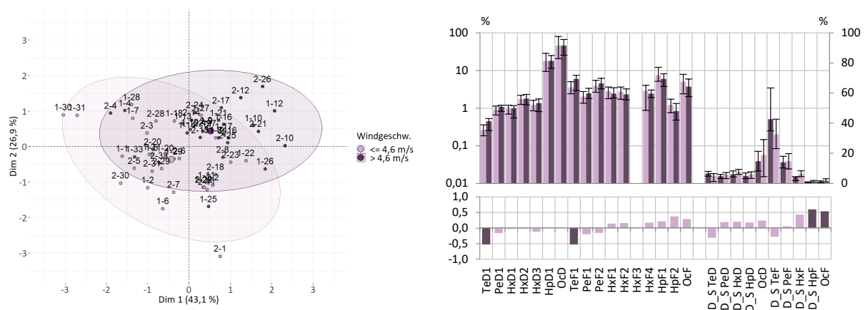
Abbildung 71: Windgeschwindigkeit – niedrig vs. hoch: Scoreplot (links) und Vergleich der mittleren Massenschlussprofile (rechts) mit den paarweisen komponentenspezifischen Abweichungen ( \Delta In-Anteile) zwischen den Profilen und die (mittleren) Aitchison-Distanzen
