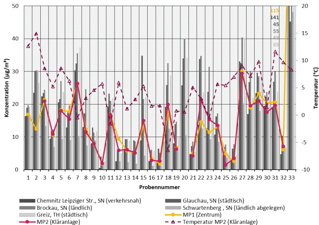
Abbildung 37: PM10-Konzentrationen ( \mu\text{g}/\text{m}^3 ) in den Kurzzeit(Wochenend)proben an MP1 (Zentrum) und MP2 (Kläranlage) im Vergleich zu Werten behördlicher Messtationen im gleichen Probenahmezeitraum
