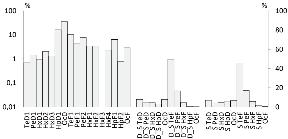
Abbildung 14: Beispiel für die in diesem Bericht allgemeine Darstellung der Massenschlussprofile zzgl. der Homologengruppensummenprofile (vollständige Summen) der PCDD/F
