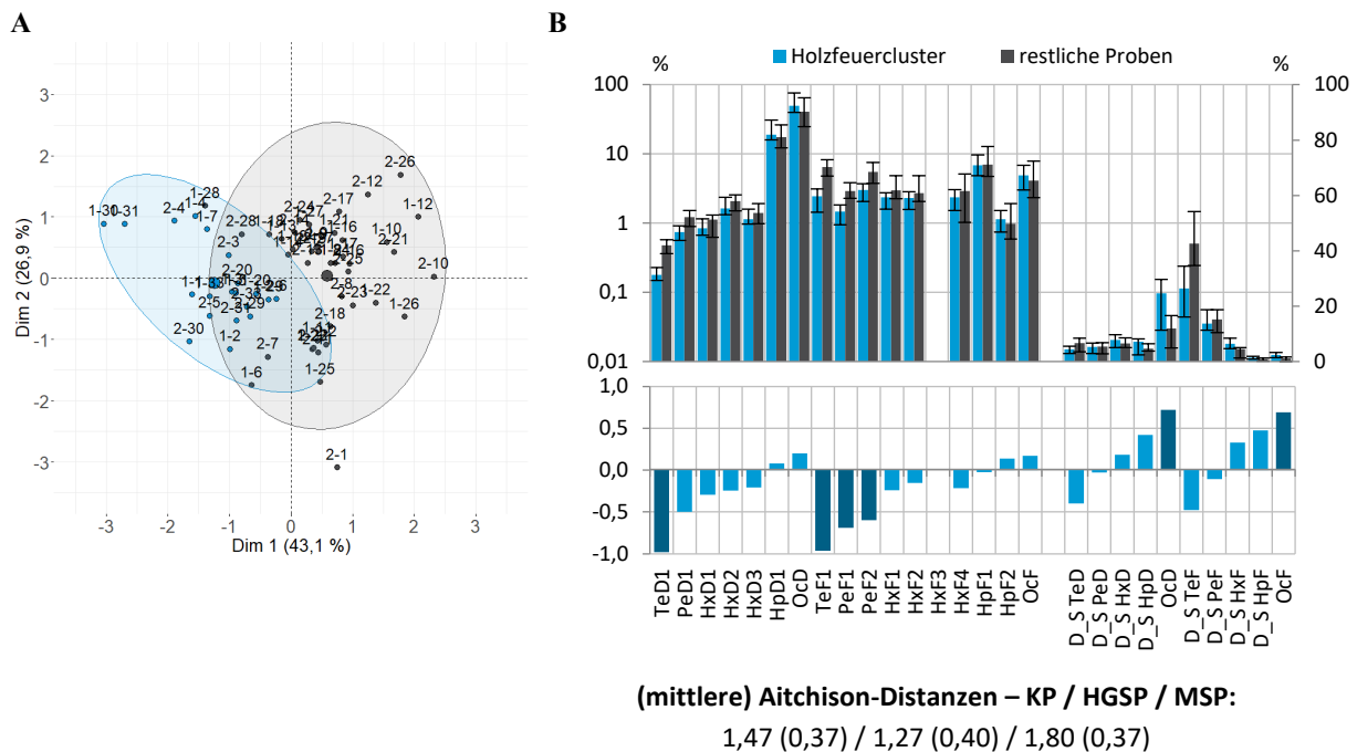
Abbildung 64: PCDD/F-Einzeldaten – Vergleich der Proben des Holzfeuerclusters mit den übrigen Proben: Scoreplot (A) und Vergleich der mittleren Massenschlussprofile (B) mit den paarweisen komponentenspezifischen Abweichungen ( \Delta In-Anteile) zwischen den Profilen und die (mittleren) Aitchison-Distanzen
