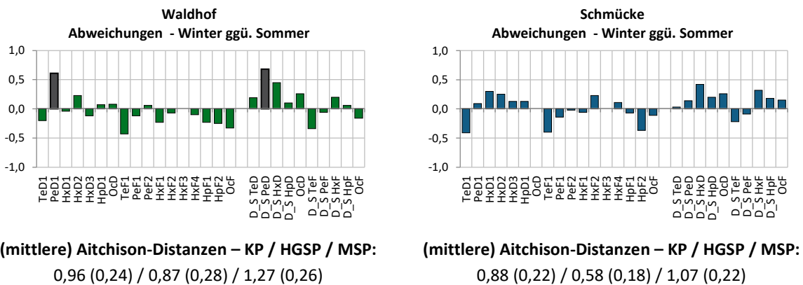
Abbildung 61: PCDD/F-Komponenten-spezifische Abweichungen ( \Delta In-Anteile) zwischen Winter und Sommermonaten und (mittlere) Aitchison-Distanzen zwischen den Winter- und Sommerprofilen
