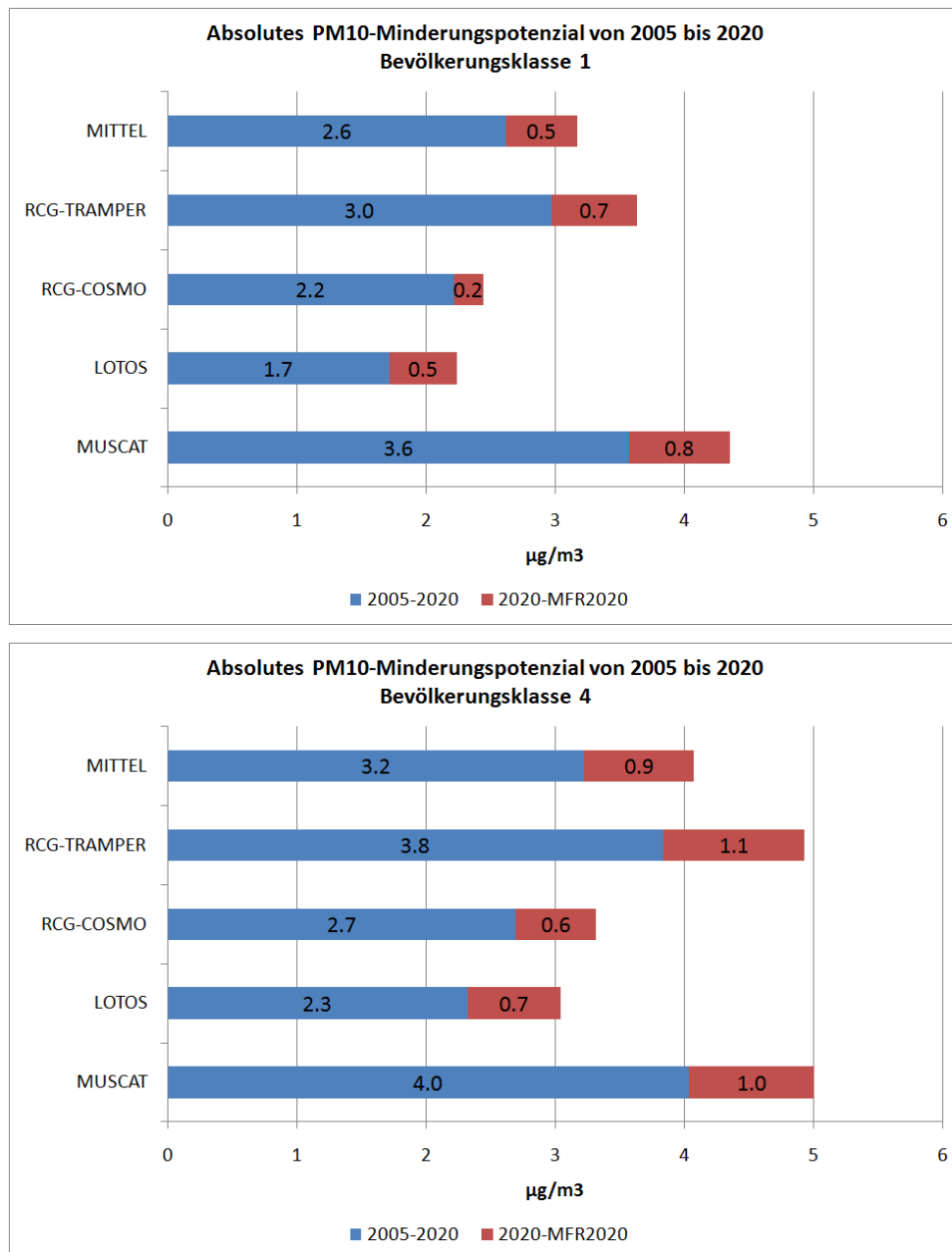
Abbildung 5-15 Absolute Abnahmen der PM10-Jahresmittelwerte, die aufgrund der Emissionsentwicklung 2005 bis 2020 (CLE-Referenzszenario) und dem zusätzlichen MFR-Szenario 2020 erreicht werden können. Mittlere bevölkerungsgewichtete Auswertung für ländliche Regionen (Bevölkerungsklasse 1) und Ballungsgebiete (Bevölkerungsklasse 4). Mittel: Mittelwert des Minderungspotenzials berechnet aus den Einzelergebnissen der 4 Modellanwendungen.
