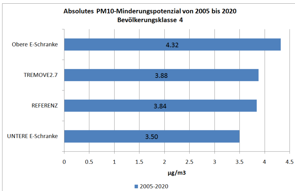
Abbildung 4-1 Absolute PM10-Immissionsminderungen in \mu\text{g}/\text{m}^3 , die aufgrund der Emissionsentwicklung 2005 bis 2020 erreicht werden können. Mittlere Emissionsreferenz, obere und untere Schranken der Emission sowie mittlere Emissionsreferenz mit der Berechnung der Verkehrsemissionen nach TREMOVE2.7. Oben: Mittlere Auswertung für Bevölkerungsklasse 1, unten für Bevölkerungsklasse 4.
