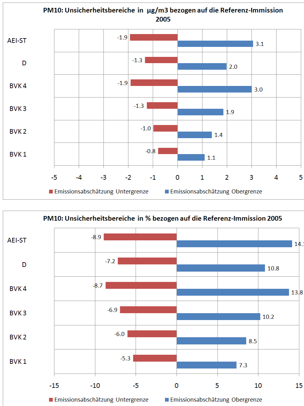
Abbildung 3-4 Absolute (oben) und relative (unten) Unsicherheitsbereiche der PM10-Jahresmittelwerte abgeleitet aus den Ober- und Unterschranken der Emissionsreferenz 2005. Mittlere bevölkerungsgewichtete Auswertung für die 6 Bewertungsklassen. Zur Definition der Klassen siehe Kapitel 2.
