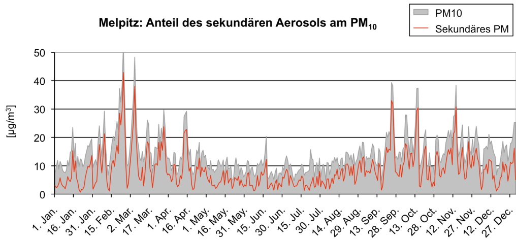
Abb. 5.7: Zeitreihen berechneten und gemessenen Tagesmittelwerte [µg/m³] an der Stationen Melpitz für die sekundär gebildete Partikelmasse.
