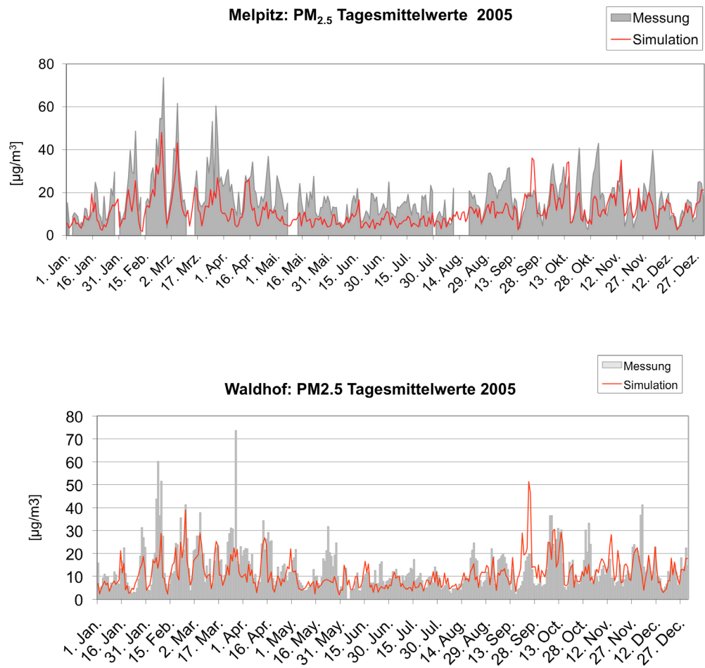
Abb. 5.5: Zeitreihen der berechneten und gemessenen PM_{2.5} -Tagesmittelwerte [ \mu g/m^3 ] an den Stationen Melpitz (oben) und Waldhof (unten).
