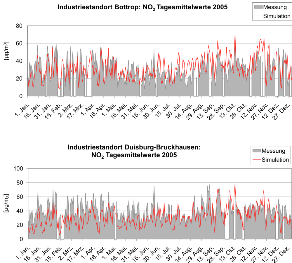
Abb. 5.8: Zeitreihen der berechneten und gemessenen NO 2 -Tagesmittelwerte [µg/m³] an den Stationen Bottrop (oben) und Duisburg-Bruckhausen (unten).
