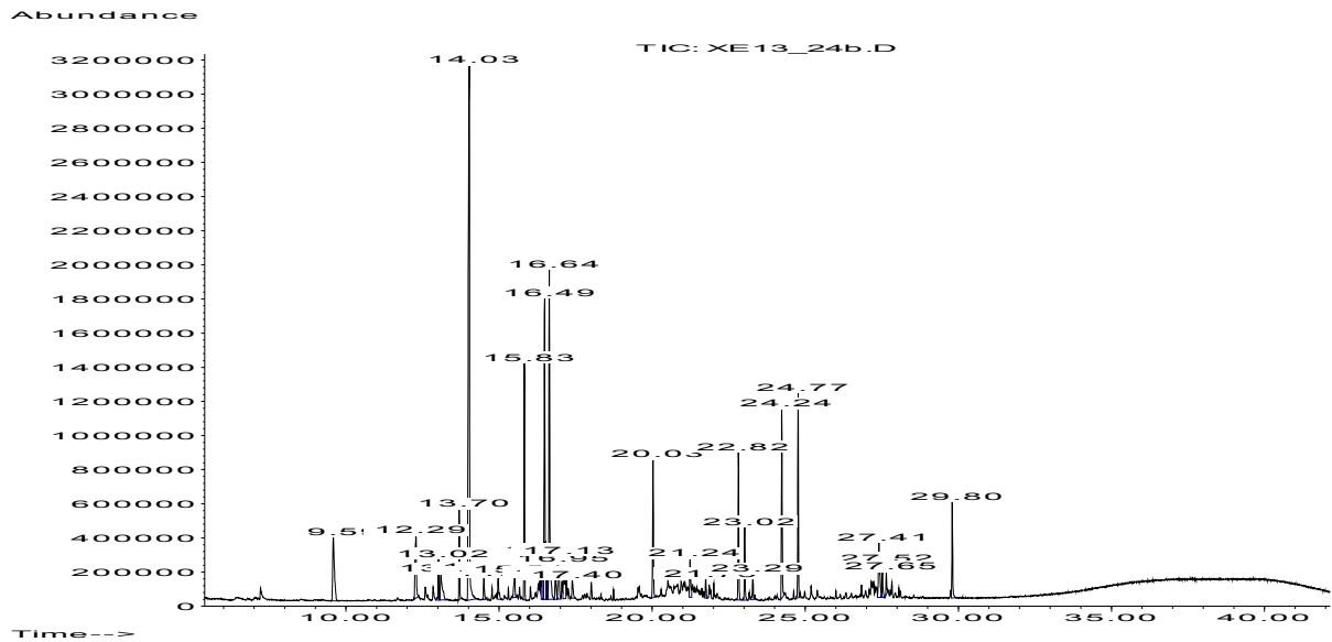
Abbildung 4161-1: GC/MS-Chromatogramm vom 29. Tag der Emissionsmessungen an einem PVC-Belag. (Peaks 15.8; 16.6; 24.2 IS)
