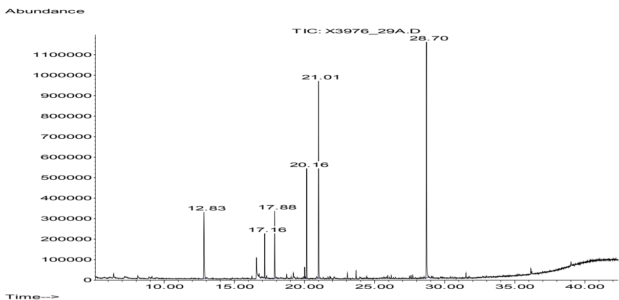
Abbildung 3976-1: GC/MS-Chromatogramm vom 29. Tag der Emissionsmessungen an einem Teppichboden. (Peaks 20.17; 21.02; 28.71 IS)
