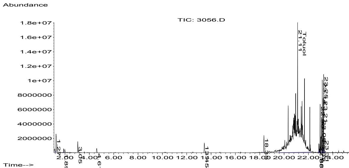
Abbildung 4200_99-1: GC/MS-Chromatogramm vom 29. Tag der Emissionsmessungen an einer Kombination Estrich PVC (4199) mit Teppichboden (4200). (Peak 18.3 IS)
