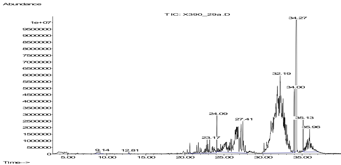
Abbildung 3900-1: GC/MS-Chromatogramm vom 29. Tag der Emissionsmessungen an einem PVC-Belag. (Peaks 25.33; 26.50; 35.06 IS)
