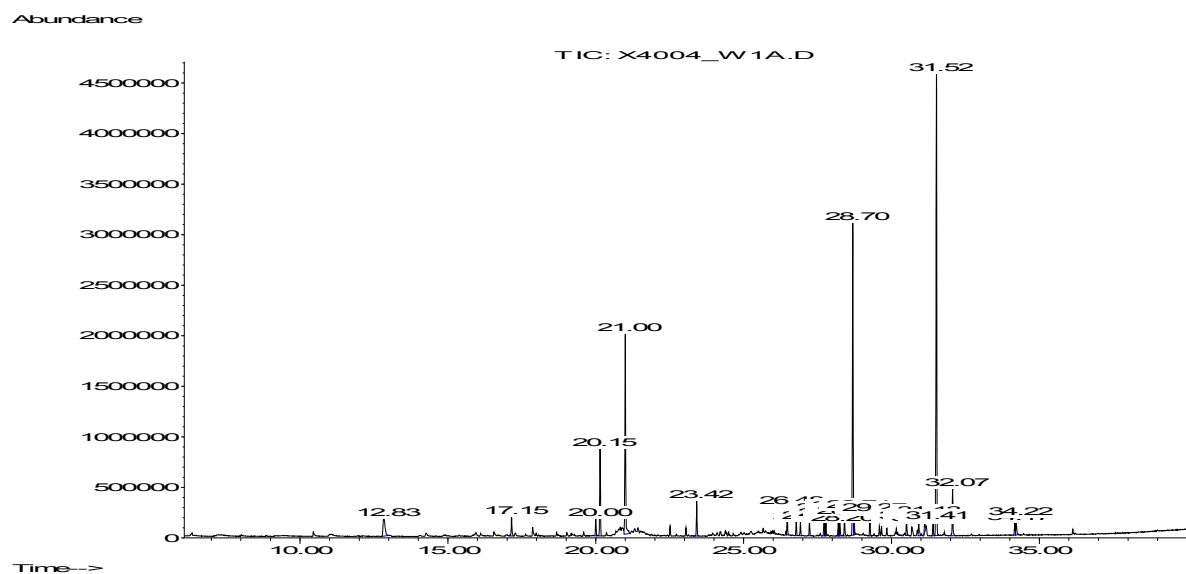
Abbildung 4004-1: GC/MS-Chromatogramm vom 29. Tag der Emissionsmessungen an einem PVC-Belag. (Peaks 20.15; 21.00; 28.70 IS)
