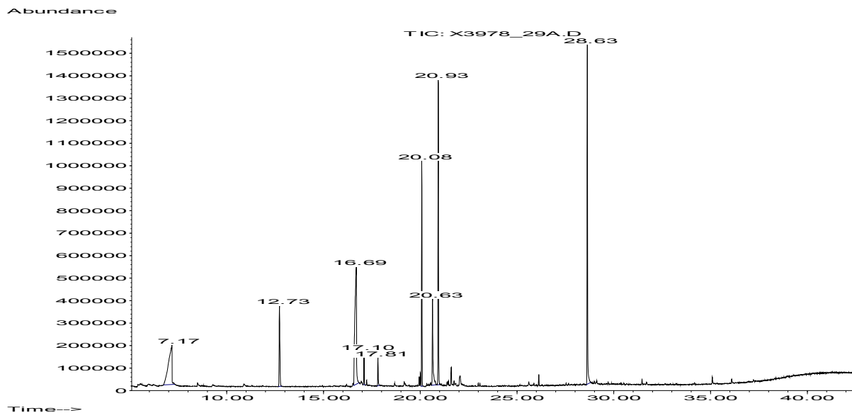
Abbildung 3978-1: GC/MS-Chromatogramm vom 29. Tag der Emissionsmessungen an einem Bodenbelagsklebstoff. (Peaks 20.17; 21.02; 28.71 IS)
