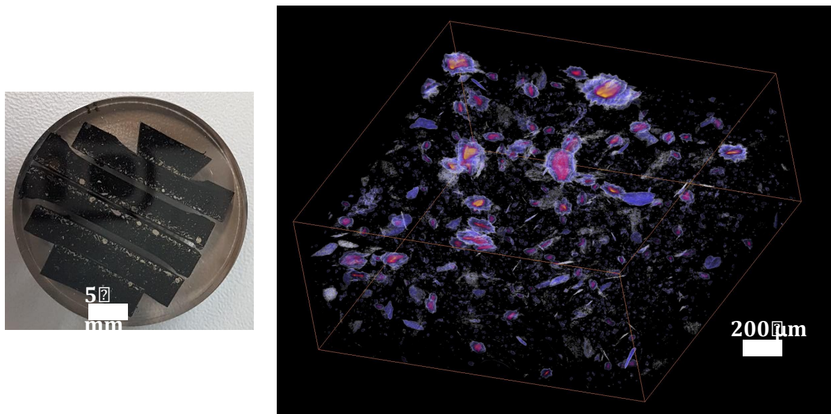
Abbildung 3-18: Rekonstruiertes 3D-Bild einer speziell präparierten Al-Mischschrottprobe (Probenbild links), die auf XRT-Messungen im Computertomographiemodus (XCT, rechts) basiert.
