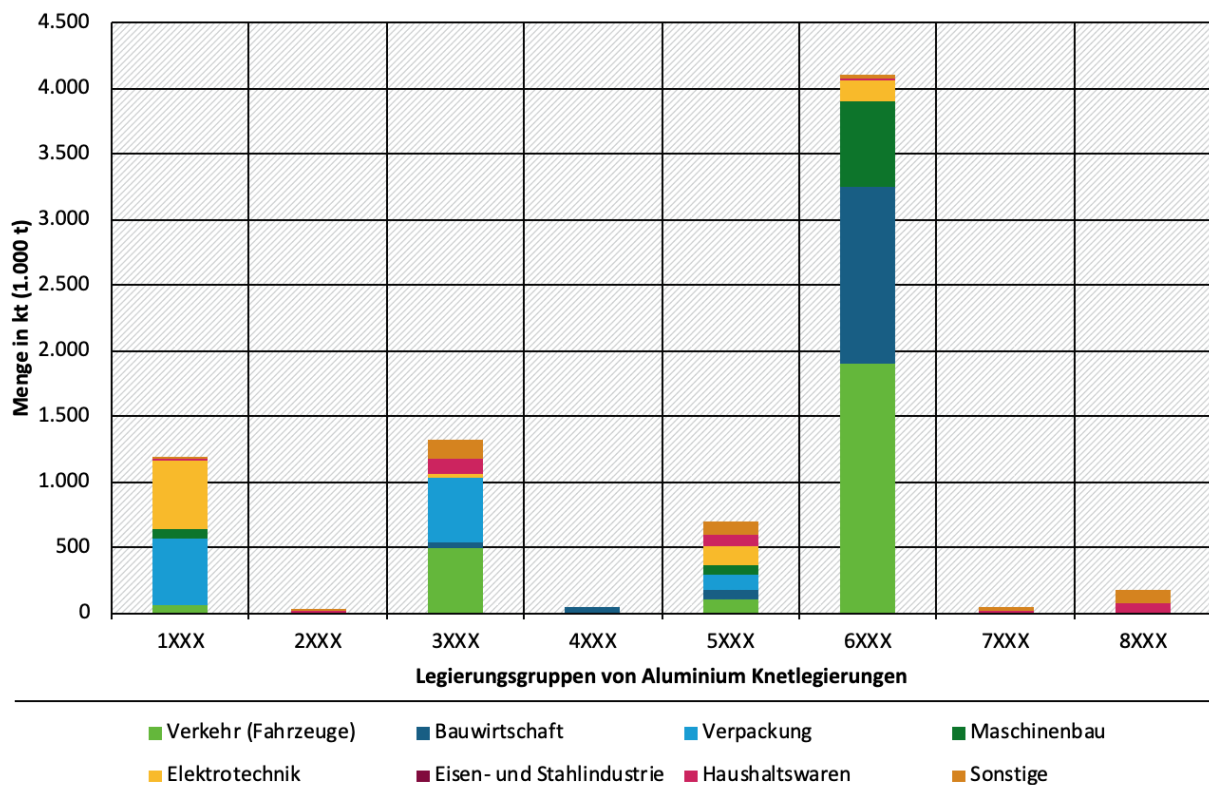
Abbildung 2-5: Europäische Nachfrage nach Aluminium Knetlegierungen in 2016 [kt]
