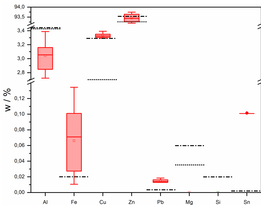
Abbildung 3-8: Mit pXRF ermittelte statistische Verteilung der Massenprozentage von verschiedenen Elementen in der Zinklegierung ZnAl4Cu3
