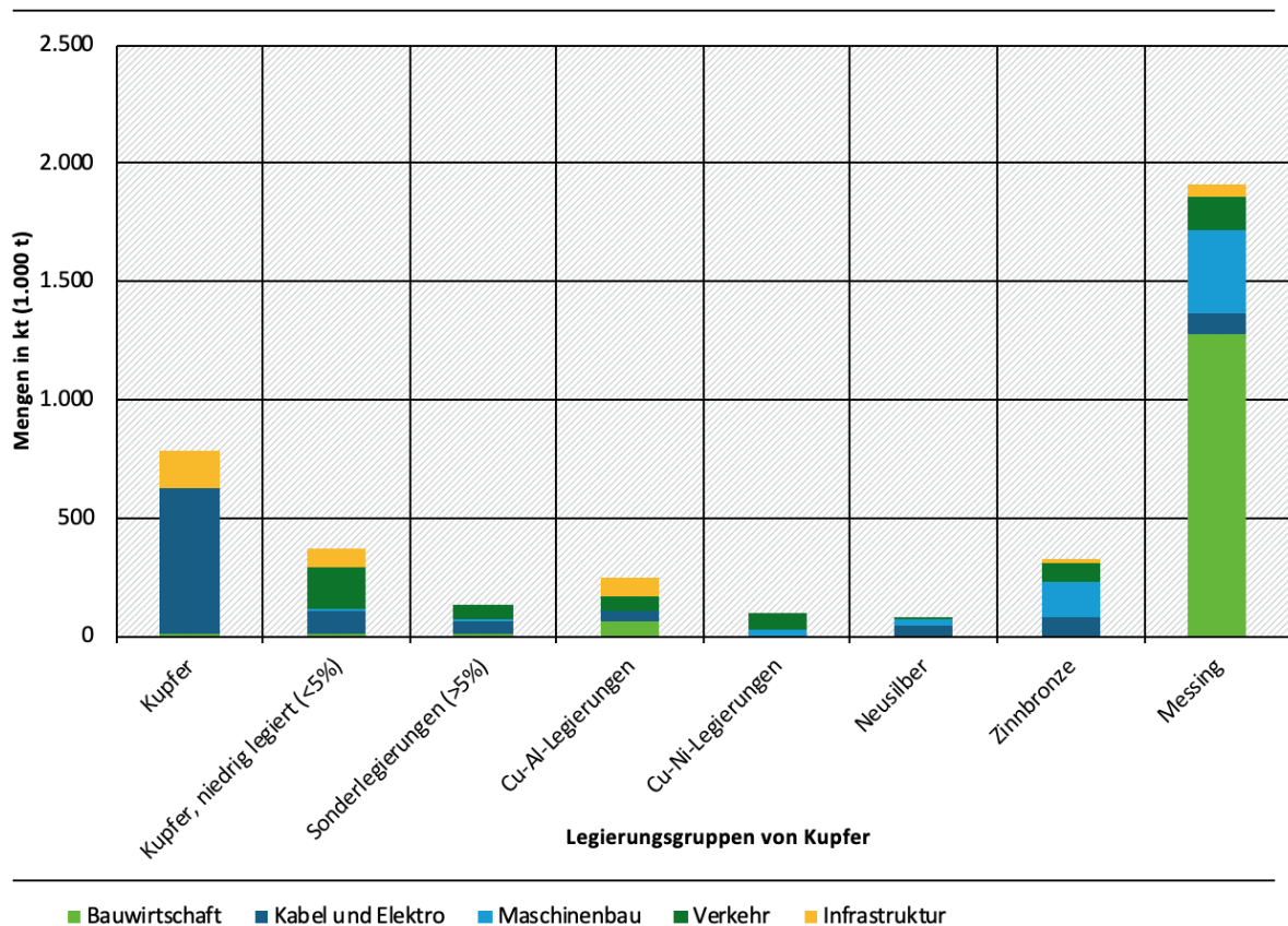
Abbildung 2-12: Europäische Nachfrage nach Kupferlegierungen in 2016 [kt]
