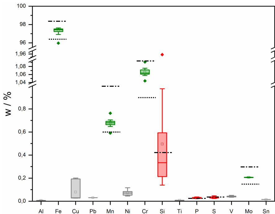
Abbildung 3-7: Mit pXRF ermittelte statistische Verteilung der Massenprozentage von verschiedenen Elementen in dem Stahl 42CrMo4.
