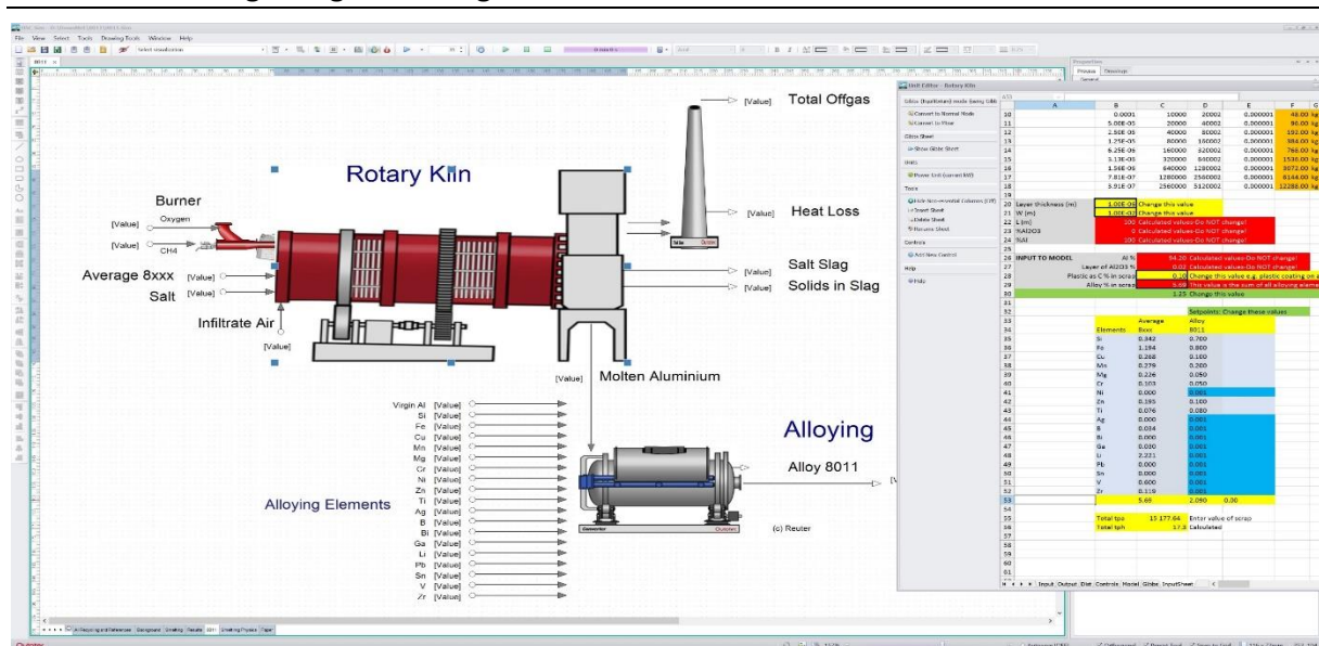
Abbildung 2-27: Ausschnitt aus der graphischen Darstellung der Simulation der Herstellung einer Legierung 8011 aus gemischtem 8xxx Aluminiumschrott
