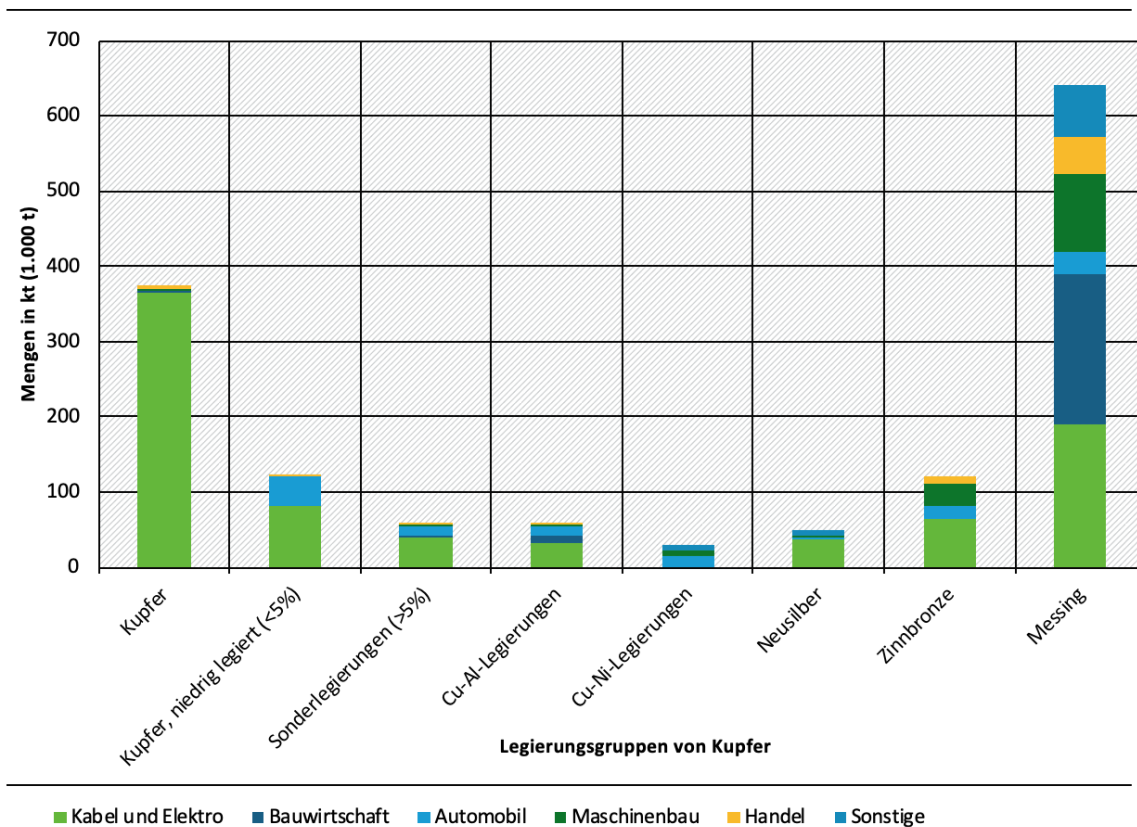
Abbildung 2-11: Deutsche Nachfrage nach Kupferlegierungen in 2016 [kt]
