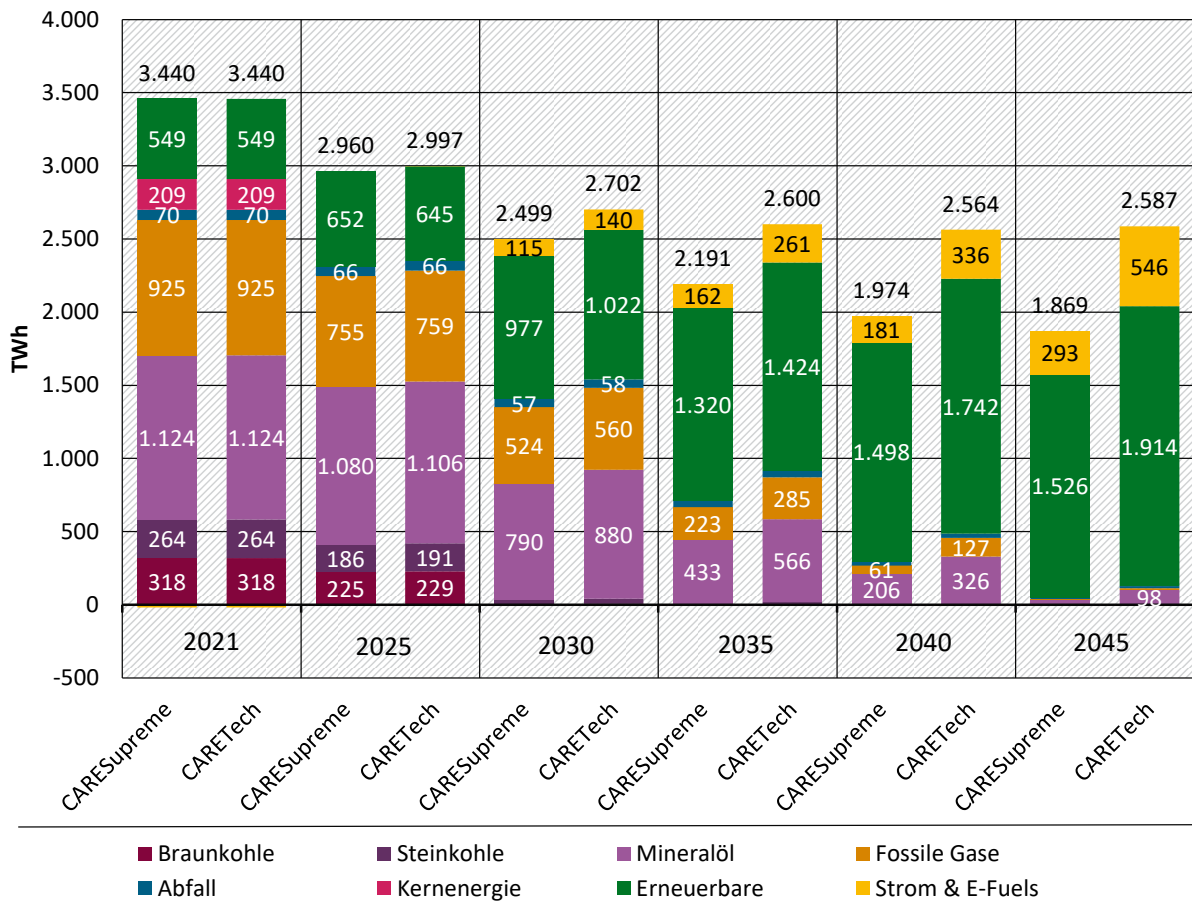
Abbildung 20: Primärenergieverbrauch nach Energieträgern in CARESupreme und CARETech, 2021-2045
