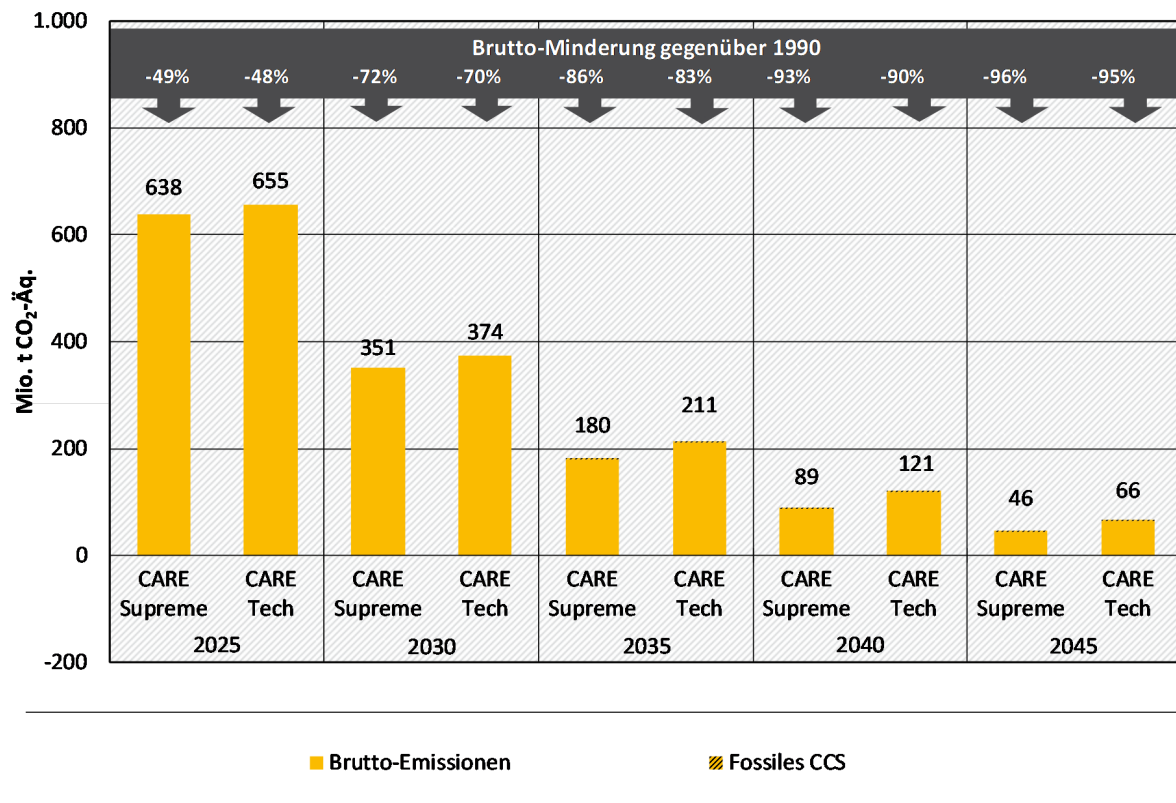
Abbildung 1: Brutto-Emissionsminderung in CARESupreme und CARETech, 2025-2045
