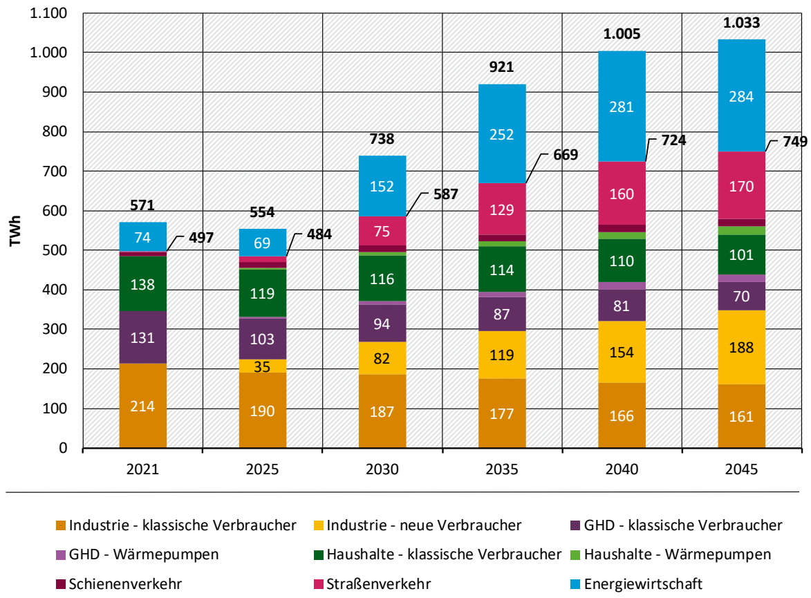
Abbildung 11: Bruttostromverbrauch in CARESupreme nach Sektoren, 2021-2045
