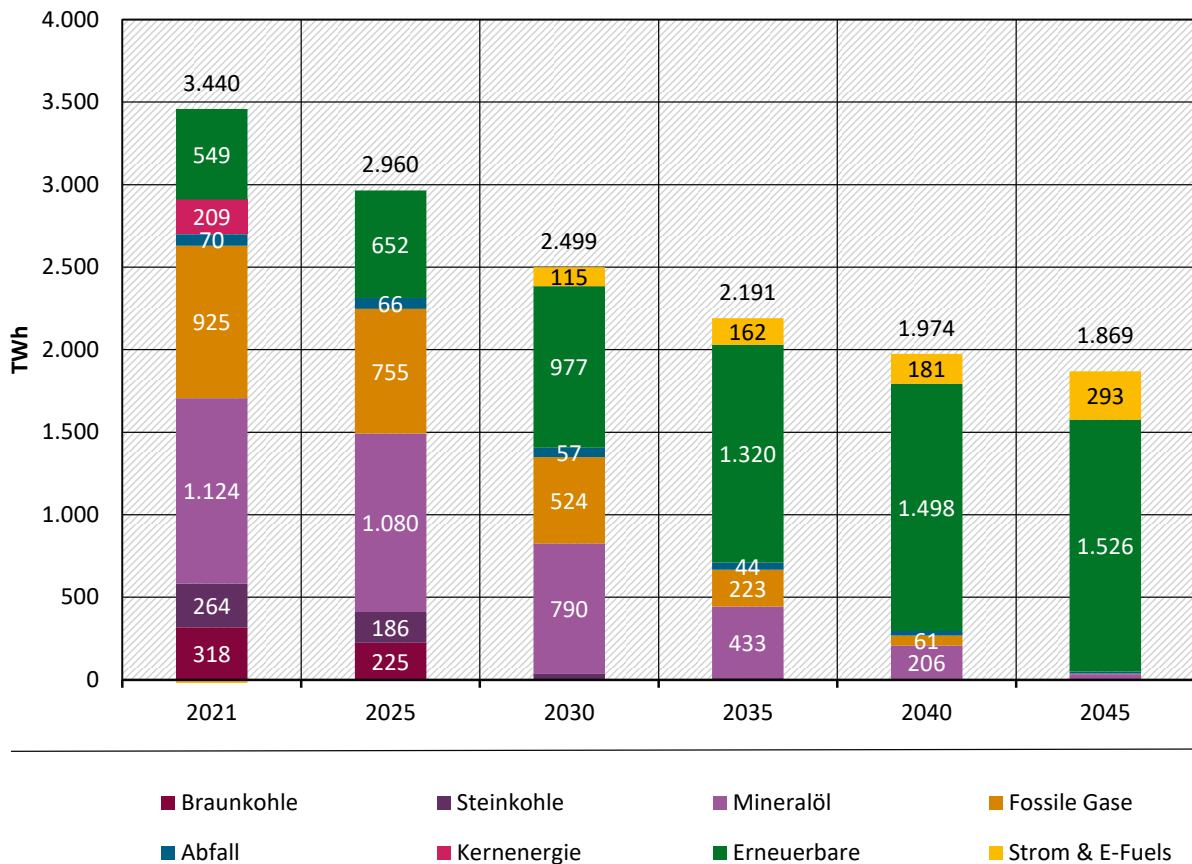
Abbildung 9: Primärenergieverbrauch nach Energieträgern in CARESupreme, 2021-2045
