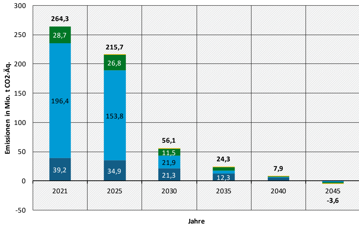
Abbildung 93: Emissionen der Energiewirtschaft nach bereitgestelltem Energieträger in CARESupreme, 2021-2045
