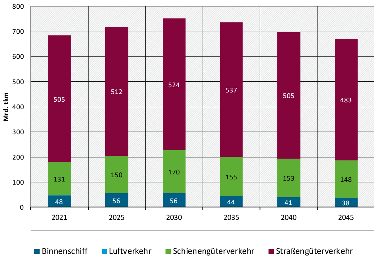
Abbildung 63: Güterverkehrsleistung (nationale Verkehre), CARESupreme, 2021-2045
