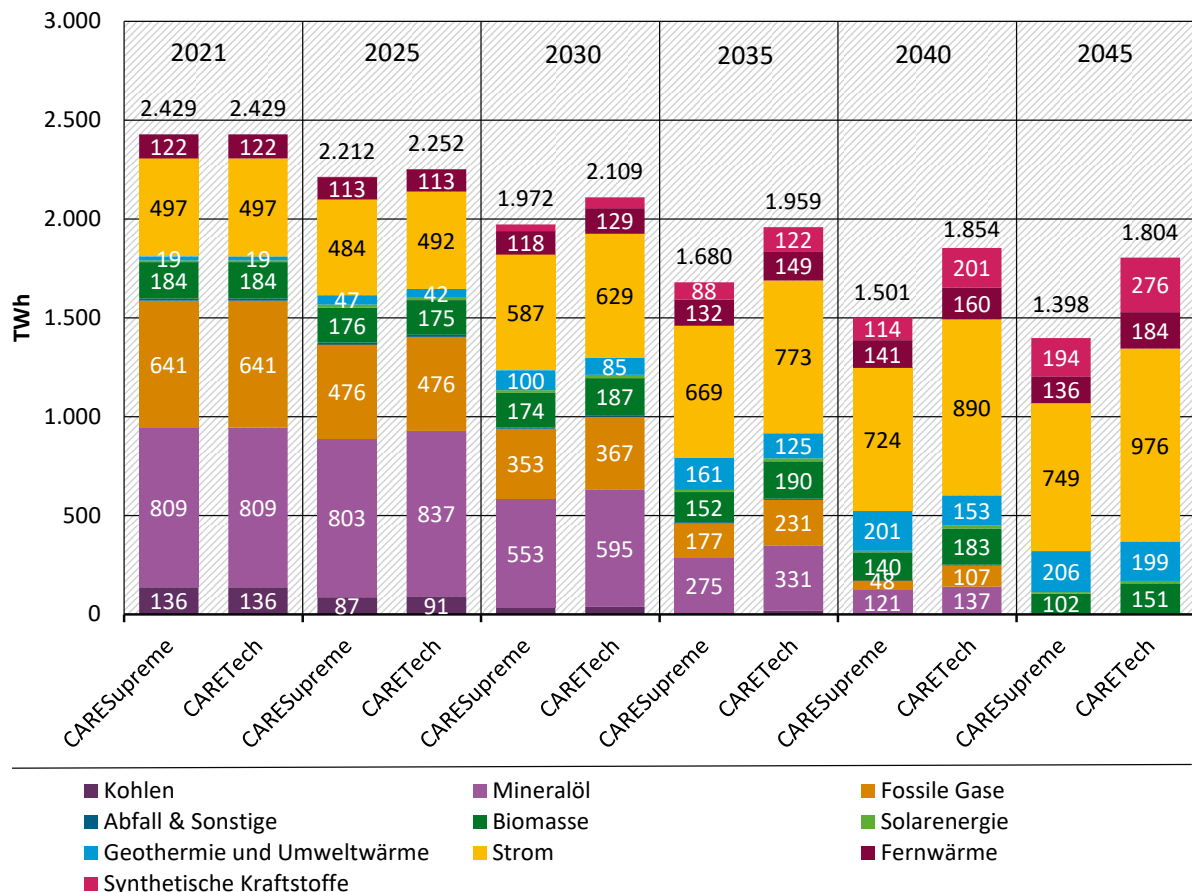
Abbildung 21: Endenergieverbrauch nach Energieträgern in CARESupreme und CARETech, 2021-2045
