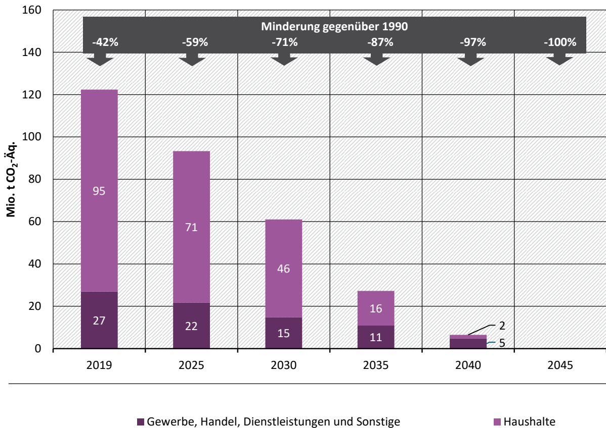
Abbildung 48: Entwicklung der Treibhausgasemissionen im Sektor Gebäude, CARESupreme, 2021-2045
