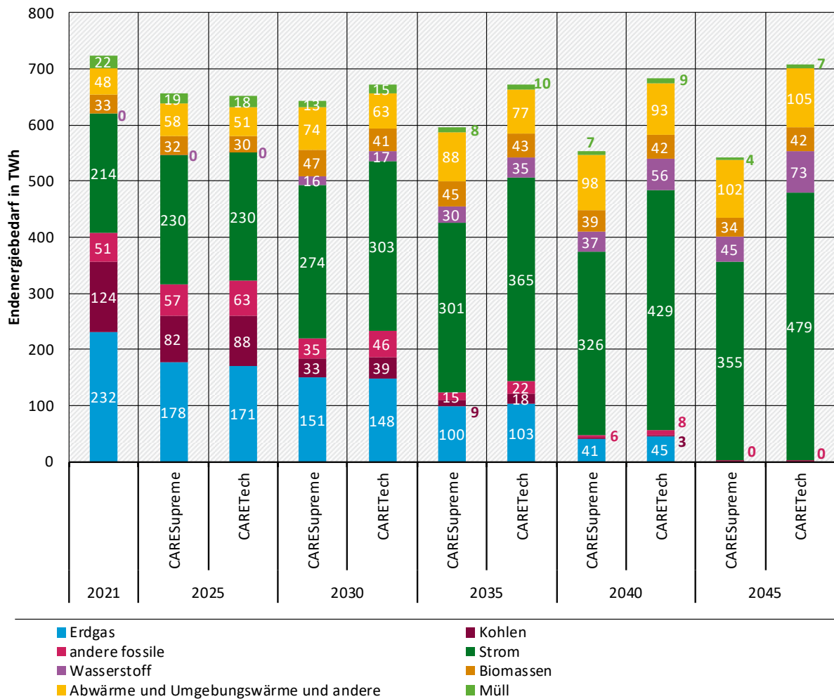
Abbildung 42: Endenergiebedarf Industrie, CARESupreme im Vergleich zu CARETech, 2021-2045
