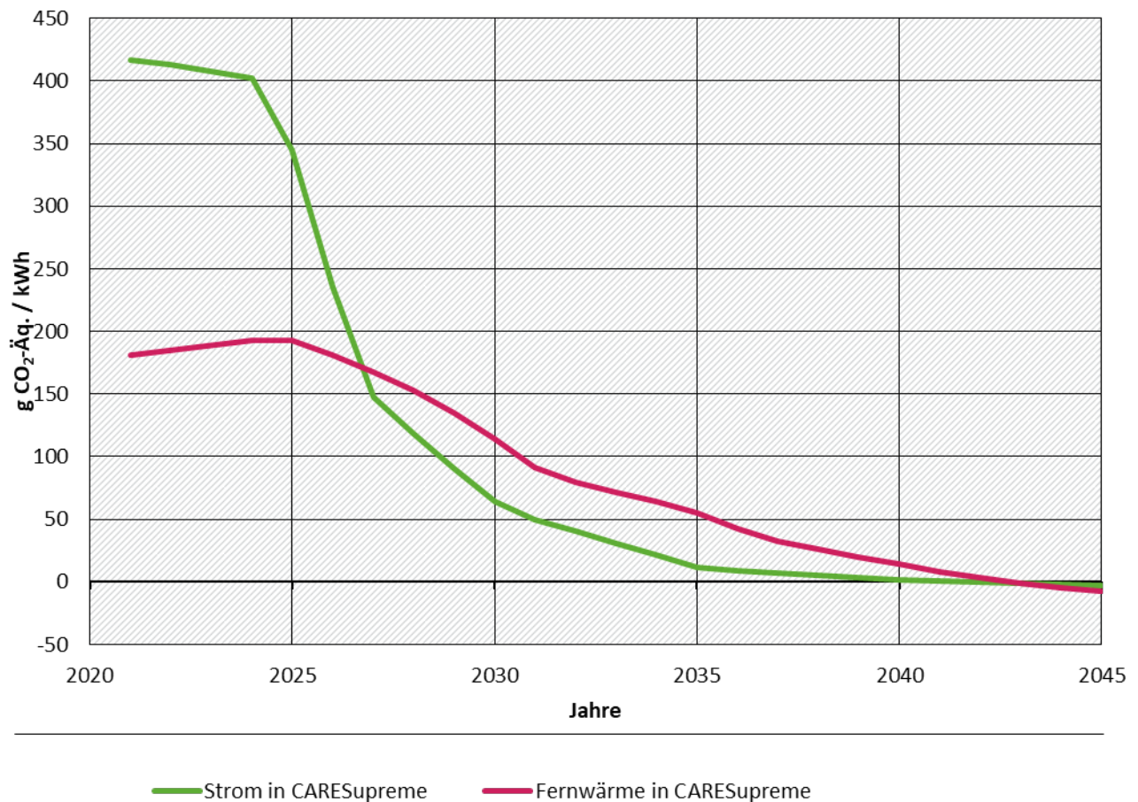
Abbildung 28: Resultierende Emissionsfaktoren für Strom und Fernwärme, CARESupreme, 2021-2045
