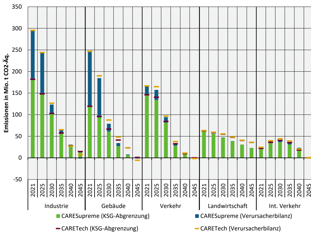
Abbildung 96: Verursacherbilanz je Sektor in CARESupreme und CARETech, 2021-2045
