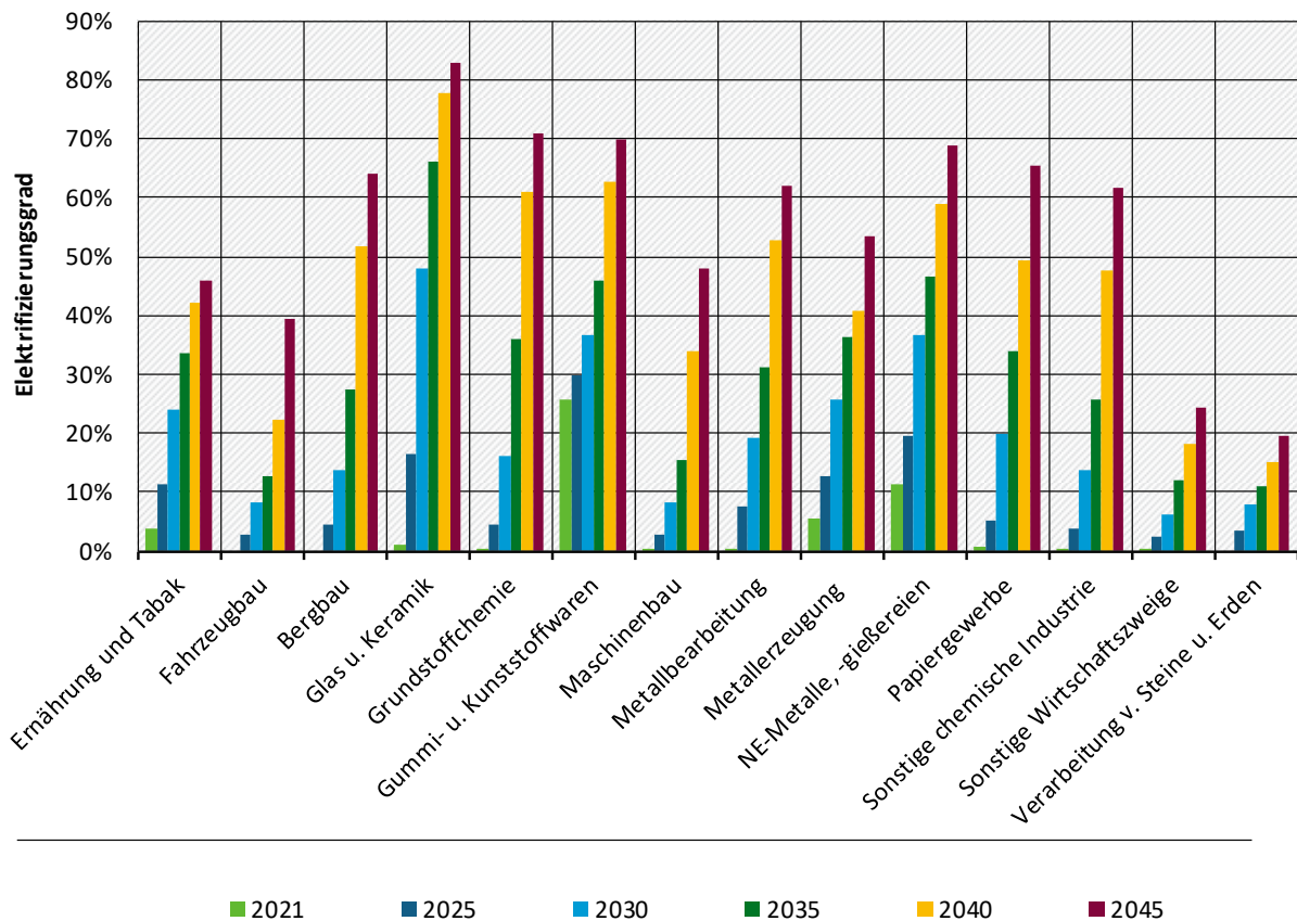
Abbildung 37: Direkter Elektrifizierungsgrad der Prozesswärme nach Subsektor, CARESupreme, 2021-2045
