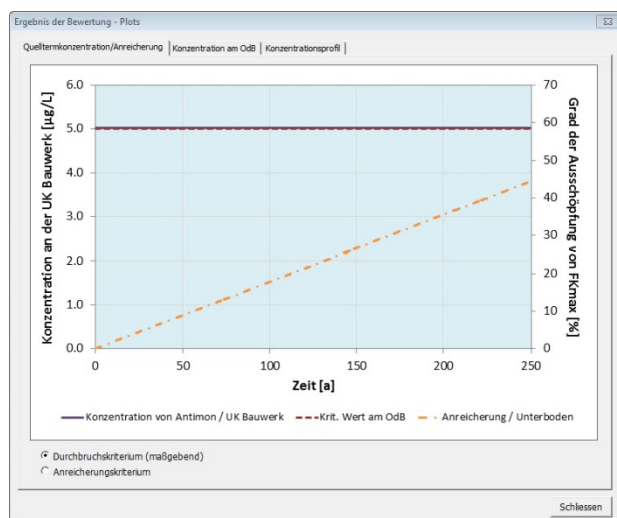
Abbildung 4-12: Ergebnisplots der individuellen Bewertung für Antimon in CUM-1 in der Einbauweise 14a für einen Quellterm mit konstanter Stofffreisetzung: Entwicklung der Konzentration im Quellterm und der Stoffanreicherung (links) und Konzentrationsdurchbruchskurve am OdB (rechts).
