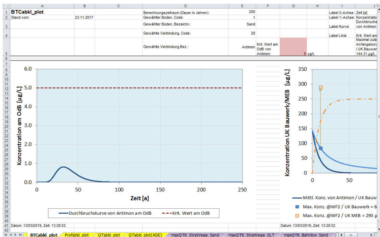
Abbildung 3-29: Tabellenblatt zur Darstellung des Konzentrationsverlaufs im Sickerwasser an der UK der MEB-Schicht, an der Bauwerk-UK und am OdB sowie der Stoffanreicherung im Bereich der Sickerstrecke als Grad der Ausschöpfung der maximalen Filterkapazität für einen Quellterm mit abklingender Freisetzungsrate (Blatt "BTCabkl_plot"): Beispiel einer individuellen Bewertung von Antimon in CUM für Einbauweise B1 unter Berücksichtigung des zeitlich abklingenden Quellterms mit dem Anreicherungskriterium als maßgebendes Kriterium) – Teil 1
