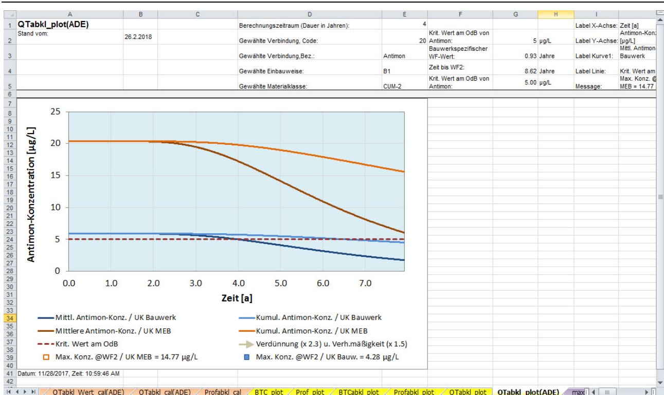
Abbildung 3-33: Tabellenblatt zur Darstellung des Konzentrationsverlaufs im Sickerwasser an der UK der MEB-Schicht sowie der UK des Bauwerks bei einer nach dem Advektions-Dispersionsmodell abklingenden Freisetzungsrate (Blatt "QTabkl_plot(ADE)"): Beispiel einer individuellen Bewertung von Antimon in CUM für die Einbauweise B1
