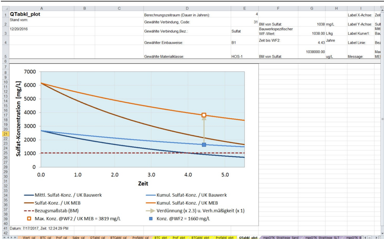
Abbildung 3-32: Tabellenblatt zur Darstellung des Konzentrationsverlaufs im Sickerwasser an der UK der MEB-Schicht sowie der UK des Bauwerks bei einer exponentiell abklingenden Freisetzungsrates (Blatt "QTabkl_plot"): Beispiel einer individuellen Bewertung von Sulfat in HOS für die Einbauweise B1
