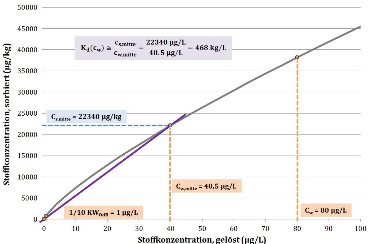
Abbildung 2-10: Schematische Darstellung der Ermittlung eines Sorptionsverteilungskoeffizienten durch Linearisierung der nicht-linearen Sorptionsisotherme mit Hilfe des Verfahrens „ K_d Mitte“ am Beispiel der substratübergreifenden Sorptionsisotherme für Chrom an sandigem Unterboden (EBV-Bodenkategorie „Sand“).
