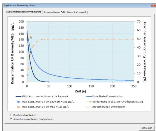
Abbildung 4-15: Ergebnisplots der individuellen Bewertung für Antimon in CUM-1 in der Einbauweise 14a für einen Quellterm mit abklingender Stofffreisetzung: Entwicklung der Konzentration im Quellterm und der Stoffanreicherung (links) und Konzentrationsdurchbruchskurve am OdB (rechts).
