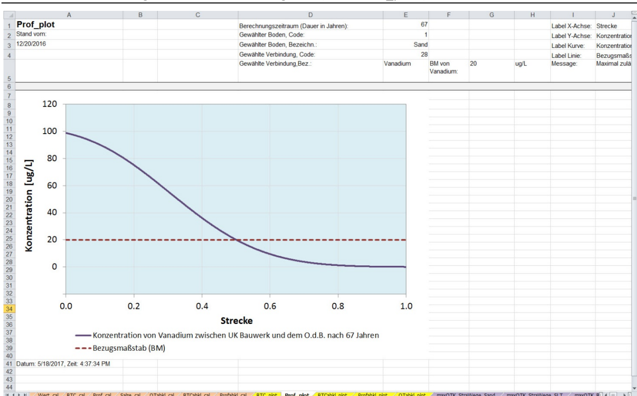
Abbildung 3-28: Tabellenblatt zur Darstellung des Konzentrationsprofils im Sickerwasser entlang der Sickerstrecke zwischen der UK des Bauwerks und dem OdB für einen Quellterm mit langfristig konstanter Freisetzungsrate (Blatt "Prof_plot")
