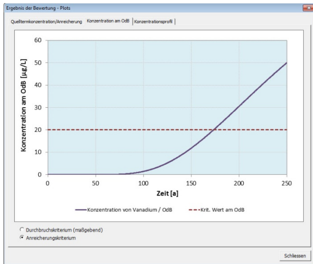
Abbildung 4-7: Ergebnisgrafiken nach einer individuellen Bewertung unter Berücksichtigung einer einzelnen materialrelevanten Stoffkomponente (Vanadium) eines MEB (RC-2): Konzentrationsdurchbruchskurve am OdB (links oben), Konzentrationsprofil entlang der Sickerstrecke (rechts oben) sowie Entwicklung der Konzentration im Quellterm und der Stoffanreicherung (links unten), jeweils für die maximal zulässige Quelltermkonzentration in der Bauweise B5 bei sandigem Unterboden für das nicht maßgebende Anreicherungskriterium.
