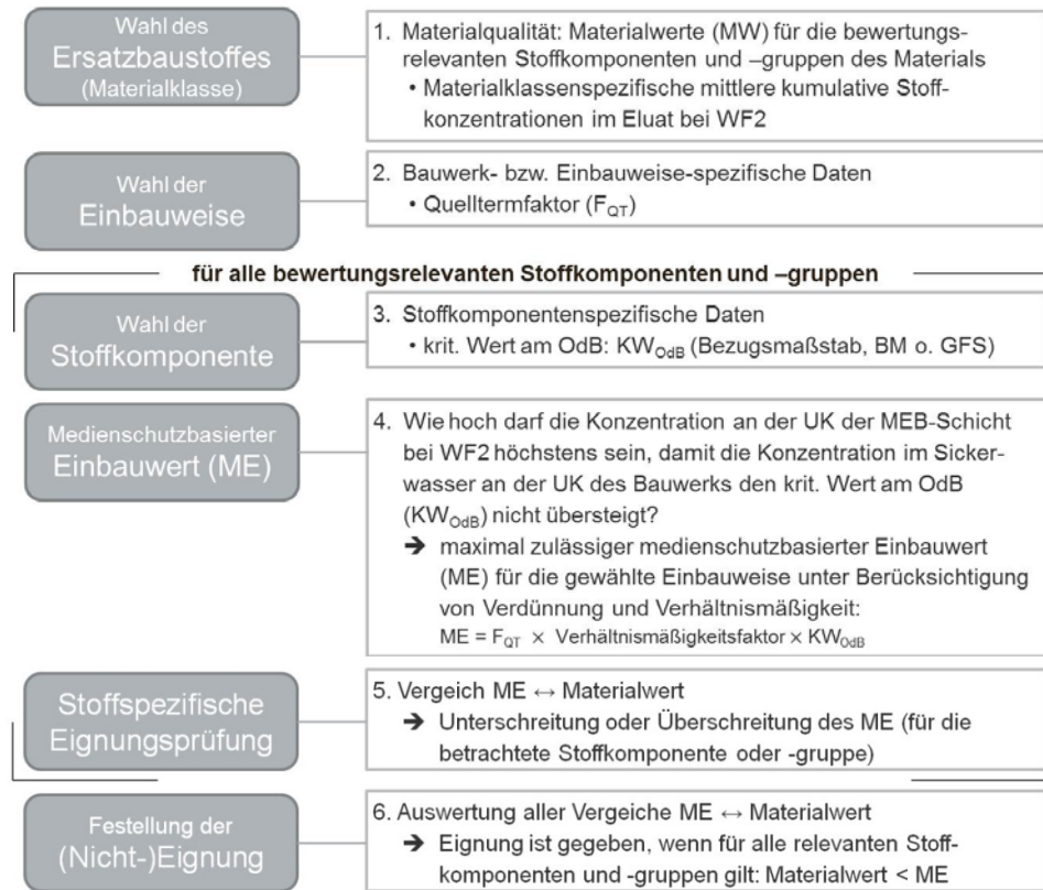
Abbildung 2-4: Teilschritte der Ableitungssystematik für Metalle und Organika sowie Fluorid, die kein deutliches und regelmäßig nachgewiesenes Abklingverhalten der Freisetzung aus dem betrachteten Material zeigen, bei ungünstigen Verhältnissen.
