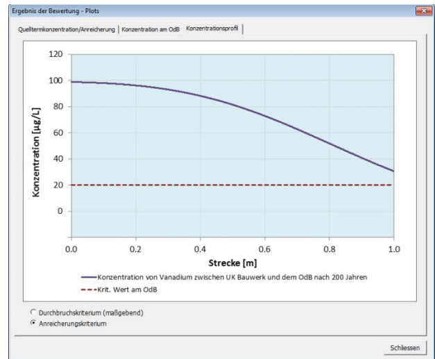
Abbildung 4-7: Ergebnisgrafiken nach einer individuellen Bewertung unter Berücksichtigung einer einzelnen materialrelevanten Stoffkomponente (Vanadium) eines MEB (RC-2): Konzentrationsdurchbruchskurve am OdB (links oben), Konzentrationsprofil entlang der Sickerstrecke (rechts oben) sowie Entwicklung der Konzentration im Quellterm und der Stoffanreicherung (links unten), jeweils für die maximal zulässige Quelltermkonzentration in der Bauweise B5 bei sandigem Unterboden für das nicht maßgebende Anreicherungskriterium.
