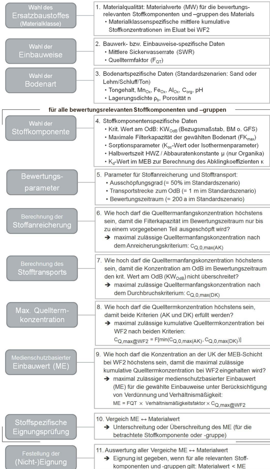
Abbildung 2-3: Teilschritte der Ableitungssystematik für Stoffkomponenten oder –gruppen und Materialien, für die ein deutliches Abklingverhalten der Freisetzung reproduzierbar nachgewiesen werden konnte bei günstigen Verhältnissen.
