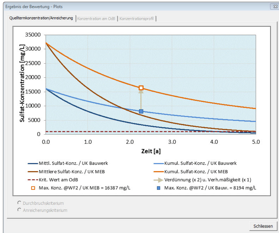
Abbildung 4-9: Ergebnisgrafiken nach einer individuellen Bewertung unter Berücksichtigung einer einzelnen materialrelevanten Stoffkomponente eines MEB: Entwicklung der mittleren aktuellen und der kumulativen Konzentration an der UK des Bauwerks sowie an der UK des MEB für die von BEMEB ermittelte maximal zulässige Quelltermkonzentration (hier Sulfat in der Einbauweise B5).
