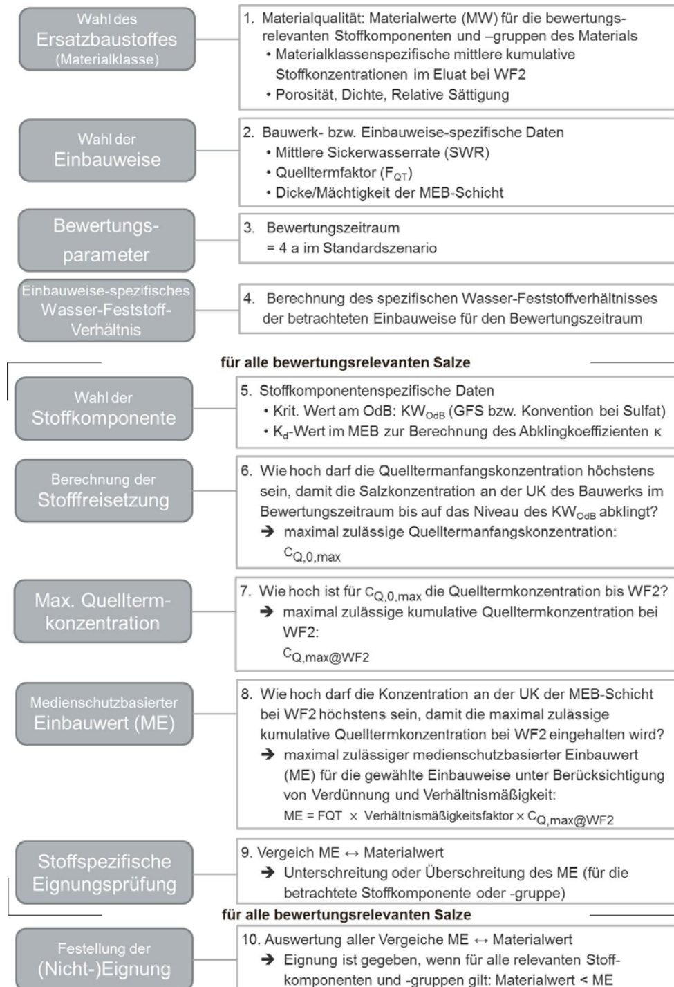
Abbildung 2-5: Teilschritte der Ableitungssystematik für Stoffkomponenten oder –gruppen und Materialien, für die ein deutliches Abklingverhalten der Freisetzung reproduzierbar nachgewiesen werden konnte bei ungünstigen Verhältnissen oder wenn die Verhältnisse nicht relevant sind, weil kein nennenswerter Rückhalt oder Abbau gegeben ist und daher der Transportterm nicht berücksichtigt wird (bei Chlorid und Sulfat).
