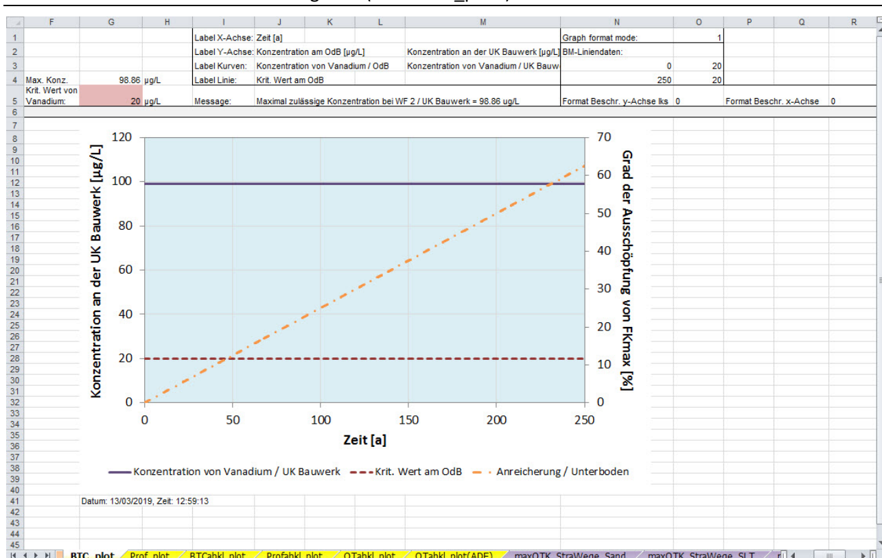
Abbildung 3-27: Tabellenblatt zur Darstellung des Konzentrationsverlaufs im Sickerwasser an der Bauwerk-UK und am OdB sowie der Stoffanreicherung im Bereich der Sickerstrecke als Grad der Ausschöpfung der maximalen Filterkapazität für einen Quellterm mit langfristig konstanter Freisetzungsrate (Blatt "BTC_plot") – Teil 2
