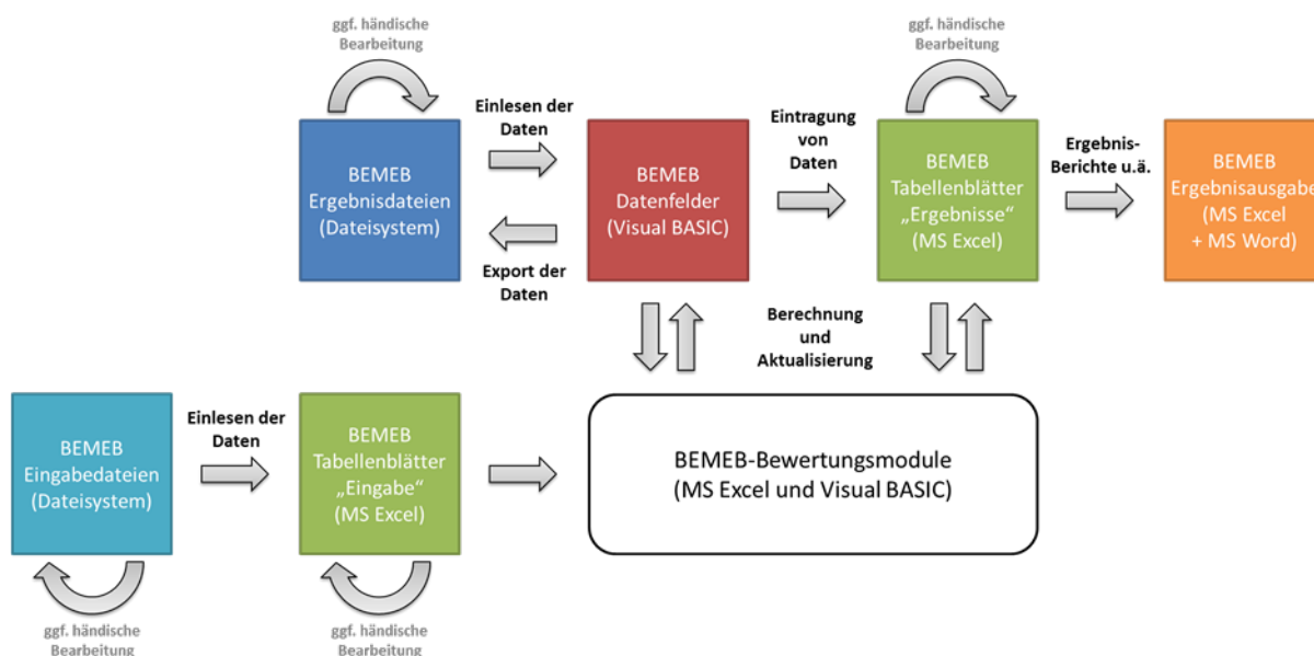
Abbildung 3-1: Schematische Darstellung der Daten, welche in BEMEB verarbeitet werden
