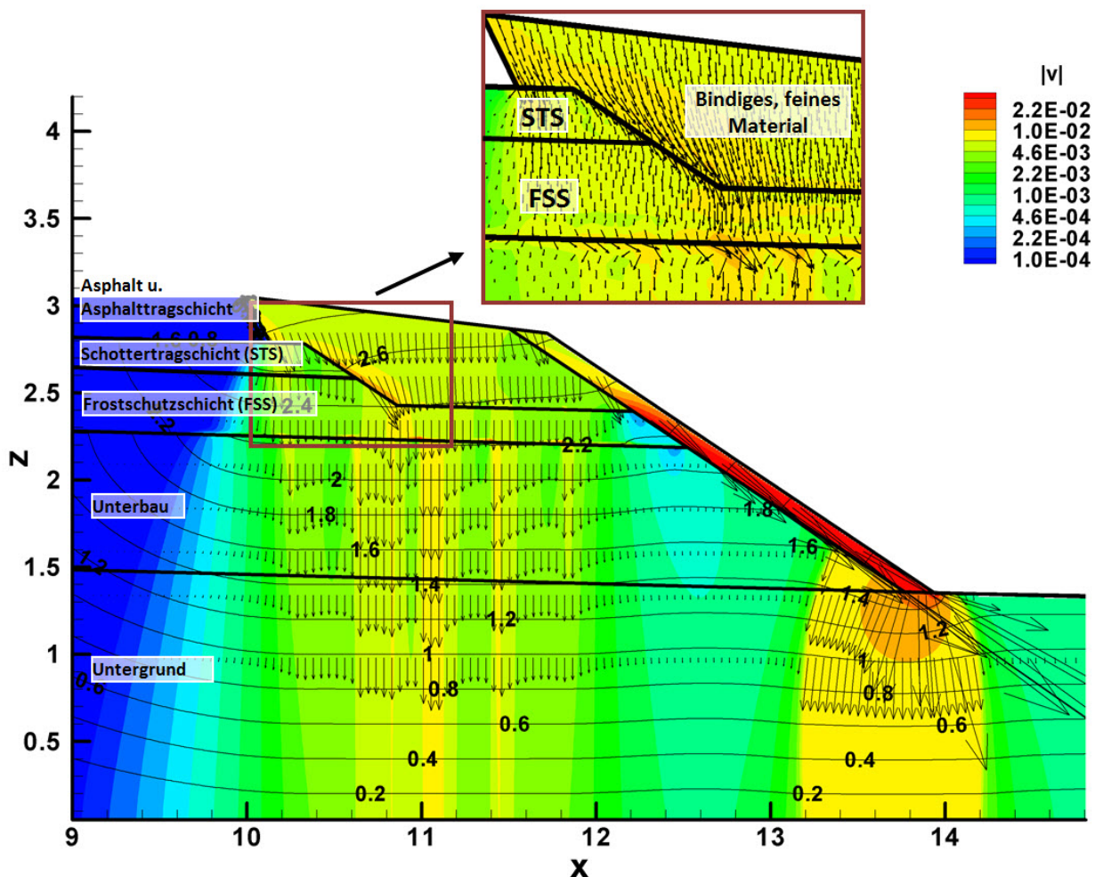
Abbildung 2-8: Strömungsvektoren und Potentiallinien der Sickerwasserströmung in einem Straßendamm. Die Strömungsvektoren sind mit Pfeilen dargestellt. Im vergrößerten Bereich wird der Kapillarsperreneffekt veranschaulicht. Die höhere Durchlässigkeit des nahezu wassergesättigten feinen Materials führt hier zu einem bevorzugten Fließen oberhalb des Übergangs zum grobkörnigen Material. Dadurch werden mineralische Ersatzbaustoffe in der Schottertragschicht (STS) und in der Frostschutzschicht (FSS) nur teilweise durchströmt (verändert nach Susset et al. 2013; S. 37).
