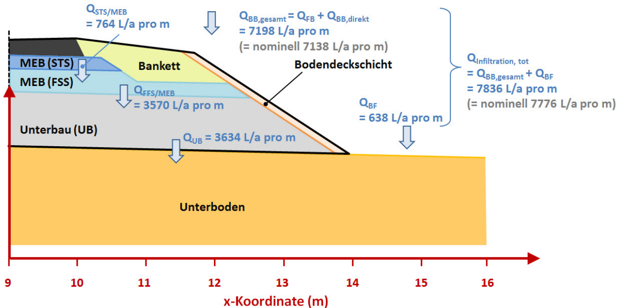
Abbildung 2-9: Schematische Darstellung der für die Berücksichtigung von Verdünnungseffekten relevanten Teilsickerwasserraten am Beispiel des Szenarios „niedriger Straßendamm“. Dargestellt sind die Ergebnisse der hydraulischen Simulation. Hinweis: Die Infiltrationsraten im Modell sind geringfügig höher als die nominellen Werte; da mit den Sickerwasserratenverhältnissen relative Ergebniswerte berechnet werden, ist dies jedoch von untergeordneter Bedeutung.
