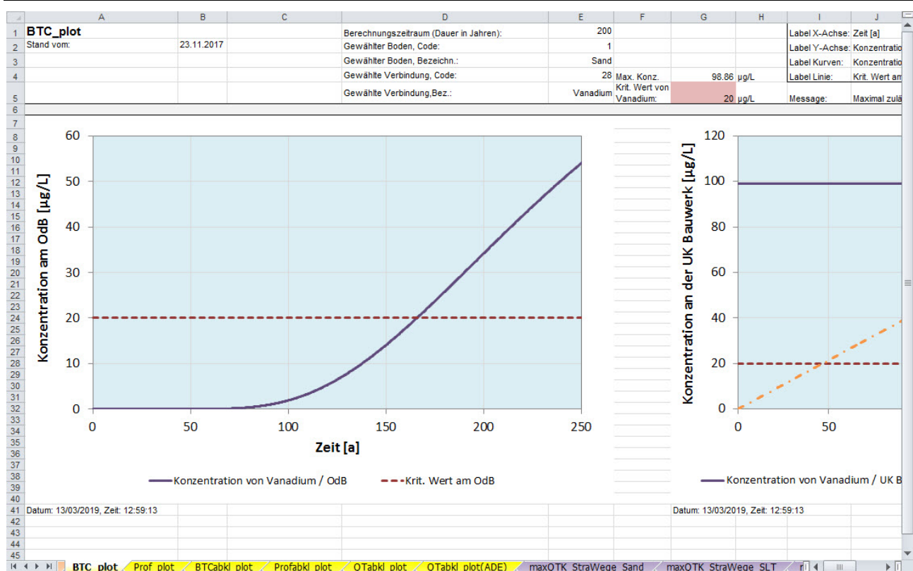
Abbildung 3-26: Tabellenblatt zur Darstellung des Konzentrationsverlaufs im Sickerwasser an der Bauwerk-UK und am OdB sowie der Stoffanreicherung im Bereich der Sickerstrecke als Grad der Ausschöpfung der maximalen Filterkapazität für einen Quellterm mit langfristig konstanter Freisetzungsrate (Blatt "BTC_plot") – Teil 1
