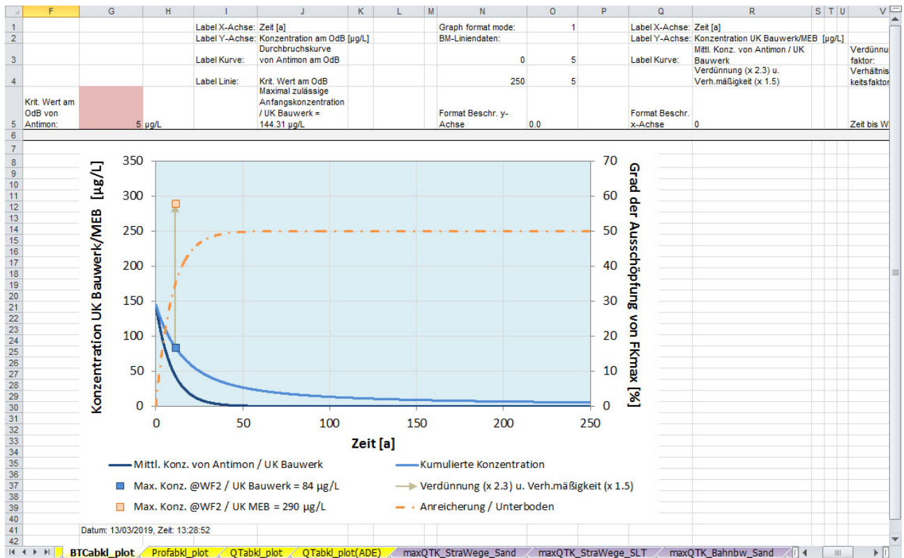
Abbildung 3-30: Tabellenblatt zur Darstellung des Konzentrationsverlaufs im Sickerwasser an der UK der MEB-Schicht, an der Bauwerk-UK und am OdB sowie der Stoffanreicherung im Bereich der Sickerstrecke als Grad der Ausschöpfung der maximalen Filterkapazität für einen Quellterm mit abklingender Freisetzungsrate (Blatt "BTCabkl_plot"): Beispiel einer individuellen Bewertung von Antimon in CUM für Einbauweise B1 unter Berücksichtigung des zeitlich abklingenden Quellterms mit dem Anreicherungskriterium als maßgebendes Kriterium) – Teil 2
