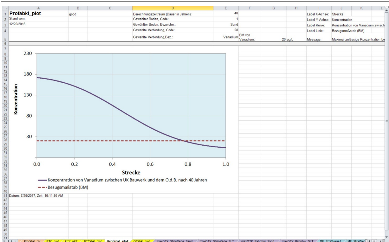
Abbildung 3-31: Tabellenblatt zur Darstellung des Konzentrationsprofils im Sickerwasser entlang der Sickerstrecke für einen Quellterm mit abklingender Freisetzungsrates (Blatt "Profabkl_plot"): Beispiel einer individuellen Bewertung von Vanadium in SFA für Einbauweise B1 nach 40 Jahren.
