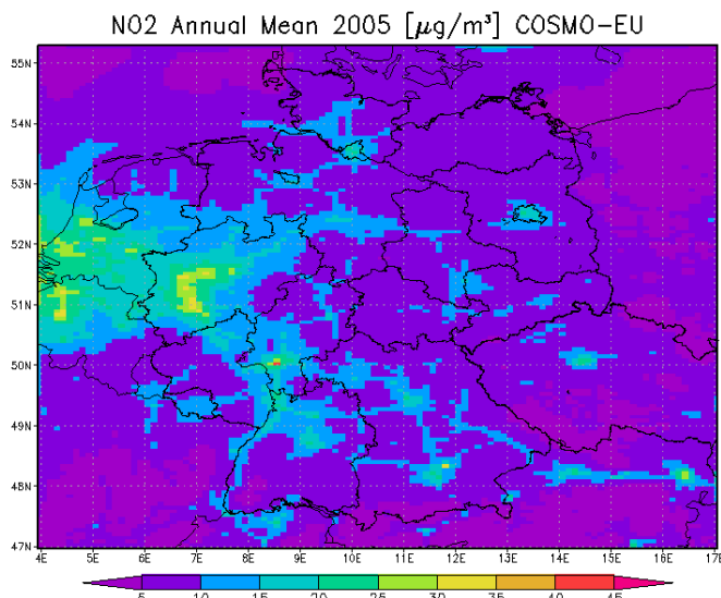
Abbildung 36 NO 2 -Jahresmittelwert in \mu\text{g}/\text{m}^3 - Kontrolllauf
