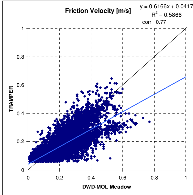
Abbildung 11 Mit TRAMPER simulierte (y-Achse) und an der Wiesenstation gemessene (x-Achse) u^* [m/s]. Lineargleichung ( y=ax+b ), Bestimmtheitsmaß ( R^2 ) und Korrelationskoeffizient (corr).
