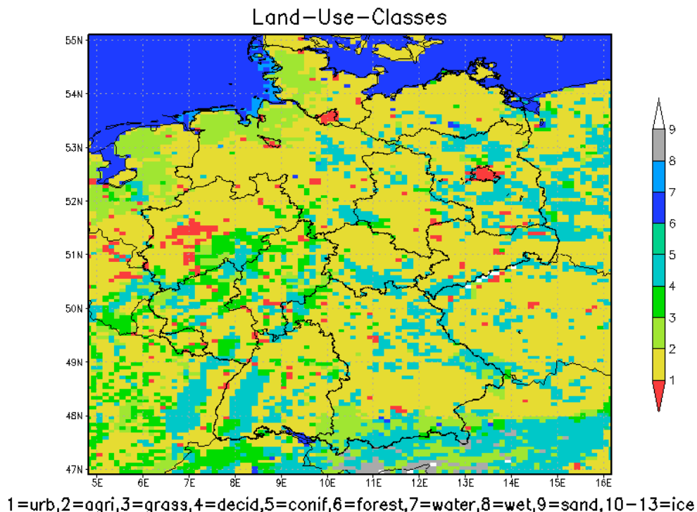
Abbildung 7 Landnutzungsklassen (Farbskalenwerte: 1 urban, 2 Landwirtschaft, 3 Grasland, 4 Laubwald, 5 Nadelwald, 6 Mischwald, 7 Wasser, 8 Feuchtgebiete, 9 Sand, 10-13 Eis) auf einem ca. 15x15 km 2 - Gitter.
