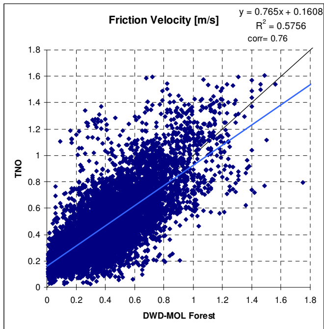
Abbildung 20 Mit TNO-EZMW simulierte (y-Achse) und an der Waldstation gemessene (x-Achse) u^* [m/s]. Lineargleichung ( y=ax+b ), Bestimmtheitsmaß ( R^2 ) und Korrelationskoeffizient ( \text{corr} ).
