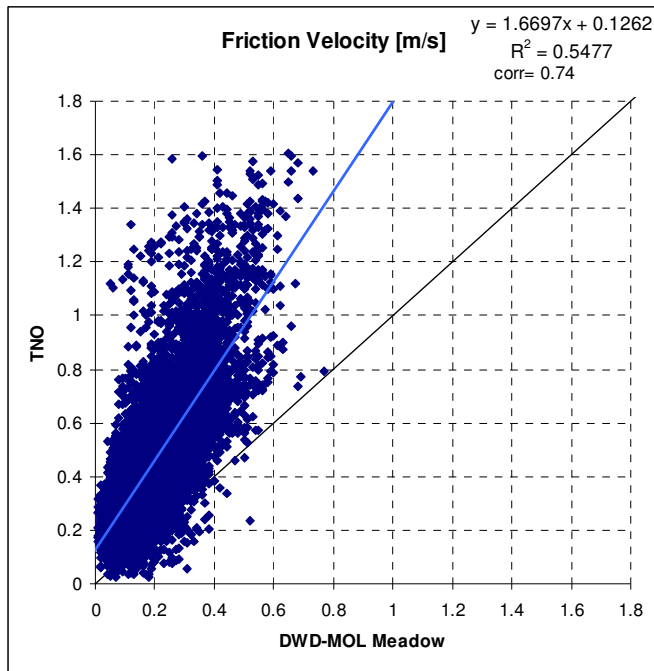
Abbildung 19 Mit TNO-EZMW simulierte (y-Achse) und an der Wiesenstation gemessene (x-Achse) u^* [m/s]. Lineargleichung ( y=ax+b ), Bestimmtheitsmaß ( R^2 ) und Korrelationskoeffizient ( \text{corr} ).
