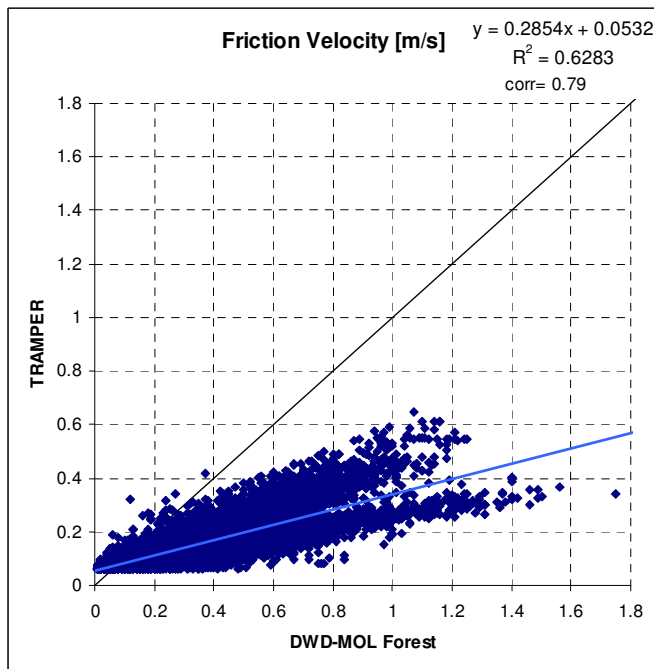
Abbildung 12 Mit TRAMPER simulierte (y-Achse) und an der Waldstation gemessene (x-Achse) u^* [m/s]. Lineargleichung ( y=ax+b ), Bestimmtheitsmaß ( R^2 ) und Korrelationskoeffizient (corr).
