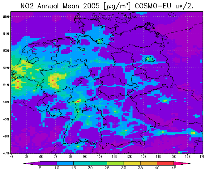
Abbildung 37 \text{NO}_2 -Jahresmittelwert in \mu\text{g}/\text{m}^3 - Sensitivitätslauf
