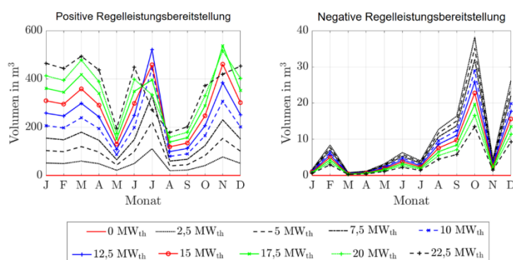
Abbildung 187: Benötigte Speichervolumina für die stationären Minutenregelleistungen des Kalina-Referenz-Geothermie-Kraftwerks mit Einsatz eines Fernwärmenetzspeichers für Fernwärmenetzleistungen von 0 MW th bis 22,5 MW th .
