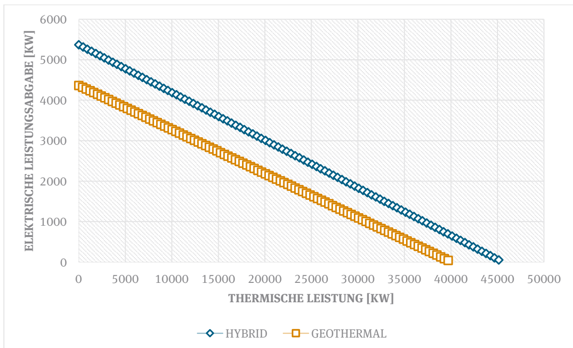
Abbildung 44: P_{el} - \dot{Q} -Diagramm für ein rein geothermisches Konzept und ein Hybridkonzept.
