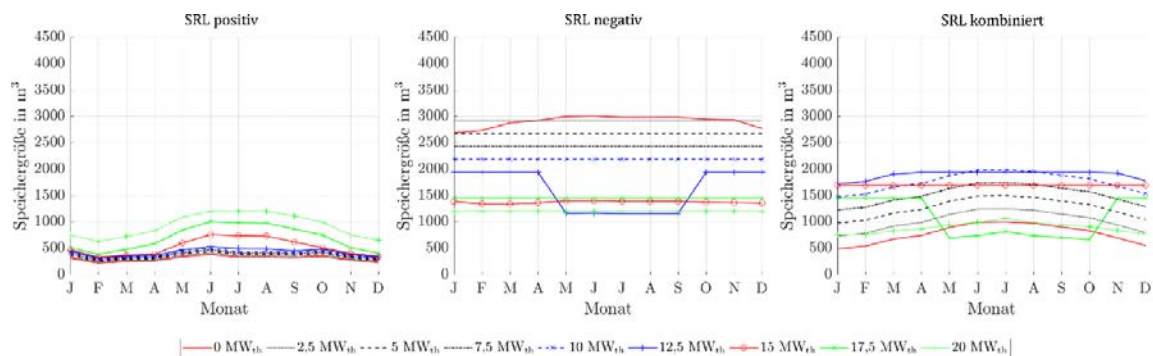
Abbildung 291: Benötigte Speichergrößen bei Angebot von positiver, negativer und kombinierter SRL des ORC-Referenz-Geothermie-Kraftwerks mit Einsatz eines Thermalwasserspeichers im Kraftwerk für Fernwärmenetzleistungen von 0 MW th bis 20 MW th bei zwei 4h-Zeitscheiben Einspeicherung und zwei aufeinanderfolgenden Zeitscheiben Angebotszeitraum.
