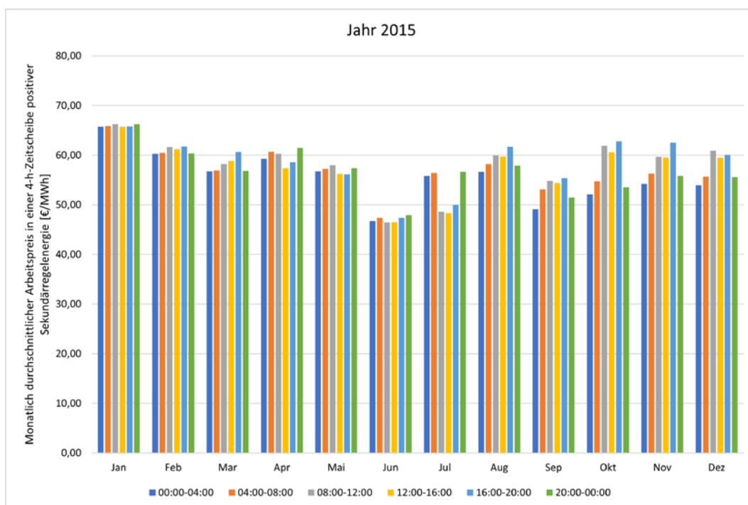
Abbildung 218: Monatlich durchschnittlicher Arbeitspreis in einer 4h-Zeitscheibe positiver Sekundärregelleistung 2015.
