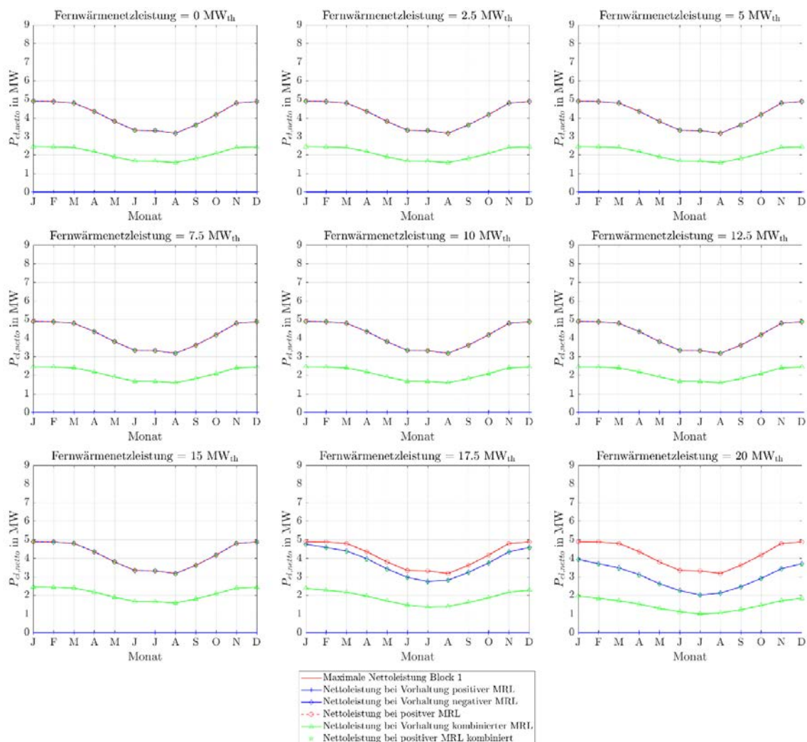
Abbildung 312: Stationäre Minutenregelleistungen des ORC-Referenz-Geothermie-Kraftwerks mit Einsatz eines Heißwasser-Wärmespeichers im Fernwärmenetz für Fernwärmenetzleistungen von 0 MW th bis 20 MW th bei zwei 4h-Zeitscheiben Einspeicherung und zwei aufeinanderfolgenden Zeitscheiben Angebotszeitraum
