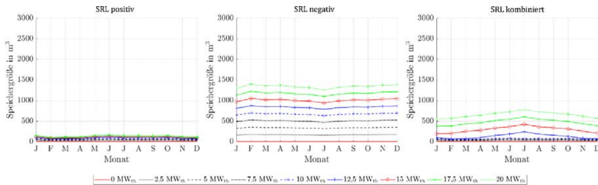
Abbildung 108: Benötigte Speichergrößen bei Angebot von positiver, negativer und kombinierter SRL des ORC-Referenz-Geothermie-Kraftwerks mit Einsatz eines Heißwasser-Wärmespeichers im Fernwärmenetz für Fernwärmenetzleistungen von 0 MW th bis 20 MW th bei zwei 4h-Zeitscheiben Einspeicherung und einer Zeitscheibe Angebotszeitraum.
