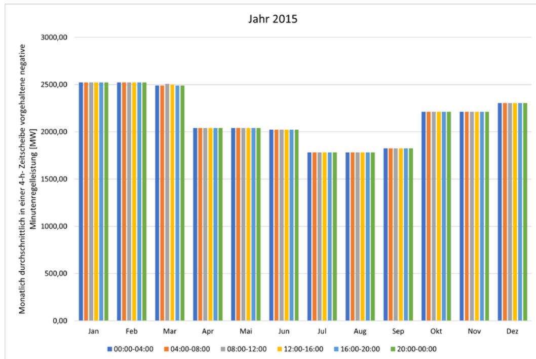
Abbildung 235: Monatlich durchschnittlich in einer 4h-Zeitscheibe vorgehaltene negative Minutenregel-leistung 2015.
