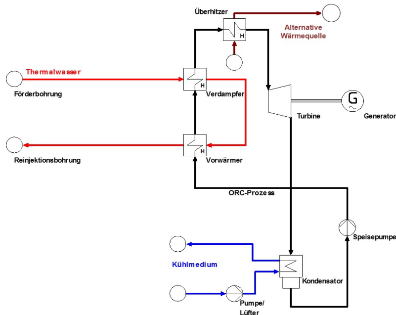
Abbildung 43: ORC-Anlagenkonzepte für Hybridkraftwerke: Überhitzung des ORC-Mediums.
