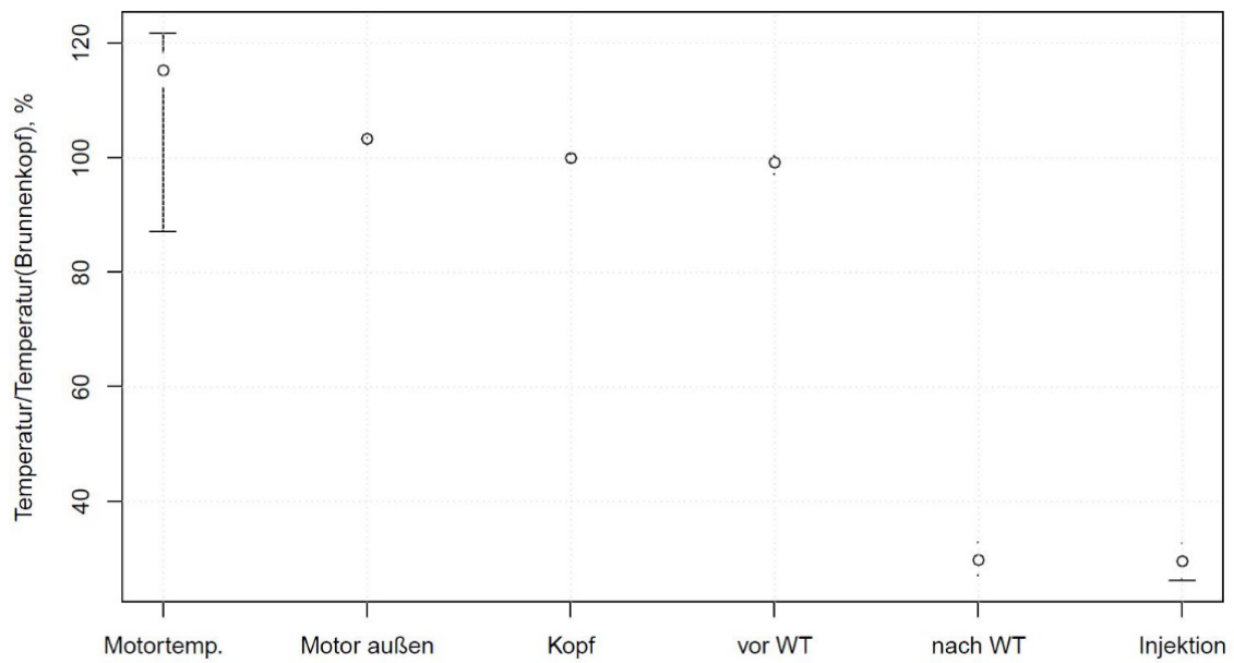
Abbildung 17: Relative Temperatur (Basis: Median der Temperatur am Brunnenkopf = 100%) entlang des Thermalwasserkreislaufs. Dargestellt sind Median und IQR.
