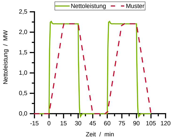
Abbildung 65: Lastprofil der dynamischen Simulation im Vergleich zum Verlauf des Musterprotokolls für die einseitig positive Tertiärregelleistung (Betrachtungsmonat Mai; Fernwärmeleistung 10 MW).
