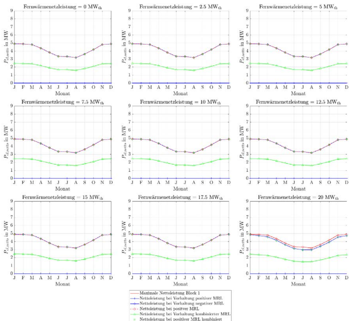
Abbildung 318: Stationäre Minutenregelleistungen des ORC-Referenz-Geothermie-Kraftwerks mit Einsatz eines Heißwasser-Wärmespeichers im Fernwärmenetz für Fernwärmenetzleistungen von 0 MW th bis 20 MW th bei drei 4h-Zeitscheiben Einspeicherung und zwei aufeinanderfolgenden Zeitscheiben Angebotszeitraum.
