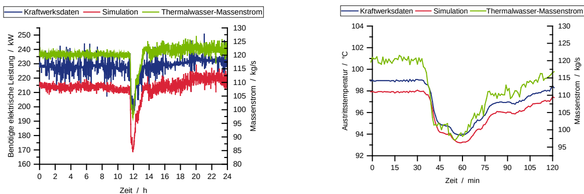
Abbildung 62: Simulations- und Kraftwerksdaten zur Eigenleistung der ORC-Speisepumpe in Abhängigkeit des Thermalwassermassenstroms (links) sowie Simulations- und Kraftwerksdaten zur Austrittstemperatur des ORC-Arbeitsmediums am Vorwärmer (rechts).
