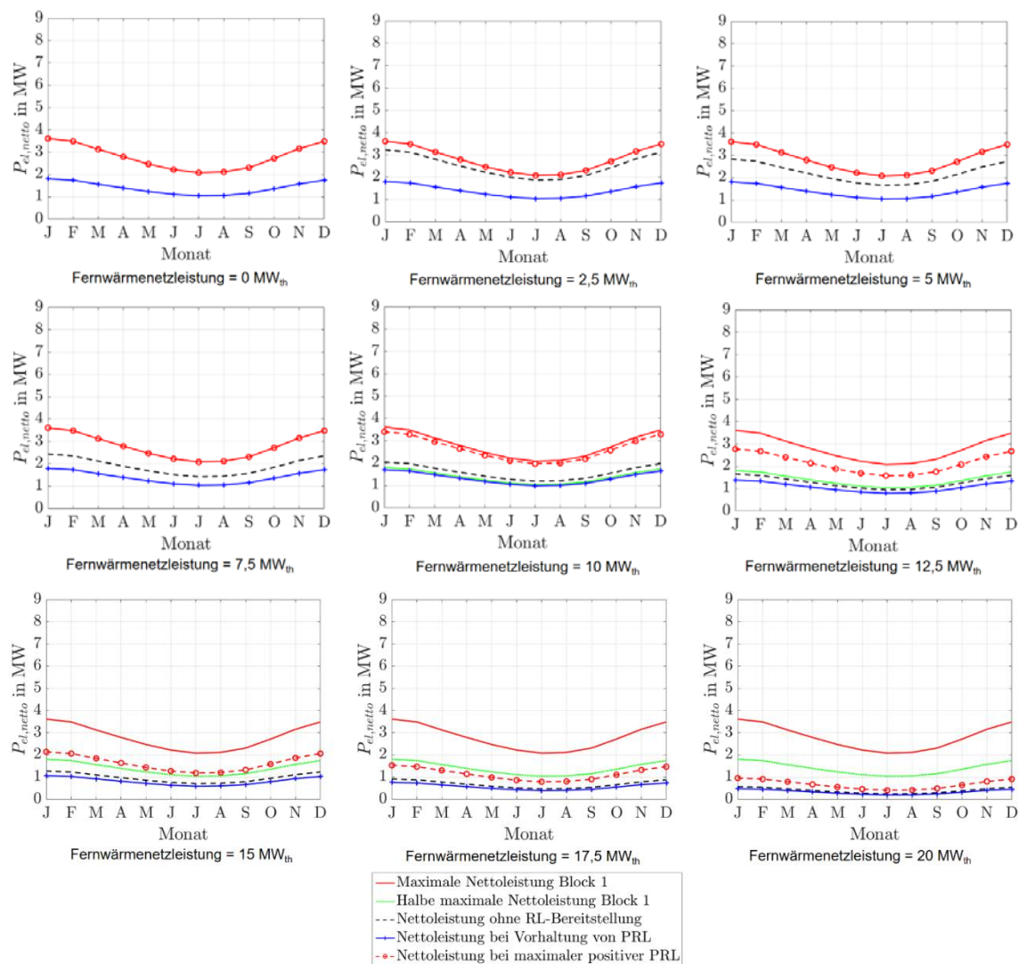
Abbildung 188: Stationäre Primärregelleistungen des Kalina-Referenz-Geothermie-Kraftwerks mit Einsatz eines Thermalwasserspeichers für Fernwärmenetzleistungen von 0 MW th bis 20 MW th .
