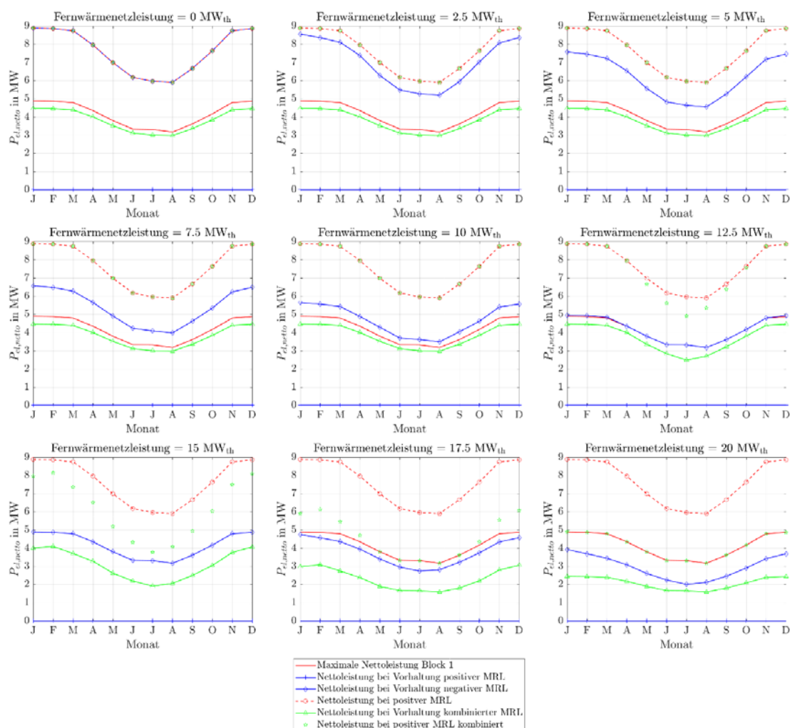
Abbildung 332: Stationäre Minutenregelleistungen des ORC-Referenz-Geothermie-Kraftwerks mit Einsatz eines Thermalwasserspeichers für Fernwärmenetzleistungen von 0 MW th bis 20 MW th bei drei 4h-Zeitscheiben Einspeicherung und zwei aufeinanderfolgenden Zeitscheiben Angebotszeitraum.
