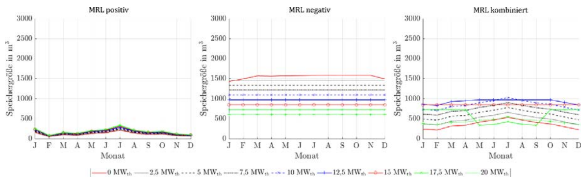
Abbildung 275: Benötigte Speichergrößen bei Angebot von positiver, negativer und kombinierter MRL des ORC-Referenz-Geothermie-Kraftwerks mit Einsatz eines Thermalwasserspeichers im Kraftwerk für Fernwärmenetzleistungen von 0 MW th bis 20 MW th bei einer 4h-Zeitscheibe Einspeicherung und einer Zeitscheibe Angebotszeitraum.
