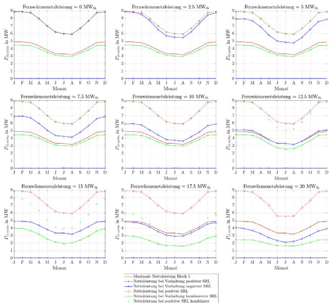
Abbildung 290: Stationäre Sekundärregelleistungen des ORC-Referenz-Geothermie-Kraftwerks mit Einsatz eines Thermalwasserspeichers für Fernwärmenetzleistungen von 0 MW th bis 20 MW th bei zwei 4h-Zeitscheiben Einspeicherung und zwei aufeinanderfolgenden Zeitscheiben Angebotszeitraum.
