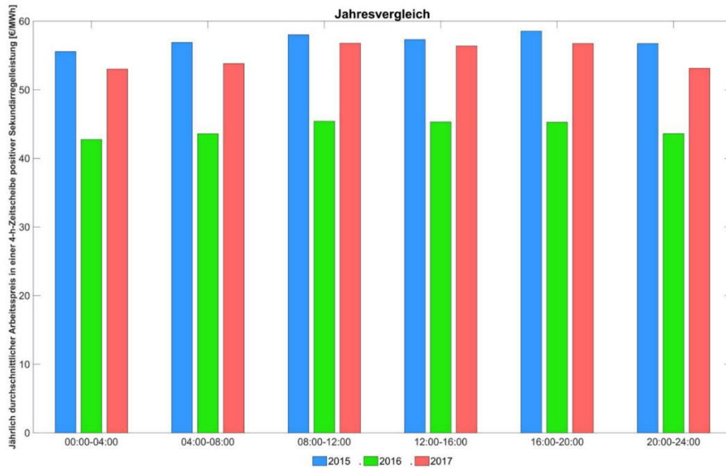
Abbildung 230: Jährlich durchschnittlicher Arbeitspreis in einer 4h-Zeitscheibe positiver Sekundärregelenergie.
