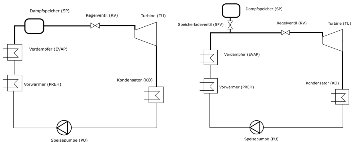
Abbildung 97: Verfahrensfliessbilder der Integration eines Dampfspeichers in das Kraftwerk einer Geothermianlage [98].
