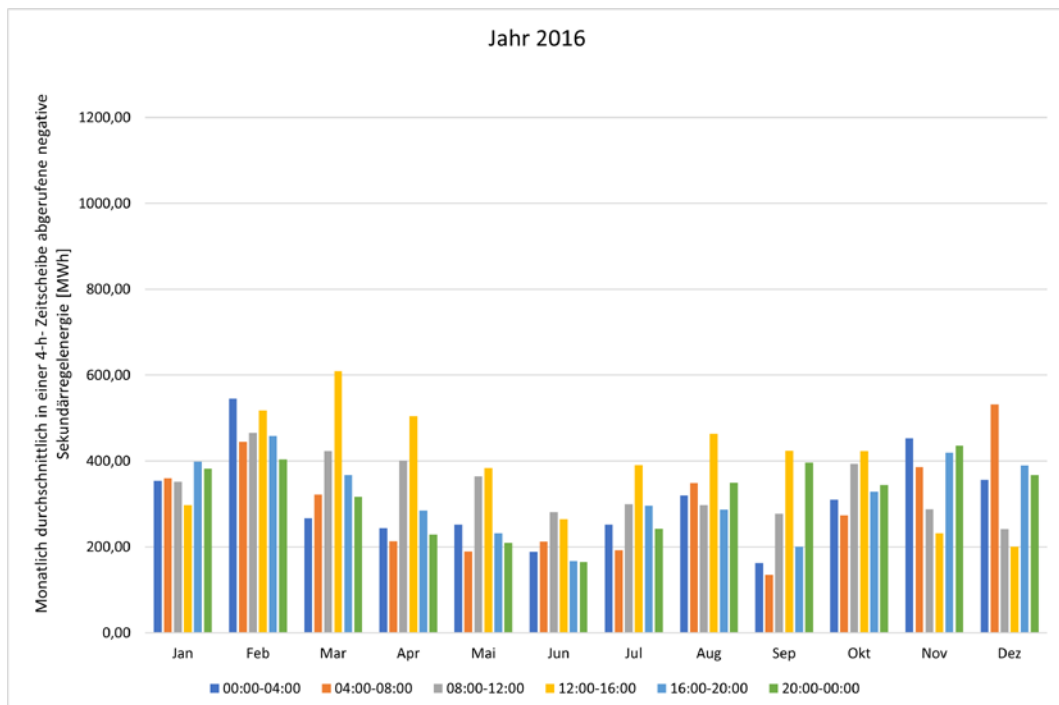
Abbildung 216: Monatlich durchschnittlich in einer 4h-Zeitscheibe abgerufene negative Sekundärregelleistung 2016.
