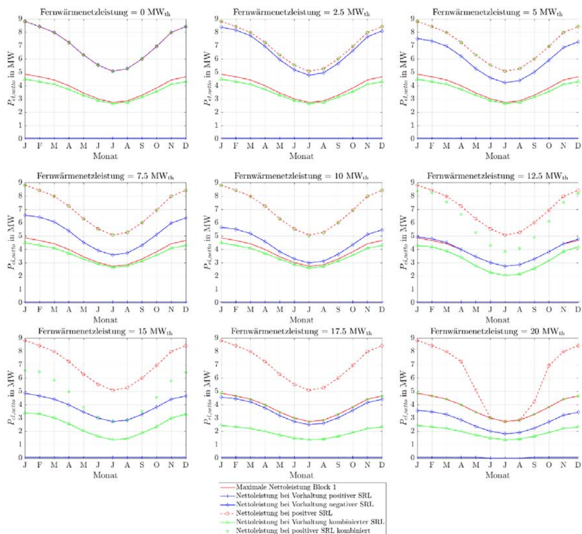
Abbildung 292: Stationäre Sekundärregelleistungen des ORC-Referenz-Geothermie-Kraftwerks mit Einsatz eines Heißwasser-Wärmespeichers des Heiz- und Kraftwerks für Fernwärmenetzleistungen von 0 MW th bis 20 MW th bei zwei 4h-Zeitscheiben Einspeicherung und zwei aufeinanderfolgenden Zeitscheiben Angebotszeitraum.
