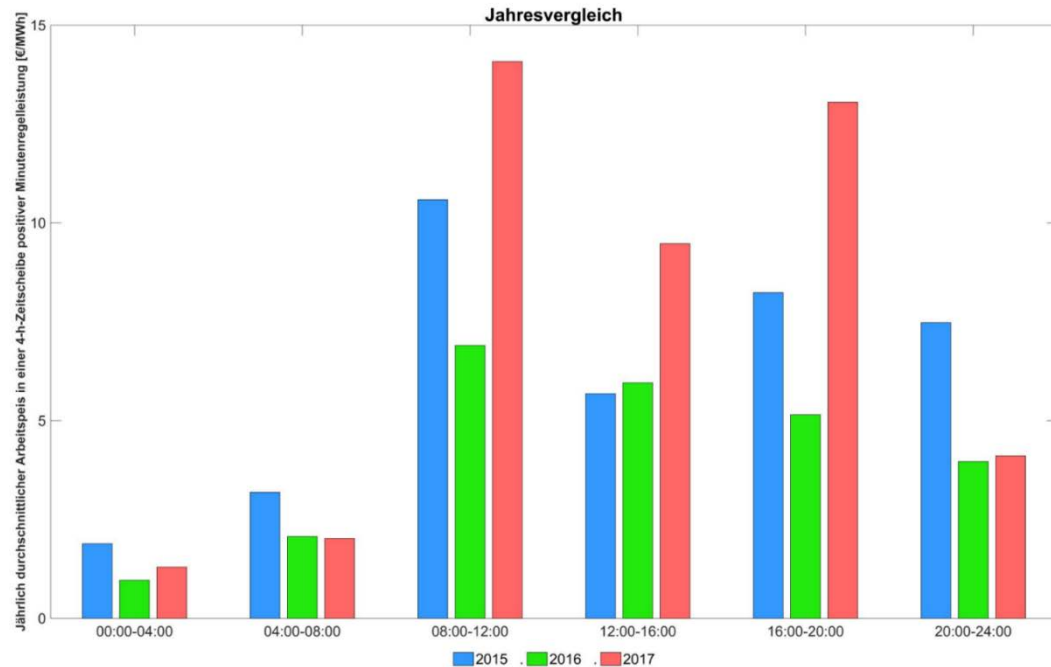
Abbildung 262: Jährlich durchschnittlicher Arbeitspreis in einer 4h-Zeitscheibe positiver Minutenregelenergie.
