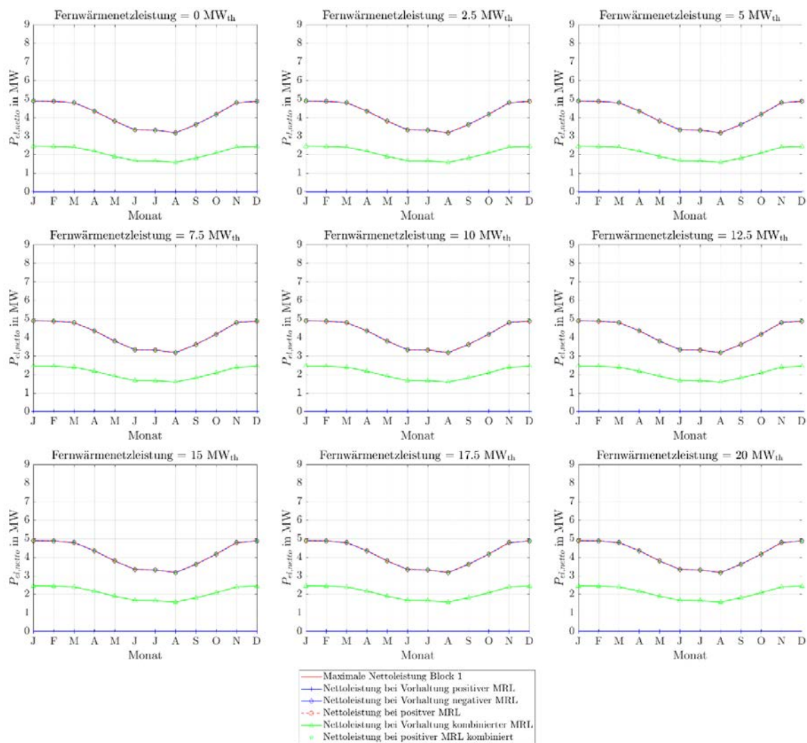
Abbildung 278: Stationäre Minutenregelleistungen des ORC-Referenz-Geothermie-Kraftwerks mit Einsatz eines Heißwasser-Wärmespeichers im Fernwärmenetz für Fernwärmenetzleistungen von 0 MW th bis 20 MW th bei zwei 4h-Zeitscheiben Einspeicherung und einer Zeitscheibe Angebotszeitraum.
