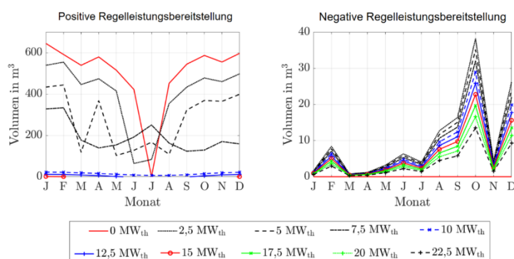
Abbildung 197: Benötigte Speichervolumina für die stationären Sekundärregelleistungen des Kalina-Referenz-Geothermie-Kraftwerks mit Einsatz eines Heißwasser-Wärmespeichers für Fernwärmenetzleistungen von 0 MW th bis 22,5 MW th .
