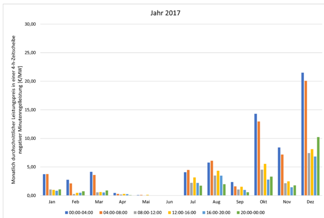
Abbildung 243: Monatlich durchschnittlicher Leistungspreis in einer 4h-Zeitscheibe negativer Minutenregelleistung 2017.
