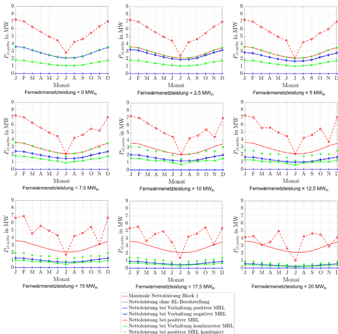
Abbildung 192: Stationäre Minutenregelleistungen des Kalina-Referenz-Geothermie-Kraftwerks mit Einsatz eines Thermalwasserspeichers für Fernwärmenetzleistungen von 0 MW th bis 20 MW th .
