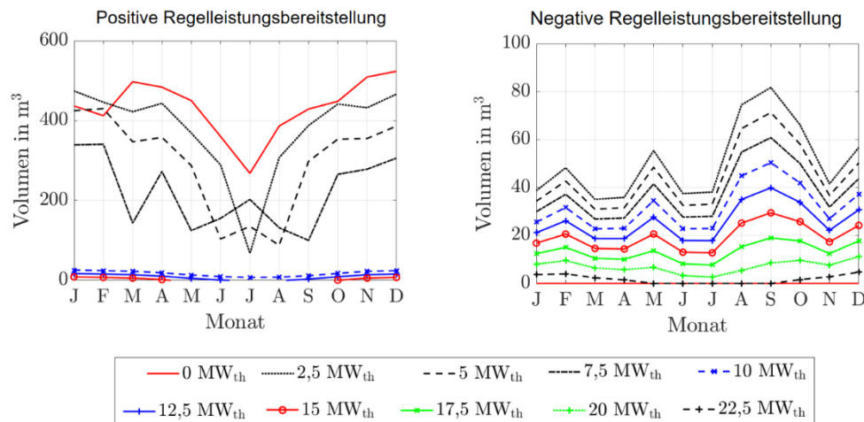
Abbildung 86: Benötigte Speichervolumina für die stationären Sekundärregelleistungen des ORC-Referenz-Geothermie-Kraftwerks mit Einsatz eines Thermalwasserspeichers für Fernwärmenetzleistungen von 0 MW th bis 22,5 MW th .
