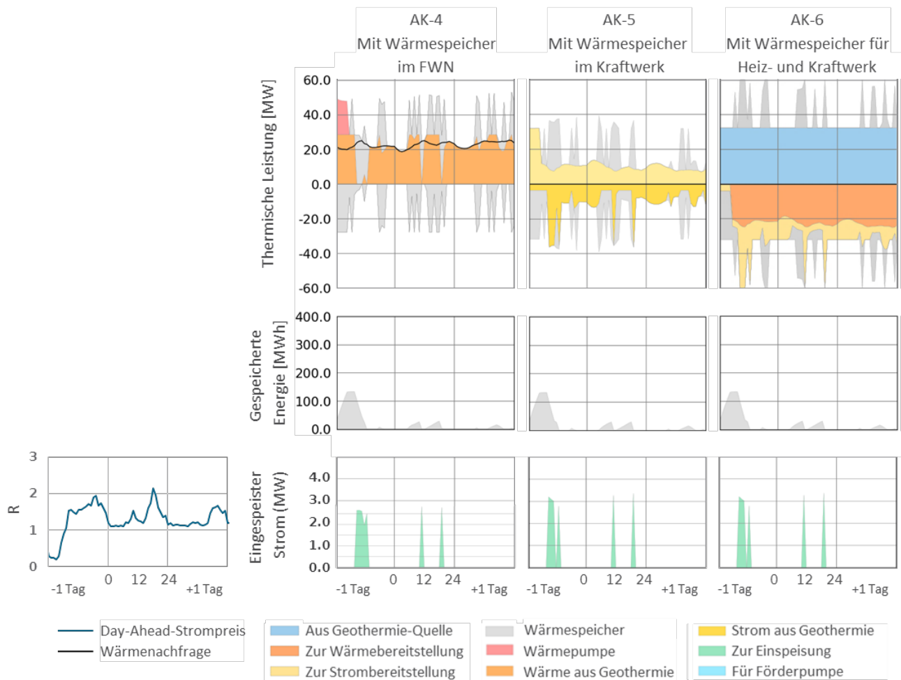
Abbildung 168: Strompreis und Energieträgerfluss an drei aufeinanderfolgenden Wintertagen (hoch) für Anlagekonfigurationen mit Wärmespeichertechnologien: Wärmespeicher im Fernwärmenetz (AK-4), Wärmespeicher im Kraftwerk (AK-5) und Wärmespeicher für den Heiz- und Kraftwerk (AK-6).
