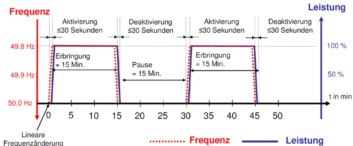
Abbildung 3: Musterprotokoll für die Erbringung von positiver Primärregelleistung [3].
