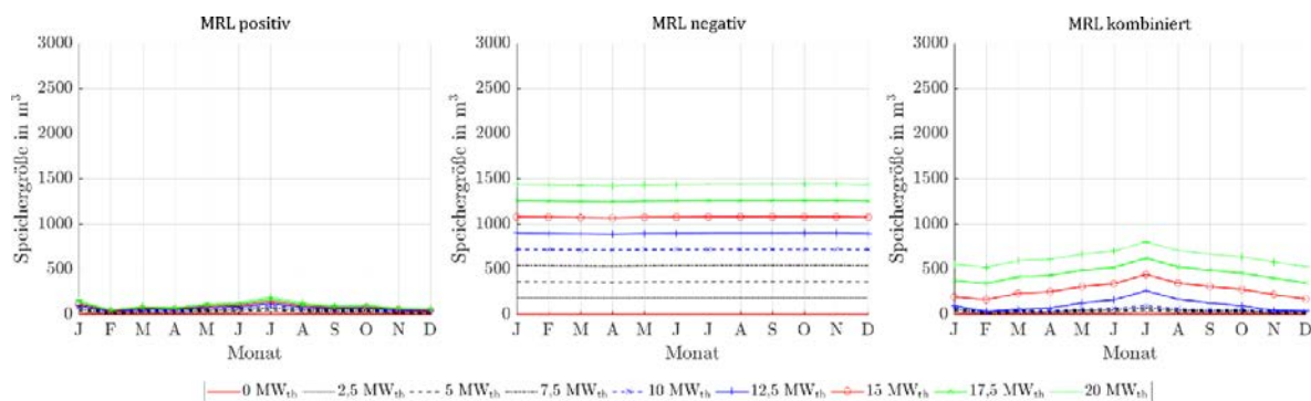
Abbildung 279: Benötigte Speichergrößen bei Angebot von positiver, negativer und kombinierter MRL des ORC-Referenz-Geothermie-Kraftwerks mit Einsatz eines Heißwasser-Wärmespeichers im Fernwärmenetz für Fernwärmenetzleistungen von 0 MW th bis 20 MW th bei zwei 4h-Zeitscheiben Einspeicherung und einer Zeitscheibe Angebotszeitraum.
