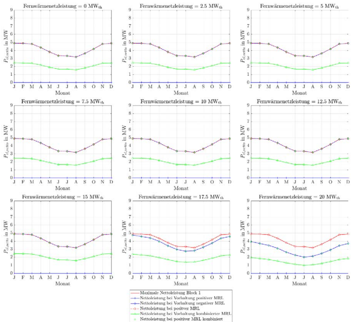
Abbildung 272: Stationäre Minutenregelleistungen des ORC-Referenz-Geothermie-Kraftwerks mit Einsatz eines Heißwasser-Wärmespeichers im Fernwärmenetz für Fernwärmenetzleistungen von 0 MW th bis 20 MW th bei einer 4h-Zeitscheibe Einspeicherung und einer Zeitscheibe Angebotszeitraum.
