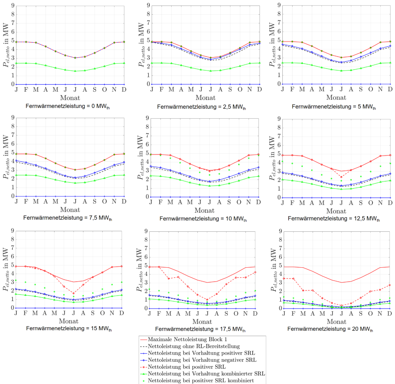
Abbildung 77: Stationäre Sekundärregelleistungen des ORC-Referenz-Geothermie-Kraftwerks mit Einsatz eines Fernwärmenetzspeichers für Fernwärmenetzleistungen von 0 MW th bis 20 MW th .
