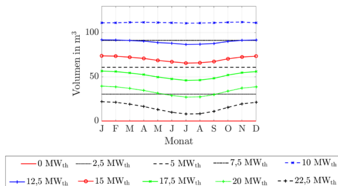
Abbildung 195: Benötigte Speichervolumina für die stationären Primärregelleistungen des Kalina-Referenz-Geothermie-Kraftwerks mit Einsatz eines Heißwasser-Wärmespeichers für Fernwärmenetzleistungen von 0 MW th bis 22,5 MW th .
