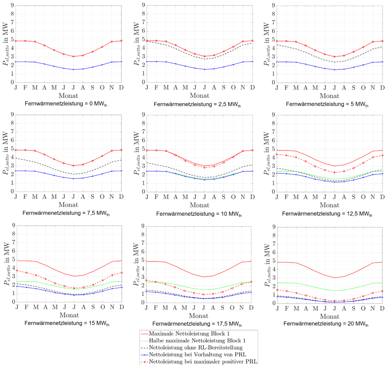
Abbildung 75: Stationäre Primärregelleistungen des ORC-Referenz-Geothermie-Kraftwerks mit Einsatz eines Fernwärmenetzspeichers für Fernwärmenetzleistungen von 0 MW th bis 20 MW th .
