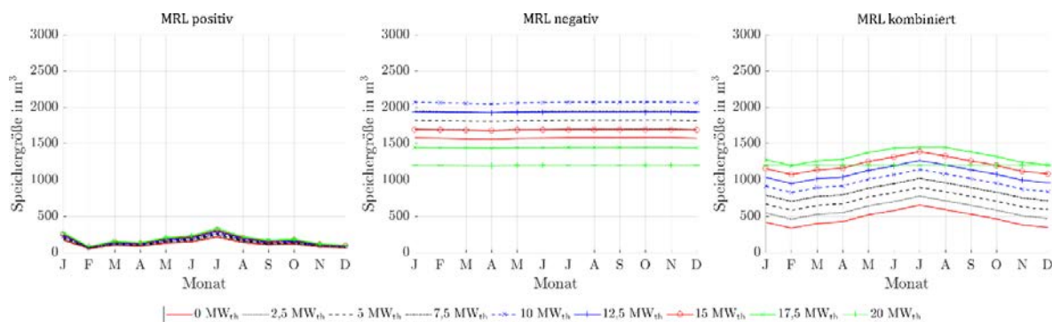
Abbildung 283: Benötigte Speichergrößen bei Angebot von positiver, negativer und kombinierter MRL des ORC-Referenz-Geothermie-Kraftwerks mit Einsatz eines Heißwasser-Wärmespeichers des Heiz- und Kraftwerks für Fernwärmenetzleistungen von 0 MW th bis 20 MW th bei zwei 4h-Zeitscheiben Einspeicherung und einer Zeitscheibe Angebotszeitraum.
