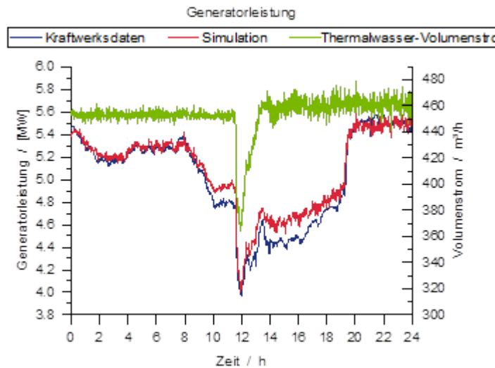
Abbildung 63: Simulations- und Kraftwerksdaten der elektrischen Leistungsabgabe des Gesamtsystems einer ORC-Zweidruckanlage.
