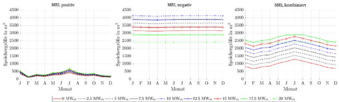
Abbildung 329: Benötigte Speichergrößen bei Angebot von positiver, negativer und kombinierter MRL des Referenz-Geothermie-Kraftwerks mit Einsatz eines Heißwasser-Wärmespeichers des Heiz- und Kraftwerks für Fernwärmenetzleistungen von 0 MW th bis 20 MW th bei vier 4h-Zeitscheiben Einspeicherung und zwei aufeinanderfolgenden Zeitscheiben Angebotszeitraum.
