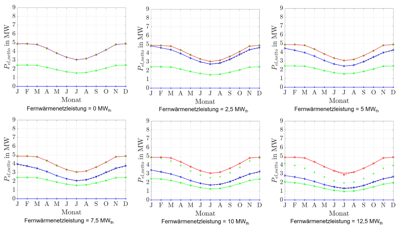
Abbildung 79: Stationäre Minutenregelleistungen des ORC-Referenz-Geothermie-Kraftwerks mit Einsatz eines Fernwärmenetzspeichers für Fernwärmenetzleistungen von 0 MW th bis 20 MW th .
