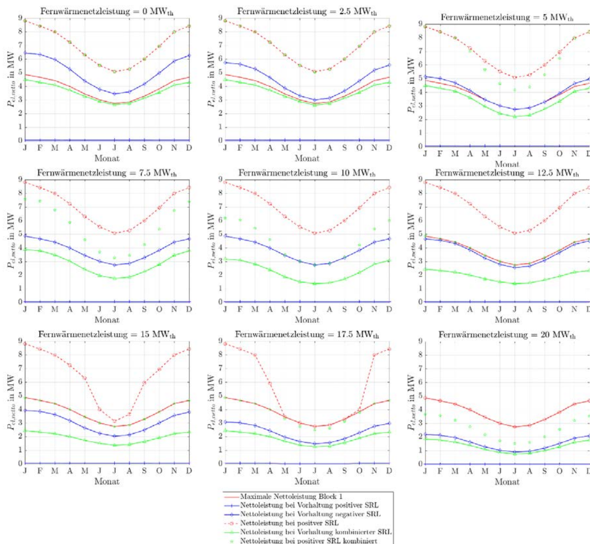
Abbildung 117: Stationäre Sekundärregelleistungen des ORC-Referenz-Geothermie-Kraftwerks mit Einsatz eines Heißwasser-Wärmespeichers des Heiz- und Kraftwerks für Fernwärmenetzleistungen von 0 MW th bis 20 MW th bei einer 4h-Zeitscheibe Einspeicherung und zwei aufeinanderfolgenden Zeitscheiben Angebotszeitraum.
