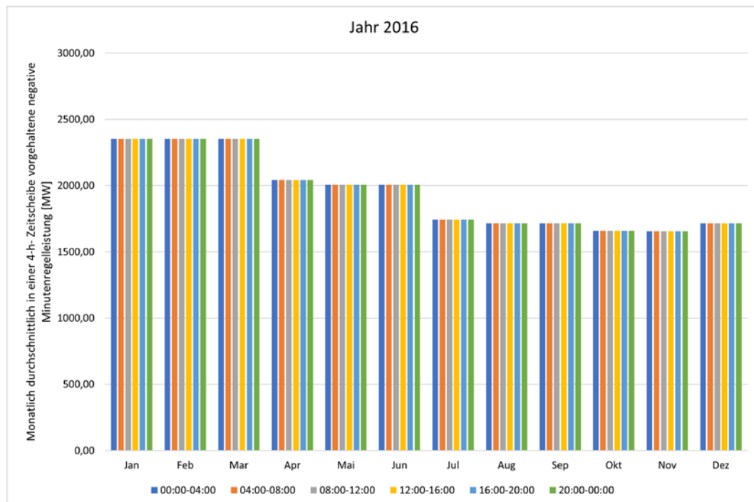
Abbildung 236: Monatlich durchschnittlich in einer 4h-Zeitscheibe vorgehaltene negative Minutenregel-leistung 2016.
