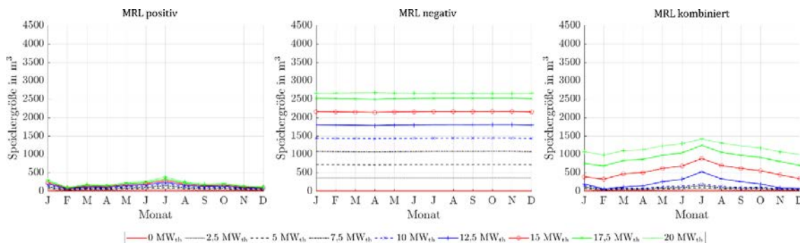
Abbildung 319: Benötigte Speichergrößen bei Angebot von positiver, negativer und kombinierter MRL des ORC-Referenz-Geothermie-Kraftwerks mit Einsatz eines Heißwasser-Wärmespeichers im Fernwärmenetz für Fernwärmenetzleistungen von 0 MW th bis 20 MW th bei drei 4h-Zeitscheiben Einspeicherung und zwei aufeinanderfolgenden Zeitscheiben Angebotszeitraum.
