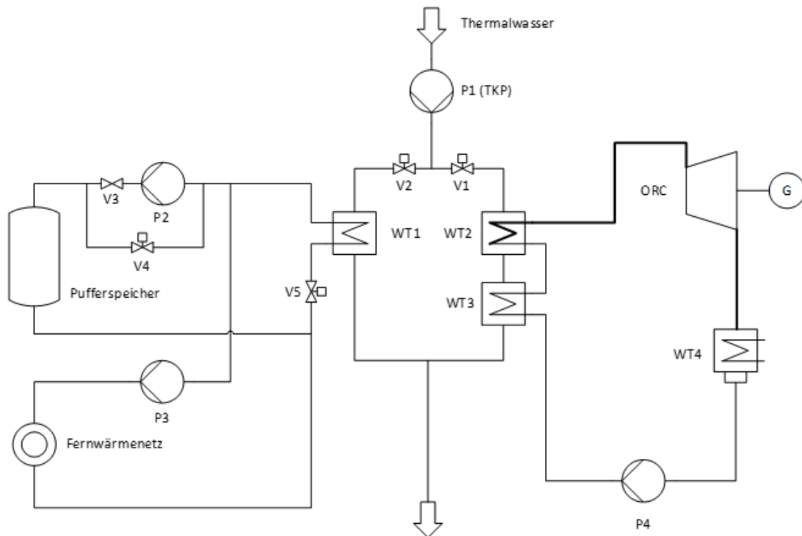
Abbildung 33: Verfahrensfließbild einer Geothermieranlage mit parallel geschaltetem Heiz- und Kraftwerk und einem in das Fernwärmenetz integrierten Heißwasser-Wärmespeicher.
