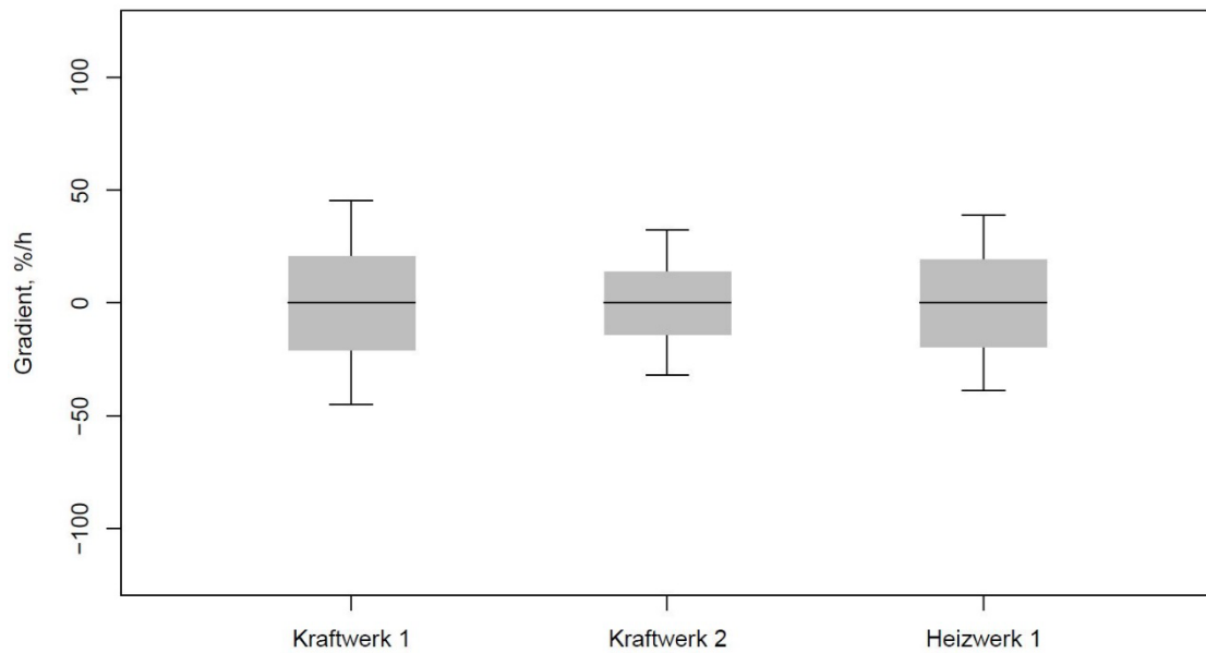
Abbildung 26: Prozentuale Veränderung des Volumenstroms für Geothermiekraftwerke und -heizwerke im Bayerischen Molassebecken.
