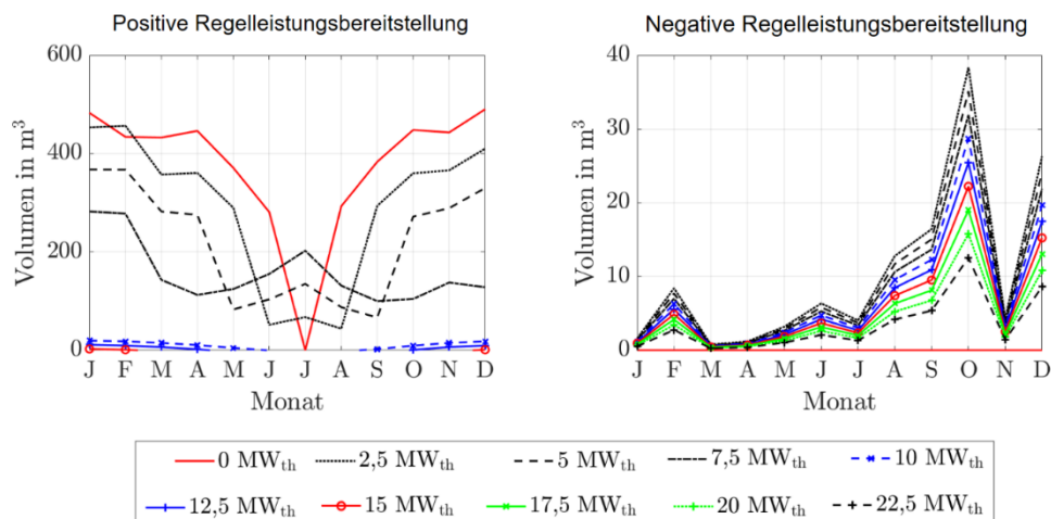
Abbildung 94: Benötigte Speichervolumina für die stationären Sekundärregelungen des ORC-Referenz-Geothermie-Kraftwerks mit Einsatz eines Heißwasser-Wärmespeichers für Fernwärmenetzleistungen von 0 \text{MW}_{\text{th}} bis 22,5 \text{MW}_{\text{th}} .
