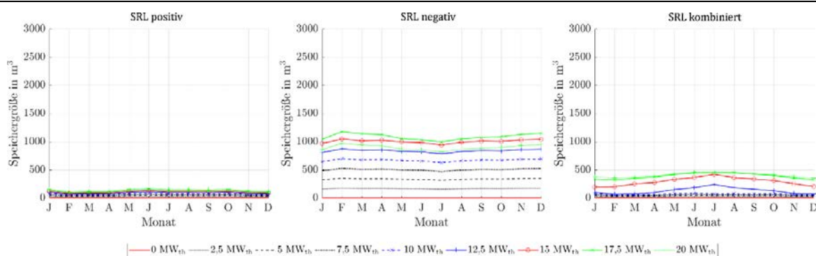
Abbildung 106: Benötigte Speichergrößen bei Angebot von positiver, negativer und kombinierter SRL des ORC-Referenz-Geothermie-Kraftwerks mit Einsatz eines Heißwasser-Wärmespeichers im Fernwärmenetz für Fernwärmenetzleistungen von 0 MW th bis 20 MW th bei einer 4h-Zeitscheibe Einspeicherung und einer Zeitscheibe Angebotszeitraum.
