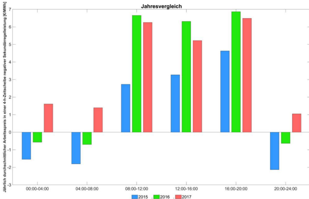
Abbildung 231: Jährlich durchschnittlicher Arbeitspreis in einer 4h-Zeitscheibe negativer Sekundärregelenergie.
