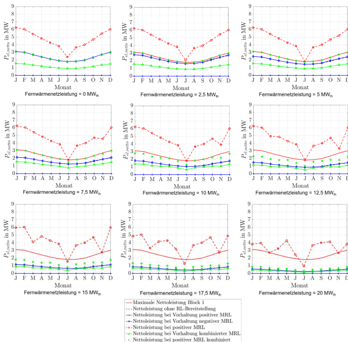
Abbildung 198: Stationäre Minutenregelleistungen des Kalina-Referenz-Geothermie-Kraftwerks mit Einsatz eines Heißwasser-Wärmespeichers für Heiz- und Kraftwerk für Fernwärmenetzleistungen von 0 MW th bis 20 MW th .
