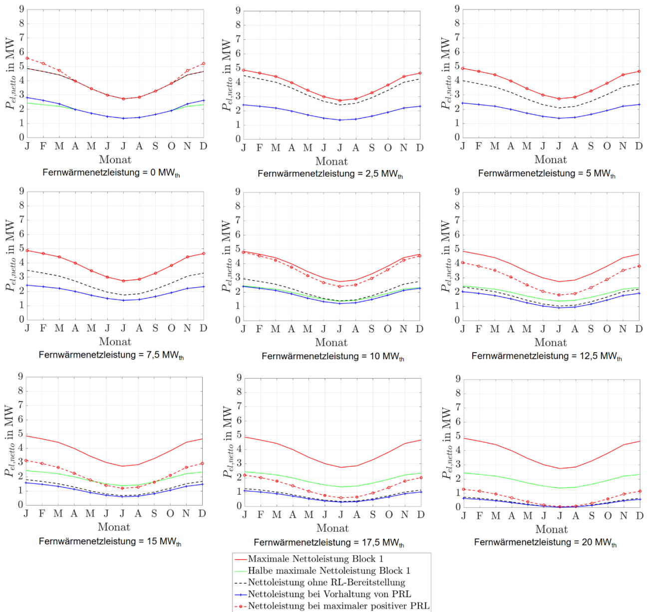
Abbildung 91: Stationäre Primärregelleistungen des ORC-Referenz-Geothermie-Kraftwerks mit Einsatz eines Heißwasser-Wärmespeichers für Heiz- und Kraftwerk für Fernwärmenetzleistungen von 0 MW th bis 20 MW th .
