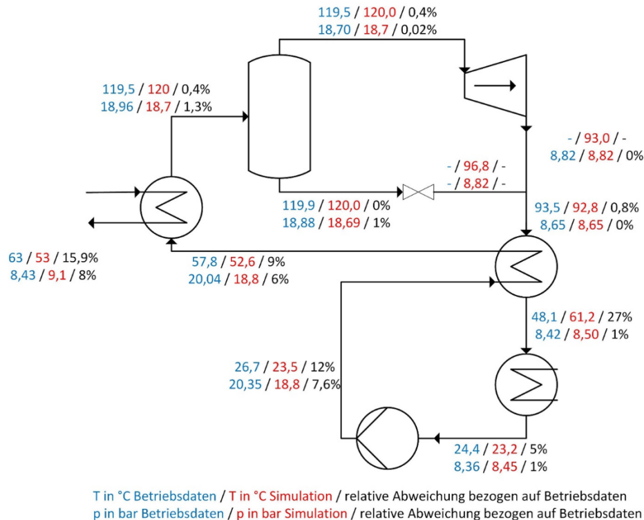
Abbildung 59: Validierung des Simulationsmodells des Kalina-Referenz-Geothermie-Kraftwerks im Standardbetriebspunkt des Jahres 2016.
