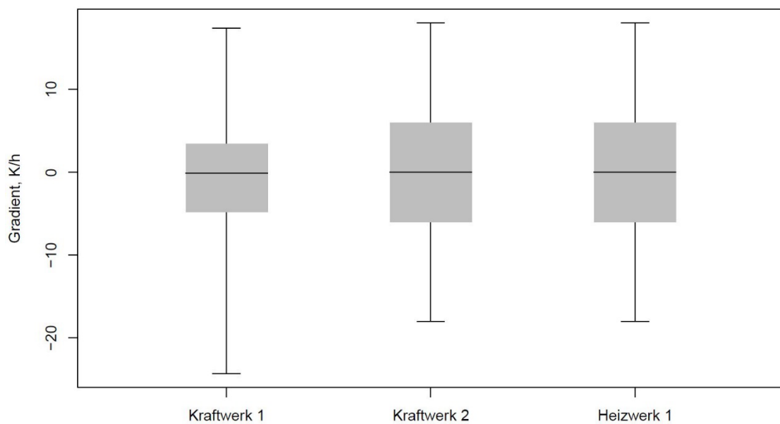
Abbildung 27: Gradienten der Injektionstemperatur für Geothermiekraftwerke und -heizwerke im Bayerischen Molassebecken.
