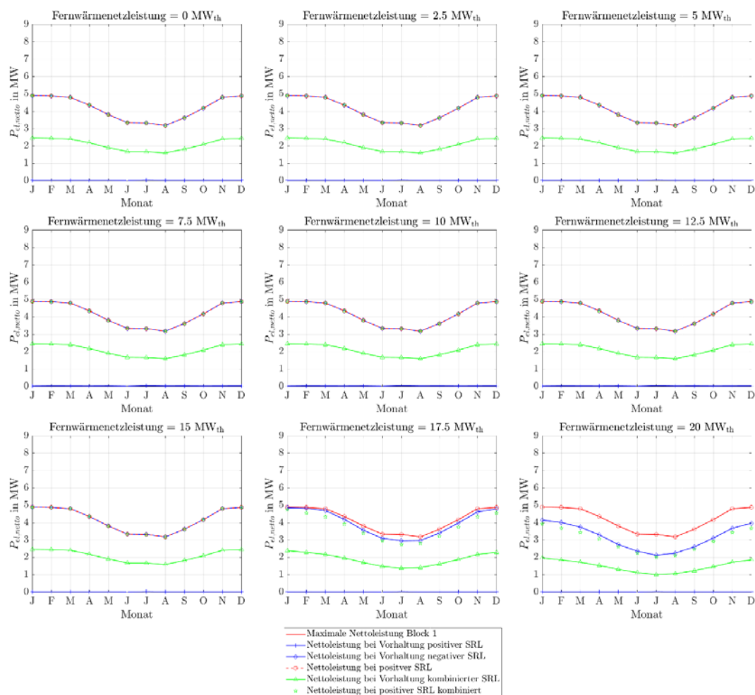
Abbildung 288: Stationäre Sekundärregelleistungen des Referenz-Geothermie-Kraftwerks mit Einsatz eines Heißwasser-Wärmespeichers im Fernwärmenetz für Fernwärmenetzleistungen von 0 MW th bis 20 MW th bei zwei 4h-Zeitscheiben Einspeicherung und zwei aufeinanderfolgenden Zeitscheiben Angebotszeitraum..
