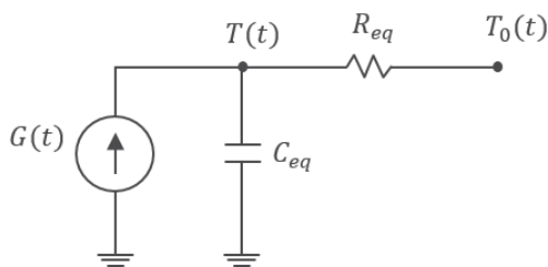
Abbildung 171: 1R1C Einzelzone Gebäudemodell.
