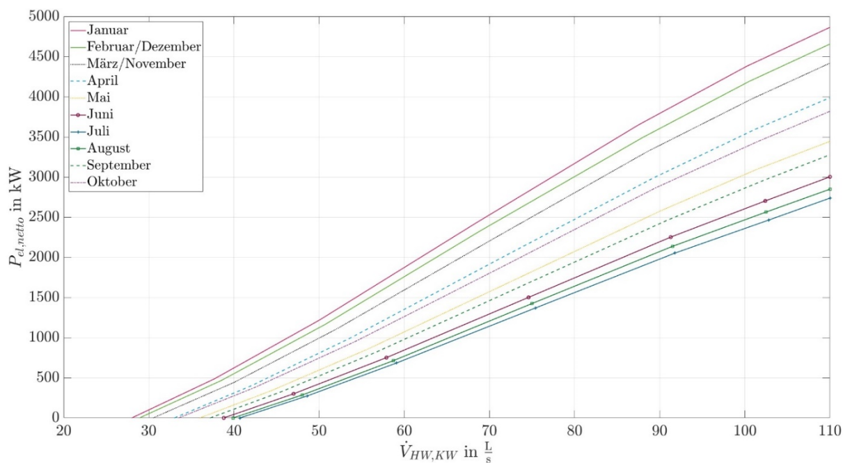
Abbildung 89: Nettoleistungs-Thermalwasservolumenstrom-Diagramm des ersten Kraftwerksblocks des ORC-Referenz-Geothermie-Kraftwerks mit einer Heißwassertemperatur von 135 °C bei Eintritt in den Kraftwerksblock.
