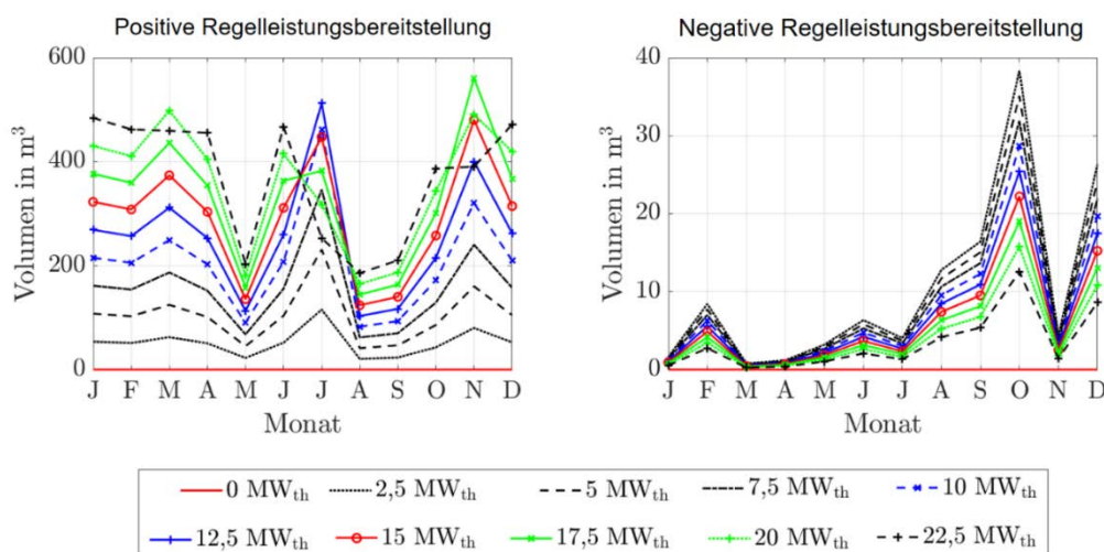
Abbildung 80: Benötigte Speichervolumina für die stationären Minutenregelleistungen des ORC-Referenz-Geothermie-Kraftwerks mit Einsatz eines Fernwärmenetzspeichers für Fernwärmenetzleistungen von 0 MW th bis 22,5 MW th .
