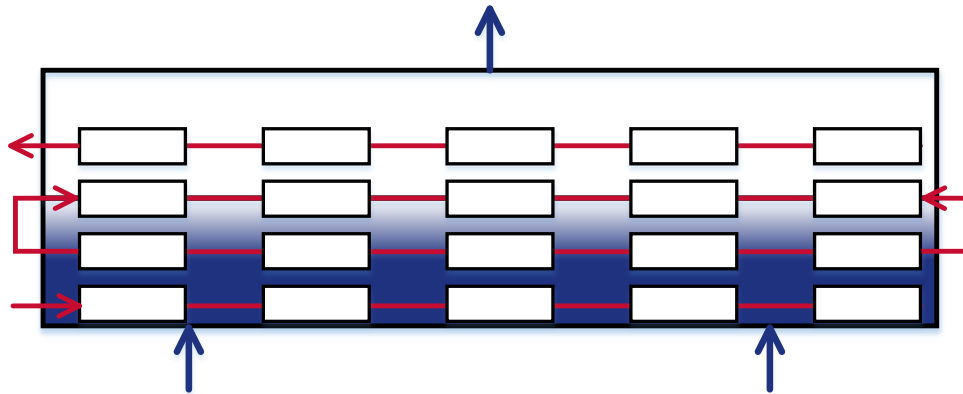
Abbildung 61: Skizze der modelltechnischen Umsetzung der Verdampfer der ORC-Zweidruckanlage (in Rot: Thermalwasserstrom; in Blau: ORC-Massenstrom).
