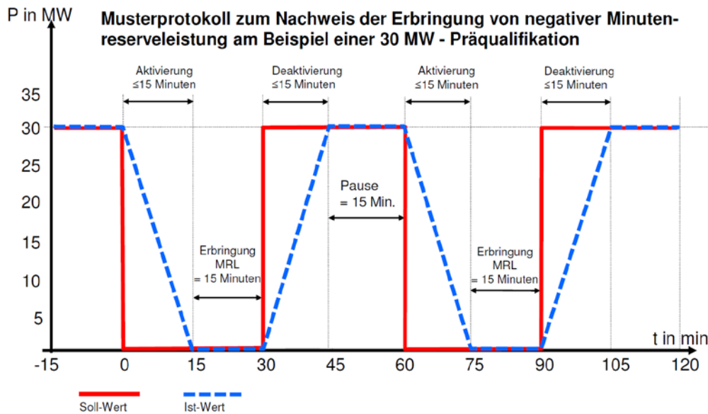
Abbildung 5: Musterprotokoll für die Erbringung von negativer Minutenregelleistung [84].
