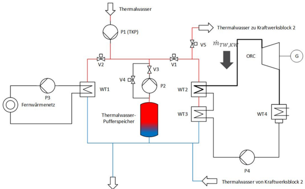
Abbildung 37: Verfahrensfließbild einer Geothermieranlage mit parallel geschaltetem Heiz- und Kraftwerk und einem in das Kraftwerk integrierten Thermalwasser-Pufferspeicher – positive Regelleistungsbereitstellung – Entladevorgang des Thermalwasser-Wärmespeichers.
