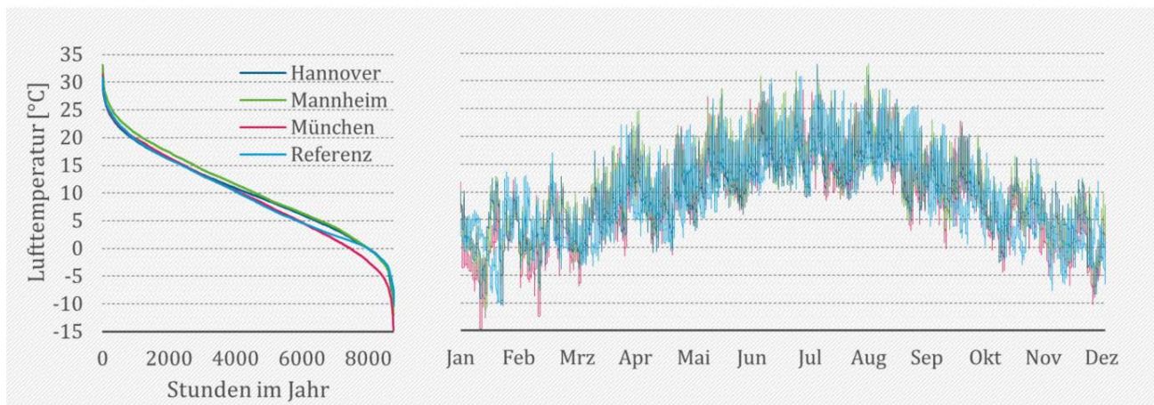
Abbildung 164: Lufttemperaturdauerkurve der Referenzregion Unterhaching und der drei repräsentativen Städte Hannover, Mannheim und München.
