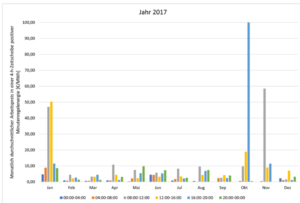
Abbildung 252: Monatlich durchschnittlicher Arbeitspreis in einer 4h-Zeitscheibe positiver Minutenregelleistung 2017.
