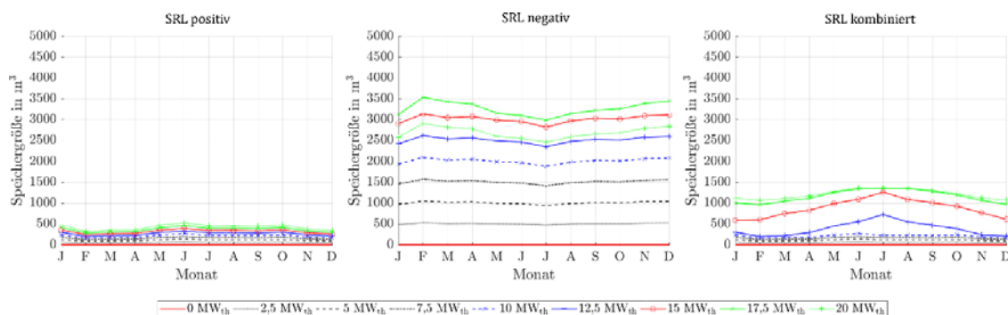
Abbildung 120: Benötigte Speichergrößen bei Angebot von positiver, negativer und kombinierter SRL des ORC-Referenz-Geothermie-Kraftwerks mit Einsatz eines Heißwasser-Wärmespeichers im Fernwärmenetz für Fernwärmenetzleistungen von 0 MW th bis 20 MW th bei drei 4h-Zeitscheiben Einspeicherung und zwei aufeinanderfolgenden Zeitscheiben Angebotszeitraum.
