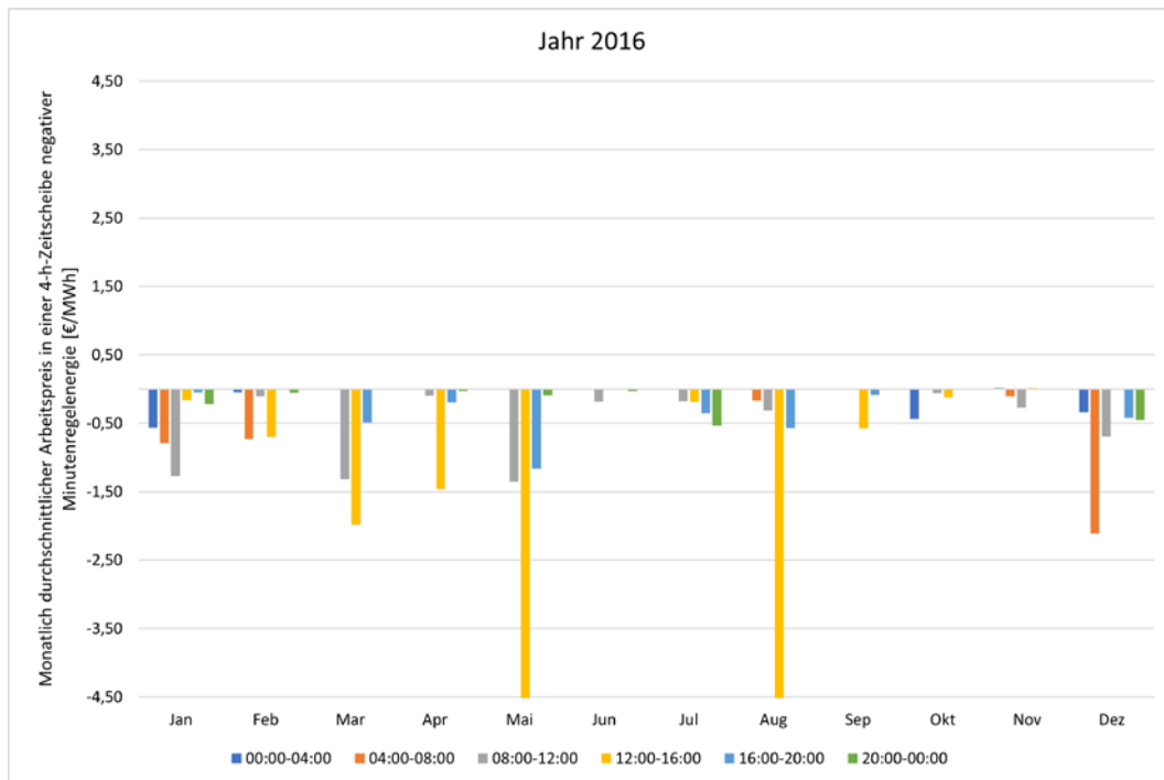
Abbildung 254: Monatlich durchschnittlicher Arbeitspreis in einer 4h-Zeitscheibe negativer Minutenregelleistung 2016.
