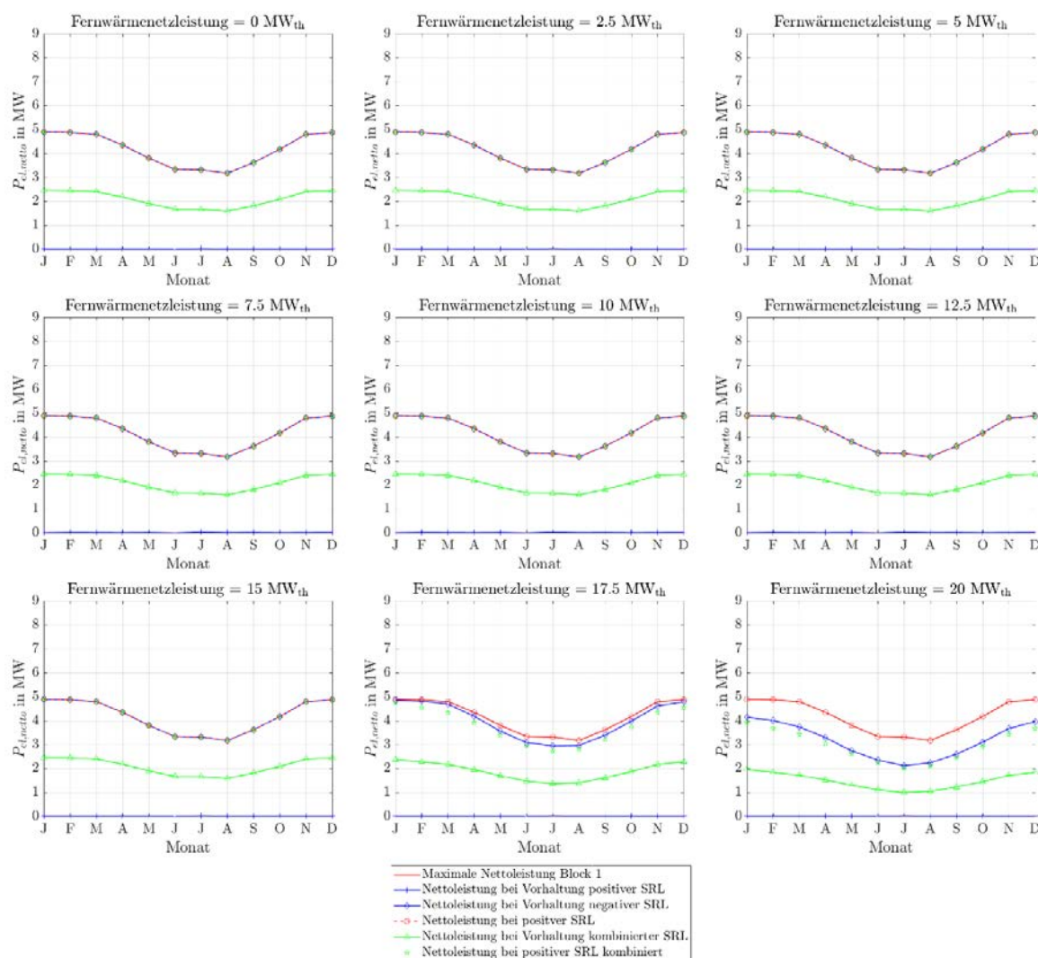
Abbildung 105: Stationäre Sekundärregelleistungen des ORC-Referenz-Geothermie-Kraftwerks mit Einsatz eines Heißwasser-Wärmespeichers im Fernwärmenetz für Fernwärmenetzleistungen von 0 MW th bis 20 MW th bei einer 4h-Zeitscheibe Einspeicherung und einer Zeitscheibe Angebotszeitraum.
