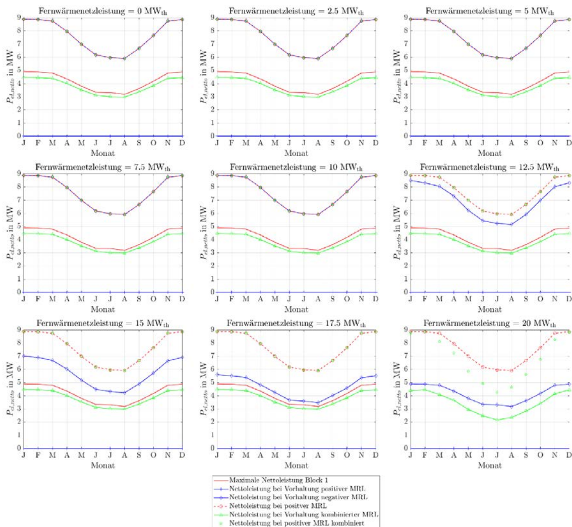
Abbildung 326: Stationäre Minutenregelleistungen des ORC-Referenz-Geothermie-Kraftwerks mit Einsatz eines Thermalwasserspeichers für Fernwärmenetzleistungen von 0 MW th bis 20 MW th bei vier 4h-Zeitscheiben Einspeicherung und zwei aufeinanderfolgenden Zeitscheiben Angebotszeitraum.
