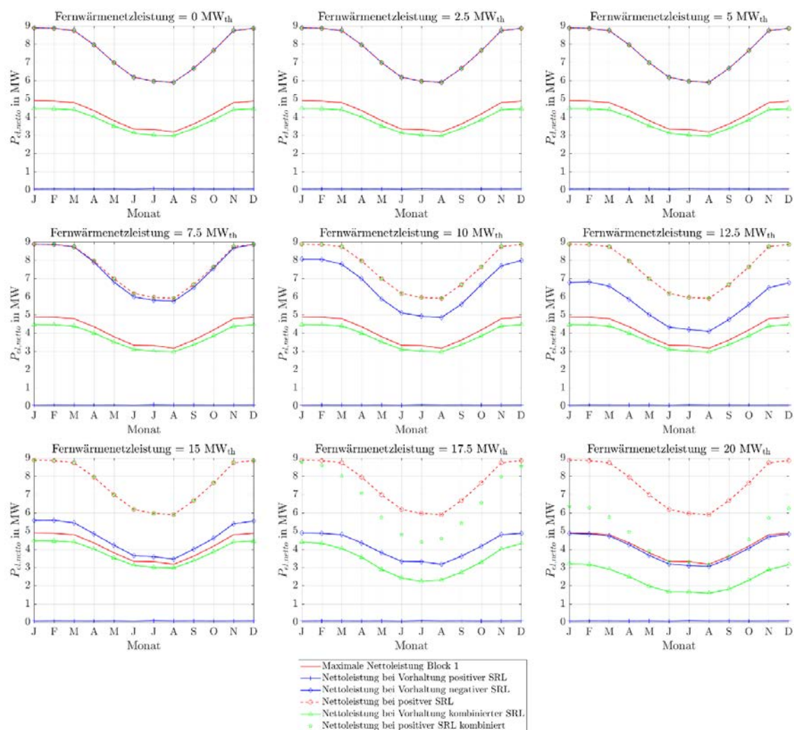
Abbildung 296: Stationäre Sekundärregelleistungen des ORC-Referenz-Geothermie-Kraftwerks mit Einsatz eines Thermalwasserspeichers für Fernwärmenetzleistungen von 0 MW th bis 20 MW th bei drei 4h-Zeitscheiben Einspeicherung und zwei aufeinanderfolgenden Zeitscheiben Angebotszeitraum.
