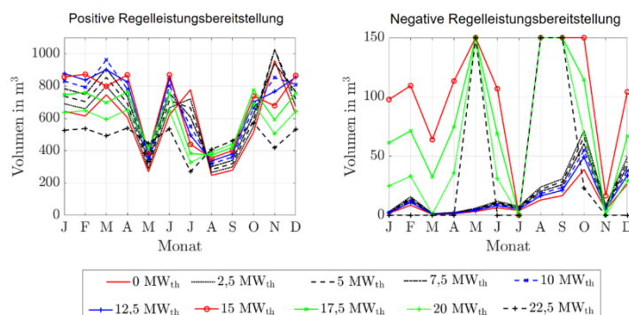
Abbildung 193: Benötigte Speichervolumina für die stationären Minutenregelleistungen des Kalina-Referenz-Geothermie-Kraftwerks mit Einsatz eines Thermalwasserspeichers für Fernwärmenetzleistungen von 0 MW th bis 22,5 MW th .
