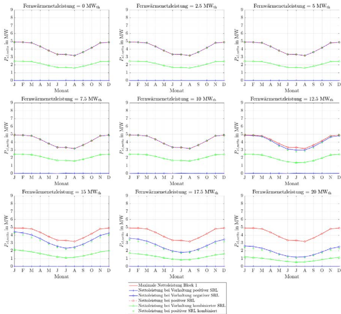
Abbildung 113: Stationäre Sekundärregelleistungen des ORC-Referenz-Geothermie-Kraftwerks mit Einsatz eines Heißwasser-Wärmespeichers im Fernwärmenetz für Fernwärmenetzleistungen von 0 MW th bis 20 MW th bei einer 4h-Zeitscheibe Einspeicherung und zwei aufeinanderfolgenden Zeitscheiben Angebotszeitraum.
