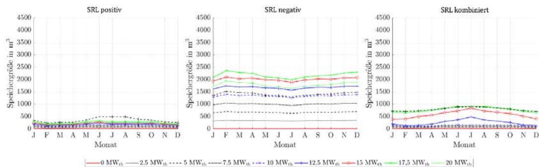
Abbildung 289: Benötigte Speichergrößen bei Angebot von positiver, negativer und kombinierter SRL des ORC-Referenz-Geothermie-Kraftwerks mit Einsatz eines Heißwasser-Wärmespeichers im Fernwärmenetz für Fernwärmenetzleistungen von 0 MW th bis 20 MW th bei zwei 4h-Zeitscheiben Einspeicherung und zwei aufeinanderfolgenden Zeitscheiben Angebotszeitraum.
