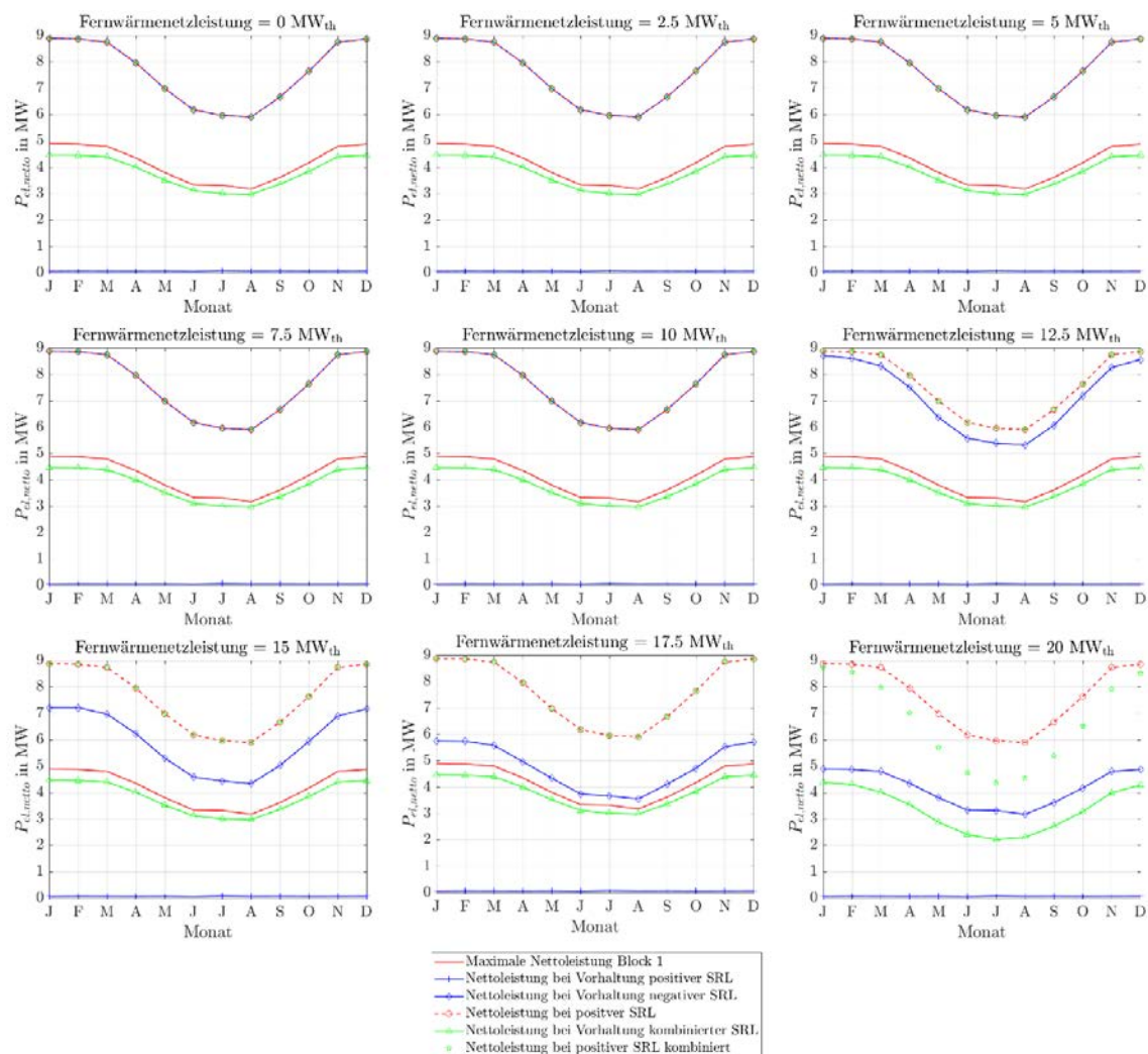
Abbildung 268: Stationäre Sekundärregelleistungen des ORC-Referenz-Geothermie-Kraftwerks mit Einsatz eines Thermalwasserspeichers für Fernwärmenetzleistungen von 0 MW th bis 20 MW th bei zwei 4h-Zeitscheiben Einspeicherung und einer Zeitscheibe Angebotszeitraum.
