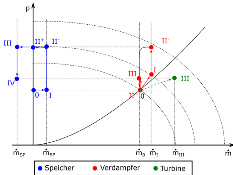
Abbildung 99: p - \dot{m} -Diagramm des Kraftwerksprozesses mit dem Betrieb eines absperrbaren Dampfspeichers [98, S. 36].
