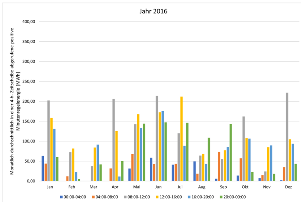
Abbildung 245: Monatlich durchschnittlich in einer 4h-Zeitscheibe abgerufene positive Minutenregelenergie 2016.
