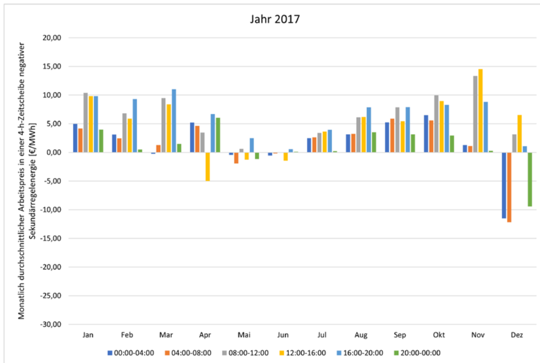
Abbildung 223: Monatlich durchschnittlicher Arbeitspreis in einer 4h-Zeitscheibe negativer Sekundärregelleistung 2017.
