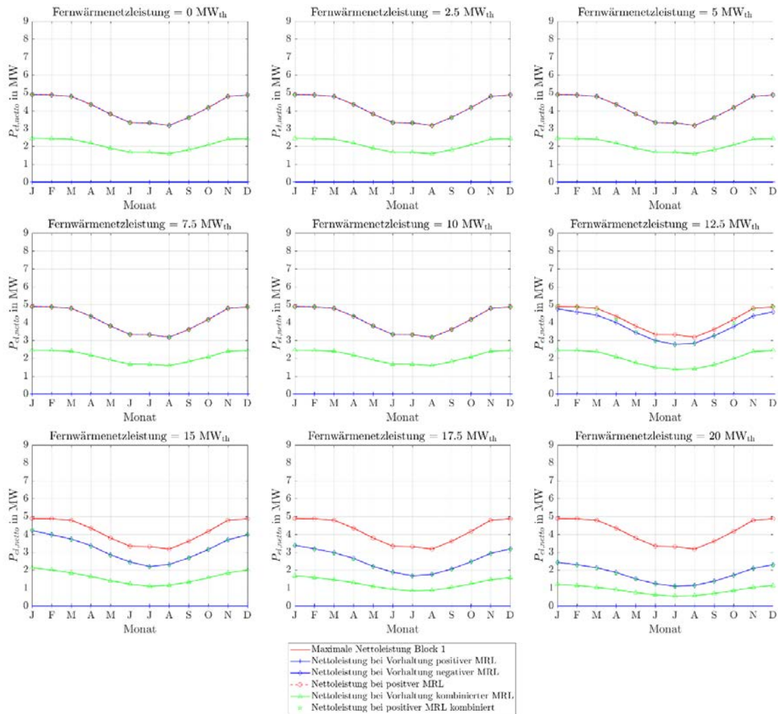
Abbildung 306: Stationäre Minutenregelleistungen des ORC-Referenz-Geothermie-Kraftwerks mit Einsatz eines Heißwasser-Wärmespeichers im Fernwärmenetz für Fernwärmenetzleistungen von 0 MW th bis 20 MW th bei einer 4h-Zeitscheibe Einspeicherung und zwei aufeinanderfolgenden Zeitscheiben Angebotszeitraum.
