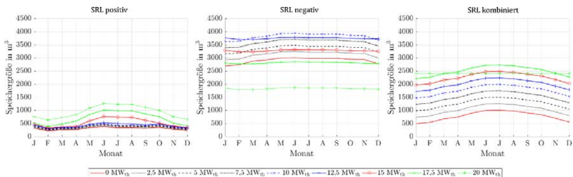
Abbildung 303: Benötigte Speichergrößen bei Angebot von positiver, negativer und kombinierter SRL des Referenz-Geothermie-Kraftwerks mit Einsatz eines Thermalwasserspeichers im Kraftwerk für Fernwärmenetzleistungen von 0 MW th bis 20 MW th bei vier 4h-Zeitscheiben Einspeicherung und zwei aufeinanderfolgenden Zeitscheiben Angebotszeitraum.
