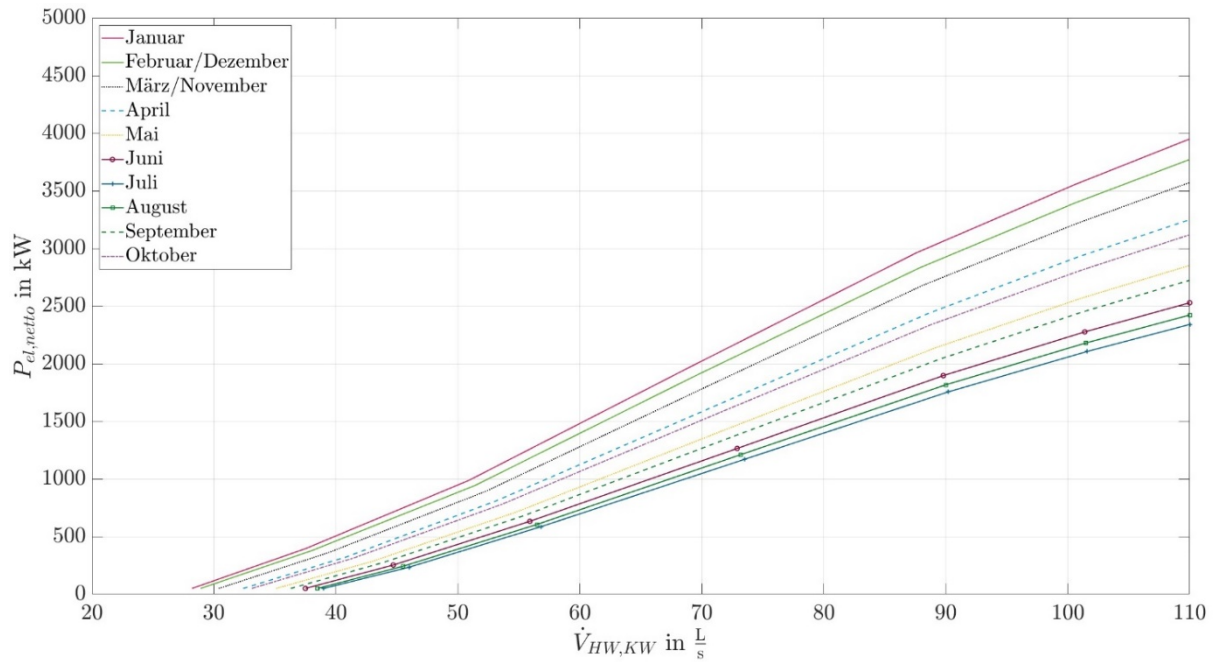
Abbildung 90: Nettoleistungs-Thermalwasservolumenstrom-Diagramm des zweiten Kraftwerksblocks des ORC-Referenz-Geothermie-Kraftwerks mit einer Heißwassertemperatur von 135 °C bei Eintritt in den Kraftwerksblock.
