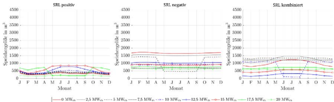
Abbildung 118: Benötigte Speichergrößen bei Angebot von positiver, negativer und kombinierter SRL des ORC-Referenz-Geothermie-Kraftwerks mit Einsatz eines Heißwasser-Wärmespeichers des Heiz- und Kraftwerks für Fernwärmenetzleistungen von 0 MW th bis 20 MW th bei einer 4h-Zeitscheibe Einspeicherung und zwei aufeinanderfolgenden Zeitscheiben Angebotszeitraum.
