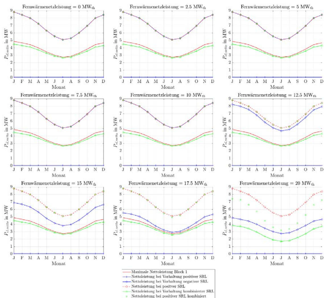
Abbildung 270: Stationäre Sekundärregelleistungen des ORC-Referenz-Geothermie-Kraftwerks mit Einsatz eines Heißwasser-Wärmespeichers des Heiz- und Kraftwerks für Fernwärmenetzleistungen von 0 MW th bis 20 MW th bei zwei 4h-Zeitscheiben Einspeicherung und einer Zeitscheibe Angebotszeitraum.
