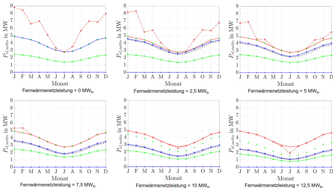
Abbildung 93: Stationäre Sekundärregelleistungen des ORC-Referenz-Geothermie-Kraftwerks mit Einsatz eines Heißwasser-Wärmespeichers für Heiz- und Kraftwerk für Fernwärmenetzleistungen von 0 MW th bis 20 MW th .
