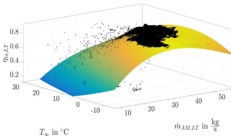
Abbildung 175: Kennfeld des isentropen Wirkungsgrads der LT-Turbine in Abhängigkeit des Arbeitsmittel-Massenstroms und der Umgebungstemperatur mit schwarzen Stützpunkten für die Korrelationsberechnung.
