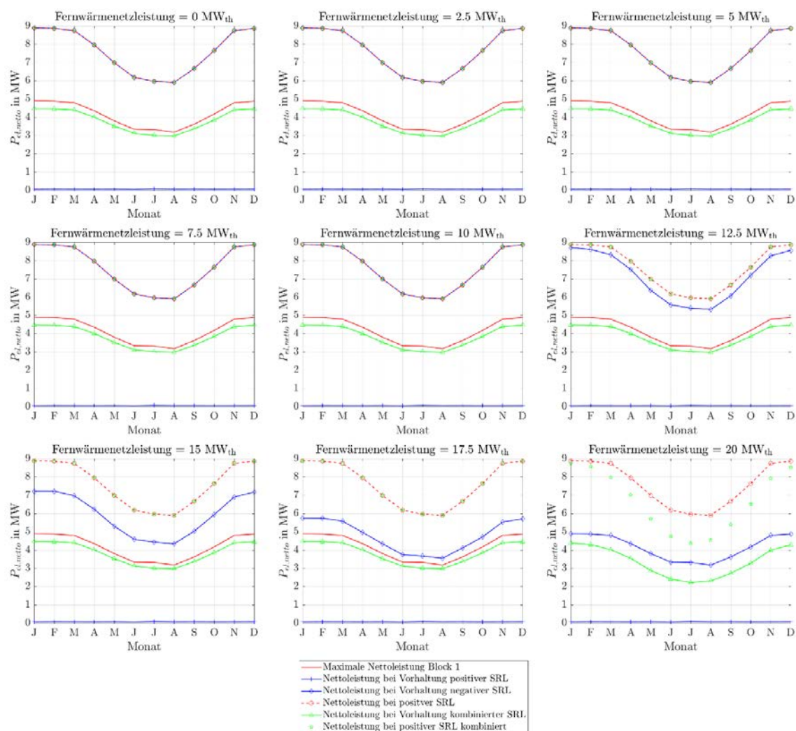
Abbildung 302: Stationäre Sekundärregelleistungen des ORC-Referenz-Geothermie-Kraftwerks mit Einsatz eines Thermalwasserspeichers für Fernwärmenetzleistungen von 0 MW th bis 20 MW th bei vier 4h-Zeitscheiben Einspeicherung und zwei aufeinanderfolgenden Zeitscheiben Angebotszeitraum.
