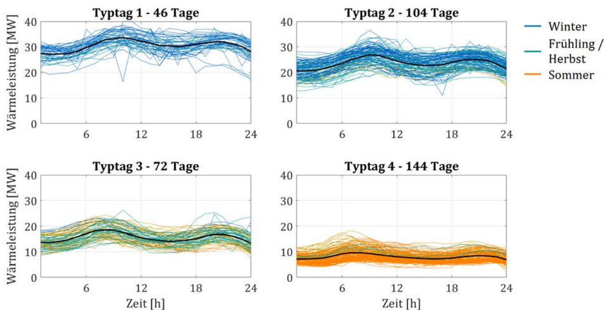
Abbildung 46: Wärmeleistungsprofile von ausgewählten Typtagen. Das schwarze Profil in jedem Plot repräsentiert die durchschnittliche Wärmeleistung für den jeweiligen Typtag.
