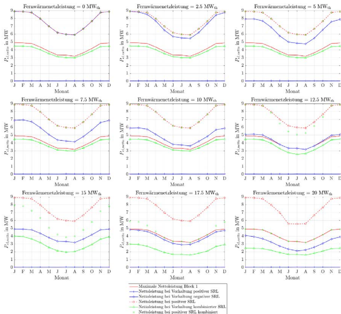
Abbildung 121: Stationäre Sekundärregelleistungen des ORC-Referenz-Geothermie-Kraftwerks mit Einsatz eines Thermalwasserspeichers für Fernwärmenetzleistungen von 0 MW th bis 20 MW th bei drei 4h-Zeitscheiben Einspeicherung und drei aufeinanderfolgenden Zeitscheiben Angebotszeitraum.
