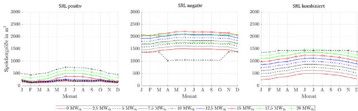
Abbildung 110: Benötigte Speichergrößen bei Angebot von positiver, negativer und kombinierter SRL des ORC-Referenz-Geothermie-Kraftwerks mit Einsatz eines Thermalwasserspeichers im Kraftwerk für Fernwärmenetzleistungen von 0 MW th bis 20 MW th bei drei 4h-Zeitscheiben Einspeicherung und einer Zeitscheibe Angebotszeitraum.
