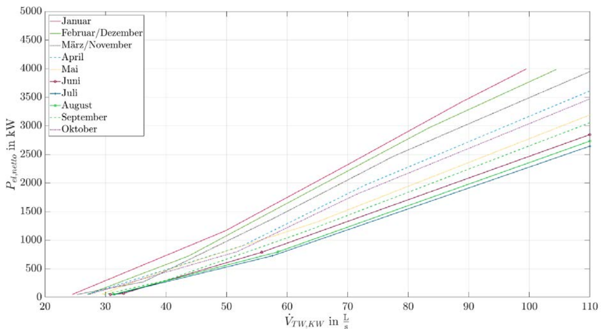
Abbildung 82: Nettoleistungs-Thermalwasservolumenstrom-Diagramm für den zweiten Kraftwerksblock des ORC-Referenz-Geothermie-Kraftwerks.
