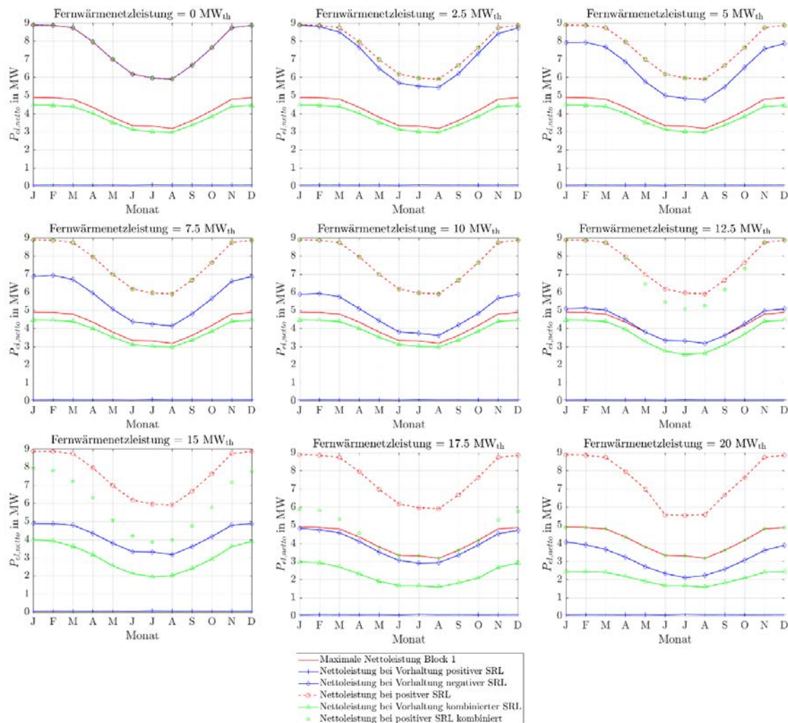
Abbildung 264: Stationäre Sekundärregelleistungen des ORC-Referenz-Geothermie-Kraftwerks mit Einsatz eines Thermalwasserspeichers für Fernwärmenetzleistungen von 0 MW th bis 20 MW th bei einer 4h-Zeitscheibe Einspeicherung und einer Zeitscheibe Angebotszeitraum.
