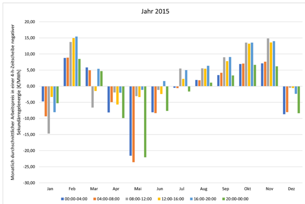
Abbildung 221: Monatlich durchschnittlicher Arbeitspreis in einer 4h-Zeitscheibe negativer Sekundärregelleistung 2015.
