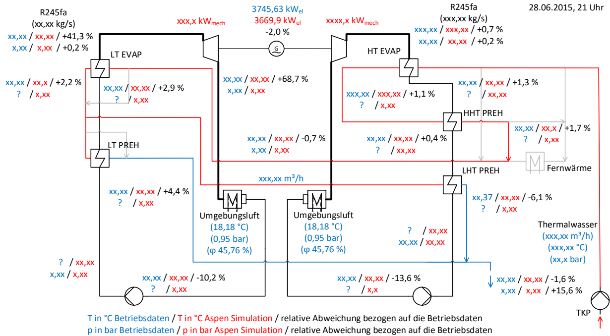
Abbildung 57: Validierung des Simulationsmodells des ORC-Referenz-Geothermie-Kraftwerks im Juni.
