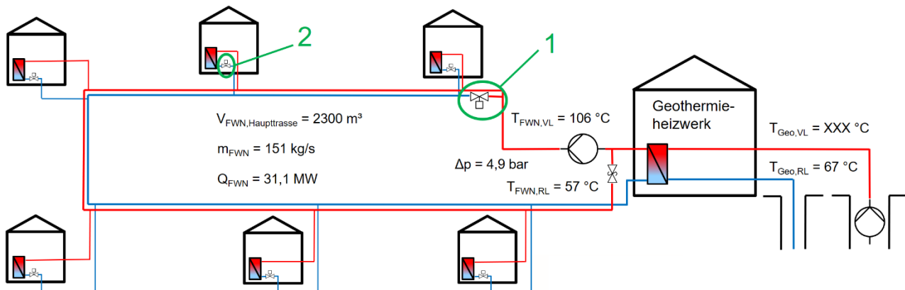
Abbildung 31: Schematischer Aufbau eines Zweileiter-Fernwärmenetzes mit Ringnetztopologie und Geothermieheizwerk (Markierung 1: Ventil, welches die Haupttrassen des Vorlaufs und Rücklaufs kurzschließt. Markierung 2: fernwärmenetzseitiges Regelventil einer Wärmeübergabestation).
