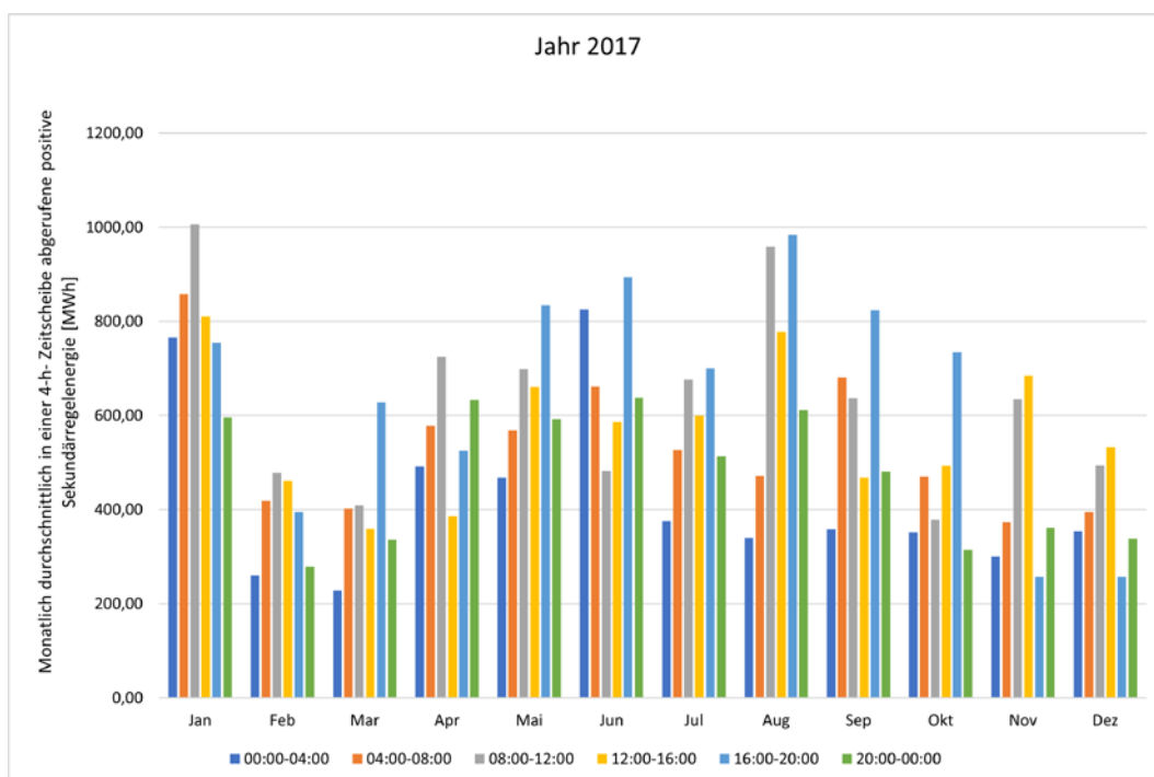
Abbildung 214: Monatlich durchschnittlich in einer 4h-Zeitscheibe abgerufene positive Sekundärregelleistung 2017.
