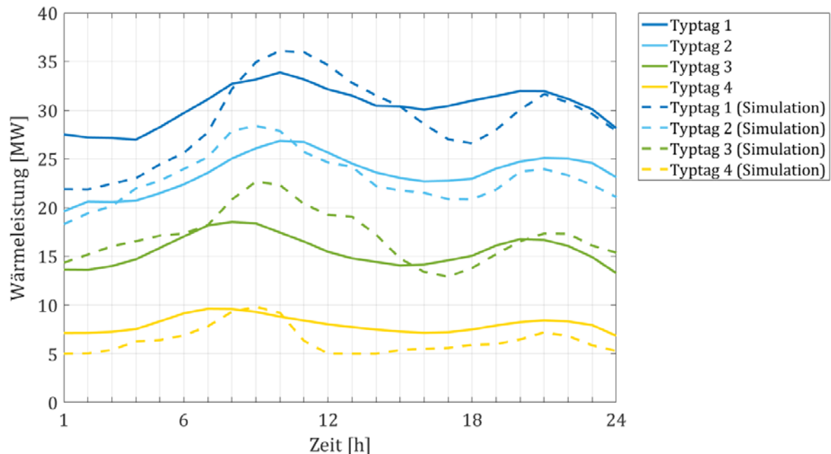
Abbildung 49: Reale Wärmeproduktionsdaten vs Simulationsergebnisse mit UrbanHeatPro: Typtage.
