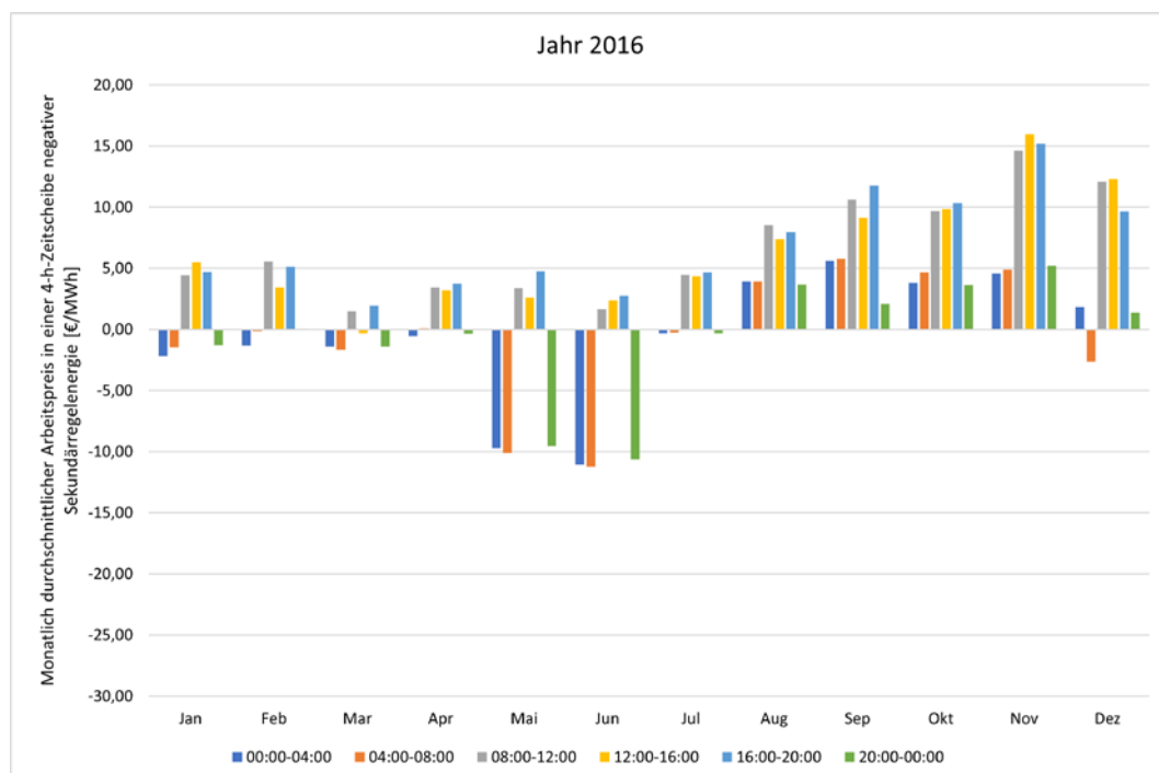
Abbildung 222: Monatlich durchschnittlicher Arbeitspreis in einer 4h-Zeitscheibe negativer Sekundärregelleistung 2016.
