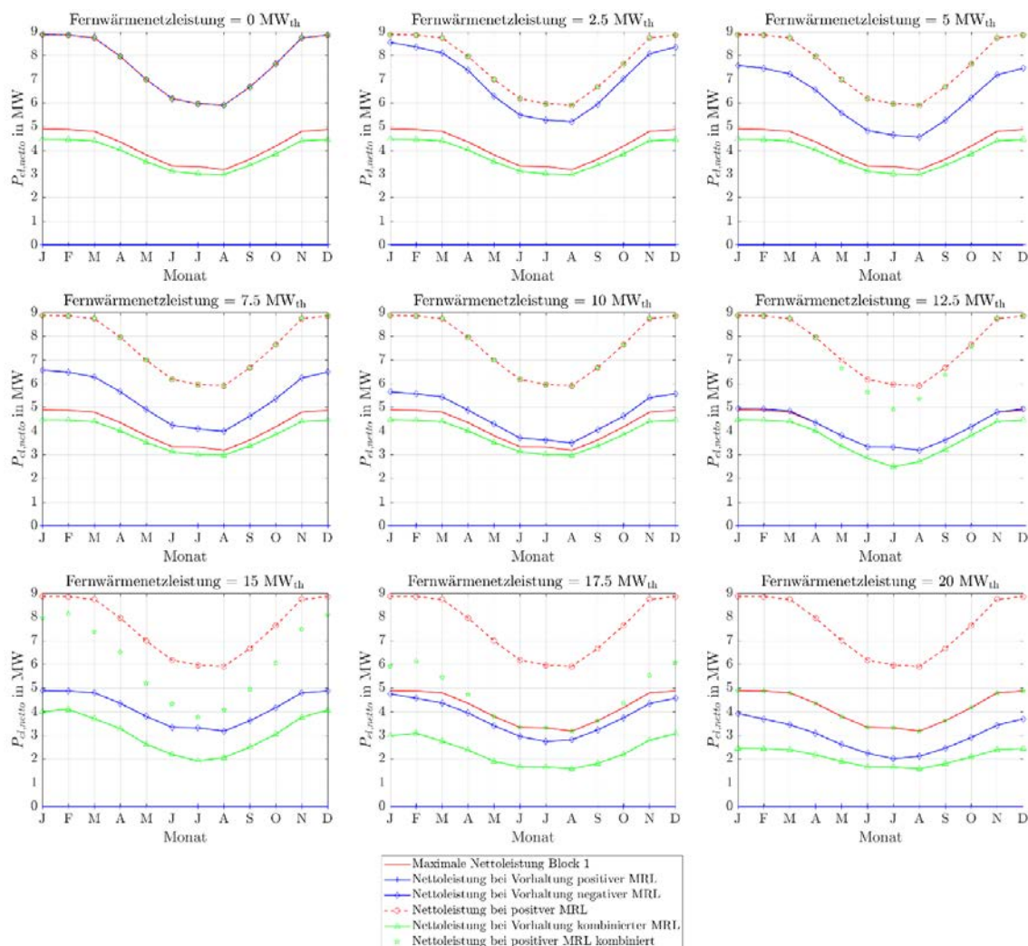
Abbildung 314: Stationäre Minutenregelleistungen des ORC-Referenz-Geothermie-Kraftwerks mit Einsatz eines Thermalwasserspeichers für Fernwärmenetzleistungen von 0 MW th bis 20 MW th bei zwei 4h-Zeitscheiben Einspeicherung und zwei aufeinanderfolgenden Zeitscheiben Angebotszeitraum.
