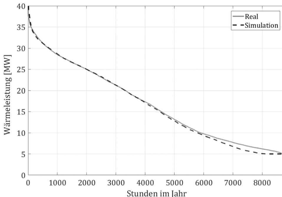
Abbildung 48: Reale Wärmeproduktionsdaten vs Simulationsergebnisse mit UrbanHeatPro: Jahresdauerlinie.
