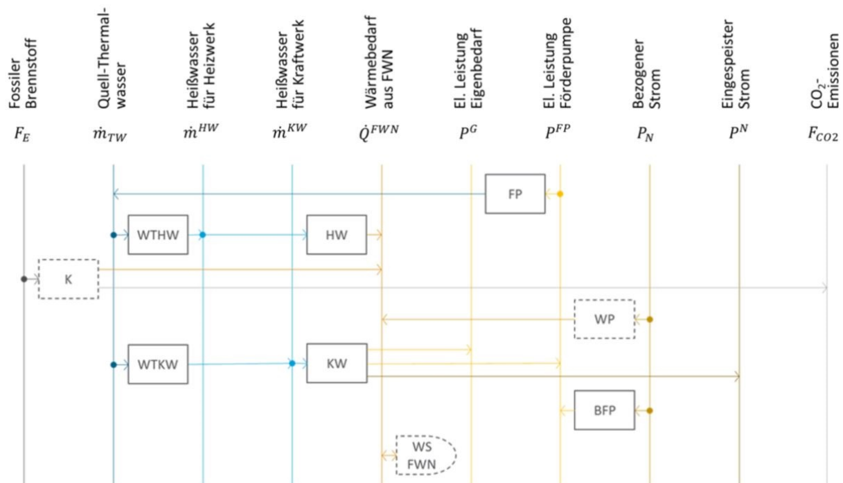
Abbildung 154: Auslegung der flexiblen Systemkonfiguration mit Geothermieranlage, Kessel, Wärmepumpe und Heißwasser-Wärmespeicher im Fernwärmenetz.
