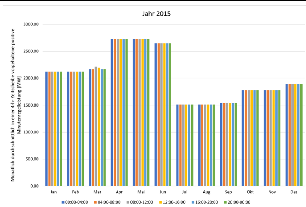
Abbildung 232: Monatlich durchschnittlich in einer 4h-Zeitscheibe vorgehaltene positive Minutenregelleistung 2015.
