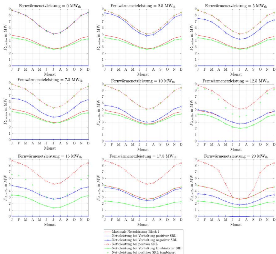
Abbildung 266: Stationäre Sekundärregelleistungen des ORC-Referenz-Geothermie-Kraftwerks mit Einsatz eines Heißwasser-Wärmespeichers des Heiz- und Kraftwerks für Fernwärmenetzleistungen von 0 MW th bis 20 MW th bei einer 4h-Zeitscheibe Einspeicherung und einer Zeitscheibe Angebotszeitraum.
