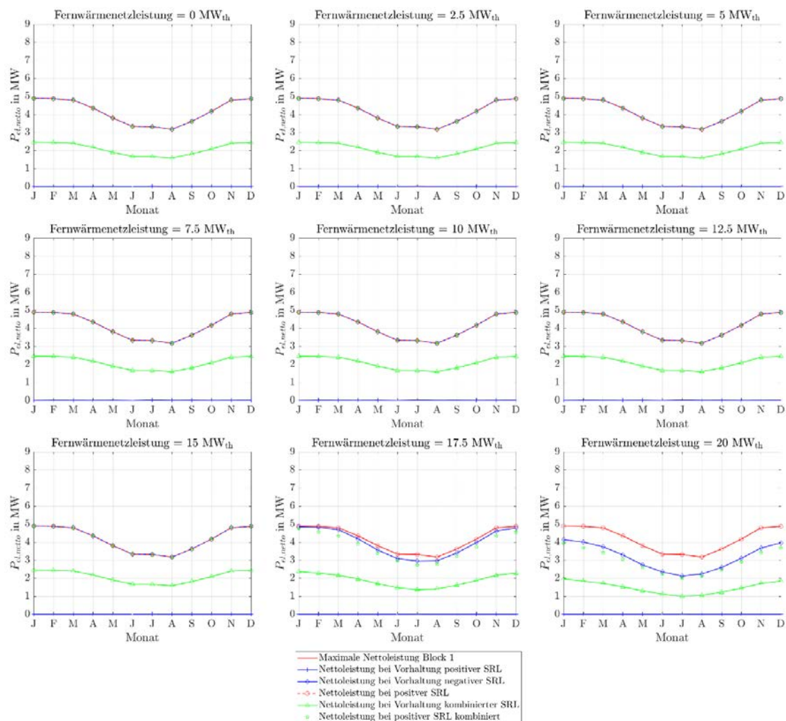
Abbildung 119: Stationäre Sekundärregelleistungen des ORC-Referenz-Geothermie-Kraftwerks mit Einsatz eines Heißwasser-Wärmespeichers im Fernwärmenetz für Fernwärmenetzleistungen von 0 MW th bis 20 MW th bei drei 4h-Zeitscheiben Einspeicherung und drei aufeinanderfolgenden Zeitscheiben Angebotszeitraum.
