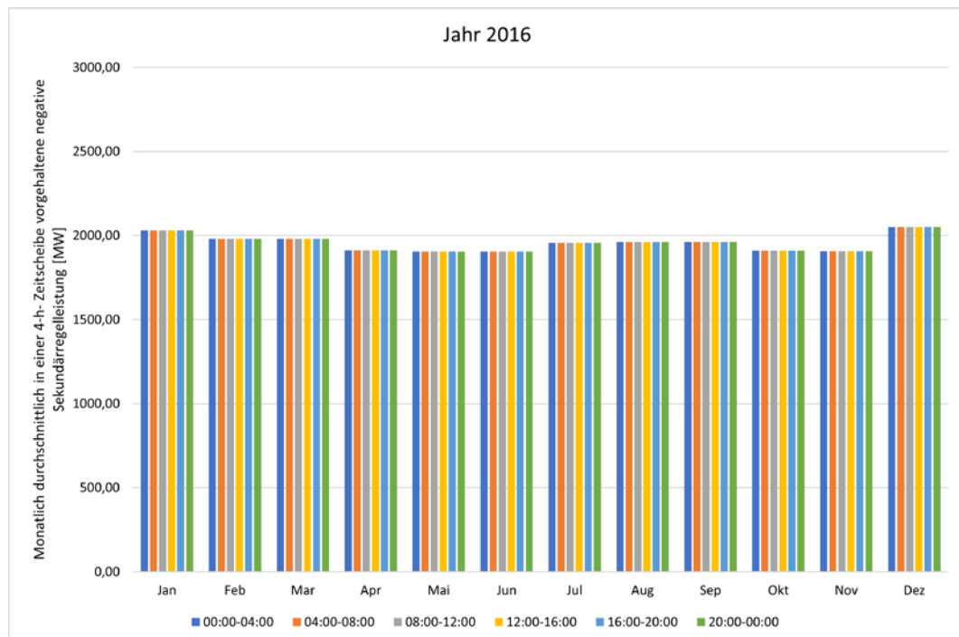
Abbildung 204: Monatlich durchschnittlich in einer 4h-Zeitscheibe vorgehaltene negative Sekundärregelleistung 2016.
