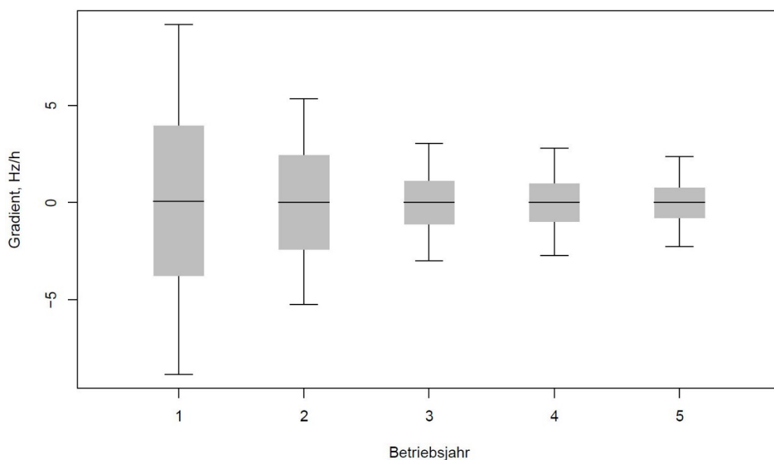
Abbildung 25: Gradienten der Pumpenfrequenz einer Tauchkreislumpumpe eines Geothermiekraftwerks im Bayerischen Molassebecken seit Inbetriebnahme. Dargestellt sind die Quartile (graue Box) und die 10 % und 90 %-Quantile (Antennen).
