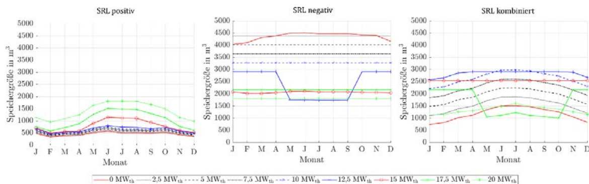
Abbildung 122: Benötigte Speichergrößen bei Angebot von positiver, negativer und kombinierter SRL des ORC-Referenz-Geothermie-Kraftwerks mit Einsatz eines Thermalwasserspeichers im Kraftwerk für Fernwärmenetzleistungen von 0 MW th bis 20 MW th bei drei 4h-Zeitscheiben Einspeicherung und drei aufeinanderfolgenden Zeitscheiben Angebotszeitraum.
