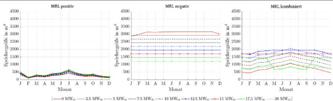
Abbildung 315: Benötigte Speichergrößen bei Angebot von positiver, negativer und kombinierter MRL des ORC-Referenz-Geothermie-Kraftwerks mit Einsatz eines Thermalwasserspeichers im Kraftwerk für Fernwärmenetzleistungen von 0 MW th bis 20 MW th bei zwei 4h-Zeitscheiben Einspeicherung und zwei aufeinanderfolgenden Zeitscheiben Angebotszeitraum.
