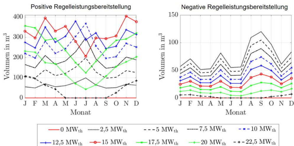
Abbildung 78: Benötigte Speichervolumina für die stationären Sekundärregelleistungen des ORC-Referenz-Geothermie-Kraftwerks mit Einsatz eines Fernwärmenetzspeichers für Fernwärmenetzleistungen von 0 MW th bis 22,5 MW th .
