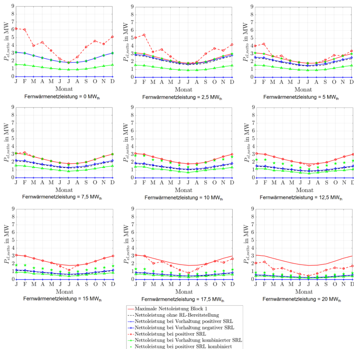
Abbildung 196: Stationäre Sekundärregelleistungen des Kalina-Referenz-Geothermie-Kraftwerks mit Einsatz eines Heißwasser-Wärmespeichers für Heiz- und Kraftwerk für Fernwärmenetzleistungen von 0 MW th bis 20 MW th .
