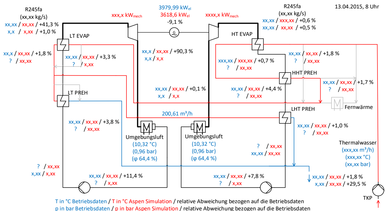
Abbildung 179: Validierung des Simulationsmodells des ORC-Referenz-Geothermie-Kraftwerks im April.
