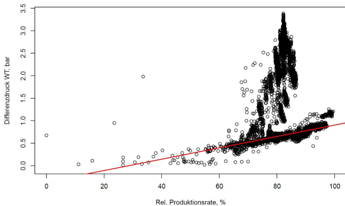
Abbildung 15: Differenzdruck am Wärmetauscher als Funktion des Volumenstromes.
