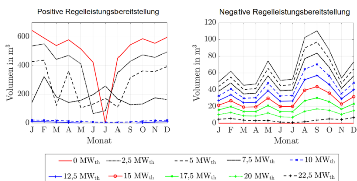
Abbildung 191: Benötigte Speichervolumina für die stationären Sekundärregelleistungen des Kalina-Referenz-Geothermie-Kraftwerks mit Einsatz eines Thermalwasserspeichers für Fernwärmenetzleistungen von 0 MW th bis 22,5 MW th .
