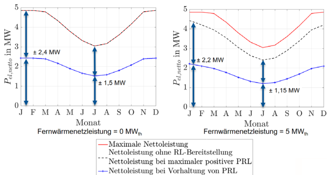
Abbildung 71: Stationäre Primärregelleistungen des ORC-Referenz-Geothermie-Kraftwerks im Bestand ohne Flexibilisierungsmaßnahmen für die Fernwärmenetzleistungen 0 MW th und 5 MW th .
