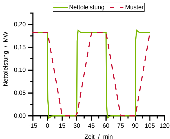
Abbildung 66: Lastprofil der dynamischen Simulation im Vergleich zum Verlauf des Musterprotokolls für die Tertiärregelleistung bei Vorhaltung negativer Regelleistung (Betrachtungsmonat Mai; Fernwärmeleistung 20 MW).
