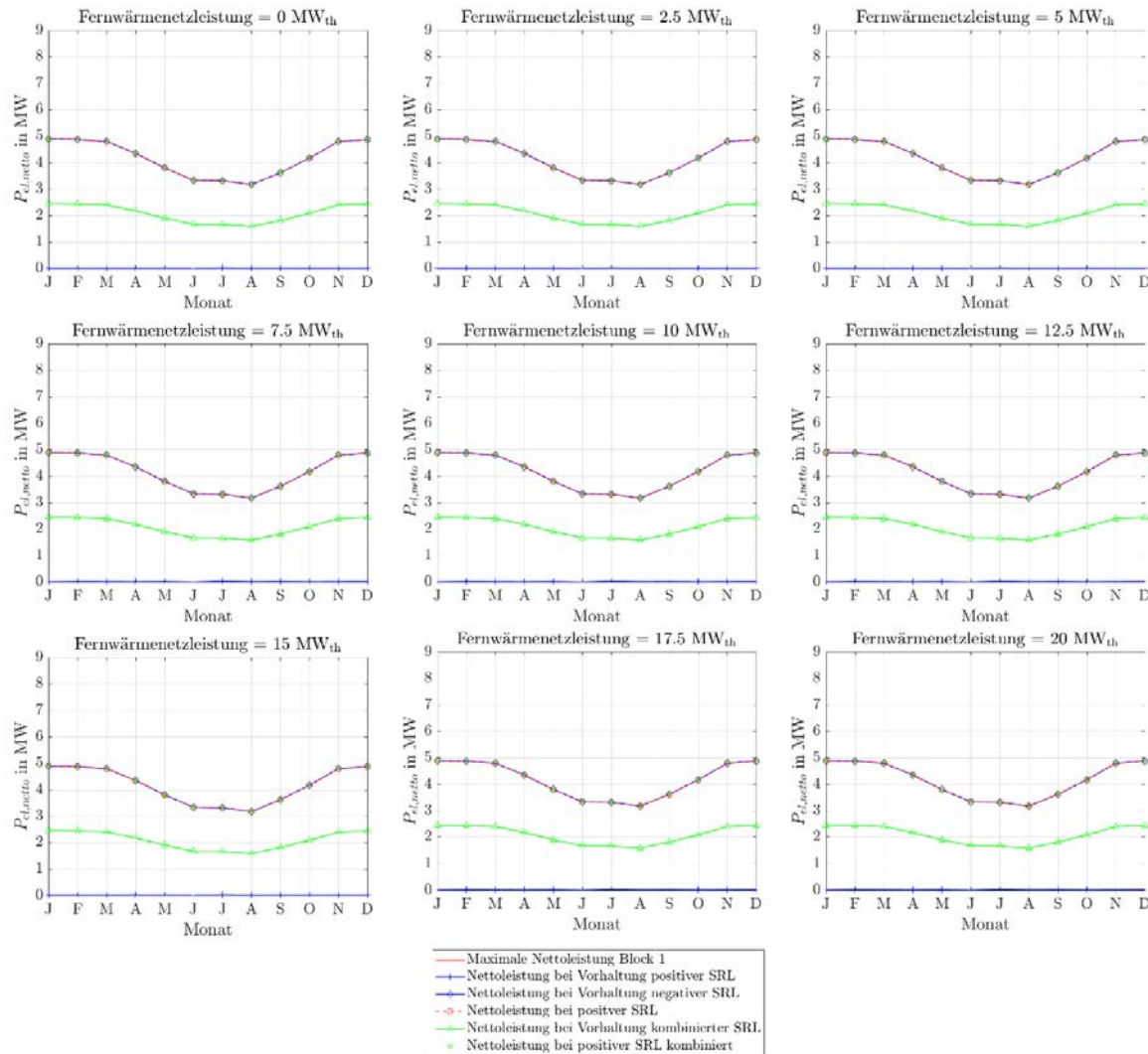
Abbildung 107: Stationäre Sekundärregelleistungen des ORC-Referenz-Geothermie-Kraftwerks mit Einsatz eines Heißwasser-Wärmespeichers im Fernwärmenetz für Fernwärmenetzleistungen von 0 \text{ MW}_{\text{th}} bis 20 \text{ MW}_{\text{th}} bei zwei 4h-Zeitscheiben Einspeicherung und einer Zeitscheibe Angebotszeitraum.
