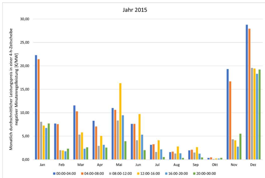
Abbildung 241: Monatlich durchschnittlicher Leistungspreis in einer 4h-Zeitscheibe negativer Minutenregelleistung 2015.
