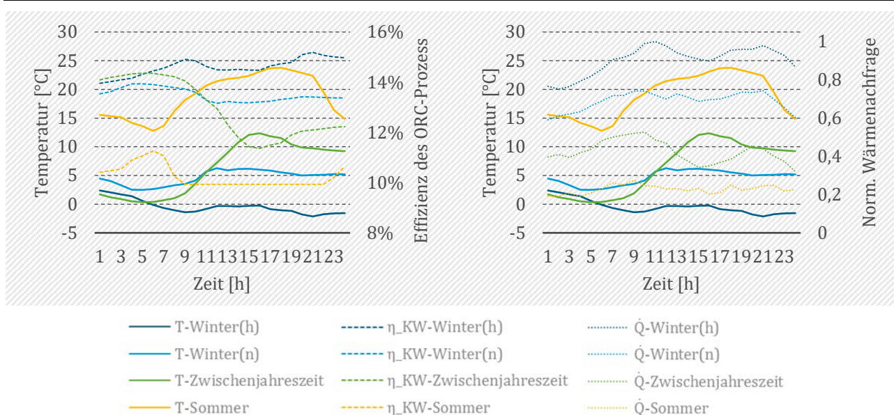
Abbildung 163: Umgebungstemperatur und der elektrische Wirkungsgrad des Referenz-ORC-Prozesses (links) sowie der Umgebungstemperatur und normierte Wärmebedarf am Fernwärmeanschluss (rechts).
