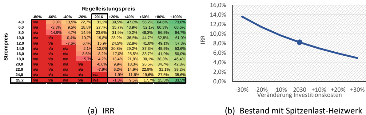
Abbildung 143: IRR für Investition in Heißwasser-Wärmespeicher (a) und Sensitivität des IRRs (b) bei fester Einspeisevergütung und Fernwärmenetz-Anschlussleistung 67,5 MW.
