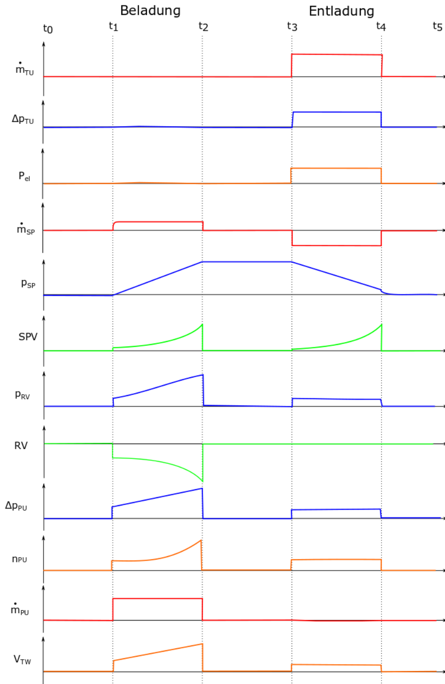
Abbildung 100: Verlauf der wichtigsten Prozess- und Stellgrößen des Kraftwerksprozesses mit dem Betrieb eines absperribaren Dampfspeichers [98, S. 37].
