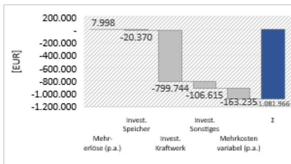
(d) Thermalwasser-Wärmespeicher
