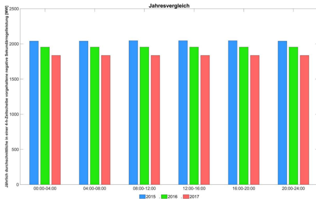
Abbildung 225: Jährlich durchschnittlicher in einer 4h-Zeitscheibe vorgehaltene negative Sekundärregelleistung.
