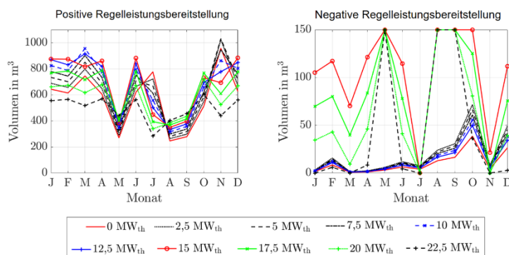
Abbildung 199: Benötigte Speichervolumina für die stationären Minutenregelleistungen des Kalina-Referenz-Geothermie-Kraftwerks mit Einsatz eines Heißwasser-Wärmespeichers für Fernwärmenetzleistungen von 0 MW th bis 22,5 MW th .
