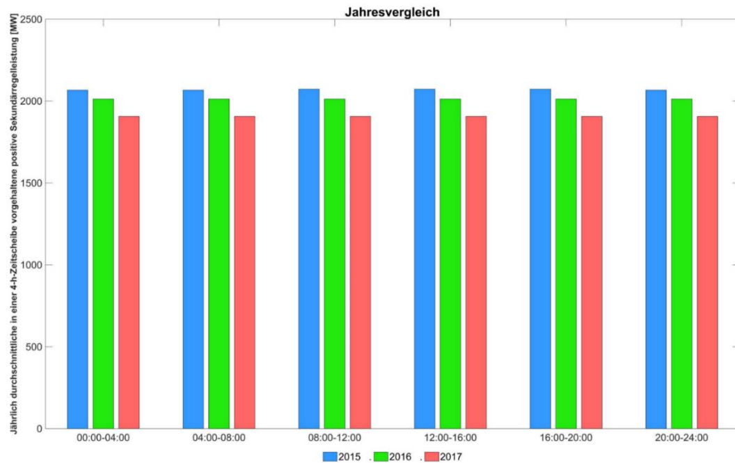
Abbildung 224: Jährlich durchschnittlicher in einer 4h-Zeitscheibe vorgehaltene positive Sekundärregelleistung.
