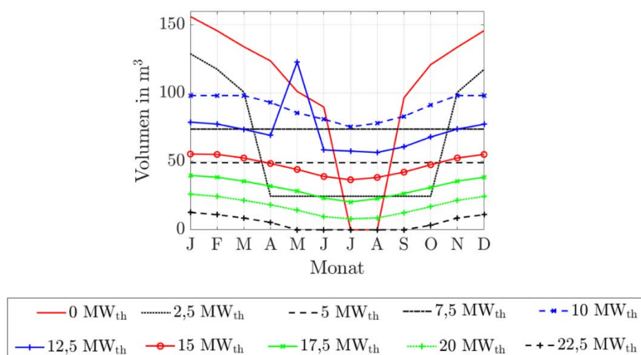
Abbildung 84: Benötigte Speichervolumina für die stationären Primärregelleistungen des ORC-Referenz-Geothermie-Kraftwerks mit Einsatz eines Thermalwasserspeichers für Fernwärmenetzleistungen von 0 MW th bis 22,5 MW th .
