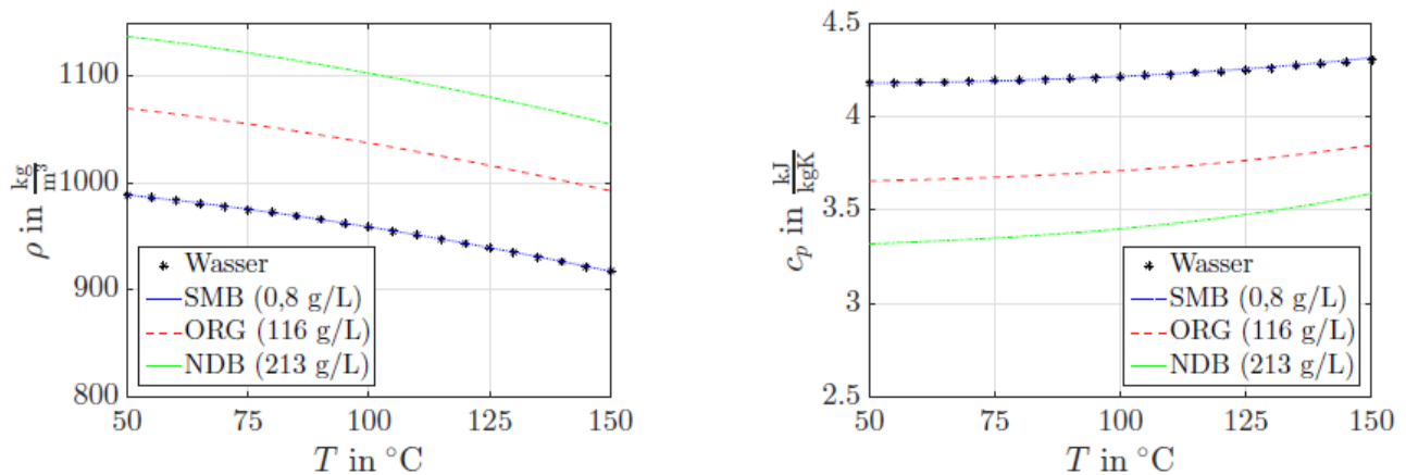
Abbildung 176: Einfluss der Thermalwassermineralisation auf die Stoffwerte Dichte (rechts) und spezifische Wärmekapazität (links) bei einem Druck von 1 bar
