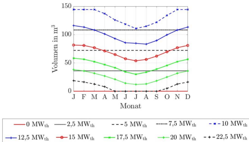
Abbildung 76: Benötigte Speichervolumina für die stationären Primärregelleistungen des ORC-Referenz-Geothermie-Kraftwerks mit Einsatz eines Fernwärmenetzspeichers für Fernwärmenetzleistungen von 0 MW th bis 22,5 MW th .
