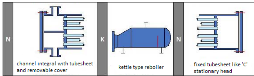
Abbildung 52: Aufbau des HT- und LT-Verdampfers nach TEMA-Standard [vgl. 81].
