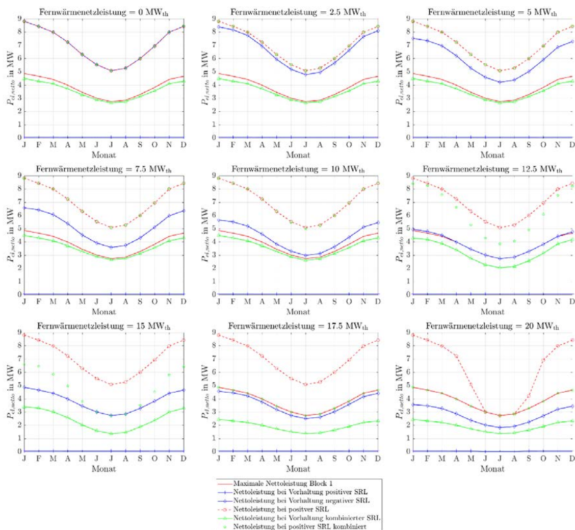
Abbildung 123: Stationäre Sekundärregelleistungen des ORC-Referenz-Geothermie-Kraftwerks mit Einsatz eines Heißwasser-Wärmespeichers des Heiz- und Kraftwerks für Fernwärmenetzleistungen von 0 MW th bis 20 MW th bei drei 4h-Zeitscheiben Einspeicherung und drei aufeinanderfolgenden Zeitscheiben Angebotszeitraum.
