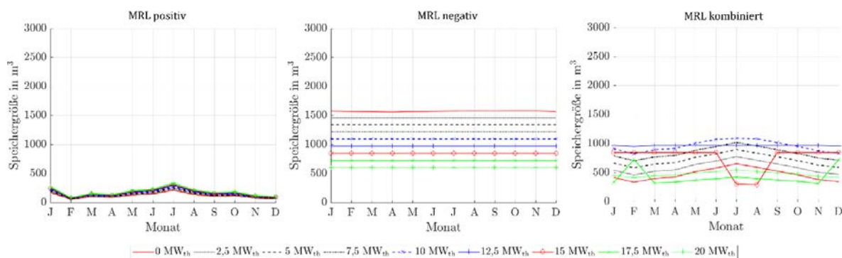
Abbildung 277: Benötigte Speichergrößen bei Angebot von positiver, negativer und kombinierter MRL des ORC-Referenz-Geothermie-Kraftwerks mit Einsatz eines Heißwasser-Wärmespeichers des Heiz- und Kraftwerks für Fernwärmenetzleistungen von 0 MW th bis 20 MW th bei einer 4h-Zeitscheibe Einspeicherung und einer Zeitscheibe Angebotszeitraum.
