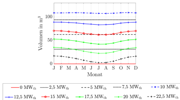
Abbildung 189: Benötigte Speichervolumina für die stationären Primärregelleistungen des Kalina-Referenz-Geothermie-Kraftwerks mit Einsatz eines Thermalwasserspeichers für Fernwärmenetzleistungen von 0 MW th bis 22,5 MW th .
