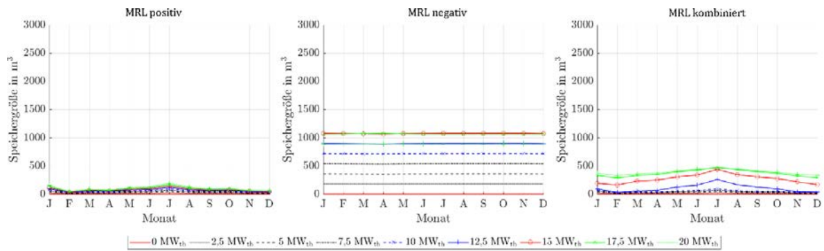
Abbildung 273: Benötigte Speichergrößen bei Angebot von positiver, negativer und kombinierter MRL des ORC-Referenz-Geothermie-Kraftwerks mit Einsatz eines Heißwasser-Wärmespeichers im Fernwärmenetz für Fernwärmenetzleistungen von 0 MW th bis 20 MW th bei und einer 4h-Zeitscheibe Einspeicherung einer Zeitscheibe Angebotszeitraum.
