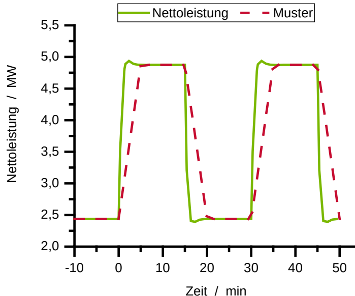
Abbildung 67: Lastprofil der dynamischen Simulation im Vergleich zum Verlauf des Musterprotokolls für die Sekundärregelleistung bei Vorhaltung symmetrisch positiver Regelleistung (Betrachtungsmonat Februar; Fernwärmeleistung 0 MW).
