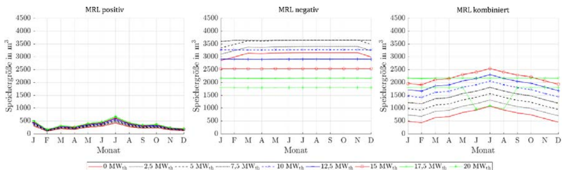
Abbildung 321: Benötigte Speichergrößen bei Angebot von positiver, negativer und kombinierter MRL des ORC-Referenz-Geothermie-Kraftwerks mit Einsatz eines Thermalwasserspeichers im Kraftwerk für Fernwärmenetzleistungen von 0 MW th bis 20 MW th bei drei 4h-Zeitscheiben Einspeicherung und zwei aufeinanderfolgenden Zeitscheiben Angebotszeitraum.
