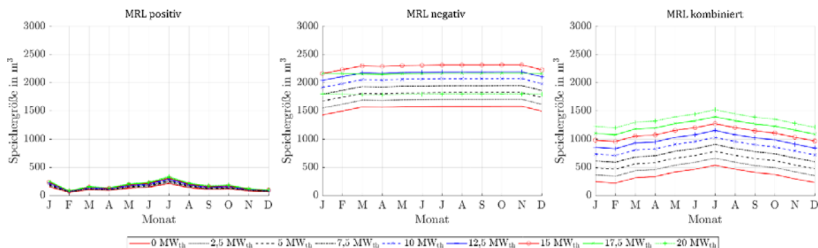
Abbildung 285: Benötigte Speichergrößen bei Angebot von positiver, negativer und kombinierter MRL des ORC-Referenz-Geothermie-Kraftwerks mit Einsatz eines Thermalwasserspeichers im Kraftwerk für Fernwärmenetzleistungen von 0 MW th bis 20 MW th bei drei 4h-Zeitscheiben Einspeicherung und einer Zeitscheibe Angebotszeitraum.
