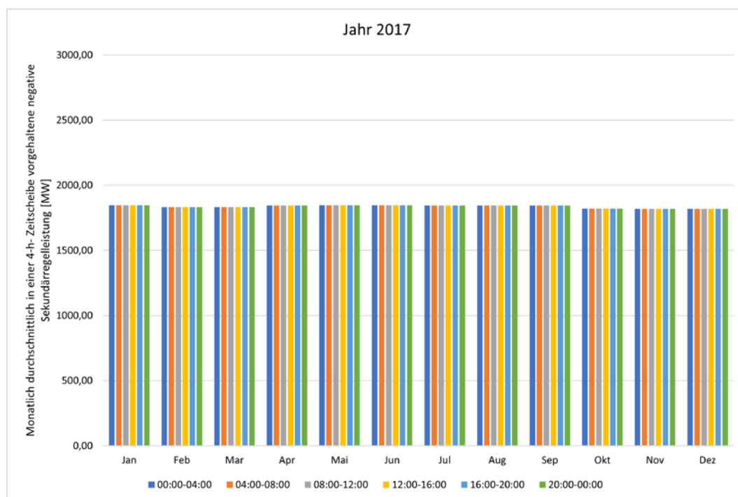
Abbildung 205: Monatlich durchschnittlich in einer 4h-Zeitscheibe vorgehaltene negative Sekundärregelleistung 2017.
