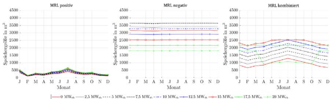
Abbildung 323: Benötigte Speichergrößen bei Angebot von positiver, negativer und kombinierter MRL des ORC-Referenz-Geothermie-Kraftwerks mit Einsatz eines Heißwasser-Wärmespeichers des Heiz- und Kraftwerks für Fernwärmenetzleistungen von 0 MW th bis 20 MW th bei drei 4h-Zeitscheiben Einspeicherung und zwei aufeinanderfolgenden Zeitscheiben Angebotszeitraum.
