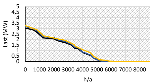
Abbildung 133: Jahresdauerlinie der ORC-Referenzanlage bei Erbringung positiver und negativer Sekundärregelleistung mit Fernwärmenetzanschlussleistung 67,5 MW und 0 MW.
