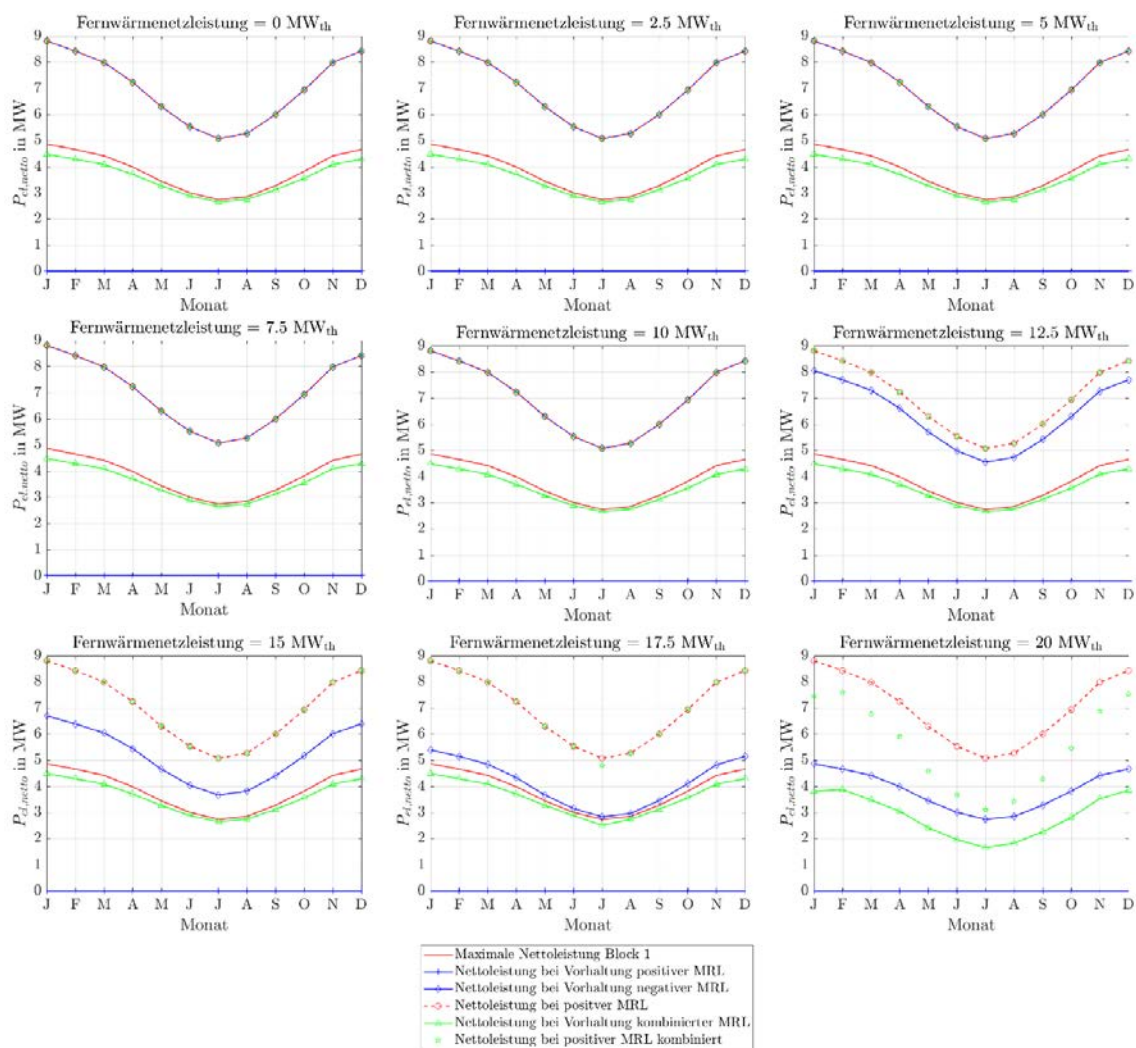
Abbildung 328: Stationäre Minutenregelleistungen des ORC-Referenz-Geothermie-Kraftwerks mit Einsatz eines Heißwasser-Wärmespeichers des Heiz- und Kraftwerks für Fernwärmenetzleistungen von 0 MW th bis 20 MW th bei vier 4h-Zeitscheiben Einspeicherung und zwei aufeinanderfolgenden Zeitscheiben Angebotszeitraum.
