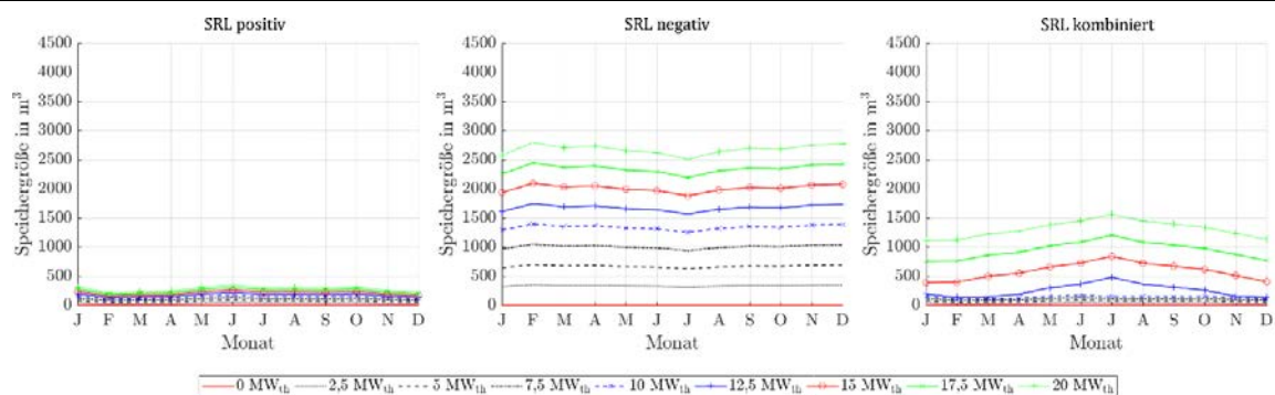
Abbildung 301: Benötigte Speichergrößen bei Angebot von positiver, negativer und kombinierter SRL des ORC-Referenz-Geothermie-Kraftwerks mit Einsatz eines Heißwasser-Wärmespeichers im Fernwärmenetz für Fernwärmenetzleistungen von 0 MW th bis 20 MW th bei vier 4h-Zeitscheiben Einspeicherung und zwei aufeinanderfolgenden Zeitscheiben Angebotszeitraum.
