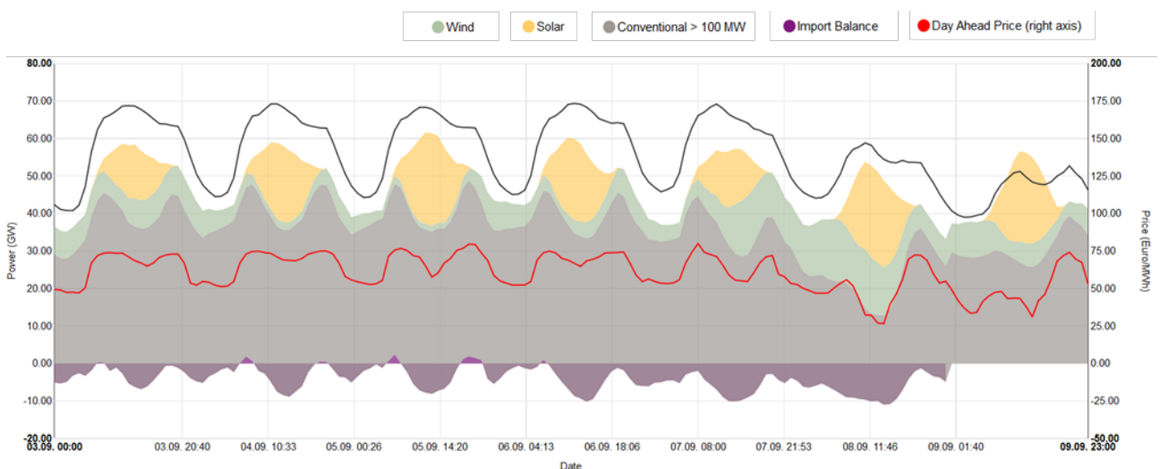
Abbildung 165: Stromproduktion und -preise in Deutschland für die Kalenderwoche 43, 2018 [122].
