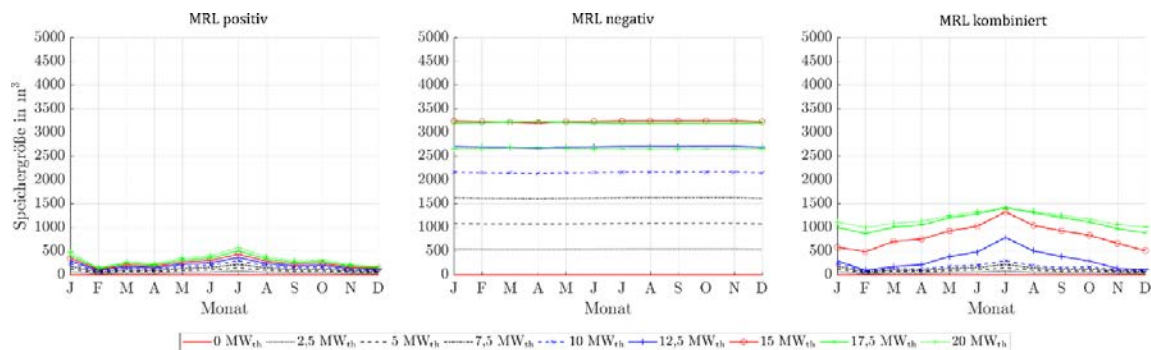
Abbildung 331: Benötigte Speichergrößen bei Angebot von positiver, negativer und kombinierter MRL des ORC-Referenz-Geothermie-Kraftwerks mit Einsatz eines Heißwasser-Wärmespeichers im Fernwärmenetz für Fernwärmenetzleistungen von 0 MW th bis 20 MW th bei drei 4h-Zeitscheiben Einspeicherung und drei aufeinanderfolgenden Zeitscheiben Angebotszeitraum.
