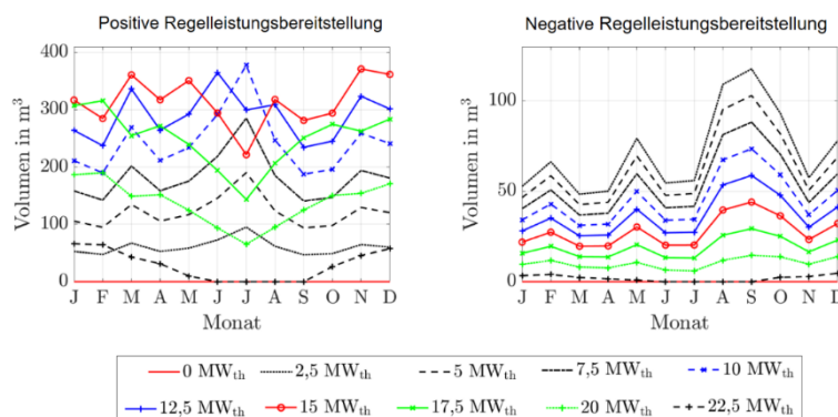
Abbildung 185: Benötigte Speichervolumina für die stationären Sekundärregelleistungen des Kalina-Referenz-Geothermie-Kraftwerks mit Einsatz eines Fernwärmenetzspeichers für Fernwärmenetzleistungen von 0 MW th bis 22,5 MW th .
