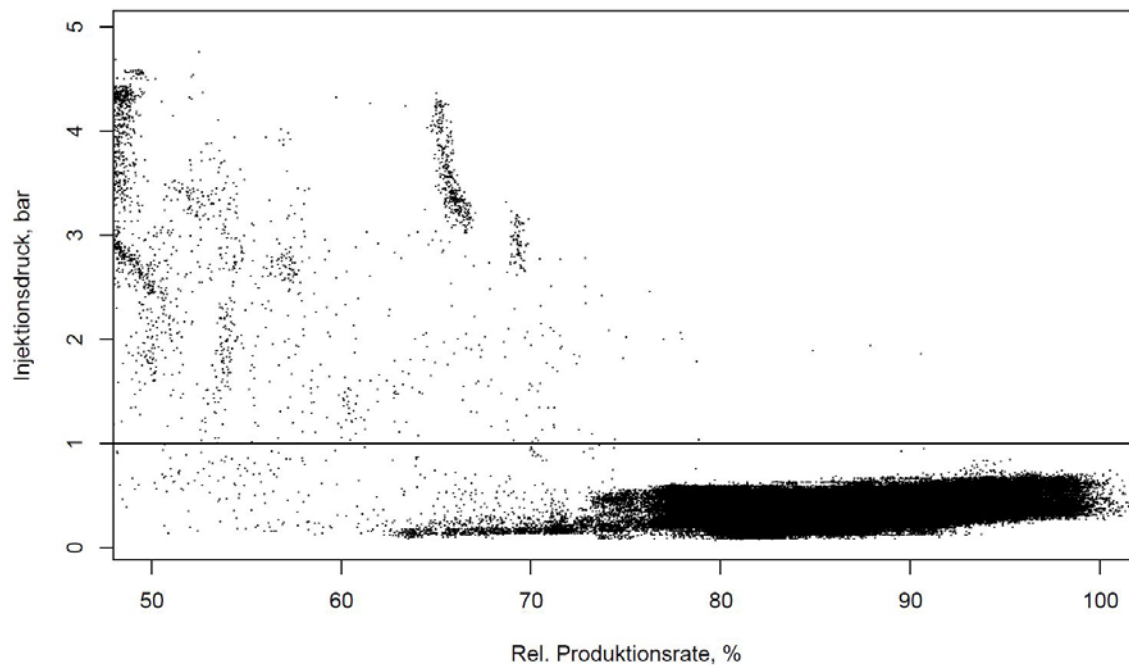
Abbildung 20: Injektionsdruck als Funktion der relativen Produktionsrate für ein Geothermiekraftwerk im Bayerischen Molassebecken.
