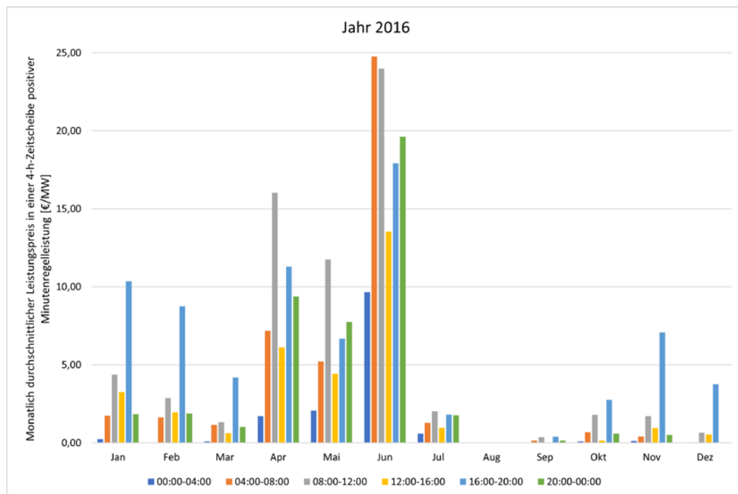
Abbildung 239: Monatlich durchschnittlicher Leistungspreis in einer 4h-Zeitscheibe positiver Minutenregelleistung 2016.
