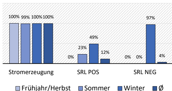
(c) Heißwasser-Wärmespeicher
