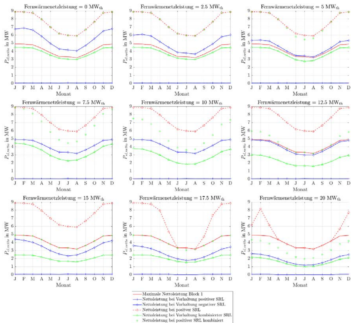
Abbildung 115: Stationäre Sekundärregelleistungen des ORC-Referenz-Geothermie-Kraftwerks mit Einsatz eines Thermalwasserspeichers für Fernwärmenetzleistungen von 0 MW th bis 20 MW th bei einer 4h-Zeitscheibe Einspeicherung und zwei aufeinanderfolgenden Zeitscheiben Angebotszeitraum.
