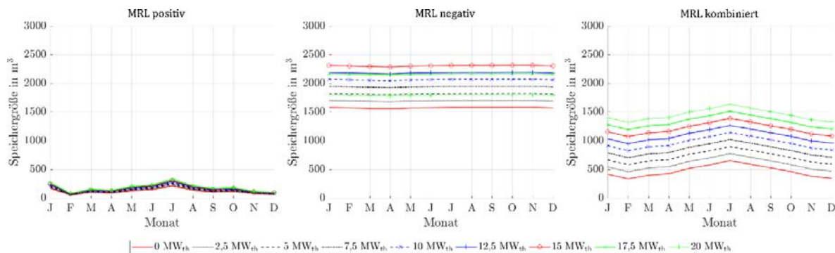
Abbildung 287: Benötigte Speichergrößen bei Angebot von positiver, negativer und kombinierter MRL des ORC-Referenz-Geothermie-Kraftwerks mit Einsatz eines Heißwasser-Wärmespeichers des Heiz- und Kraftwerks für Fernwärmenetzleistungen von 0 MW th bis 20 MW th bei drei 4h-Zeitscheiben Einspeicherung und einer Zeitscheibe Angebotszeitraum.
