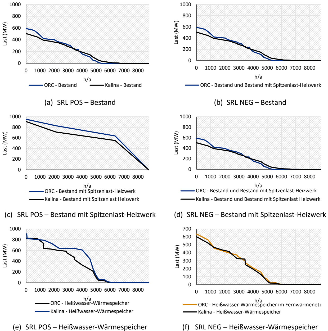
Abbildung 145: Vergleich der Jahresdauerlinie für die Regelleistungsbereitstellung des ORC-Zweidruck-Prozess und Kalina-Prozess bei Fernwärmenetz-Anschlussleistung von 67,5 MW.
