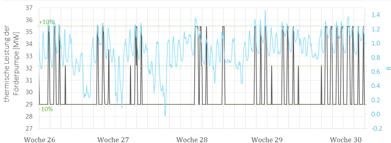
Abbildung 170: Thermische Leistung der Förderpumpe und Strompreis in Brennstoffpreis Einheiten (R) für Anlagekonfiguration AK-8 für fünf Wochen in Sommer.
