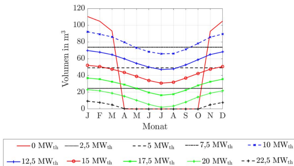
Abbildung 92: Benötigte Speichervolumina für die stationären Primärregelleistungen des ORC-Referenz-Geothermie-Kraftwerks mit Einsatz eines Heißwasser-Wärmespeichers für Fernwärmenetzleistungen von 0 MW th bis 22,5 MW th .
