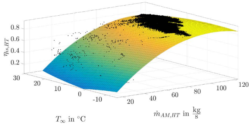
Abbildung 56: Kennfeld des isentropen Wirkungsgrads der HT-Turbine in Abhängigkeit des Arbeitsmittel-Massenstroms und der Umgebungstemperatur mit schwarzen Stützpunkten für die Korrelationsberechnung.
