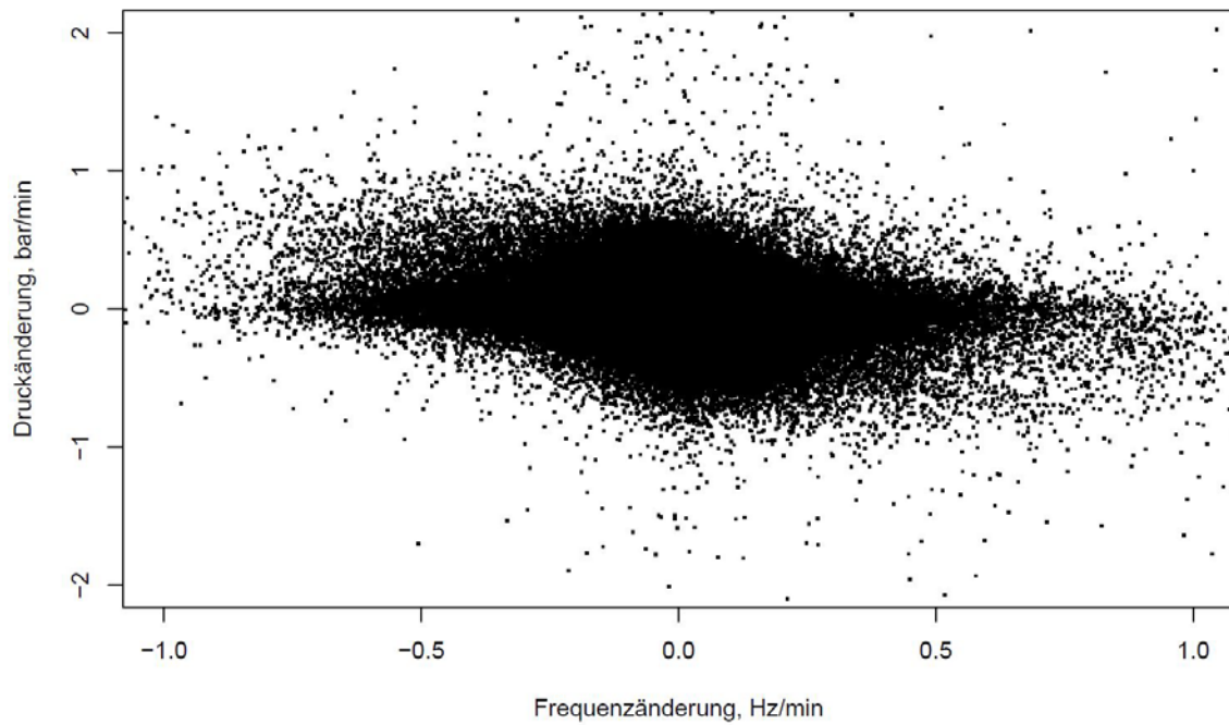
Abbildung 19: Druckänderung als Funktion der Frequenzänderung der Tauchkreislpumpe an einem Geothermiekraftwerk im Molassebecken.
