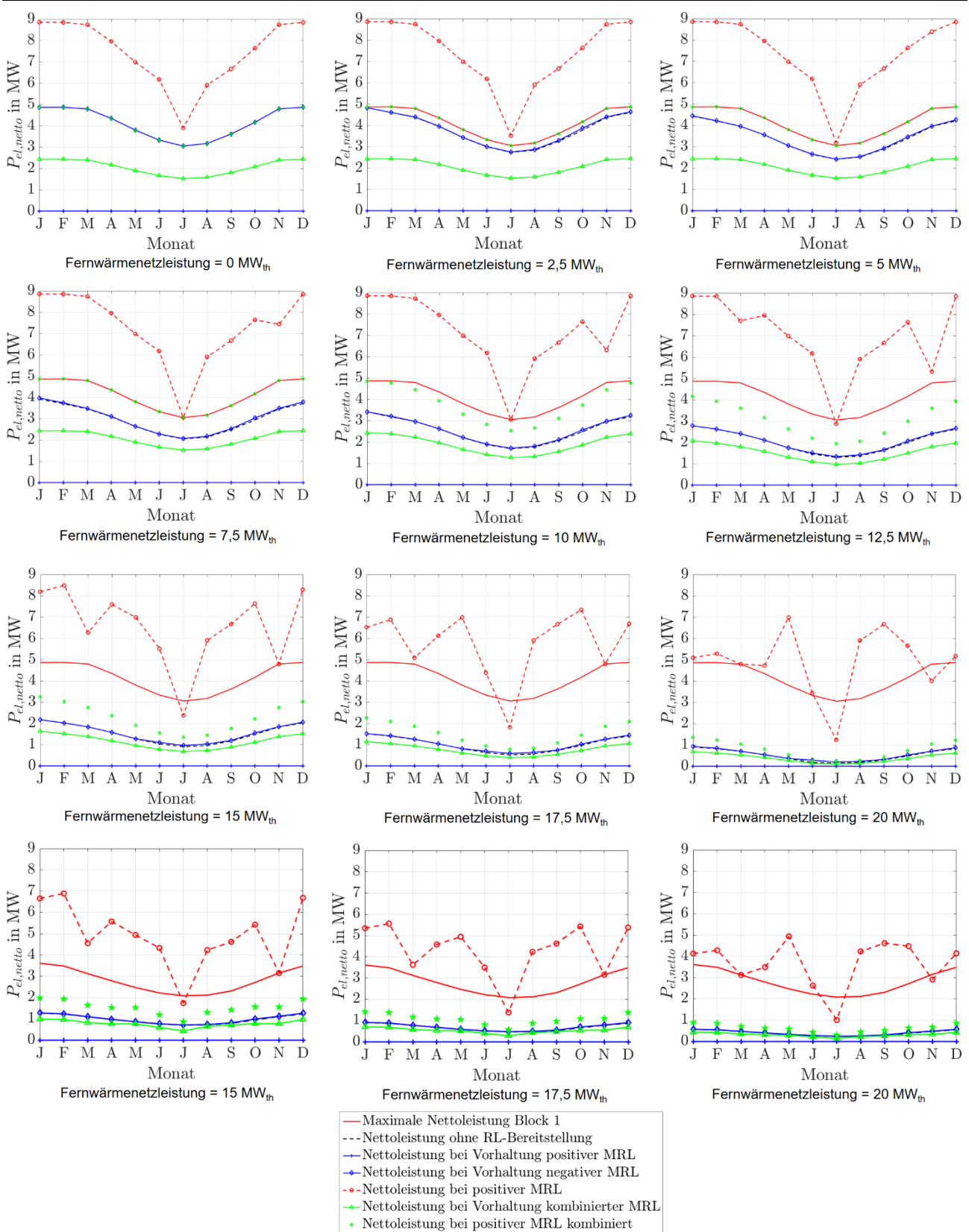
Abbildung 87: Stationäre Minutenregelleistungen des ORC-Referenz-Geothermie-Kraftwerks mit Einsatz eines Thermalwasserspeichers für Fernwärmenetzleistungen von 0 MW th bis 20 MW th .
