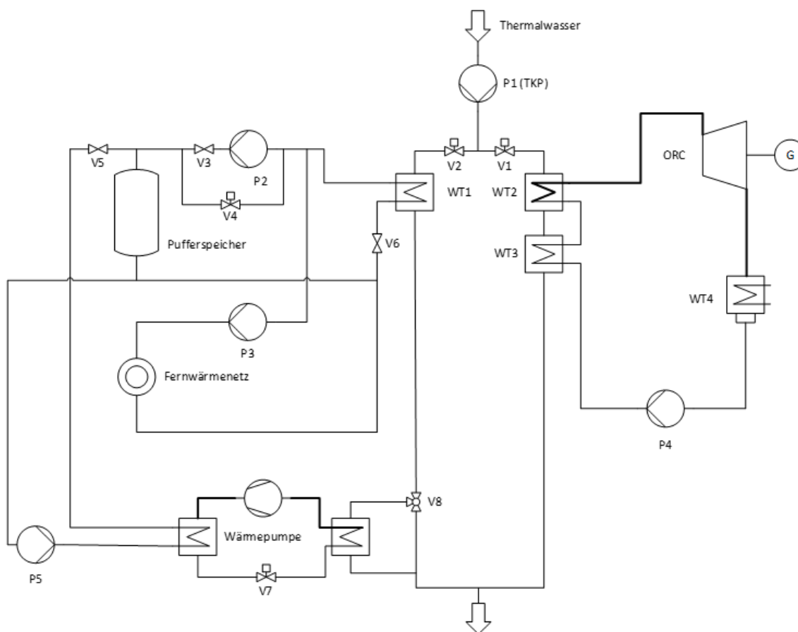
Abbildung 41: Geothermie-basiertes Strom-Wärme-System mit Integration einer Wärmepumpe und eines Heißwasser-Pufferspeichers in das Fernwärmenetz.
