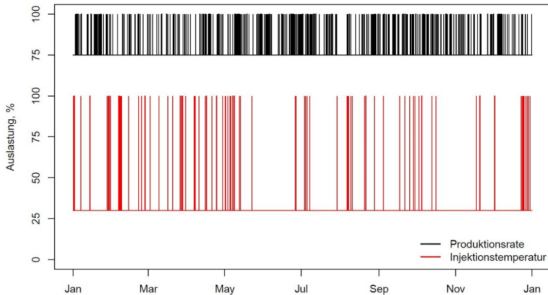
Abbildung 16: Abwicklung der Produktionsrate und der Injektionstemperatur während des hypothetischen Regelbetriebs an einem Geothermiekraftwerks im Molassebecken.
