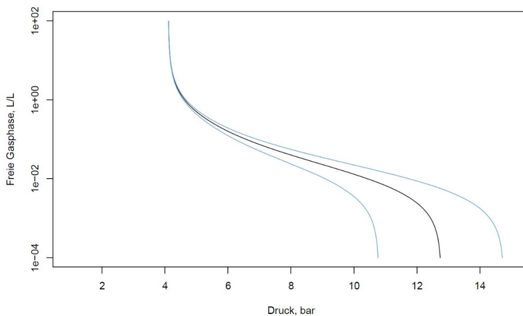
Abbildung 9: Berechnete Schwankungsbreite der Gasdrücke an einem Geothermiekraftwerk im Molassebecken für eine Thermalwassertemperatur von 145 °C. Dargestellt sind der Mittelwert und der 95 %-Vertrauensbereich.
