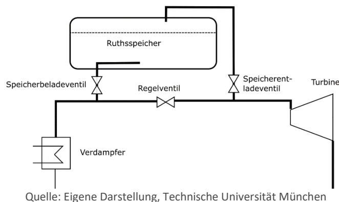
Abbildung 98: Ausschnitt aus einem Verfahrensfließbild der Integration eines Ruths-Speichers in das Kraftwerk [98, S. 29].
