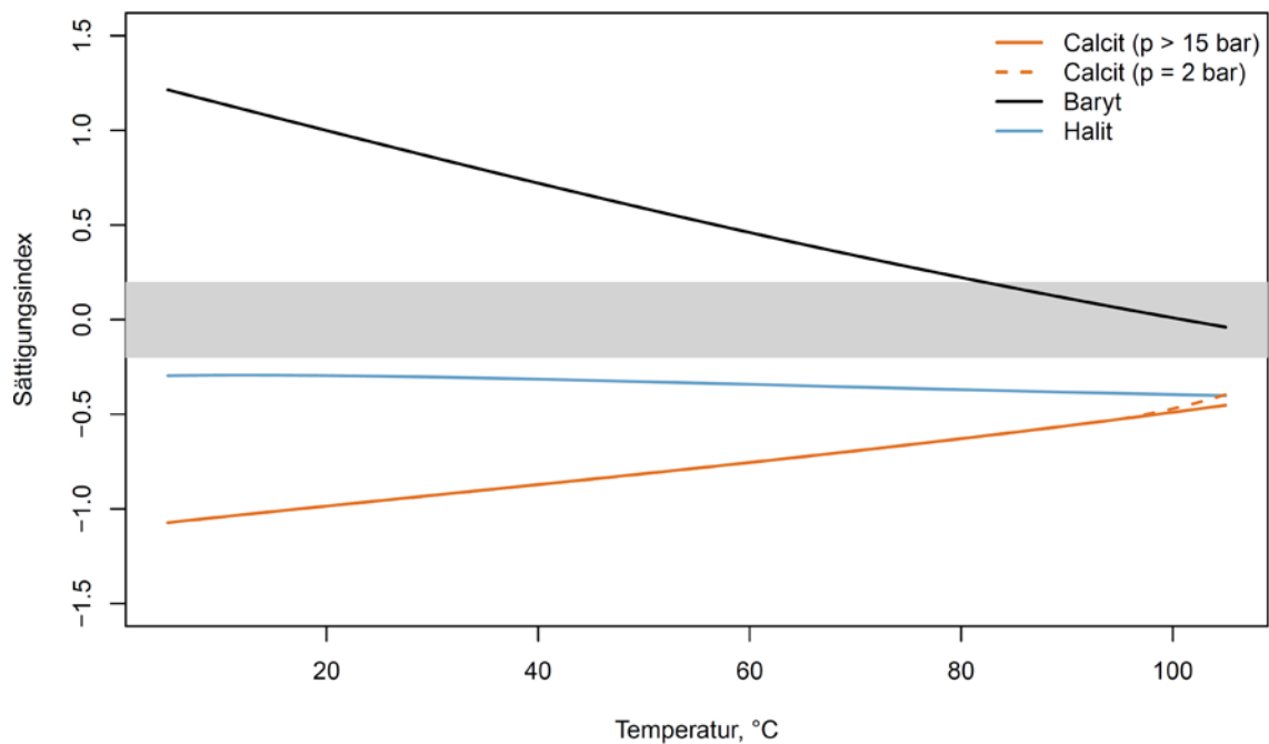
Abbildung 23: Sättigungsindex für Baryt, Halit und Calcit für eine Anlage im Norddeutschen Becken als Funktion der Temperatur.
