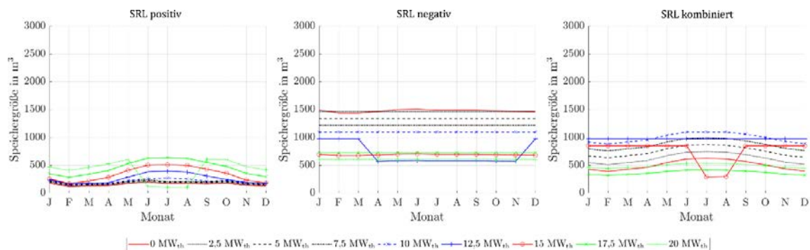
Abbildung 267: Benötigte Speichergrößen bei Angebot von positiver, negativer und kombinierter SRL des ORC-Referenz-Geothermie-Kraftwerks mit Einsatz eines Heißwasser-Wärmespeichers des Heiz- und Kraftwerks für Fernwärmenetzleistungen von 0 MW th bis 20 MW th bei einer 4h-Zeitscheibe Einspeicherung und einer Zeitscheibe Angebotszeitraum.
