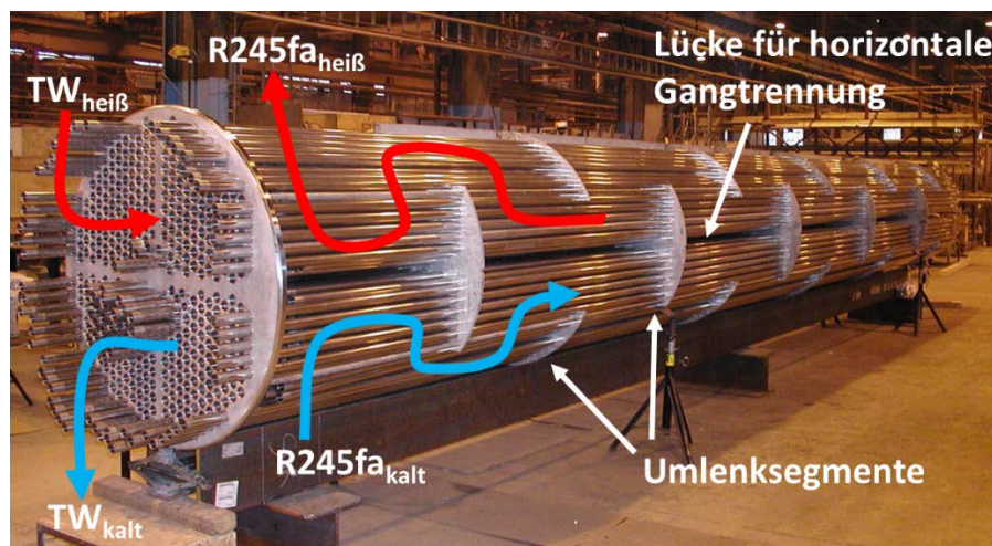
Abbildung 53: Teilmontierter Rohrbündel-Wärmeübertrager [vgl. 83].
