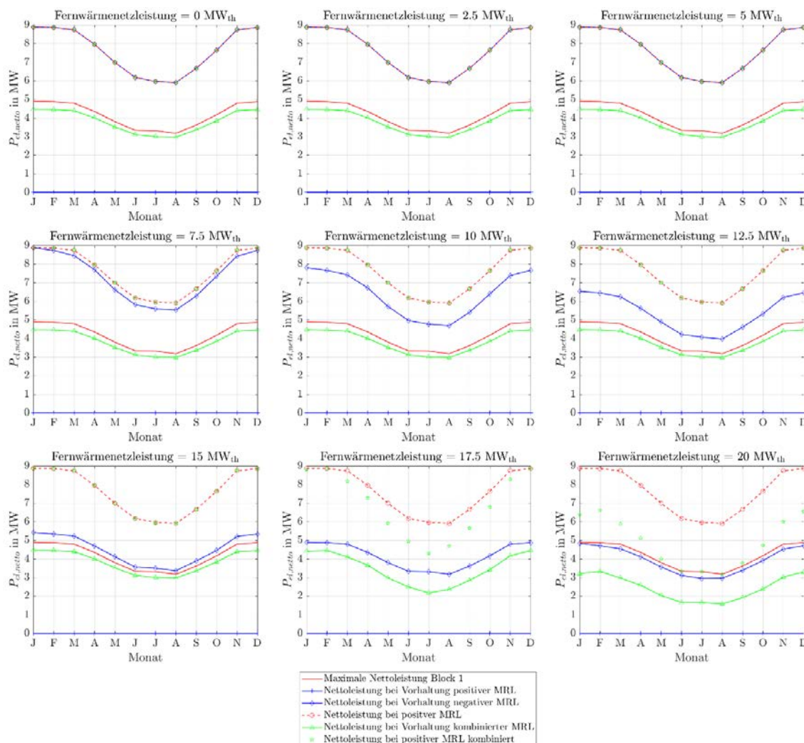
Abbildung 320: Stationäre Minutenregelleistungen des ORC-Referenz-Geothermie-Kraftwerks mit Einsatz eines Thermalwasserspeichers für Fernwärmenetzleistungen von 0 MW th bis 20 MW th bei drei 4h-Zeitscheiben Einspeicherung und zwei aufeinanderfolgenden Zeitscheiben Angebotszeitraum.
