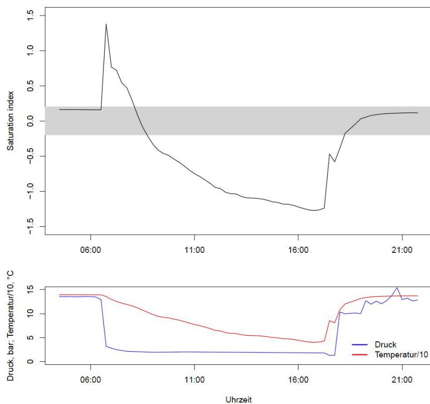
Abbildung 29: Druck, Temperatur und Sättigungsindex für Kalzit während einer kurzfristigen Abschaltung einer Anlage im Bayerischen Molassebecken.
