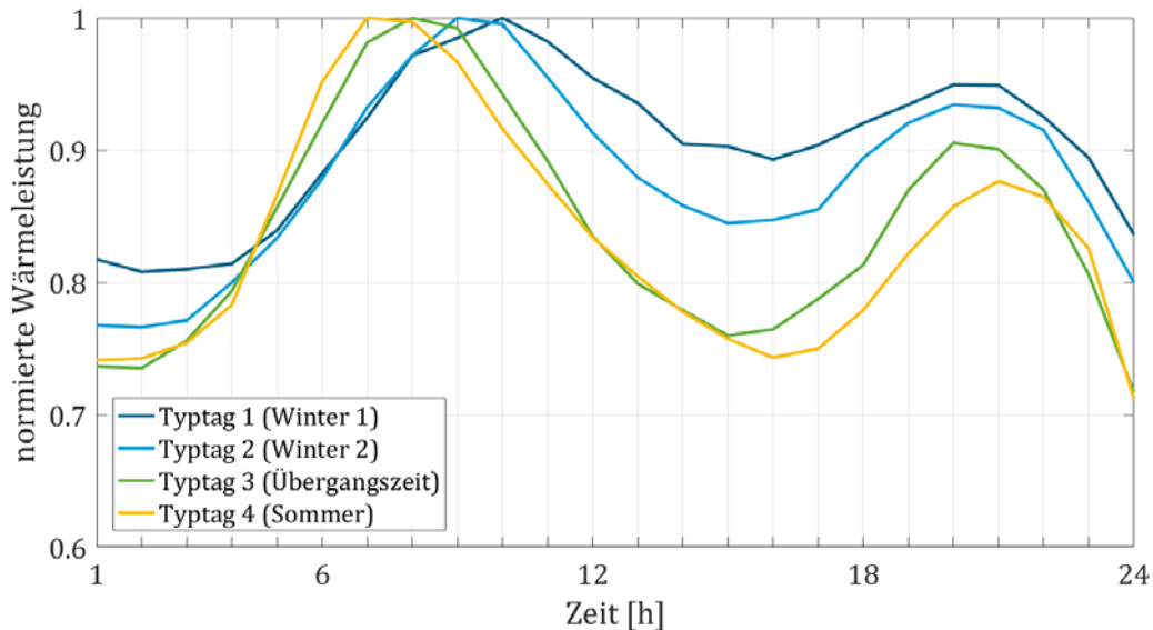
Abbildung 47: Normierte Wärmeleistung von ausgewählten Typtagen.
