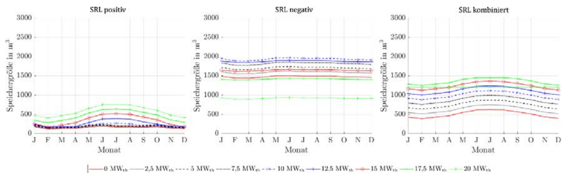
Abbildung 271: Benötigte Speichergrößen bei Angebot von positiver, negativer und kombinierter SRL des ORC-Referenz-Geothermie-Kraftwerks mit Einsatz eines Heißwasser-Wärmespeichers des Heiz- und Kraftwerks für Fernwärmenetzleistungen von 0 MW th bis 20 MW th bei zwei 4h-Zeitscheiben Einspeicherung und einer Zeitscheibe Angebotszeitraum.
