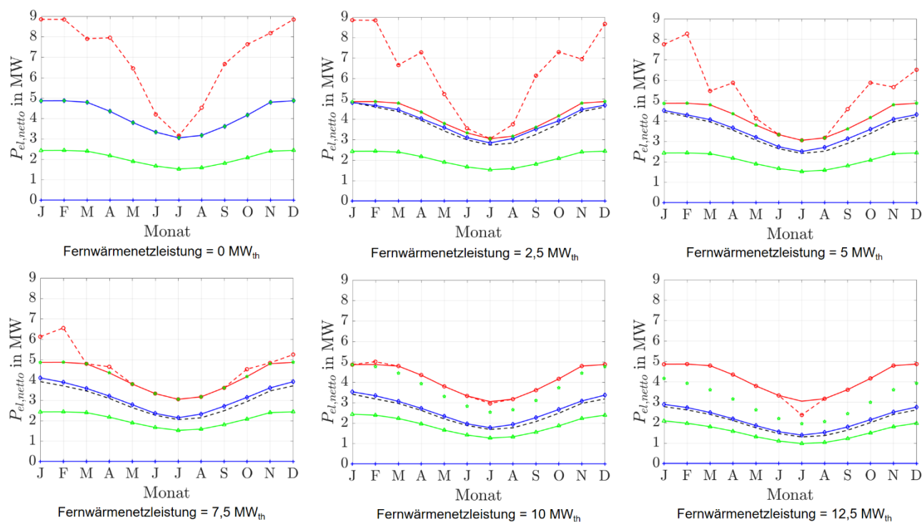
Abbildung 85: Stationäre Sekundärregelleistungen des ORC-Referenz-Geothermie-Kraftwerks mit Einsatz eines Thermalwasserspeichers für Fernwärmenetzleistungen von 0 MW th bis 20 MW th .
