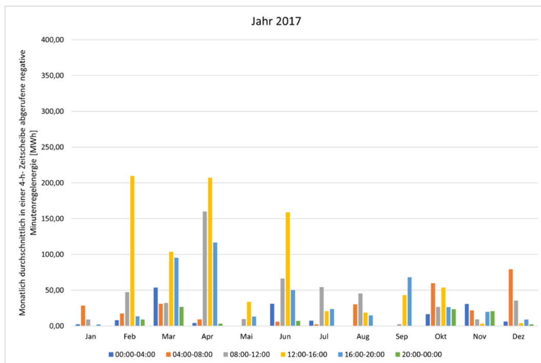
Abbildung 249: Monatlich durchschnittlich in einer 4h-Zeitscheibe abgerufene negative Minutenregelenergie 2017.
