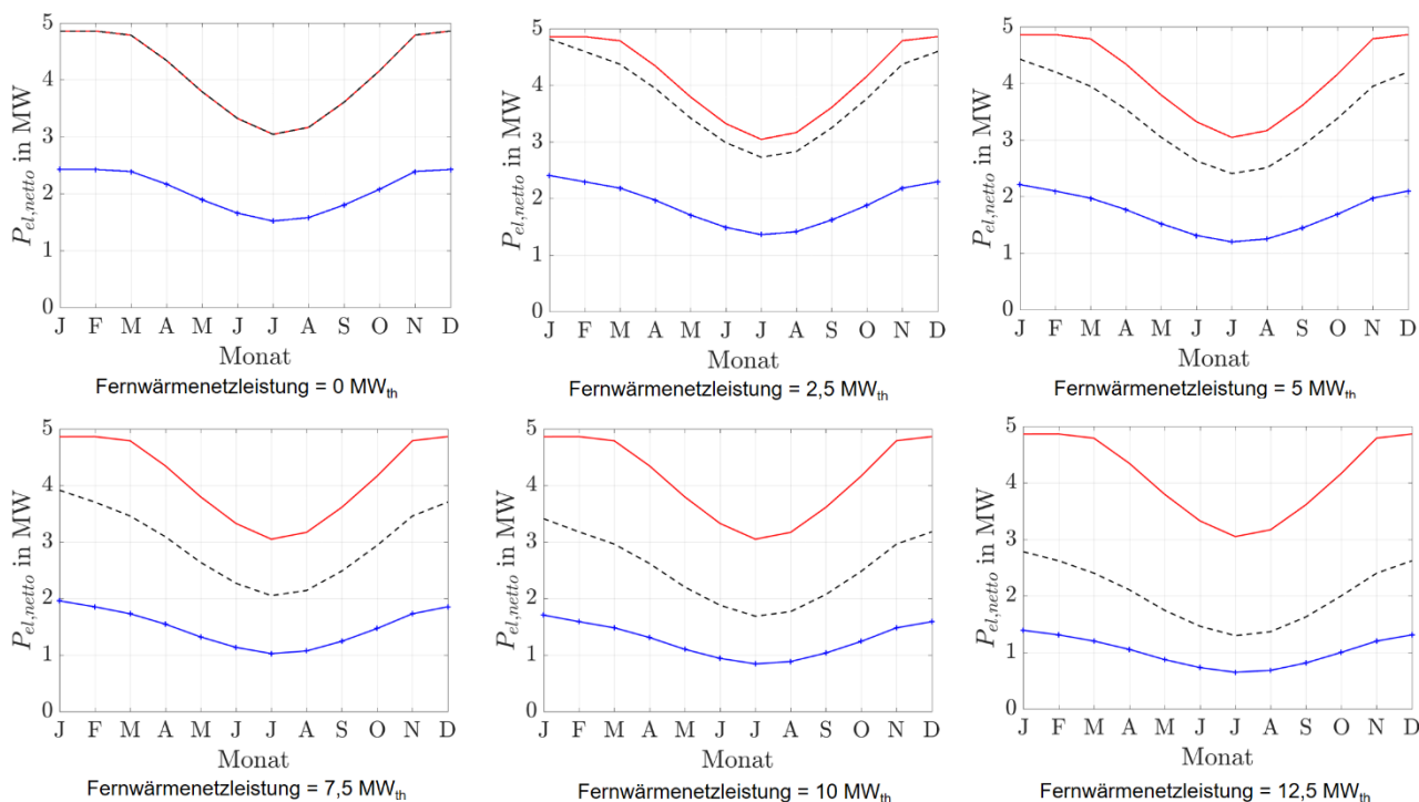
Abbildung 72: Stationäre Primärregelleistungen des ORC-Referenz-Geothermie-Kraftwerks im Bestand ohne Flexibilisierungsmaßnahmen für Fernwärmenetzleistungen von 0 MW th bis 20 MW th .
