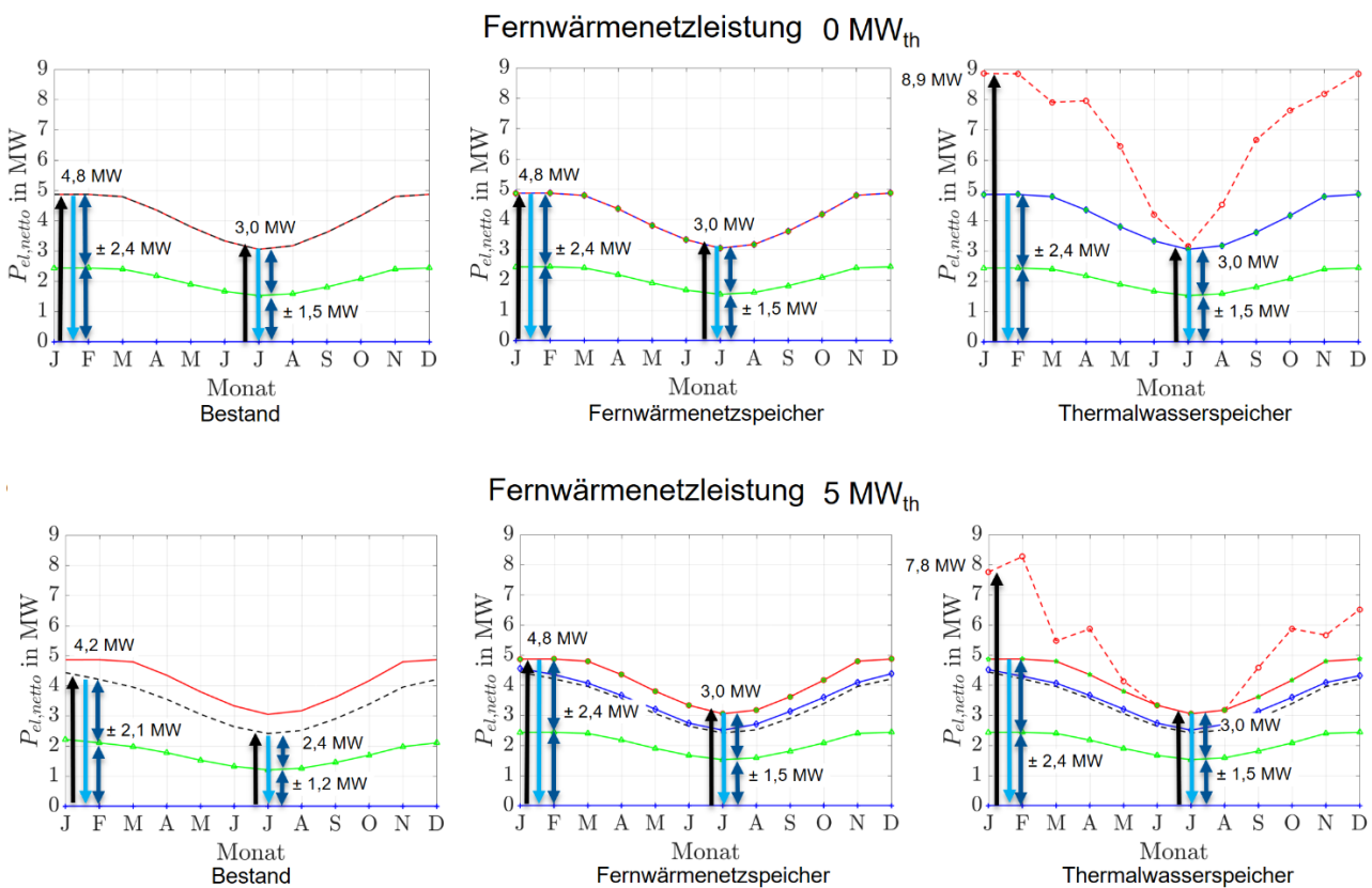
Abbildung 103: Vergleich der bereitstellbaren stationären Sekundärregelleistungen des ORC-Referenz-Geothermie-Kraftwerks mit den verschiedenen Flexibilisierungsoptionen für Heiz- und Kraftwerk für Fernwärmenetzleistungen von 0 \text{ MW}_{\text{th}} , 5 \text{ MW}_{\text{th}} und 10 \text{ MW}_{\text{th}} .
