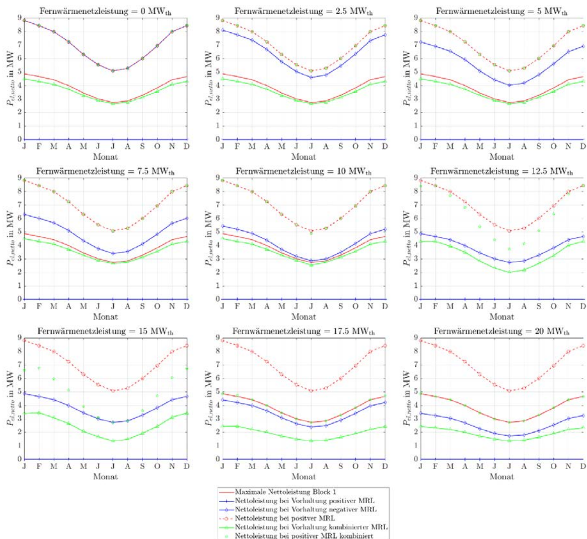
Abbildung 276: Stationäre Minutenregelleistungen des ORC-Referenz-Geothermie-Kraftwerks mit Einsatz eines Heißwasser-Wärmespeichers des Heiz- und Kraftwerks für Fernwärmenetzleistungen von 0 MW th bis 20 MW th bei einer 4h-Zeitscheibe Einspeicherung und einer Zeitscheibe Angebotszeitraum.
