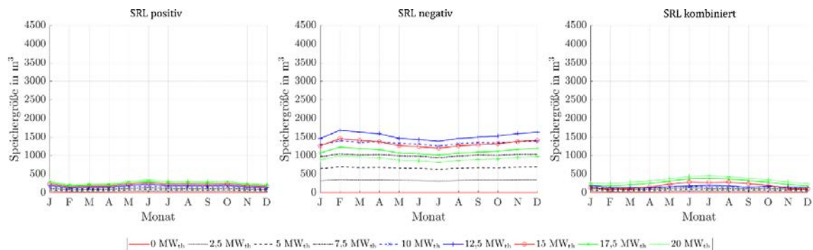
Abbildung 114: Benötigte Speichergrößen bei Angebot von positiver, negativer und kombinierter SRL des ORC-Referenz-Geothermie-Kraftwerks mit Einsatz eines Heißwasser-Wärmespeichers im Fernwärmenetz für Fernwärmenetzleistungen von 0 MW th bis 20 MW th bei einer 4h-Zeitscheibe Einspeicherung und zwei aufeinanderfolgenden Zeitscheiben Angebotszeitraum.
