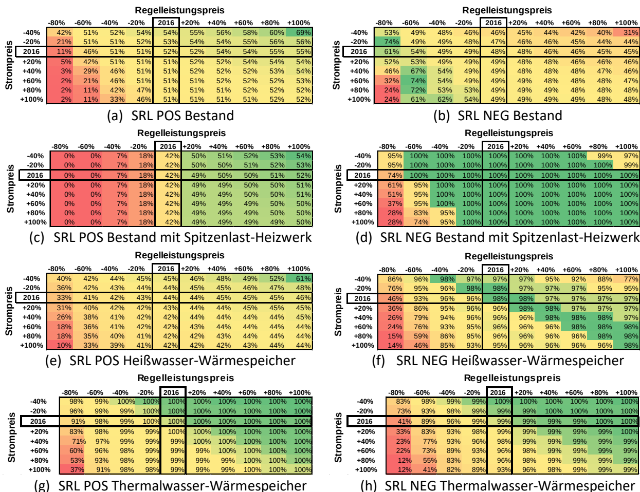
Abbildung 136: Ausnutzung des Potentials für positive und negative Sekundärregelleistung im wirtschaftlich optimalen Betrieb bei Marktpreisvergütung und Fernwärmenetz-Anschlussleistung 67,5 MW.
