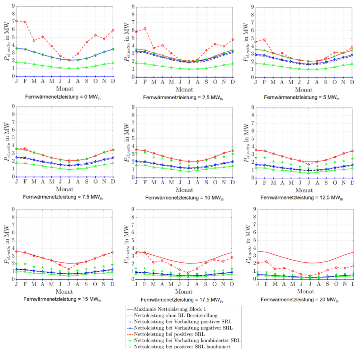
Abbildung 190: Stationäre Sekundärregelleistungen des Kalina-Referenz-Geothermie-Kraftwerks mit Einsatz eines Thermalwasserspeichers für Fernwärmenetzleistungen von 0 MW th bis 20 MW th .
