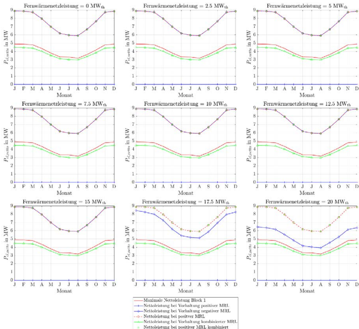
Abbildung 284: Stationäre Minutenregelleistungen des ORC-Referenz-Geothermie-Kraftwerks mit Einsatz eines Thermalwasserspeichers für Fernwärmenetzleistungen von 0 MW th bis 20 MW th bei drei 4h-Zeitscheiben Einspeicherung und einer Zeitscheibe Angebotszeitraum.
