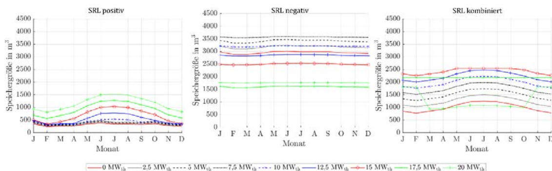
Abbildung 299: Benötigte Speichergrößen bei Angebot von positiver, negativer und kombinierter SRL des Referenz-Geothermie-Kraftwerks mit Einsatz eines Heißwasser-Wärmespeichers des Heiz- und Kraftwerks für Fernwärmenetzleistungen von 0 MW th bis 20 MW th bei drei 4h-Zeitscheiben Einspeicherung und zwei aufeinanderfolgenden Zeitscheiben Angebotszeitraum.
