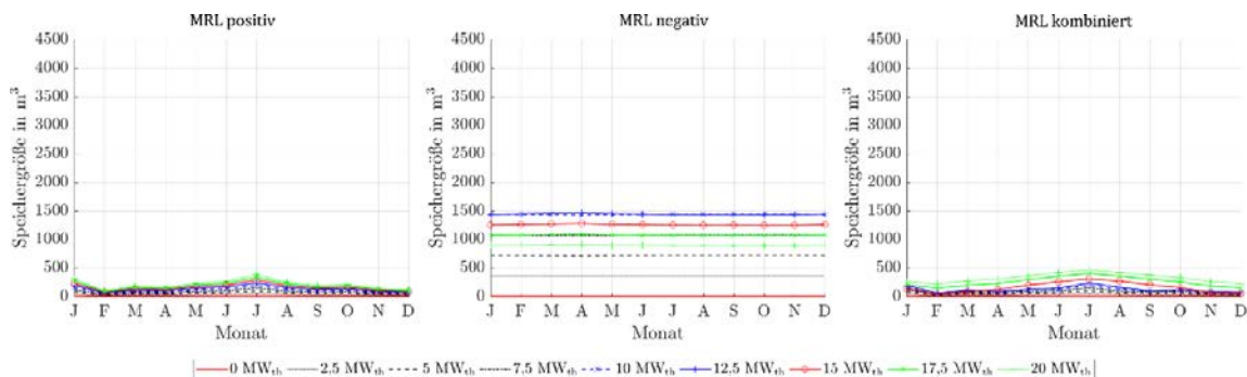
Abbildung 307: Benötigte Speichergrößen bei Angebot von positiver, negativer und kombinierter MRL des ORC-Referenz-Geothermie-Kraftwerks mit Einsatz eines Heißwasser-Wärmespeichers im Fernwärmenetz für Fernwärmenetzleistungen von 0 MW th bis 20 MW th bei einer 4h-Zeitscheibe Einspeicherung und zwei aufeinanderfolgenden Zeitscheiben Angebotszeitraum.
