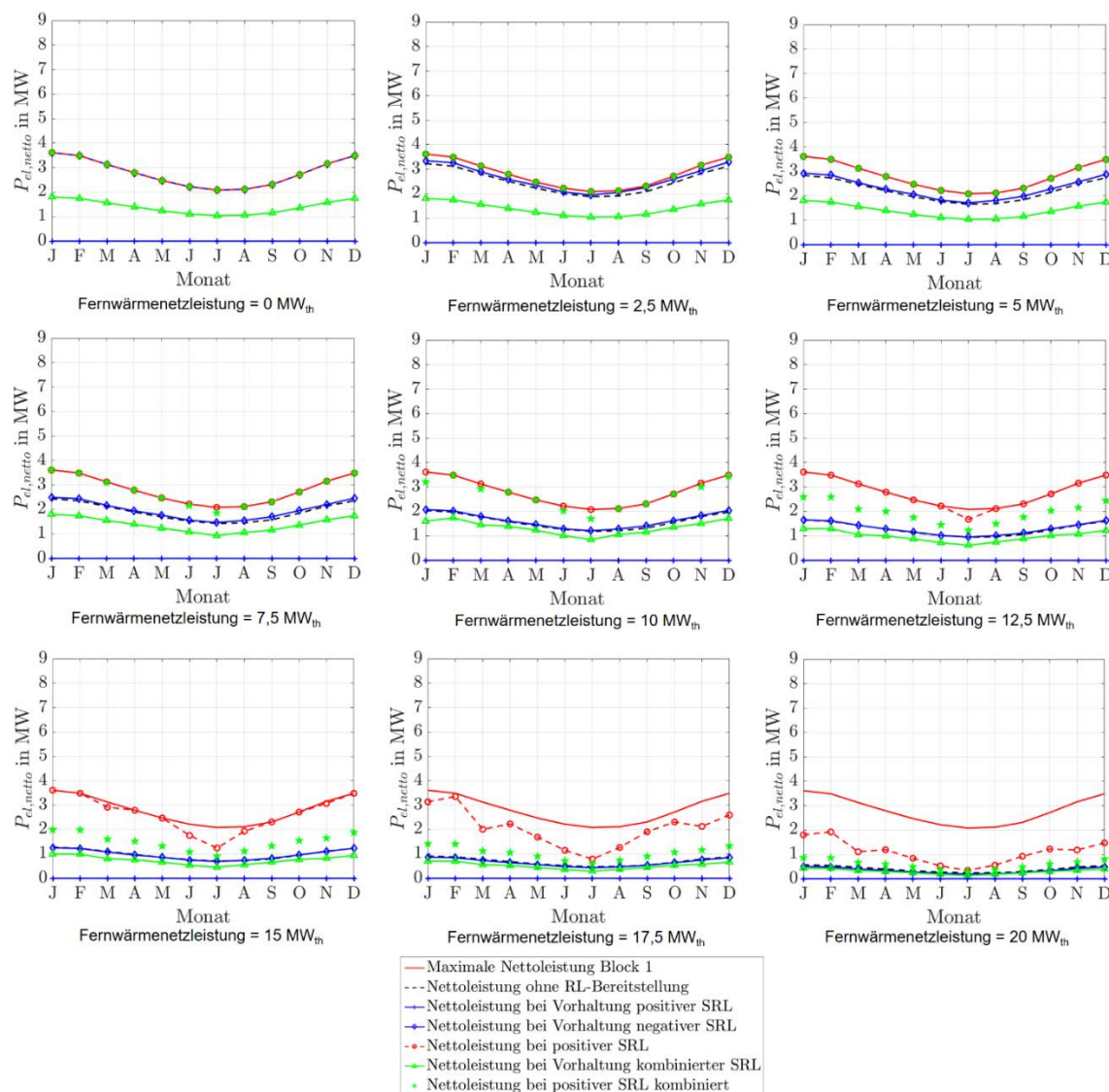
Abbildung 184: Stationäre Sekundärregelleistungen des Kalina-Referenz-Geothermie-Kraftwerks mit Einsatz eines Fernwärmenetzspeichers für Fernwärmenetzleistungen von 0 MW th bis 20 MW th .
