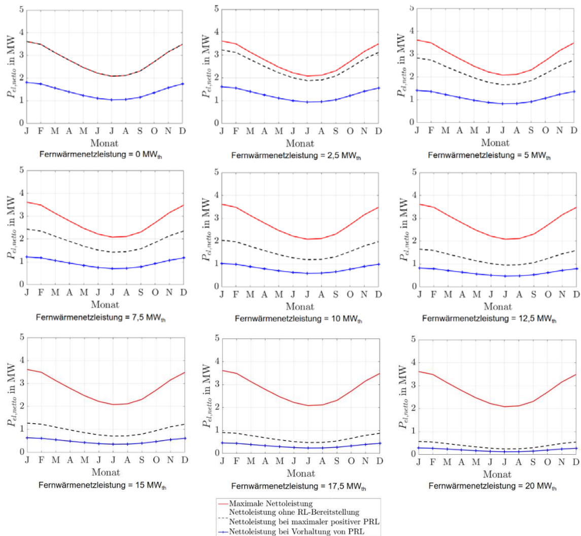
Abbildung 180: Stationäre Primärregelleistungen des Kalina-Referenz-Geothermie-Kraftwerks im Bestand ohne Flexibilisierungsmaßnahmen für Fernwärmenetzleistungen von 0 MW th bis 20 MW th .
