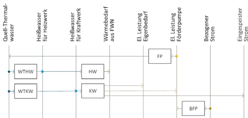
Abbildung 149: Referenzgeothermieranlage mit Umwandlungsprozessen: Wärmetauscher für Heizwerk (WTHW), Wärmetauscher für Kraftwerk (WTKW), Heizwerk (HW), Kraftwerk (KW), Förderpumpe (FP) und Strombezug für Förderpumpe (BFP).
