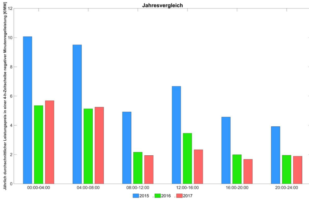
Abbildung 259: Jährlich durchschnittlicher Leistungspreis in einer 4h-Zeitscheibe negativer Minutenregelleistung.
