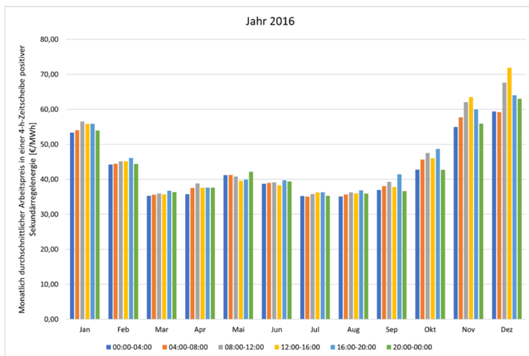
Abbildung 219: Monatlich durchschnittlicher Arbeitspreis in einer 4h-Zeitscheibe positiver Sekundärregelleistung 2016.
