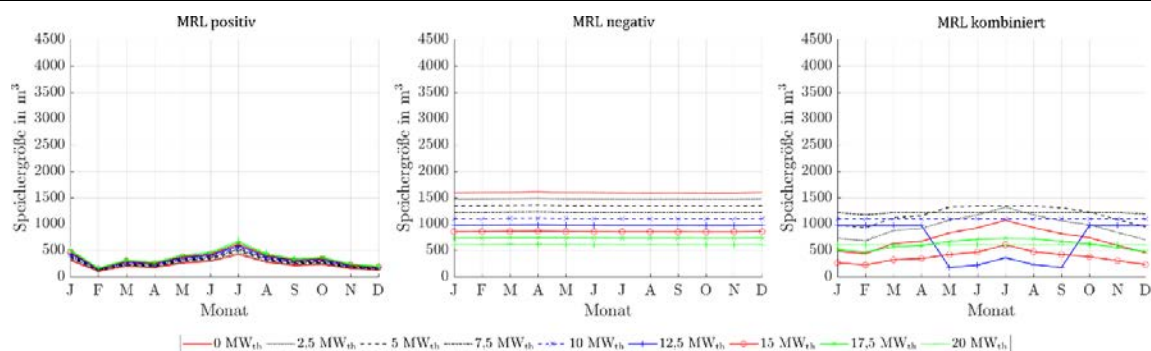
Abbildung 309: Benötigte Speichergrößen bei Angebot von positiver, negativer und kombinierter MRL des ORC-Referenz-Geothermie-Kraftwerks mit Einsatz eines Thermalwasserspeichers im Kraftwerk für Fernwärmenetzleistungen von 0 MW th bis 20 MW th bei einer 4h-Zeitscheibe Einspeicherung und zwei aufeinanderfolgenden Zeitscheiben Angebotszeitraum.
