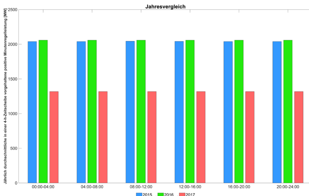
Abbildung 256: Jährlich durchschnittlicher in einer 4h-Zeitscheibe vorgehaltene positive Minutenregelleistung.
