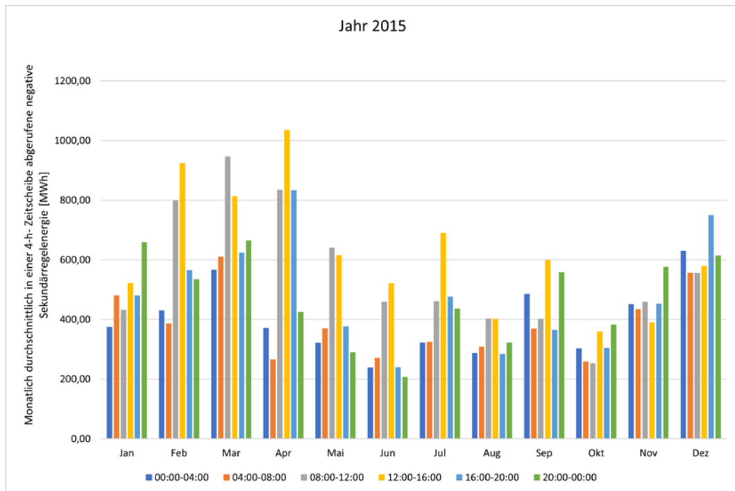
Abbildung 215: Monatlich durchschnittlich in einer 4h-Zeitscheibe abgerufene negative Sekundärregelleistung 2015.
