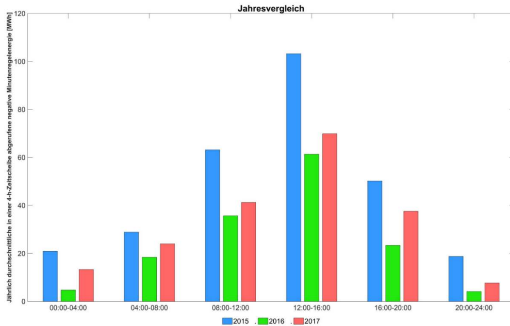
Abbildung 261: Jährlich durchschnittlich in einer 4h-Zeitscheibe abgerufene negative Minutenregelenergie.
