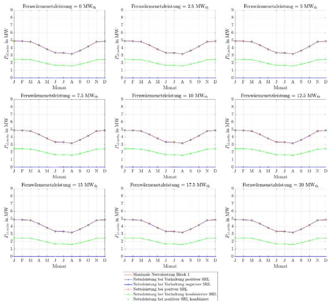
Abbildung 300: Stationäre Sekundärregelleistungen des ORC-Referenz-Geothermie-Kraftwerks mit Einsatz eines Heißwasser-Wärmespeichers im Fernwärmenetz für Fernwärmenetzleistungen von 0 MW th bis 20 MW th bei vier 4h-Zeitscheiben Einspeicherung und zwei aufeinanderfolgenden Zeitscheiben Angebotszeitraum.
