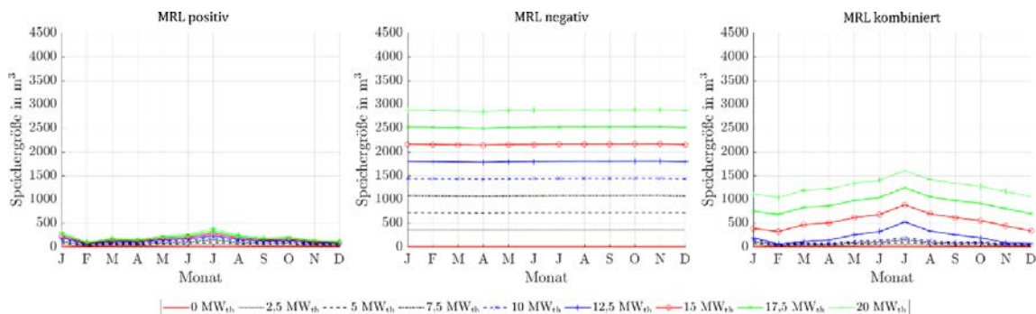
Abbildung 325: Benötigte Speichergrößen bei Angebot von positiver, negativer und kombinierter MRL des ORC-Referenz-Geothermie-Kraftwerks mit Einsatz eines Heißwasser-Wärmespeichers im Fernwärmenetz für Fernwärmenetzleistungen von 0 MW th bis 20 MW th bei vier 4h-Zeitscheiben Einspeicherung und zwei aufeinanderfolgenden Zeitscheiben Angebotszeitraum.
