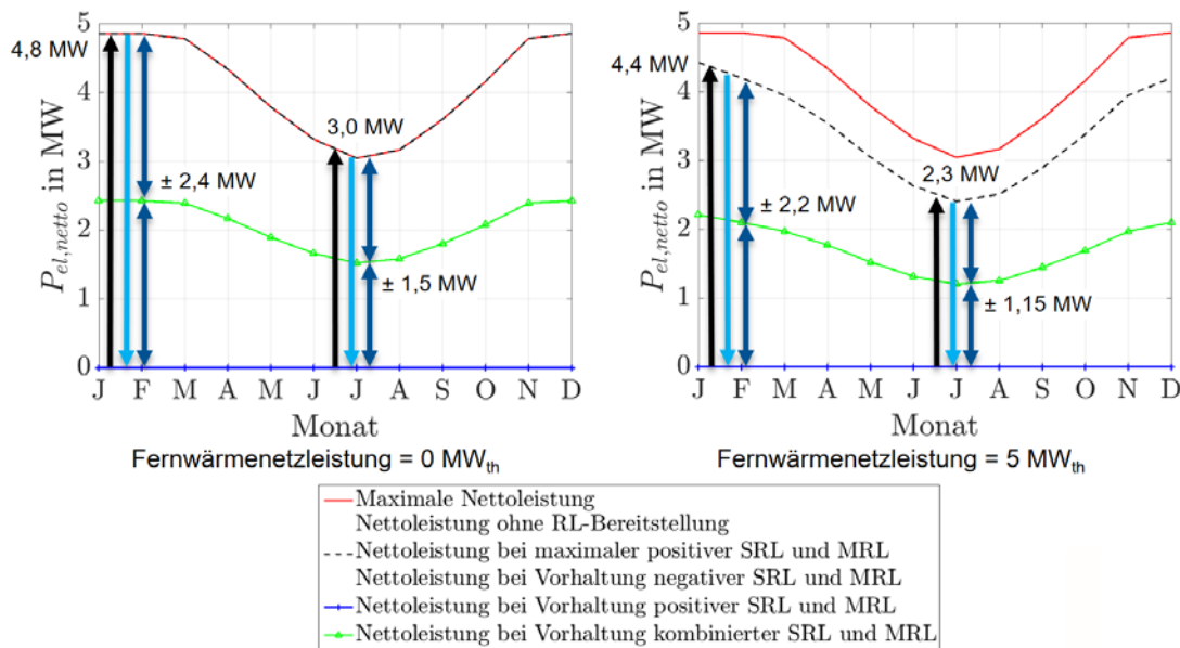
Abbildung 73: Stationäre Sekundär- und Minutenregelleistung des ORC-Referenz-Geothermie-Kraftwerks im Bestand ohne Flexibilisierungsmaßnahmen für die Fernwärmenetzleistungen 0 MW th und 5 MW th .
