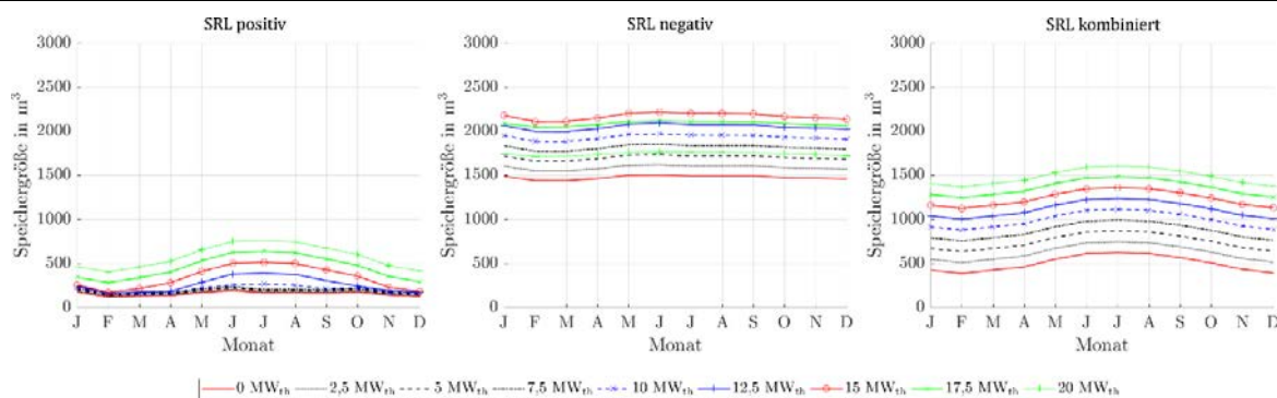
Abbildung 112: Benötigte Speichergrößen bei Angebot von positiver, negativer und kombinierter SRL des ORC-Referenz-Geothermie-Kraftwerks mit Einsatz eines Heißwasser-Wärmespeichers des Heiz- und Kraftwerks für Fernwärmenetzleistungen von 0 MW th bis 20 MW th bei drei 4h-Zeitscheiben Einspeicherung und einer Zeitscheibe Angebotszeitraum.
