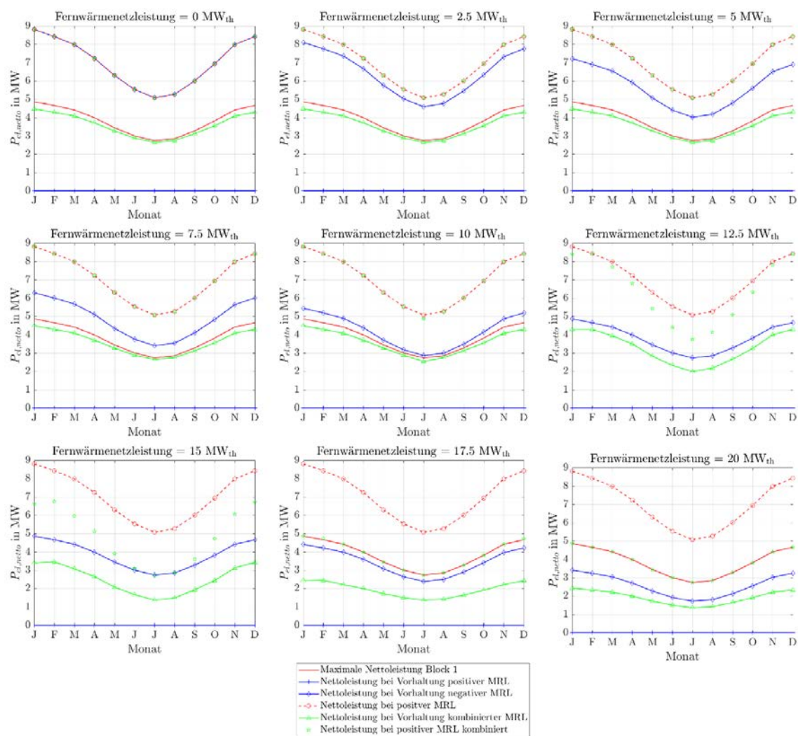
Abbildung 316: Stationäre Minutenregelleistungen des ORC-Referenz-Geothermie-Kraftwerks mit Einsatz eines Heißwasser-Wärmespeichers des Heiz- und Kraftwerks für Fernwärmenetzleistungen von 0 MW th bis 20 MW th bei zwei 4h-Zeitscheiben Einspeicherung und zwei aufeinanderfolgenden Zeitscheiben Angebotszeitraum.
