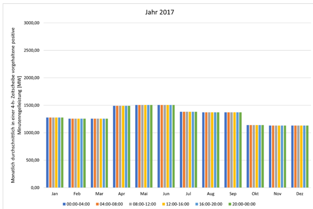
Abbildung 234: Monatlich durchschnittlich in einer 4h-Zeitscheibe vorgehaltene positive Minutenregel-leistung 2017.
