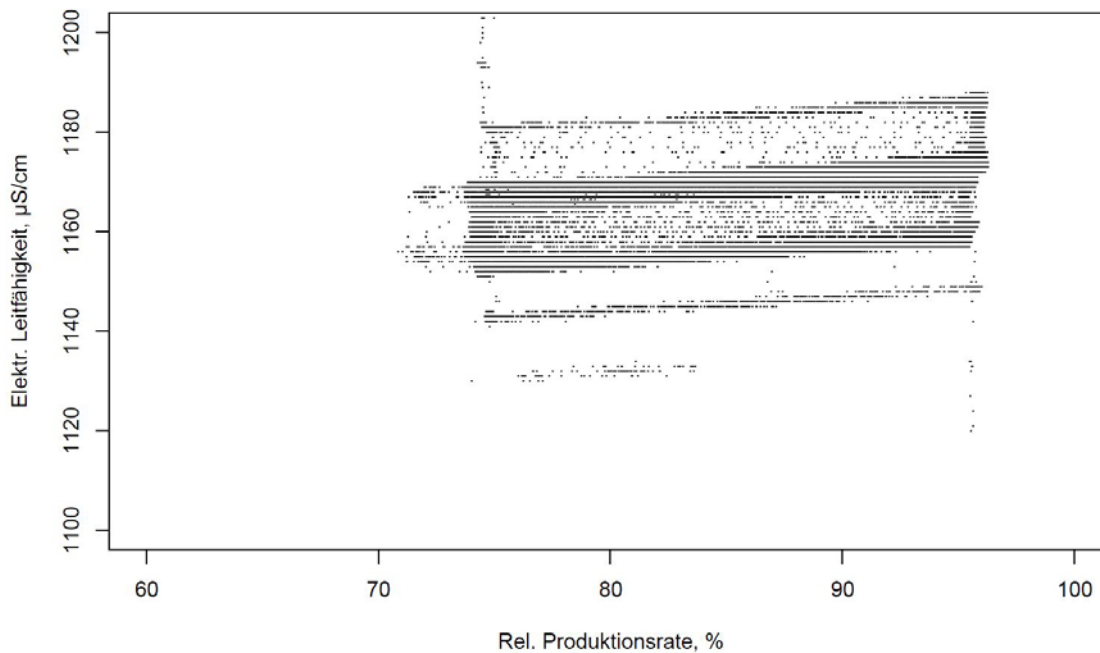
Abbildung 12: Elektrische Leitfähigkeit des produzierten Wassers als Funktion der relativen Produktionsrate in einem Geothermieheizwerk im Molassebecken.
