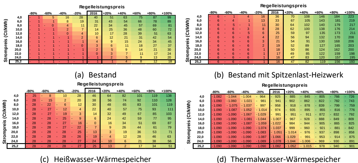
Abbildung 142: Sensitivität der Mehrgewinne (p.a.) in 10 3 EUR im wirtschaftlich optimalen Betrieb bei fester Einspeisevergütung und Fernwärmenetz-Anschlussleistung von 67,5 MW.
