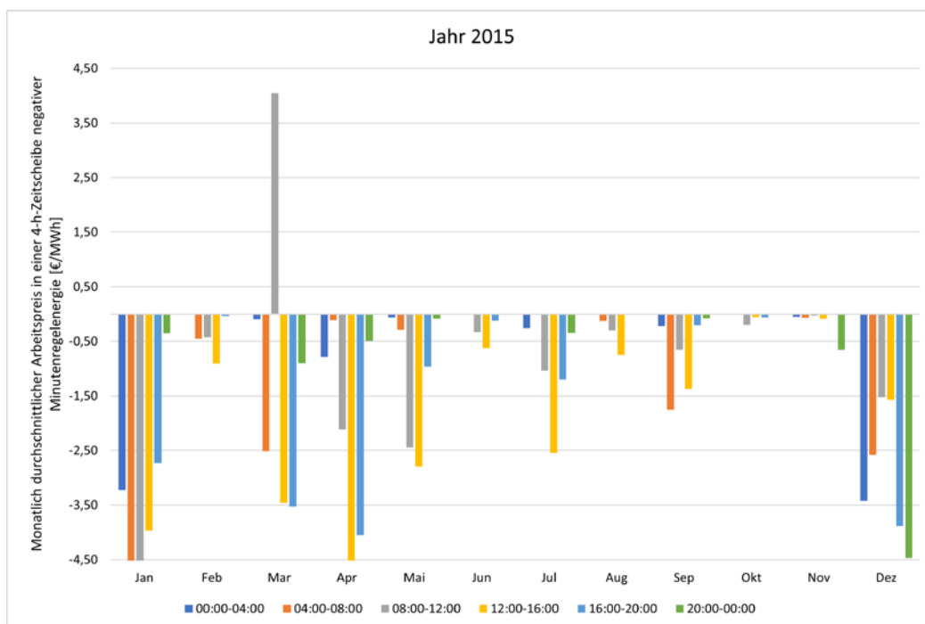
Abbildung 253: Monatlich durchschnittlicher Arbeitspreis in einer 4h-Zeitscheibe negativer Minutenregelleistung 2015.
