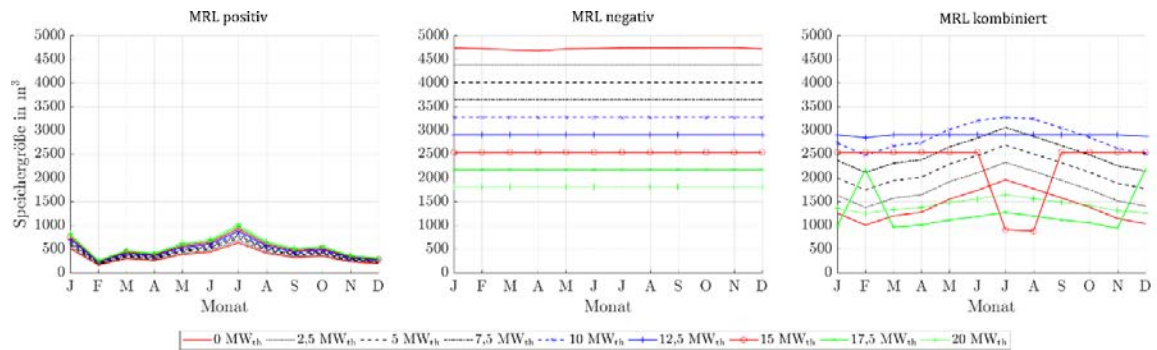
Abbildung 335: Benötigte Speichergrößen bei Angebot von positiver, negativer und kombinierter MRL des Referenz-Geothermie-Kraftwerks mit Einsatz eines Heißwasser-Wärmespeichers des Heiz- und Kraftwerks für Fernwärmenetzleistungen von 0 MW th bis 20 MW th bei drei 4h-Zeitscheiben Einspeicherung und drei aufeinanderfolgenden Zeitscheiben Angebotszeitraum.
