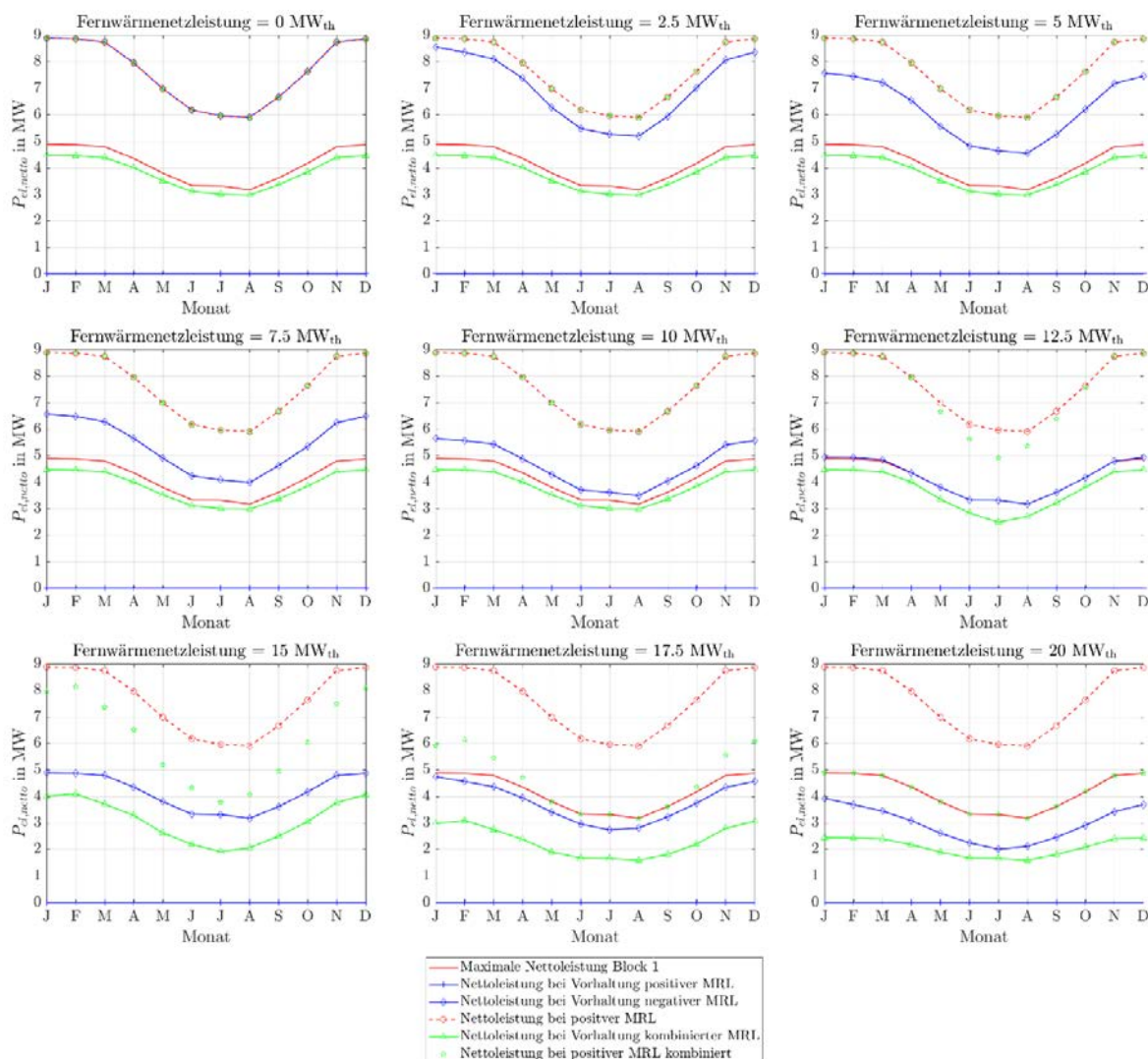
Abbildung 274: Stationäre Minutenregelleistungen des ORC-Referenz-Geothermie-Kraftwerks mit Einsatz eines Thermalwasserspeichers für Fernwärmenetzleistungen von 0 MW th bis 20 MW th bei einer 4h-Zeitscheibe Einspeicherung und einer Zeitscheibe Angebotszeitraum.
