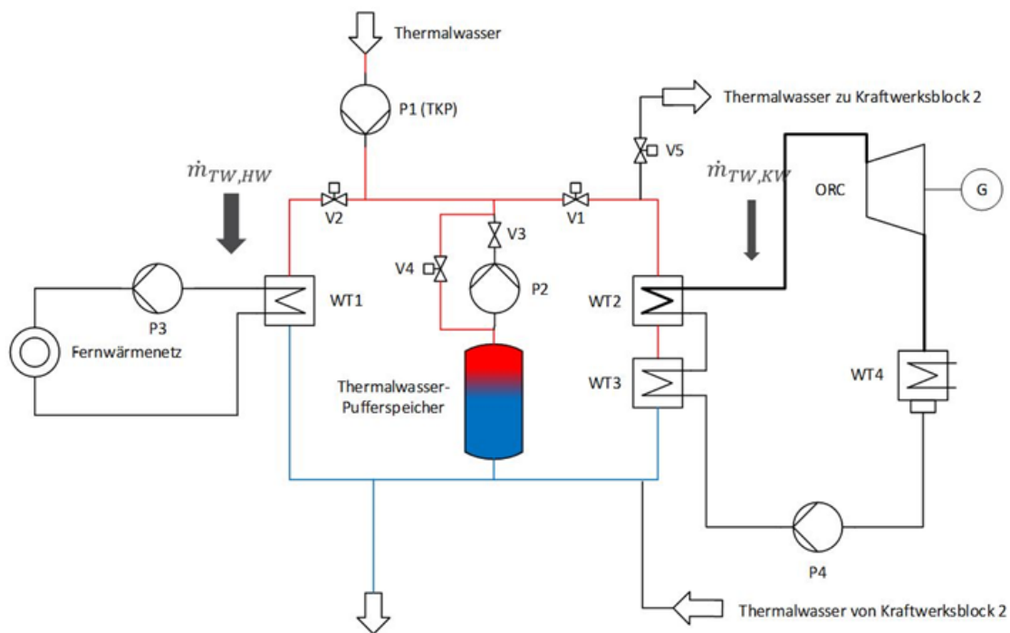
Abbildung 38: Verfahrensfließbild einer Geothermieranlage mit parallel geschaltetem Heiz- und Kraftwerk und einem in das Kraftwerk integrierten Thermalwasser-Wärmespeicher – negative Regelleistungsbereitstellung – Ladevorgang des Thermalwasser-Wärmespeichers.
