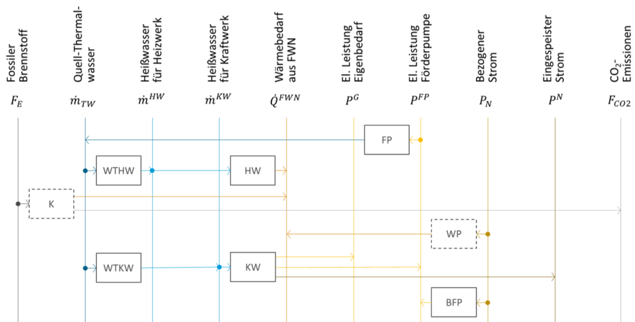
Abbildung 151: Geothermieranlage im Bestand mit einem fossilen Heizkessel und einer Wärmepumpe als alternative Wärmeerzeugungstechnologien.
