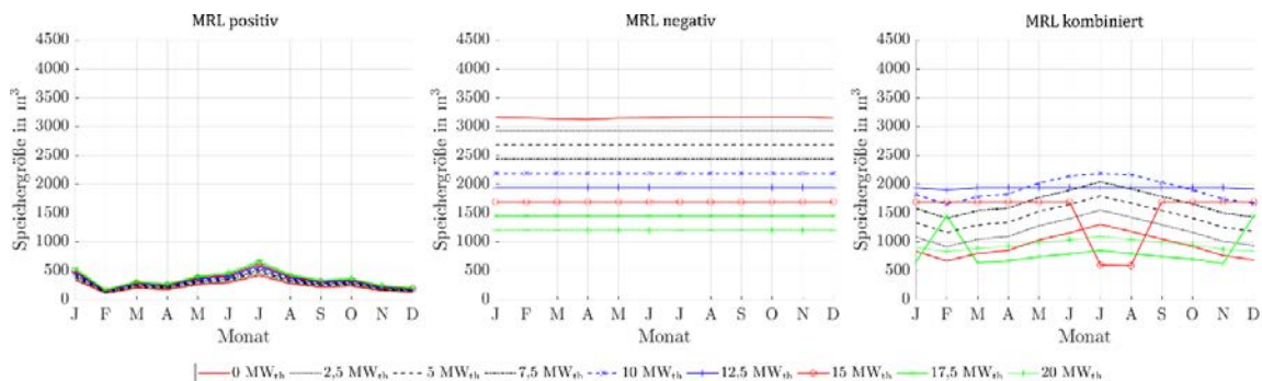
Abbildung 317: Benötigte Speichergrößen bei Angebot von positiver, negativer und kombinierter MRL des ORC-Referenz-Geothermie-Kraftwerks mit Einsatz eines Heißwasser-Wärmespeichers des Heiz- und Kraftwerks für Fernwärmenetzleistungen von 0 MW th bis 20 MW th bei zwei 4h-Zeitscheiben Einspeicherung und zwei aufeinanderfolgenden Zeitscheiben Angebotszeitraum.
