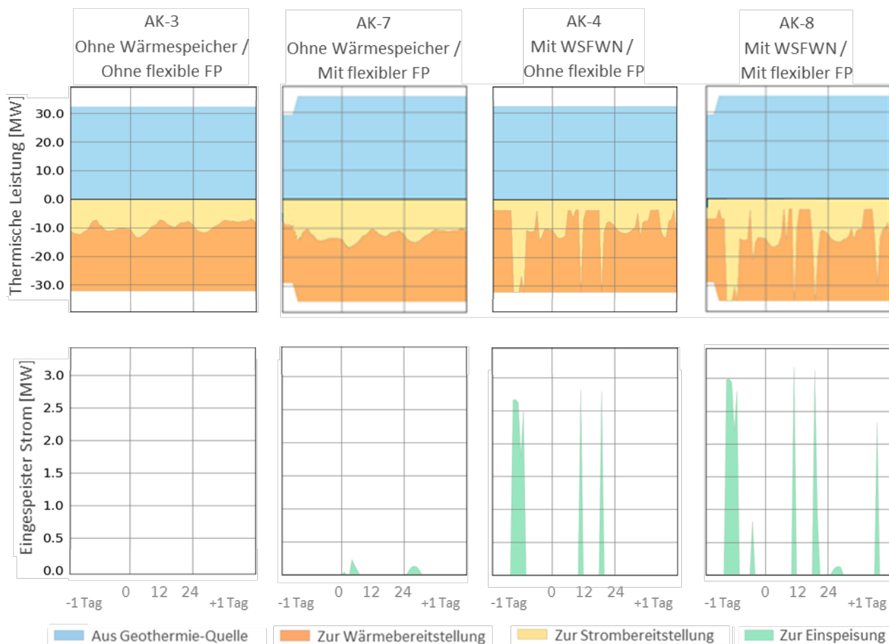
Abbildung 169: Thermalwasserfluss und Einspeisung an drei aufeinanderfolgenden Wintertagen (hoch) für Anlagenkonfigurationen: ohne Wärmespeicher und ohne flexiblen Betrieb der Förderpumpe (AK-3), ohne Wärmespeicher und mit flexiblen Betrieb der Förderpumpe (AK-7), mit Wärmespeicher im FWN und ohne flexiblen Betrieb (AK-4) und mit Wärmespeicher im FWN (AK-5) und mit flexiblen Betrieb der Förderpumpe (AK-8).
