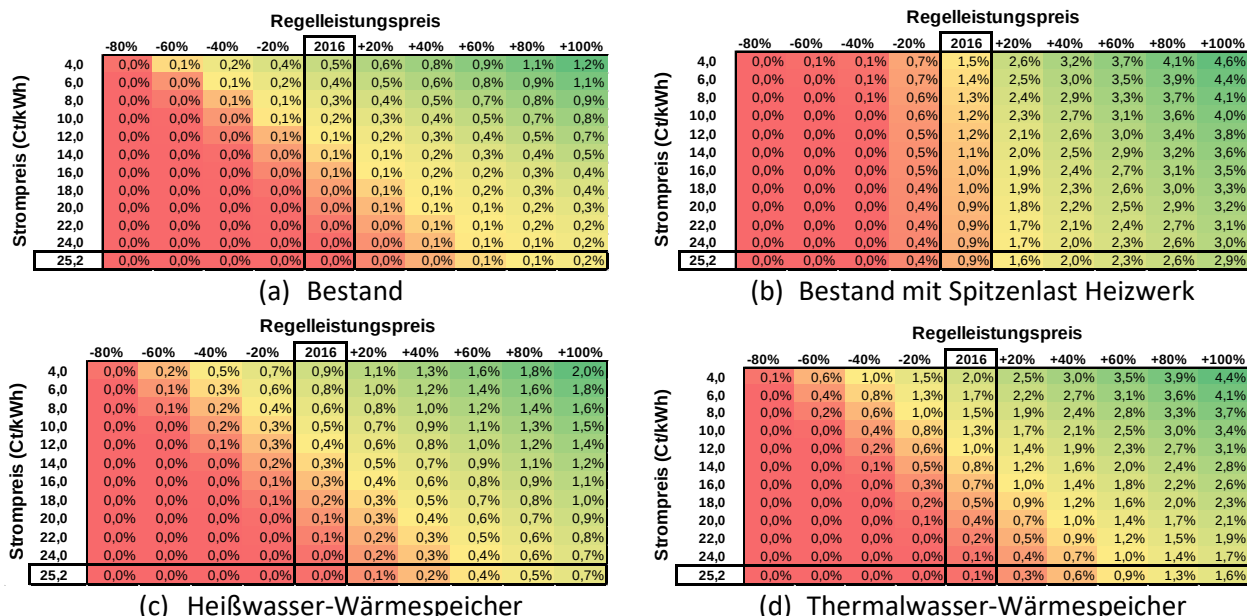
Abbildung 139: Sensitivität der Mehrerlöse der ORC-Referenzanlage im wirtschaftlich optimalen Betrieb für unterschiedliche Flexibilitätsoptionen bei EEG-Vergütung und Fernwärmenetz-Anschlussleistung von 67,5 MW.
