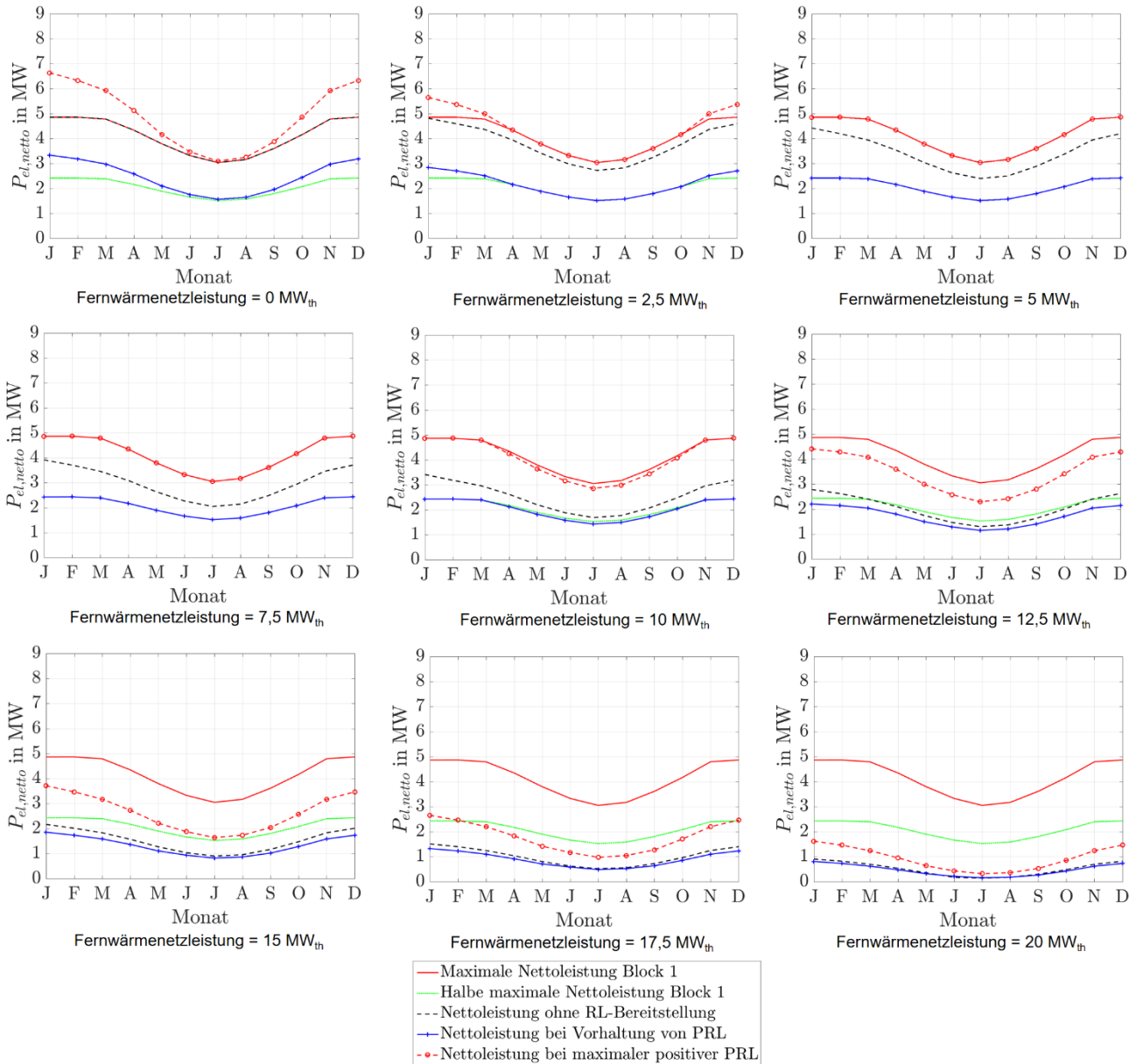
Abbildung 83: Stationäre Primärregelleistungen des ORC-Referenz-Geothermie-Kraftwerks mit Einsatz eines Thermalwasserspeichers für Fernwärmenetzleistungen von 0 MW th bis 20 MW th .
