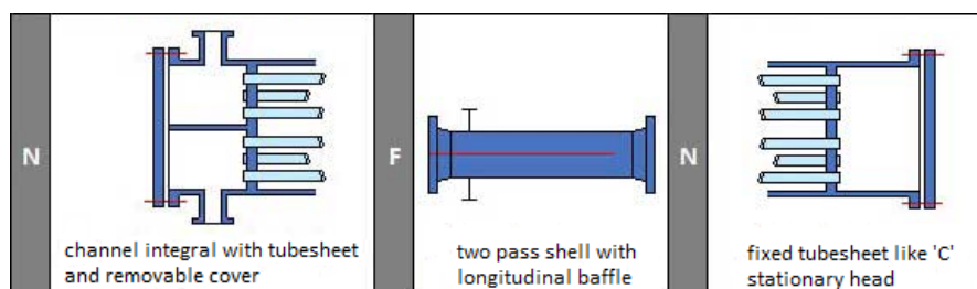
Abbildung 51: Aufbau des HHT-, LHT und LT-Vorwärmer nach TEMA-Standard [vgl. 81].
