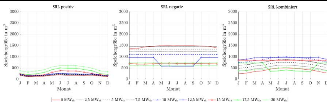
Abbildung 265: Benötigte Speichergrößen bei Angebot von positiver, negativer und kombinierter SRL des ORC-Referenz-Geothermie-Kraftwerks mit Einsatz eines Thermalwasserspeichers im Kraftwerk für Fernwärmenetzleistungen von 0 MW th bis 20 MW th bei einer 4h-Zeitscheibe Einspeicherung und einer Zeitscheibe Angebotszeitraum.
