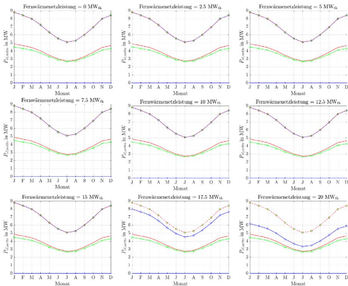
Abbildung 286: Stationäre Minutenregelleistungen des ORC-Referenz-Geothermie-Kraftwerks mit Einsatz eines Heißwasser-Wärmespeichers des Heiz- und Kraftwerks für Fernwärmenetzleistungen von 0 MW th bis 20 MW th bei drei 4h-Zeitscheiben Einspeicherung und einer Zeitscheibe Angebotszeitraum.
