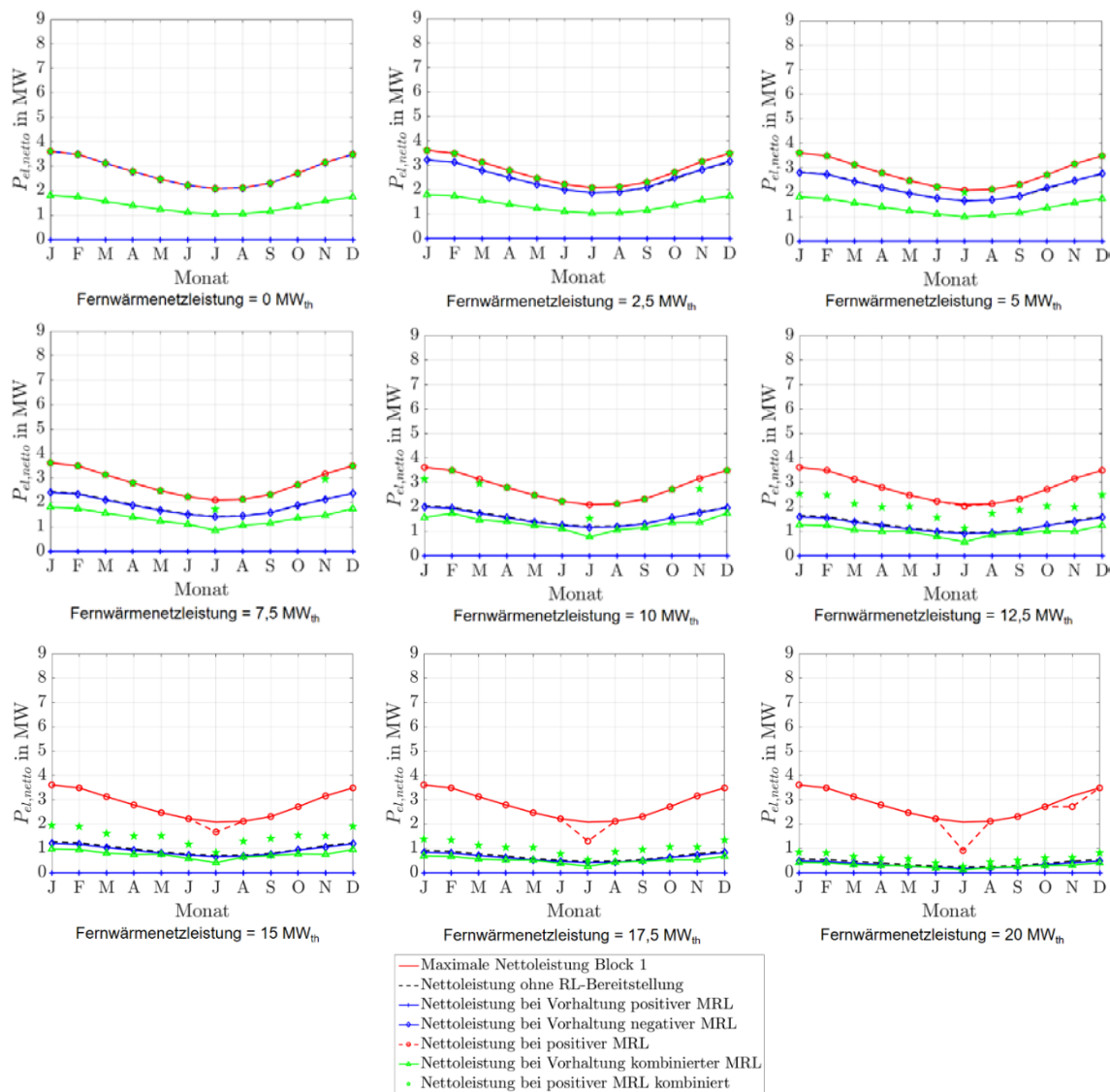
Abbildung 186: Stationäre Minutenregelleistungen des Kalina-Referenz-Geothermie-Kraftwerks mit Einsatz eines Fernwärmenetzspeichers für Fernwärmenetzleistungen von 0 MW th bis 20 MW th .
