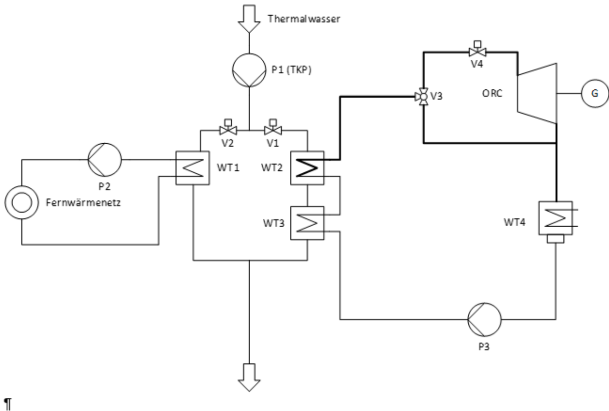
Abbildung 32: Verfahrensfließbild von Geothermieranlagen im Bestand mit parallel geschaltetem Heiz- und Kraftwerk, einem einstufigen ORC-Prozess und Turbinenregelventil.
