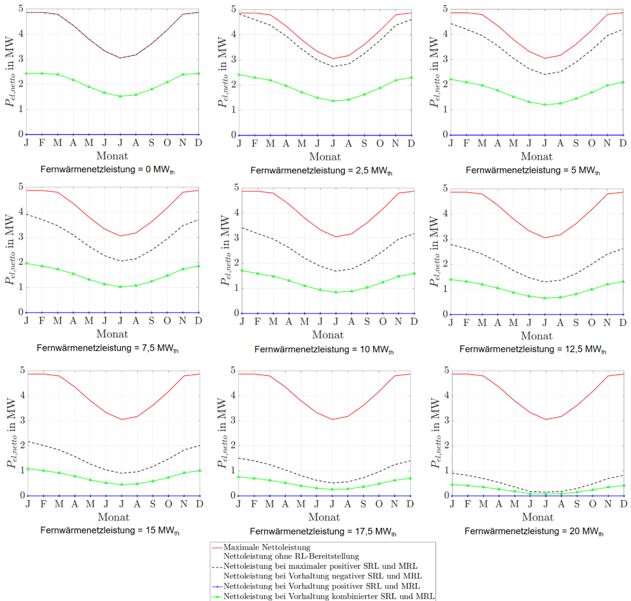
Abbildung 74: Stationäre Sekundär- und Minutenregelleistung des ORC-Referenz-Geothermie-Kraftwerks im Bestand ohne Flexibilisierungsmaßnahmen für Fernwärmenetzleistungen von 0 MW th bis 20 MW th .
