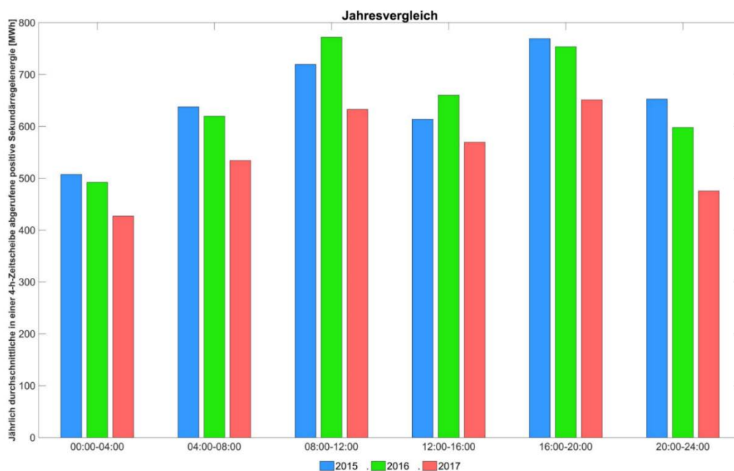
Abbildung 228: Jährlich durchschnittlich in einer 4h-Zeitscheibe abgerufene positive Sekundärregelenergie.
