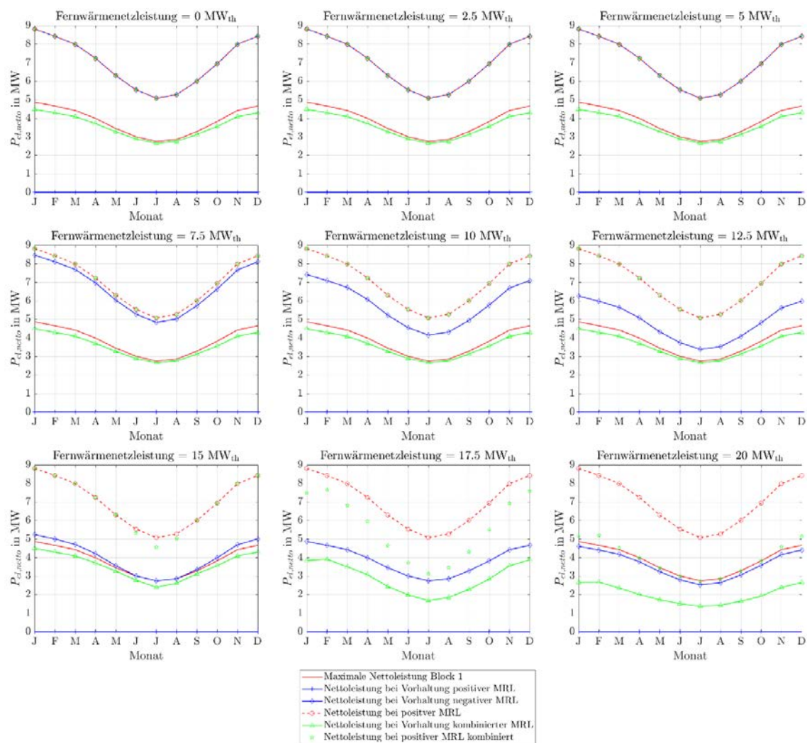
Abbildung 322: Stationäre Minutenregelleistungen des ORC-Referenz-Geothermie-Kraftwerks mit Einsatz eines Heißwasser-Wärmespeichers des Heiz- und Kraftwerks für Fernwärmenetzleistungen von 0 MW th bis 20 MW th bei drei 4h-Zeitscheiben Einspeicherung und zwei aufeinanderfolgenden Zeitscheiben Angebotszeitraum.
