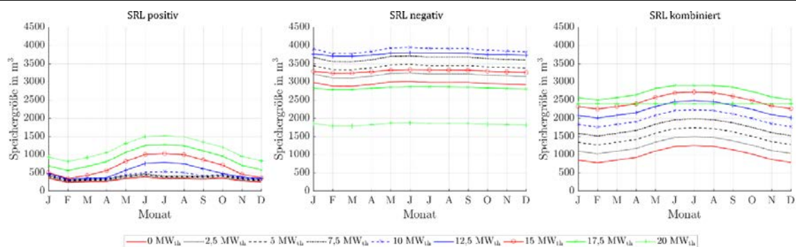
Abbildung 305: Benötigte Speichergrößen bei Angebot von positiver, negativer und kombinierter SRL des Referenz-Geothermie-Kraftwerks mit Einsatz eines Heißwasser-Wärmespeichers des Heiz- und Kraftwerks für Fernwärmenetzleistungen von 0 MW th bis 20 MW th bei vier 4h-Zeitscheiben Einspeicherung und zwei aufeinanderfolgenden Zeitscheiben Angebotszeitraum.
