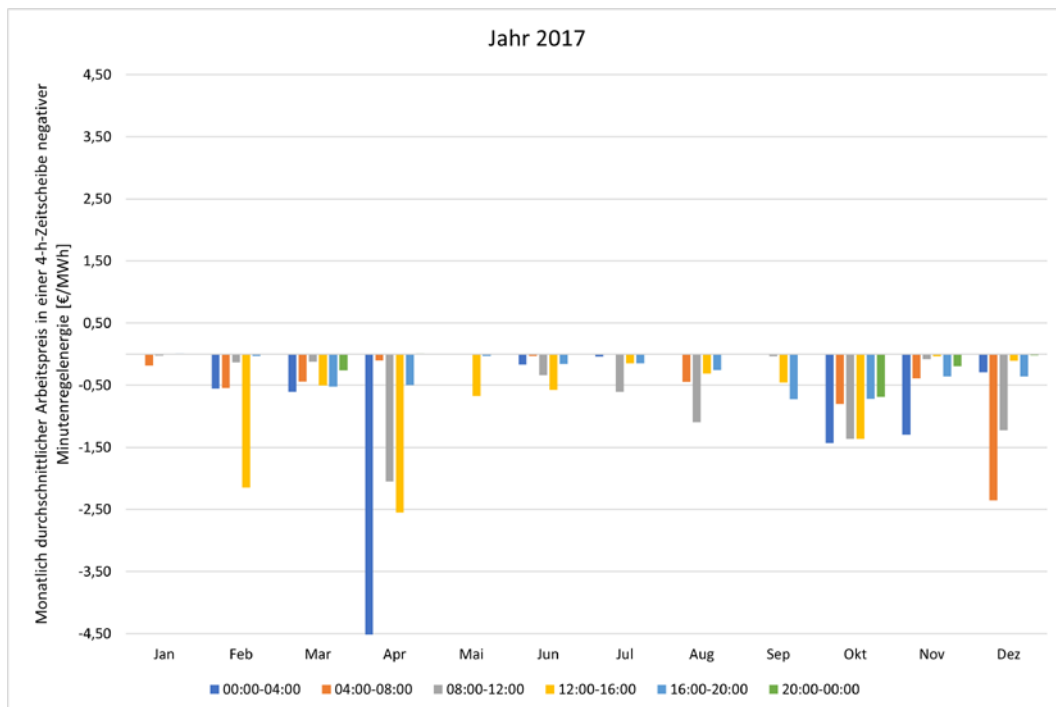
Abbildung 255: Monatlich durchschnittlicher Arbeitspreis in einer 4h-Zeitscheibe negativer Minutenregelleistung 2017.
