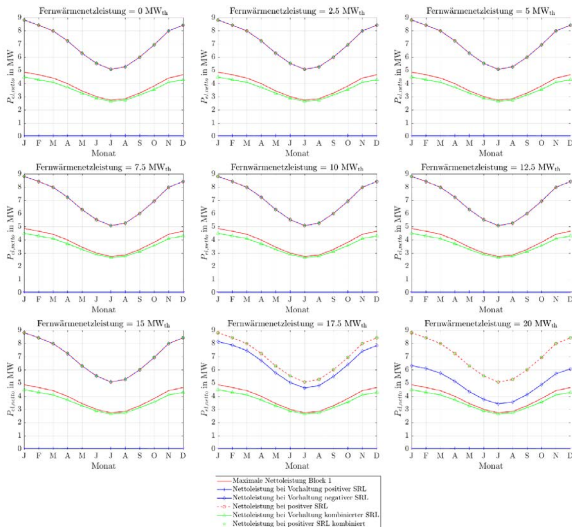
Abbildung 111: Stationäre Sekundärregelleistungen des ORC-Referenz-Geothermie-Kraftwerks mit Einsatz eines Heißwasser-Wärmespeichers des Heiz- und Kraftwerks für Fernwärmenetzleistungen von 0 MW th bis 20 MW th bei drei 4h-Zeitscheiben Einspeicherung und einer Zeitscheibe Angebotszeitraum.
