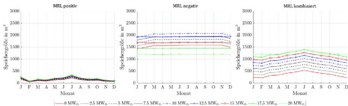
Abbildung 281: Benötigte Speichergrößen bei Angebot von positiver, negativer und kombinierter MRL des ORC-Referenz-Geothermie-Kraftwerks mit Einsatz eines Thermalwasserspeichers im Kraftwerk für Fernwärmenetzleistungen von 0 MW th bis 20 MW th bei zwei 4h-Zeitscheiben Einspeicherung und einer Zeitscheibe Angebotszeitraum.
