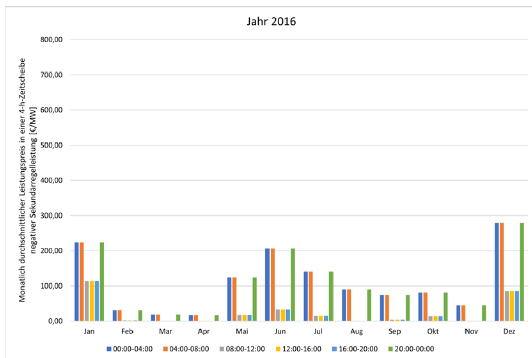
Abbildung 210: Monatlich durchschnittlicher Leistungspreis in einer 4h-Zeitscheibe negativer Sekundärregelleistung 2016.
