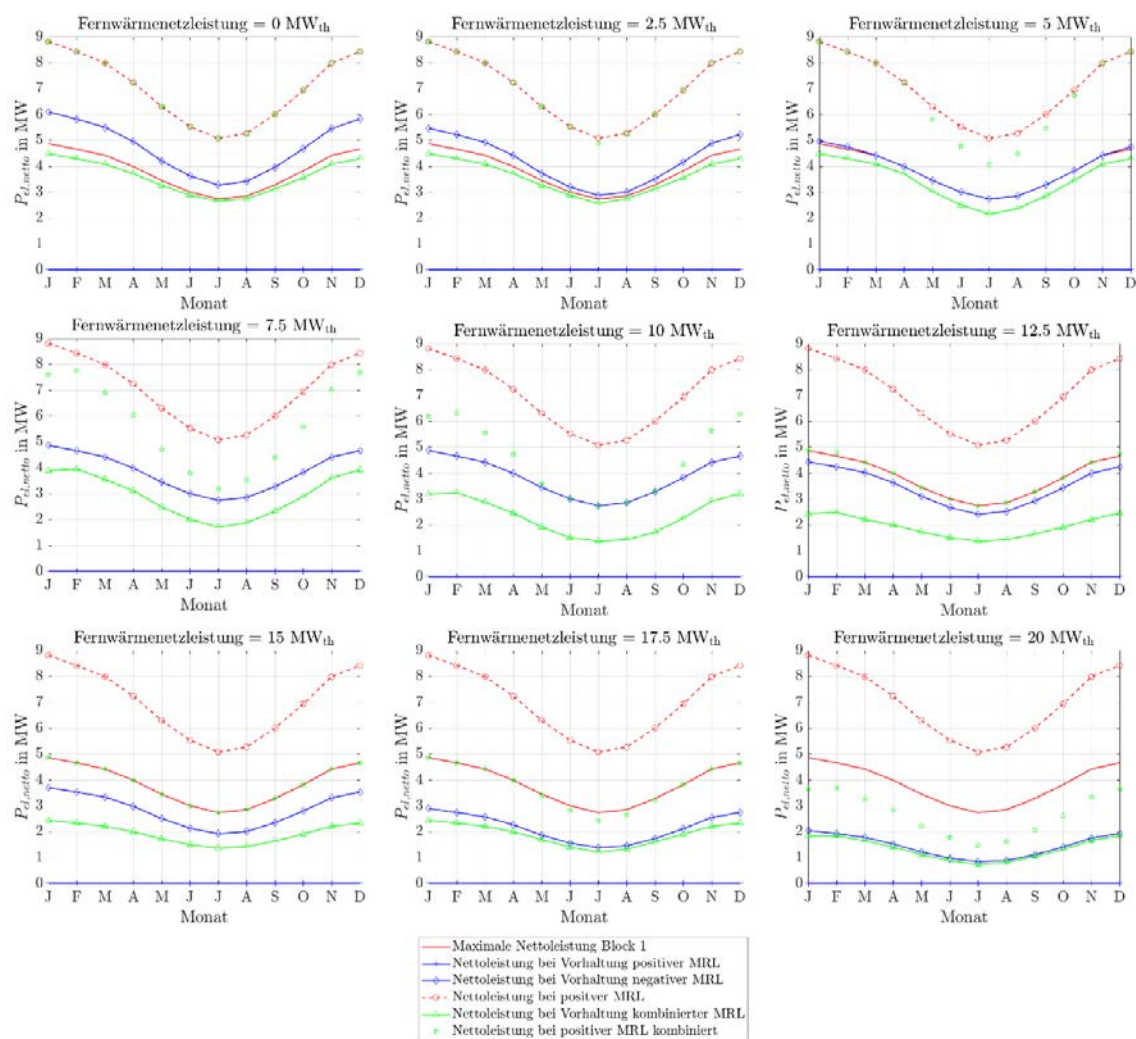
Abbildung 310: Stationäre Minutenregelleistungen des ORC-Referenz-Geothermie-Kraftwerks mit Einsatz eines Heißwasser-Wärmespeichers des Heiz- und Kraftwerks für Fernwärmenetzleistungen von 0 MW th bis 20 MW th bei einer 4h-Zeitscheibe Einspeicherung und zwei aufeinanderfolgenden Zeitscheiben Angebotszeitraum
