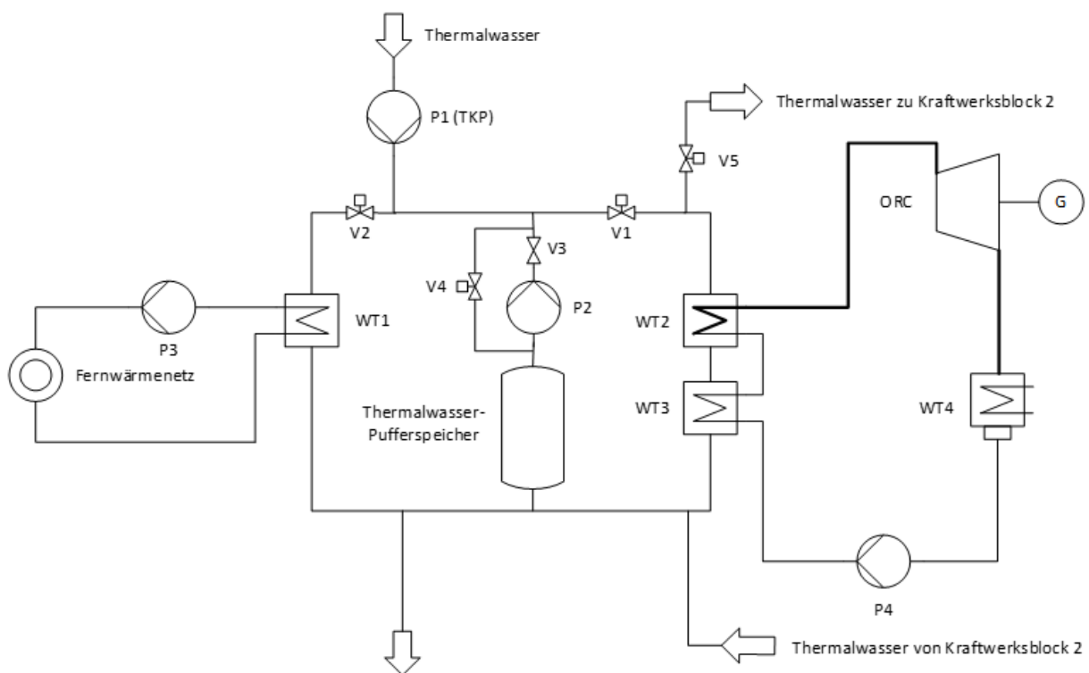
Abbildung 36: Verfahrensfliessbild einer Geothermianlage mit parallel geschaltetem Heiz- und Kraftwerk und einem in das Kraftwerk integrierten Thermalwasser-Wärmespeicher.
