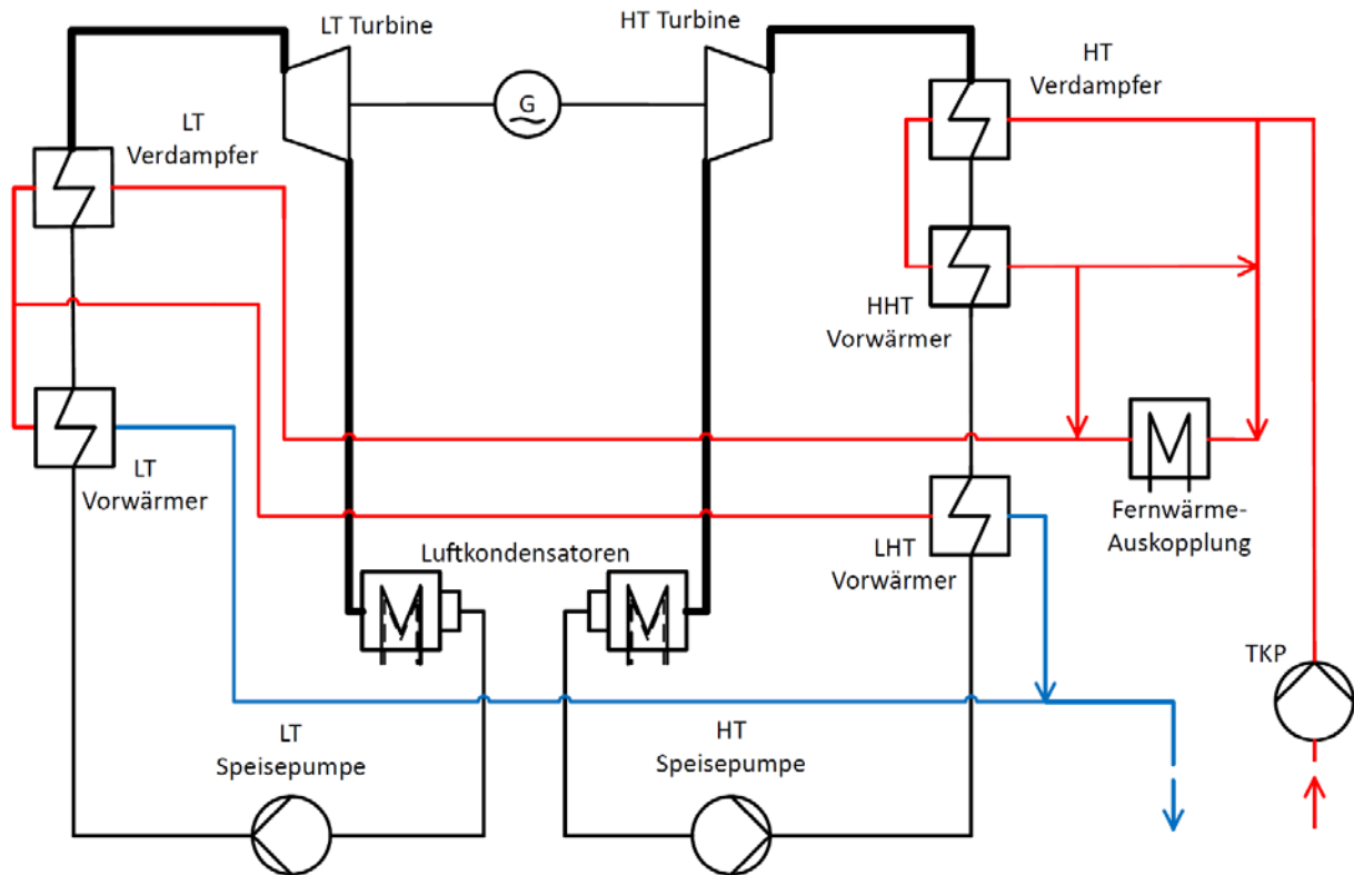
Abbildung 50: Prozessschaltbild des ORC-Zweidruckprozesses [79, vgl. S. 13].
