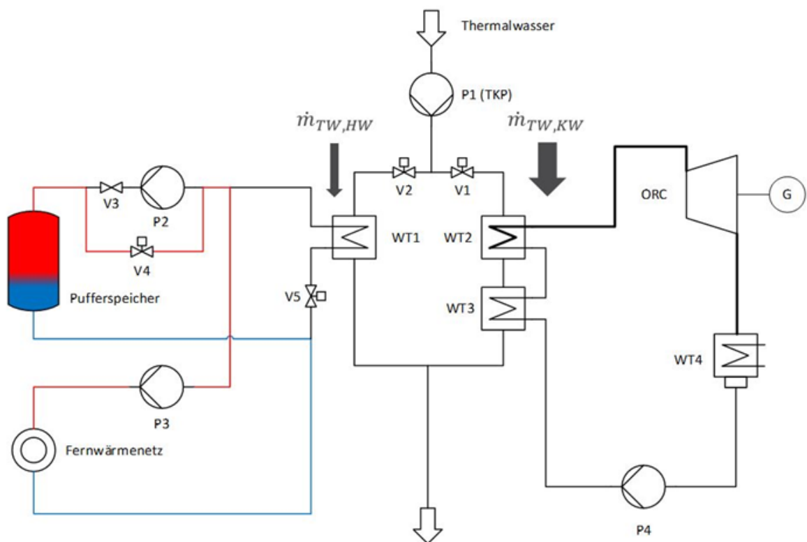
Abbildung 35: Verfahrensfließbild einer Geothermianlage mit parallel geschaltetem Heiz- und Kraftwerk und einem in das Fernwärmenetz integrierten Heißwasser-Wärmespeicher – positive Regelleistungsbereitstellung – Entladevorgang des Heißwasser-Wärmespeichers.
