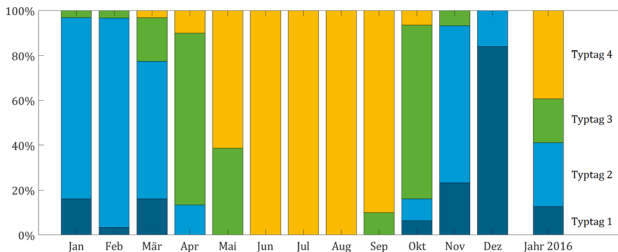
Abbildung 45: Typtage der Wärmeleistung der Geothermie Unterhaching GmbH & Co KG in 2016.
