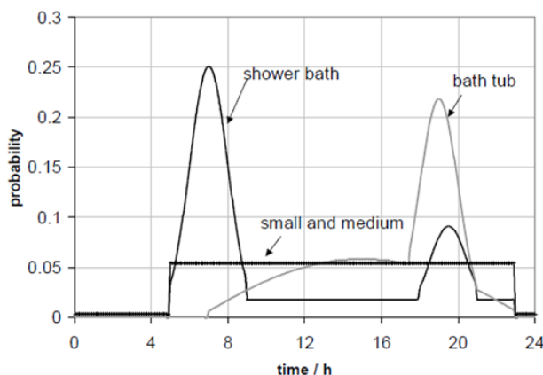
Abbildung 173: Wahrscheinlichkeitsverteilung der Warmwasserverbrauchskategorien im Laufe des Tages [66]. Die Aufttrittswahrscheinlichkeit kleiner und mittlerer Wärmelasten ist gleichmäßig zwischen 5:00 und 23:00 verteilt.
