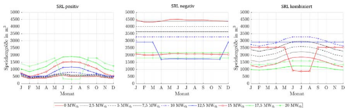
Abbildung 124: Benötigte Speichergrößen bei Angebot von positiver, negativer und kombinierter SRL des ORC-Referenz-Geothermie-Kraftwerks mit Einsatz eines Heißwasser-Wärmespeichers des Heiz- und Kraftwerks für Fernwärmenetzleistungen von 0 MW th bis 20 MW th bei drei 4h-Zeitscheiben Einspeicherung und drei aufeinanderfolgenden Zeitscheiben Angebotszeitraum.
