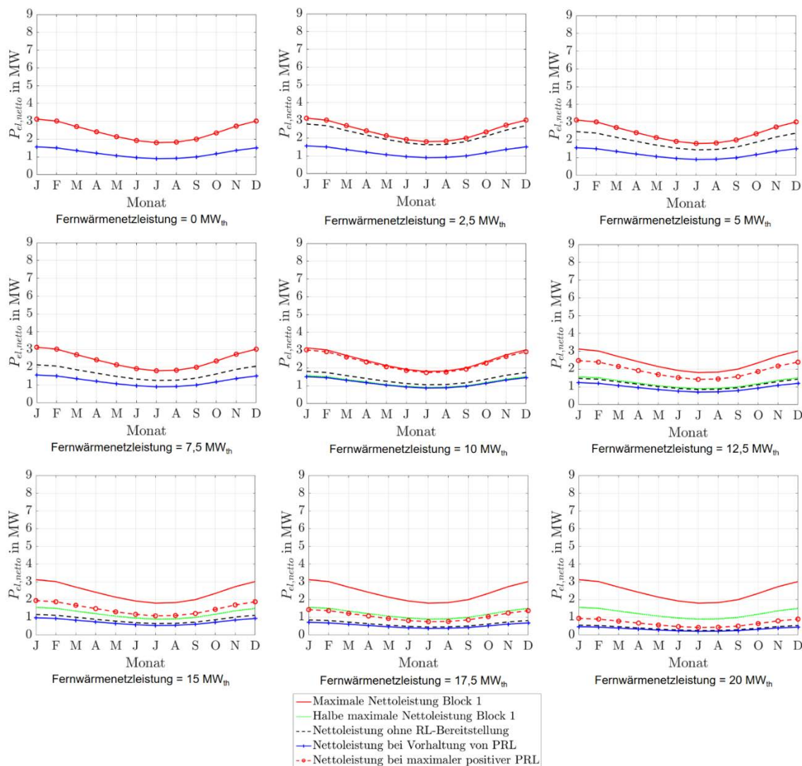
Abbildung 194: Stationäre Primärregelleistungen des Kalina-Referenz-Geothermie-Kraftwerks mit Einsatz eines Heißwasser-Wärmespeichers für Heiz- und Kraftwerk für Fernwärmenetzleistungen von 0 MW th bis 20 MW th .
