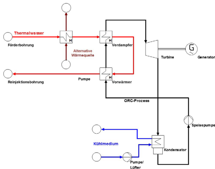
Abbildung 42: ORC-Anlagenkonzepte für Hybridkraftwerke: Vorwärmung des Thermalwassers.
