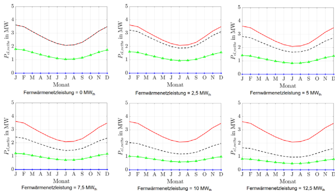
Abbildung 181: Stationäre Sekundär- und Minutenregelleistung des Kalina-Referenz-Geothermie-Kraftwerks im Bestand ohne Flexibilisierungsmaßnahmen für Fernwärmenetzleistungen von 0 MW th bis 20 MW th .
