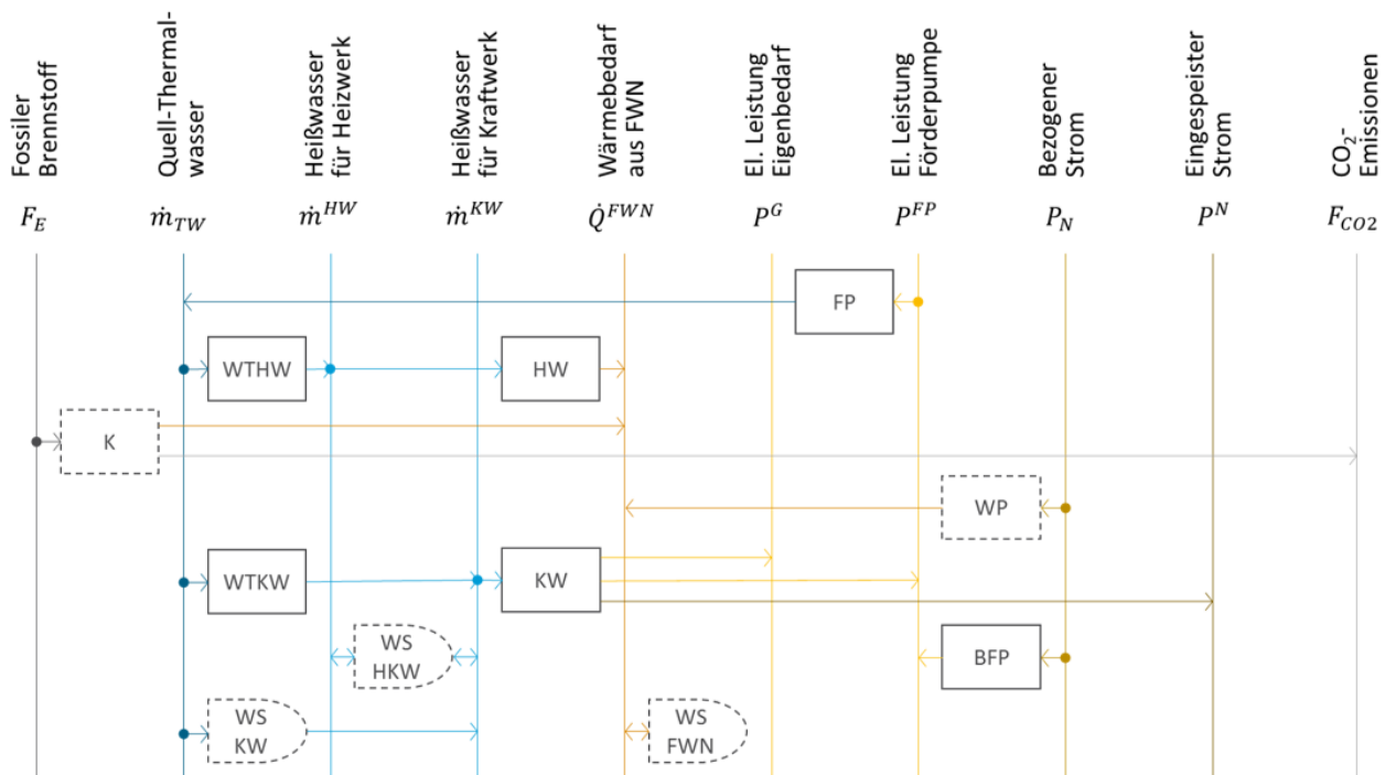
Abbildung 146: Allgemeine Auslegung des Energiesystemmodells mit vertikalen Linien als Energieträger, Kästen als Energiewandlungsprozesse und Halbellipsen als Wärmespeichertechnologien. Flexibilisierungsoptionen sind mit gestricheltem Rand dargestellt.
