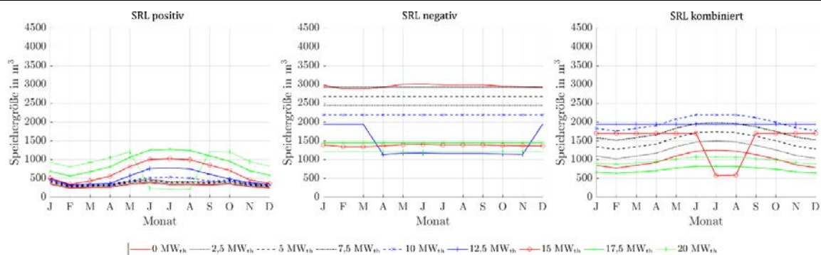
Abbildung 293: Benötigte Speichergrößen bei Angebot von positiver, negativer und kombinierter SRL des ORC-Referenz-Geothermie-Kraftwerks mit Einsatz eines Heißwasser-Wärmespeichers des Heiz- und Kraftwerks für Fernwärmenetzleistungen von 0 MW th bis 20 MW th bei zwei 4h-Zeitscheiben Einspeicherung und zwei aufeinanderfolgenden Zeitscheiben Angebotszeitraum.
