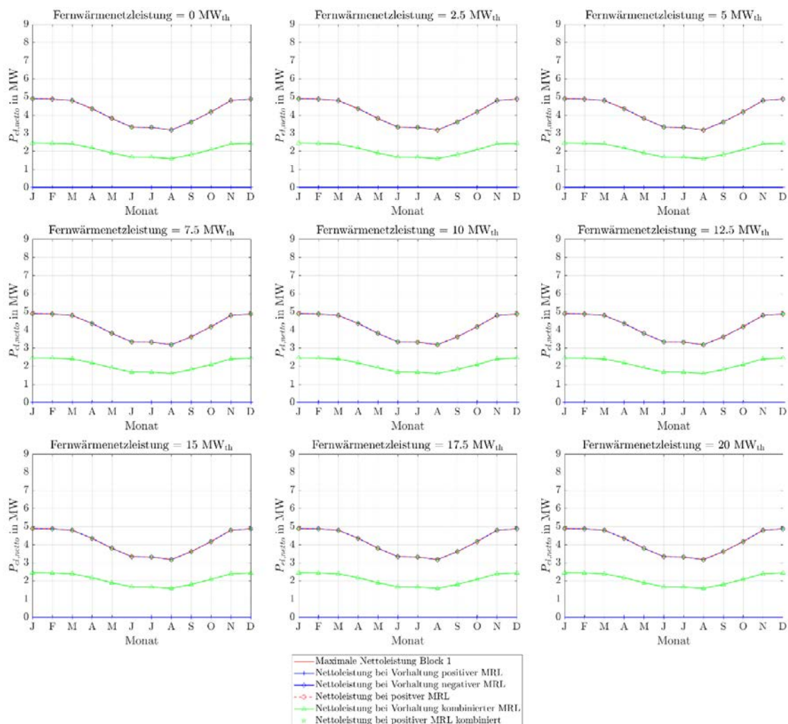
Abbildung 324: Stationäre Minutenregelleistungen des ORC-Referenz-Geothermie-Kraftwerks mit Einsatz eines Heißwasser-Wärmespeichers im Fernwärmenetz für Fernwärmenetzleistungen von 0 MW th bis 20 MW th bei vier 4h-Zeitscheiben Einspeicherung und zwei aufeinanderfolgenden Zeitscheiben Angebotszeitraum.
