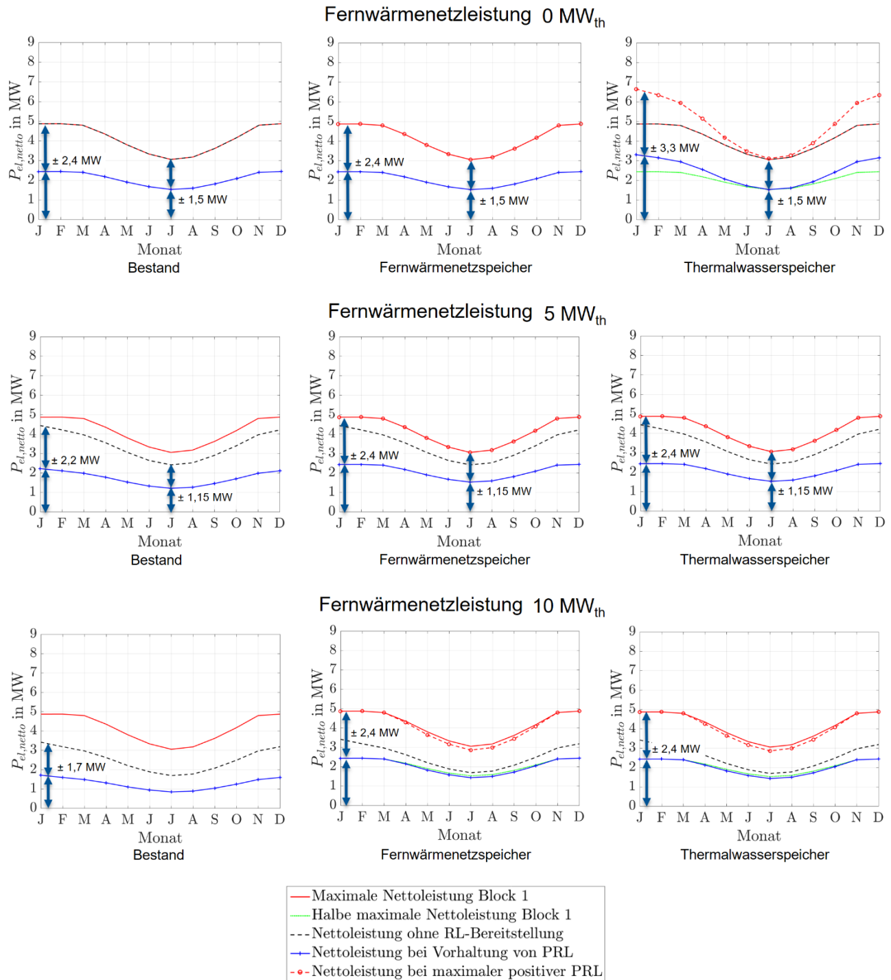
Abbildung 102: Vergleich der bereitstellbaren stationären Primärregelleistungen des ORC-Referenz-Geothermie-Kraftwerks mit den verschiedenen Flexibilisierungsoptionen für Heiz- und Kraftwerk für Fernwärmenetzleistungen von 0 MW th , 5 MW th und 10 MW th .
