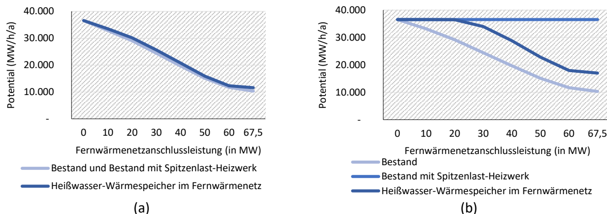
Abbildung 131: Jährliches Potential für negative Sekundärregelleistungserbringung (a) und positive Sekundärregelleistungserbringung (b) für unterschiedliche Flexibilitätsoptionen der ORC-Referenzanlage.
