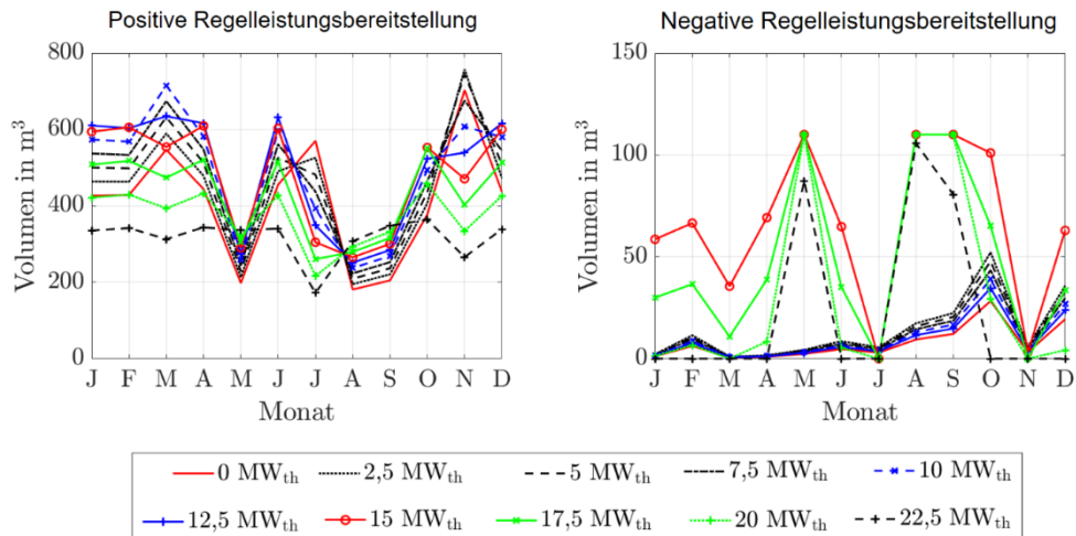
Abbildung 88: Benötigte Speichervolumina für die stationären Minutenregelleistungen des ORC-Referenz-Geothermie-Kraftwerks mit Einsatz eines Thermalwasserspeichers für Fernwärmenetzleistungen von 0 MW th bis 22,5 MW th .
