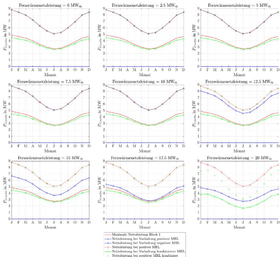
Abbildung 282: Stationäre Minutenregelleistungen des ORC-Referenz-Geothermie-Kraftwerks mit Einsatz eines Heißwasser-Wärmespeichers des Heiz- und Kraftwerks für Fernwärmenetzleistungen von 0 MW th bis 20 MW th bei zwei 4h-Zeitscheiben Einspeicherung und einer Zeitscheibe Angebotszeitraum.
