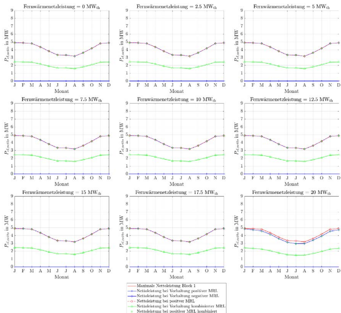
Abbildung 294: Stationäre Sekundärregelleistungen des ORC-Referenz-Geothermie-Kraftwerks mit Einsatz eines Heißwasser-Wärmespeichers im Fernwärmenetz für Fernwärmenetzleistungen von 0 MW th bis 20 MW th bei drei 4h-Zeitscheiben Einspeicherung und zwei aufeinanderfolgenden Zeitscheiben Angebotszeitraum.
