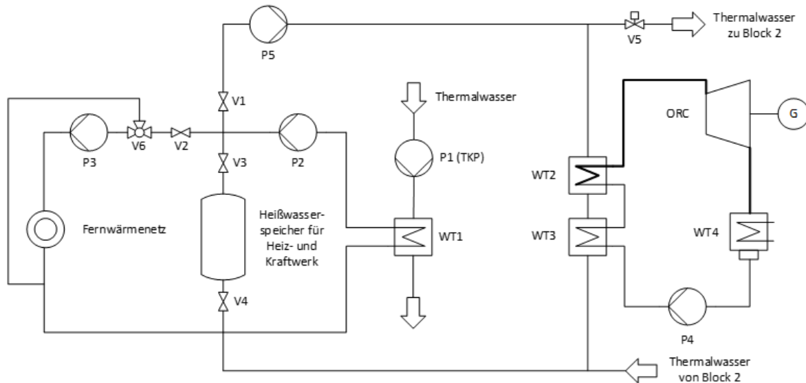
Abbildung 39: Verfahrensfließbild mit parallel geschaltetem Heiz- und Kraftwerk und einem in die Geothermieanlage integrierten Heißwasser-Wärmespeicher für das Kraftwerk und das Heizwerk.
