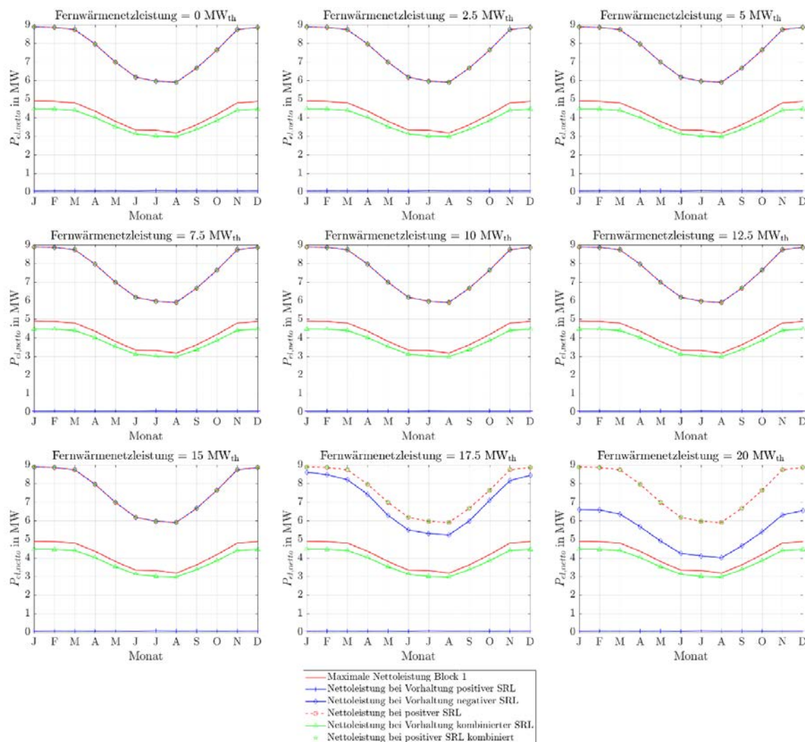
Abbildung 109: Stationäre Sekundärregelleistungen des ORC-Referenz-Geothermie-Kraftwerks mit Einsatz eines Thermalwasserspeichers für Fernwärmenetzleistungen von 0 MW th bis 20 MW th bei drei 4h-Zeitscheiben Einspeicherung und einer Zeitscheibe Angebotszeitraum.
