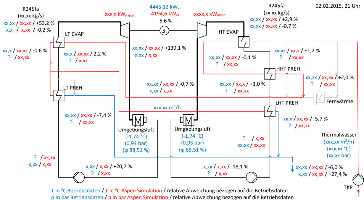
Abbildung 178: Validierung des Simulationsmodells des ORC-Referenz-Geothermie-Kraftwerks im Februar.
