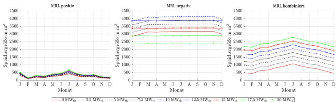
Abbildung 327: Benötigte Speichergrößen bei Angebot von positiver, negativer und kombinierter MRL des ORC-Referenz-Geothermie-Kraftwerks mit Einsatz eines Thermalwasserspeichers im Kraftwerk für Fernwärmenetzleistungen von 0 MW th bis 20 MW th bei vier 4h-Zeitscheiben Einspeicherung und zwei aufeinanderfolgenden Zeitscheiben Angebotszeitraum.
