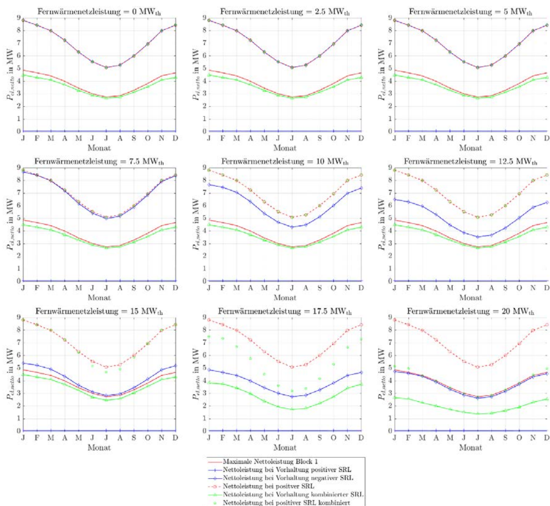
Abbildung 298: Stationäre Sekundärregelleistungen des ORC-Referenz-Geothermie-Kraftwerks mit Einsatz eines Heißwasser-Wärmespeichers des Heiz- und Kraftwerks für Fernwärmenetzleistungen von 0 MW th bis 20 MW th bei drei 4h-Zeitscheiben Einspeicherung und zwei aufeinanderfolgenden Zeitscheiben Angebotszeitraum.
