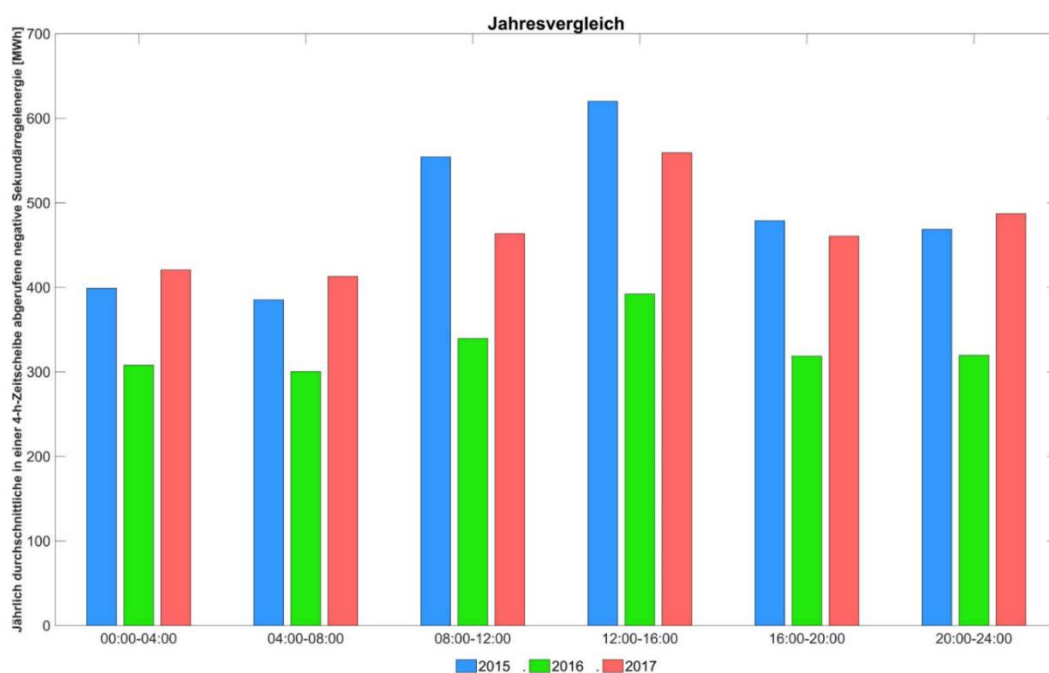
Abbildung 229: Jährlich durchschnittlich in einer 4h-Zeitscheibe abgerufene negative Sekundärregelenergie.
