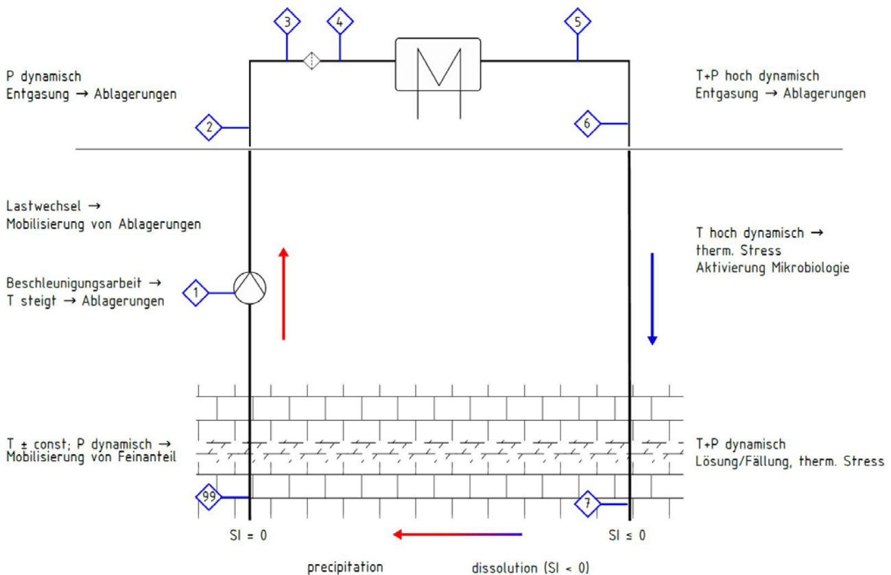
Abbildung 11: Konzeptmodell der geothermischen Anlage mit Simulationspunkten.
