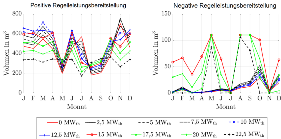
Abbildung 96: Benötigte Speichervolumina für die stationären Minutenregelleistungen des ORC-Referenz-Geothermie-Kraftwerks mit Einsatz eines Heißwasser-Wärmespeichers für Fernwärmenetzleistungen von 0 MW th bis 22,5 MW th .
