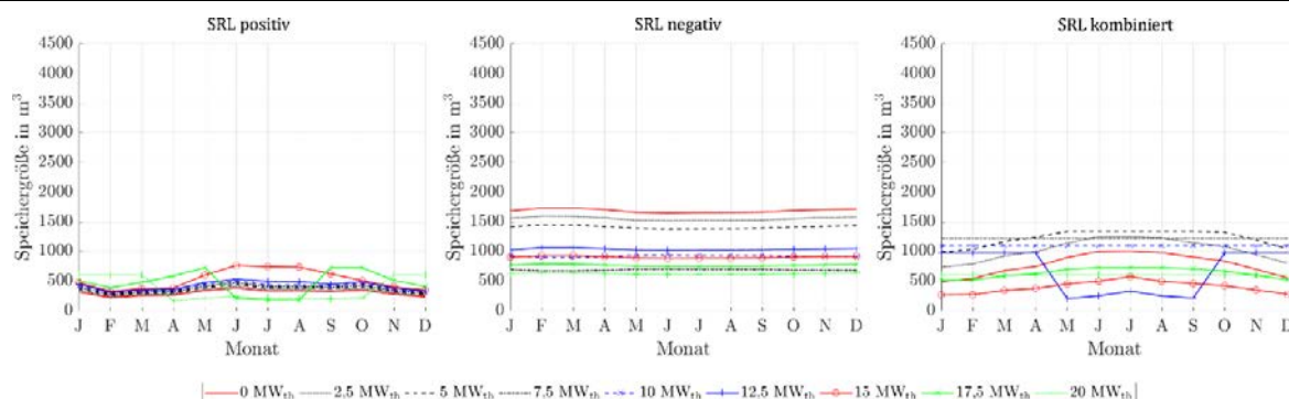
Abbildung 116: Benötigte Speichergrößen bei Angebot von positiver, negativer und kombinierter SRL des ORC-Referenz-Geothermie-Kraftwerks mit Einsatz eines Thermalwasserspeichers im Kraftwerk für Fernwärmenetzleistungen von 0 MW th bis 20 MW th bei einer 4h-Zeitscheibe Einspeicherung und zwei aufeinanderfolgenden Zeitscheiben Angebotszeitraum.
