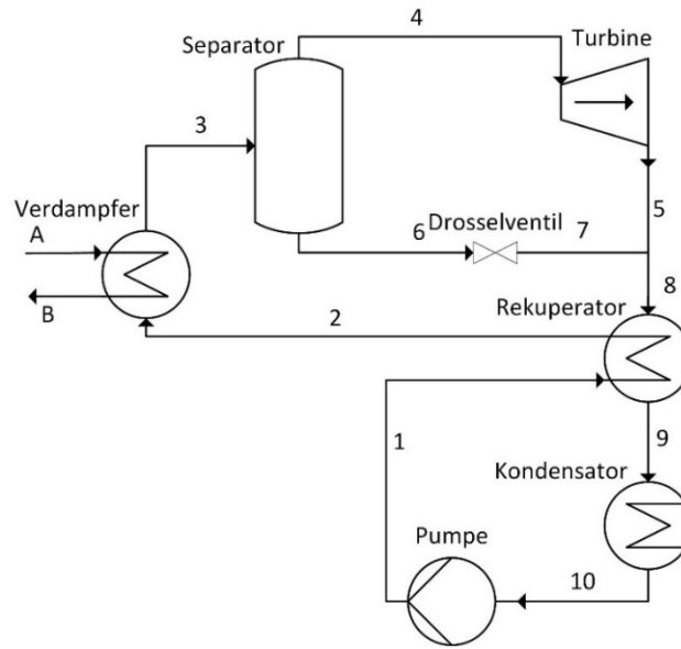
Abbildung 58: Fließbild des Simulationsmodells des Kalina-Referenz-Geothermie-Kraftwerks.
