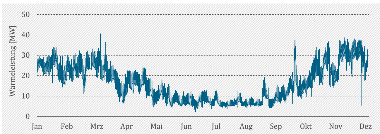
Abbildung 159: Wärmeleistung aus dem Fernwärmenetz der Geothermie-Anlage Unterhaching.
