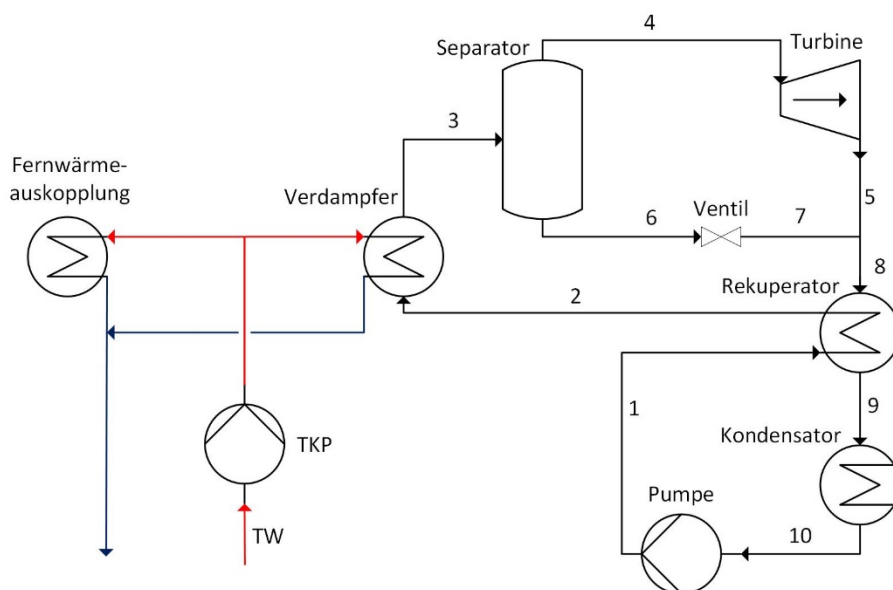
Abbildung 54: Prozessschaltbild des Kalina-Prozesses.
