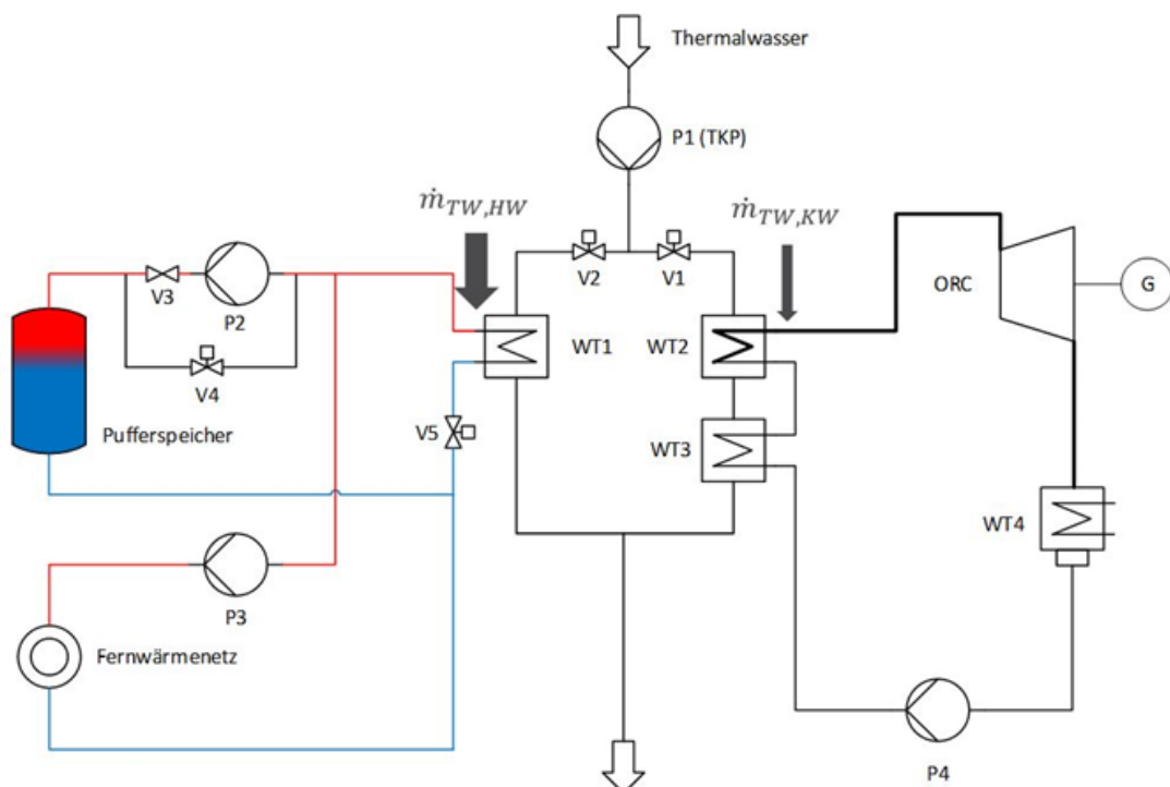
Abbildung 34: Verfahrensfließbild einer Geothermieranlage mit parallel geschaltetem Heiz- und Kraftwerk und einem in das Fernwärmenetz integrierten Heißwasser-Wärmespeicher – negative Regelleistungsbereitstellung – Ladevorgang des Heißwasser-Wärmespeichers.
