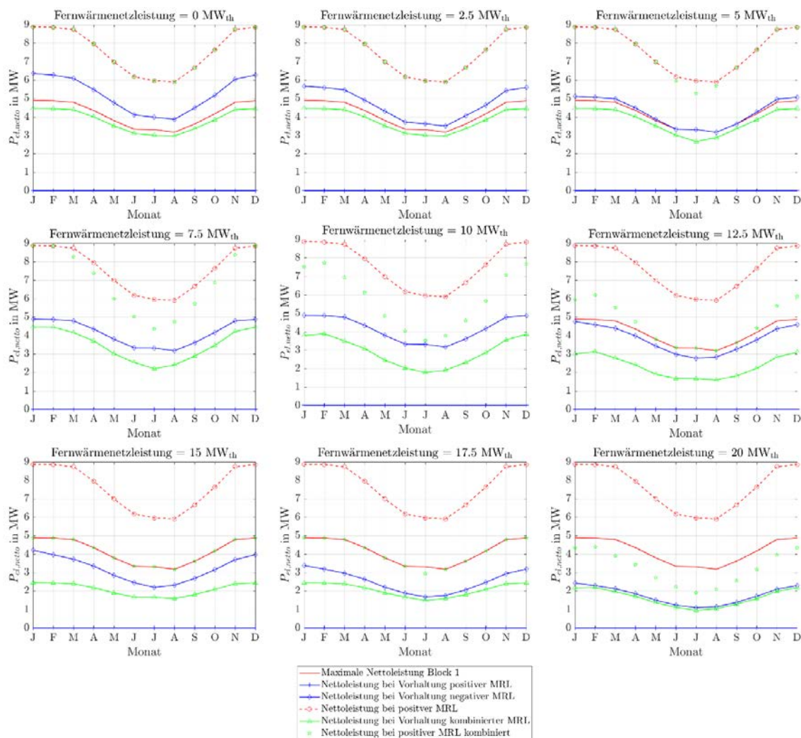
Abbildung 308: Stationäre Minutenregelleistungen des ORC-Referenz-Geothermie-Kraftwerks mit Einsatz eines Thermalwasserspeichers für Fernwärmenetzleistungen von 0 MW th bis 20 MW th bei einer 4h-Zeitscheibe Einspeicherung und zwei aufeinanderfolgenden Zeitscheiben Angebotszeitraum.
