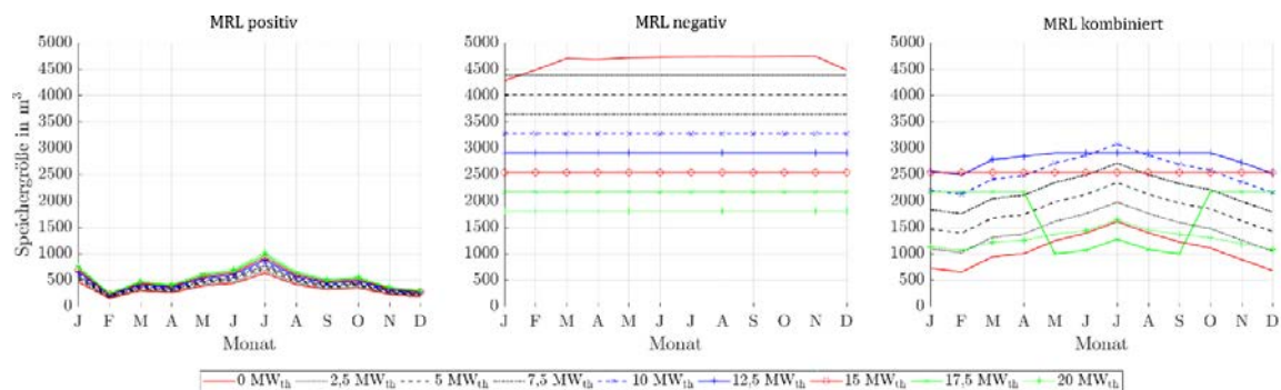
Abbildung 333: Benötigte Speichergrößen bei Angebot von positiver, negativer und kombinierter MRL des ORC-Referenz-Geothermie-Kraftwerks mit Einsatz eines Thermalwasserspeichers im Kraftwerk für Fernwärmenetzleistungen von 0 MW th bis 20 MW th bei drei 4h-Zeitscheiben Einspeicherung und drei aufeinanderfolgenden Zeitscheiben Angebotszeitraum.
