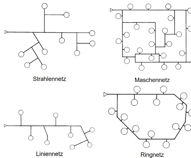
Abbildung 30: Fernwärmenetztopologien [49, S. 25 f.].
