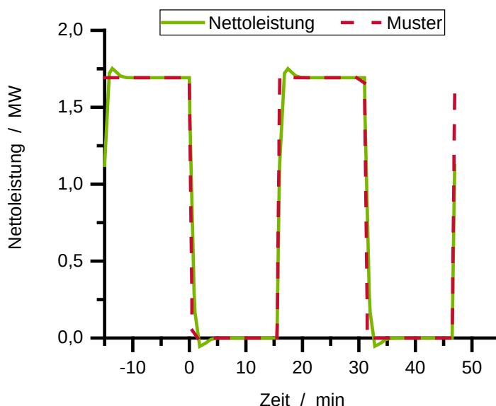
Abbildung 68: Lastprofil der dynamischen Simulation im Vergleich zum Verlauf des Musterprotokolls für die Primärregelleistung bei Vorhaltung symmetrisch negativer Regelleistung (Betrachtungsmonat Juli; Fernwärmeleistung 10 MW).
