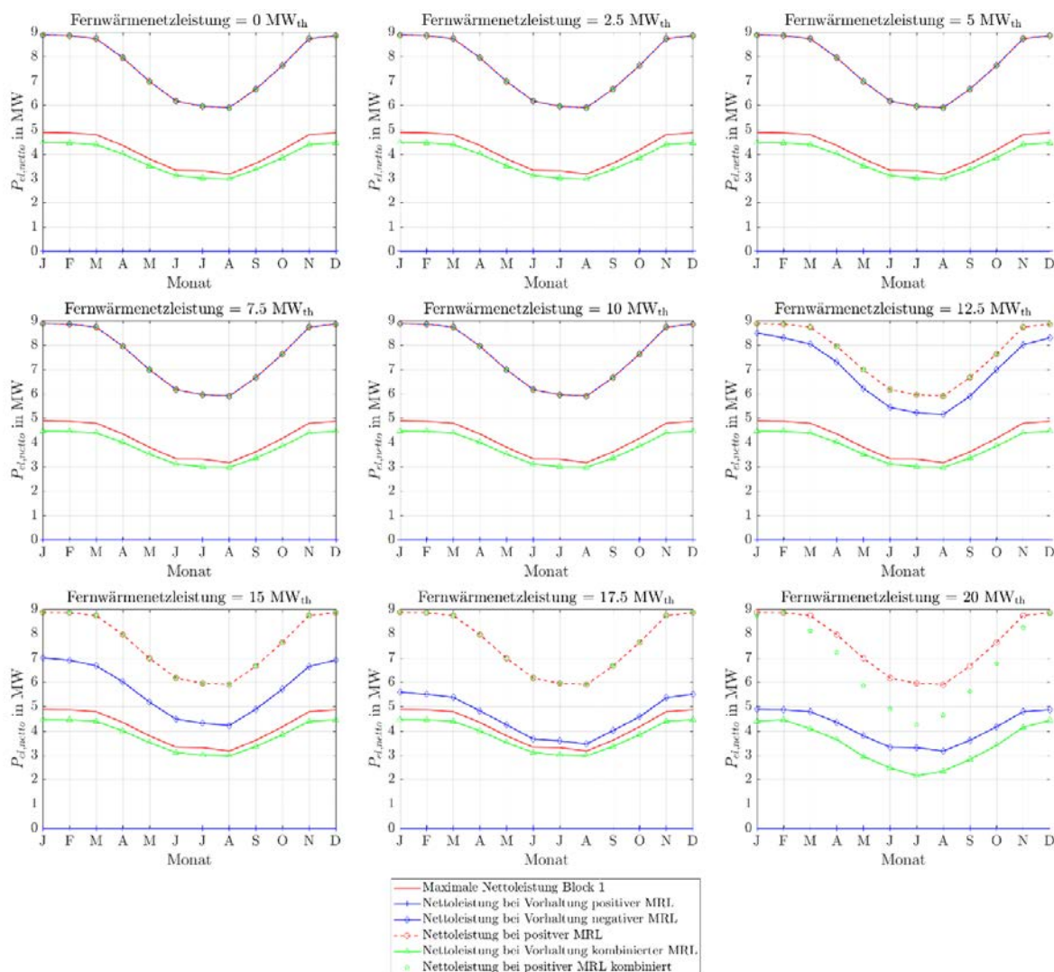
Abbildung 280: Stationäre Minutenregelleistungen des ORC-Referenz-Geothermie-Kraftwerks mit Einsatz eines Thermalwasserspeichers für Fernwärmenetzleistungen von 0 MW th bis 20 MW th bei zwei 4h-Zeitscheiben Einspeicherung und einer Zeitscheibe Angebotszeitraum.
