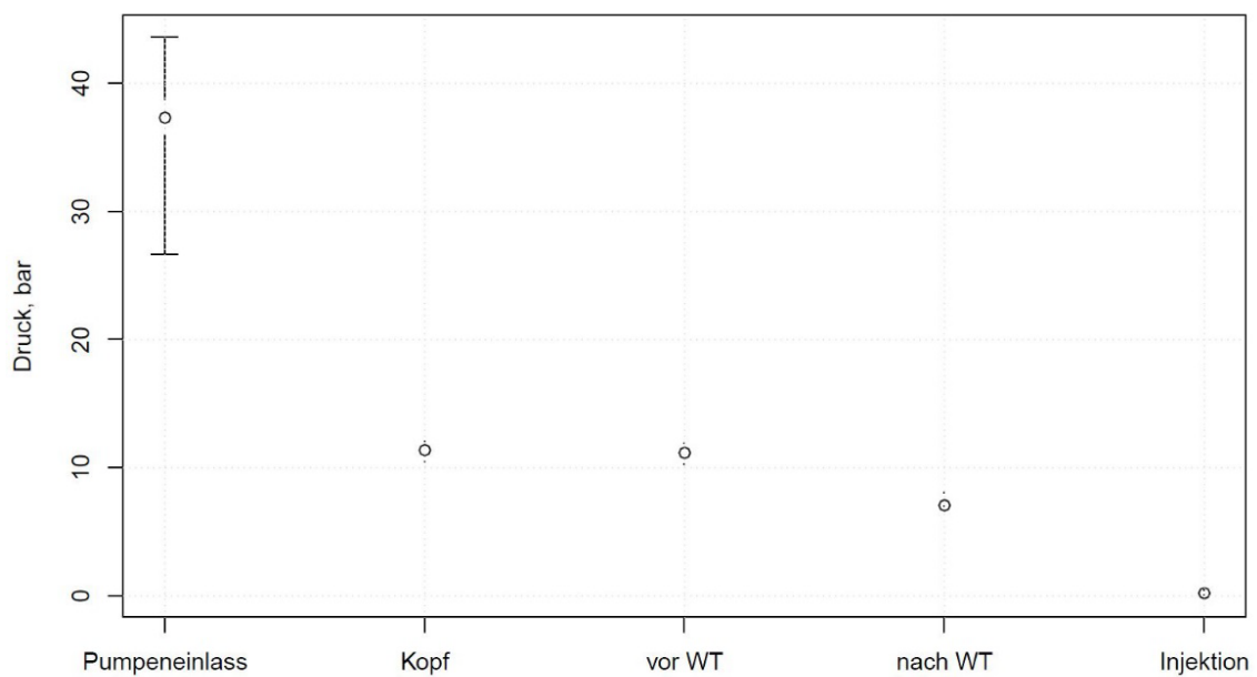
Abbildung 18: Druck entlang des Thermalwasserkreislaufs.
