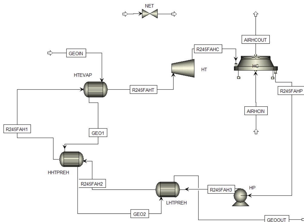
Abbildung 81: Flowsheet des Simulationsmodells des HT-Arbeitskreises des ORC-Referenz-Geothermiekraftwerks in Aspen Plus.
