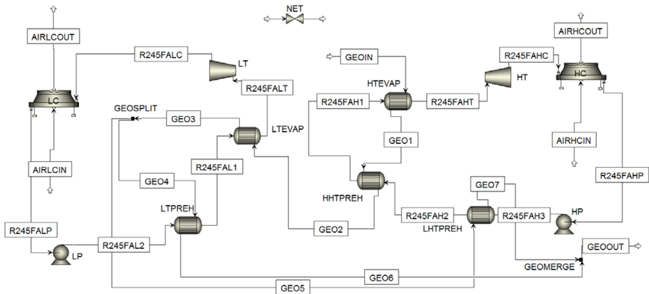
Abbildung 55: Flowsheet des Simulationsmodells des ORC-Referenz-Geothermie-Kraftwerks in Aspen Plus.
