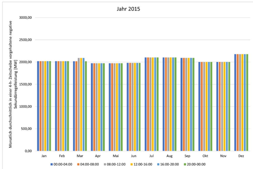
Abbildung 203: Monatlich durchschnittlich in einer 4h-Zeitscheibe vorgehaltene negative Sekundärregelleistung 2015.
