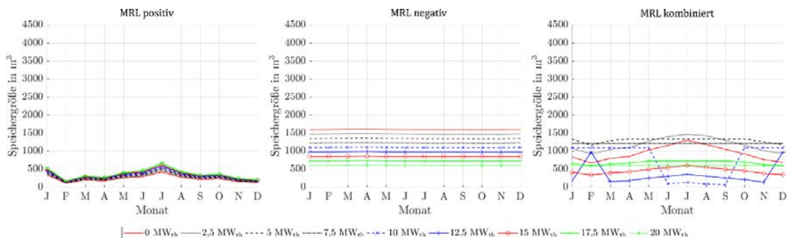
Abbildung 311: Benötigte Speichergrößen bei Angebot von positiver, negativer und kombinierter MRL des ORC-Referenz-Geothermie-Kraftwerks mit Einsatz eines Heißwasser-Wärmespeichers des Heiz- und Kraftwerks für Fernwärmenetzleistungen von 0 MW th bis 20 MW th bei einer 4h-Zeitscheibe Einspeicherung und zwei aufeinanderfolgenden Zeitscheiben Angebotszeitraum.
