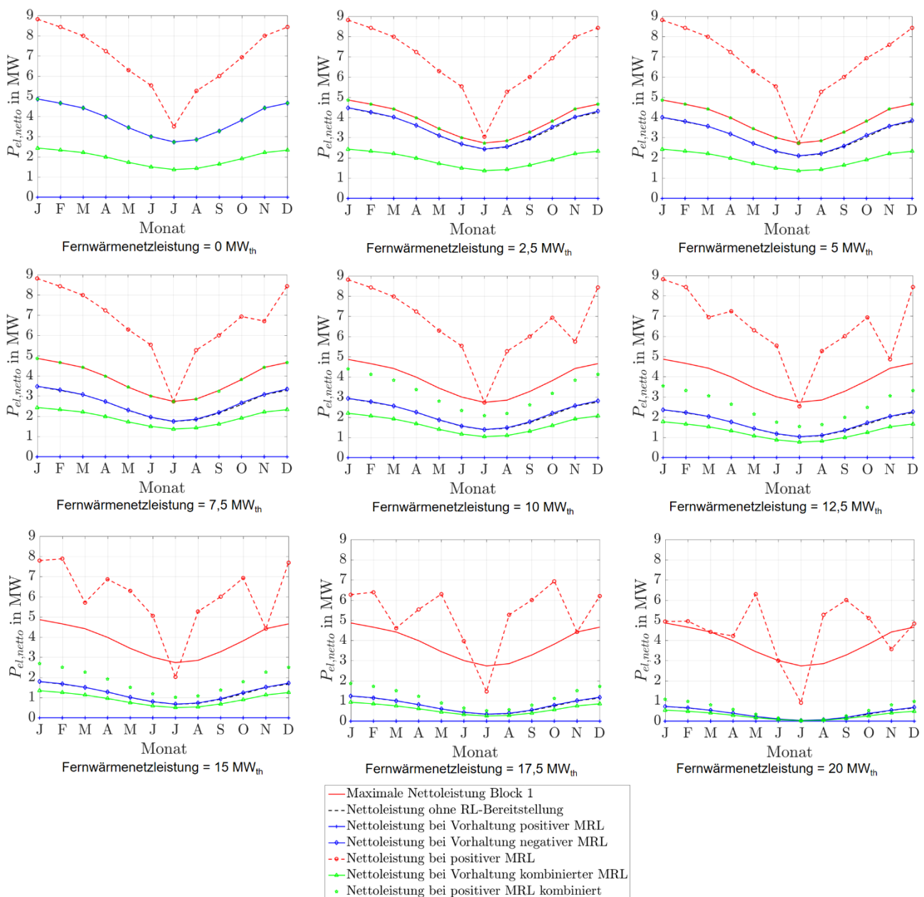
Abbildung 95: Stationäre Minutenregelleistungen des ORC-Referenz-Geothermie-Kraftwerks mit Einsatz eines Heißwasser-Wärmespeichers für Heiz- und Kraftwerk für Fernwärmenetzleistungen von 0 MW th bis 20 MW th .
