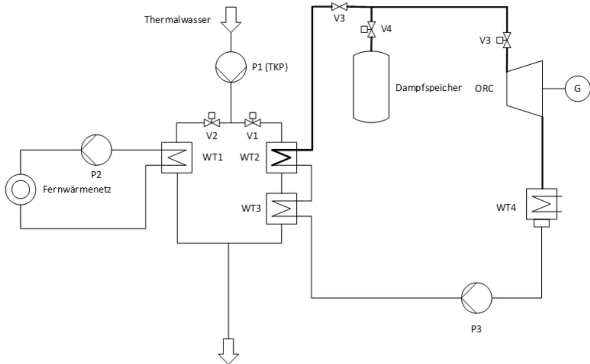
Abbildung 40: Verfahrensfließbild einer Geothermieranlage mit parallel geschaltetem Heiz- und Kraftwerk und einem in das Kraftwerk integrierten Dampfspeicher.
