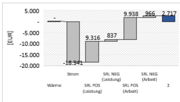
(c) Heißwasser-Wärmespeicher
