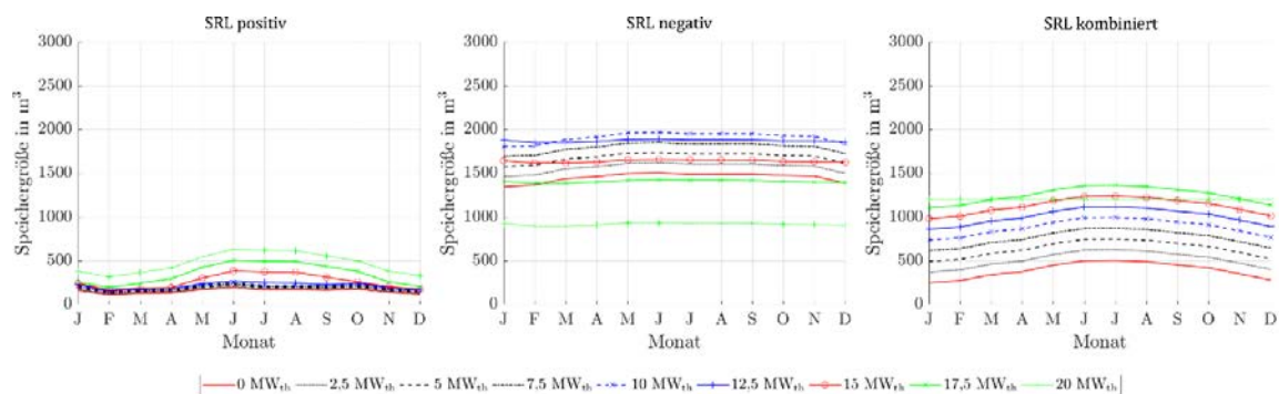
Abbildung 269: Benötigte Speichergrößen bei Angebot von positiver, negativer und kombinierter SRL des ORC-Referenz-Geothermie-Kraftwerks mit Einsatz eines Thermalwasserspeichers im Kraftwerk für Fernwärmenetzleistungen von 0 MW th bis 20 MW th bei zwei 4h-Zeitscheiben Einspeicherung und einer Zeitscheibe Angebotszeitraum.
