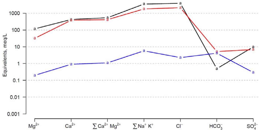
Abbildung 10: Schoeller-Diagramm für die in der Simulation verwendeten Wässer aus den drei Regionen (Molassebecken: blau, Oberrheingraben: rot, Norddeutsches Becken: schwarz).
