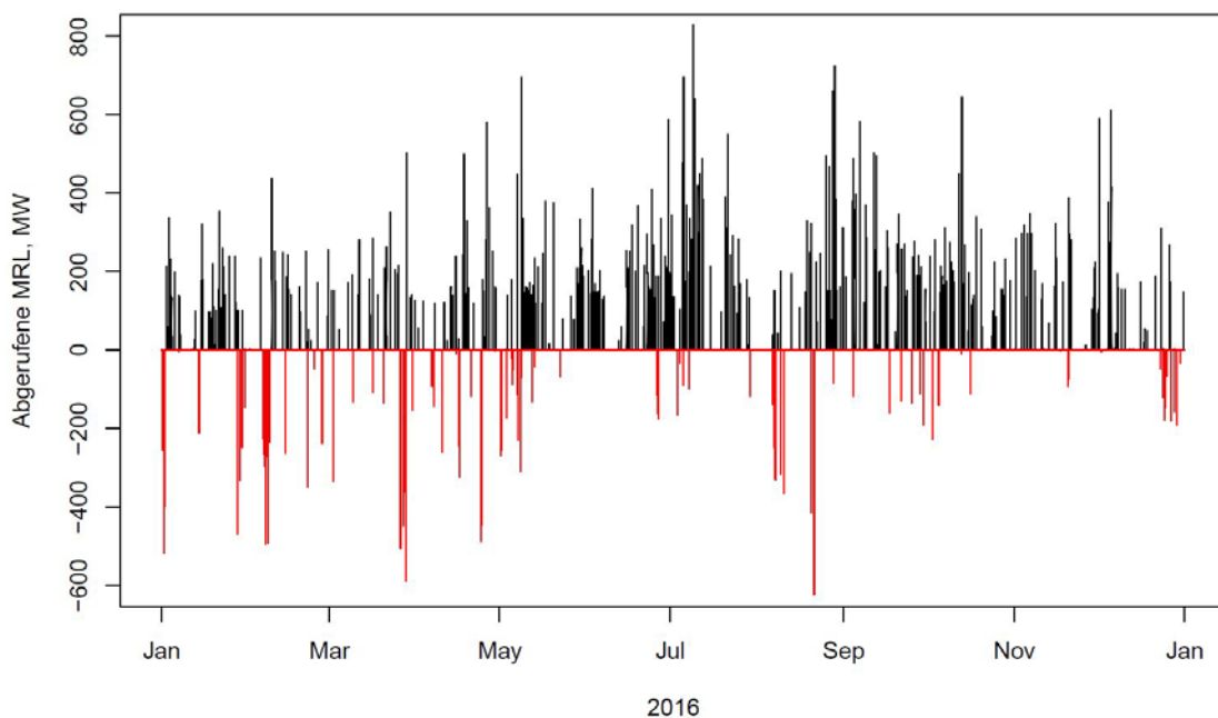
Abbildung 13: Abgerufenene Minutenregelleistung im Netz des Betreibers TenneT im Jahr 2016.
