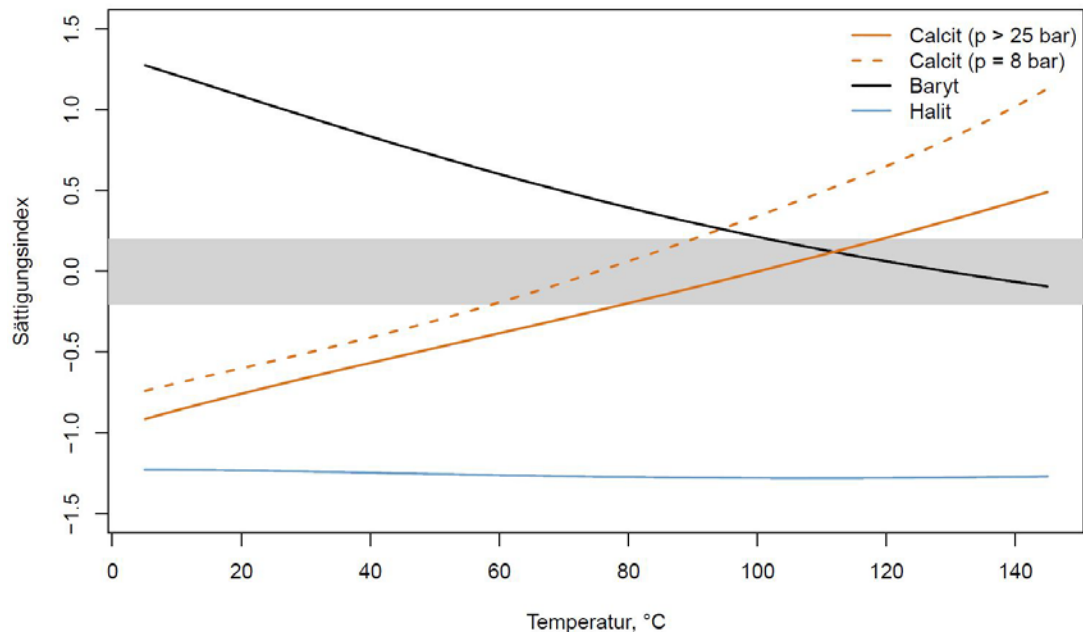
Abbildung 24: Sättigungsindex für Baryt, Halit und Calcit für eine Anlage im Oberrheingraben als Funktion der Temperatur.
