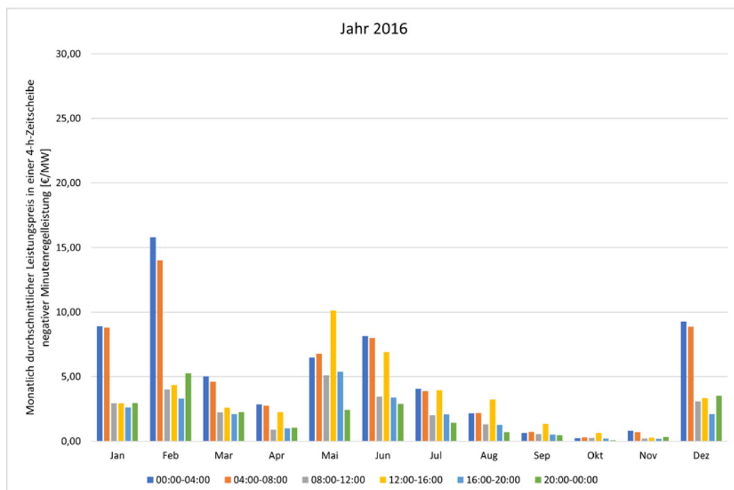
Abbildung 242: Monatlich durchschnittlicher Leistungspreis in einer 4h-Zeitscheibe negativer Minutenregelleistung 2016.
