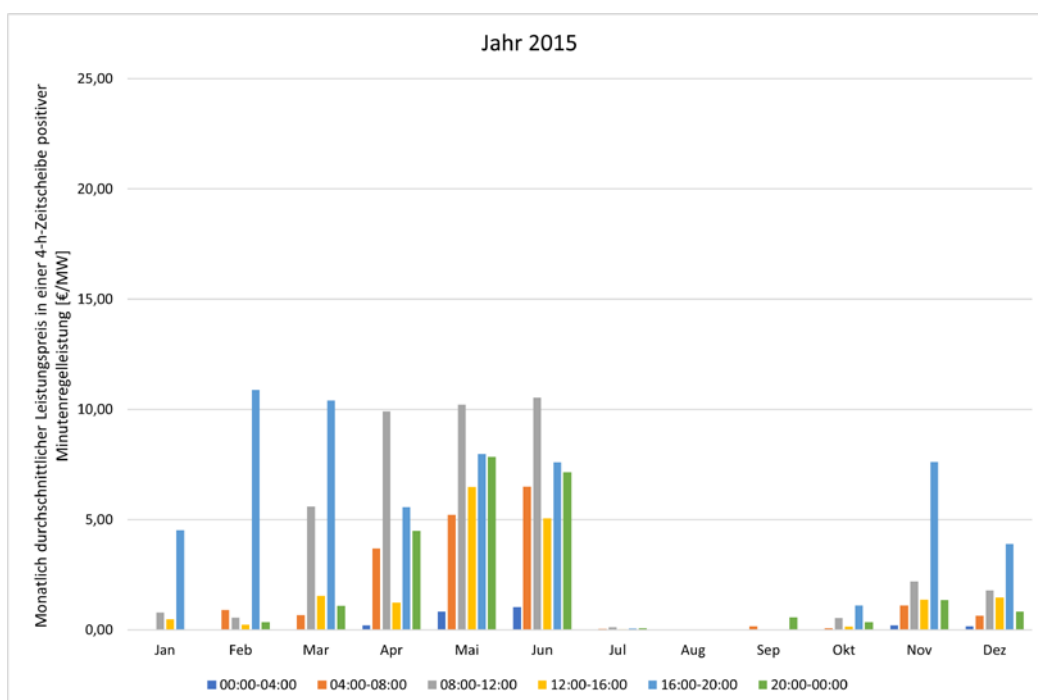
Abbildung 238: Monatlich durchschnittlicher Leistungspreis in einer 4h-Zeitscheibe positiver Minutenregelleistung 2015.
