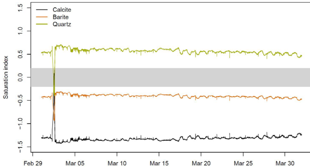
Abbildung 28: Sättigungsindizes für Kalzit, Baryt und Quarz nach dem Wärmetauscher im laufenden Betrieb einer Anlage im Bayerischen Molassebecken.
