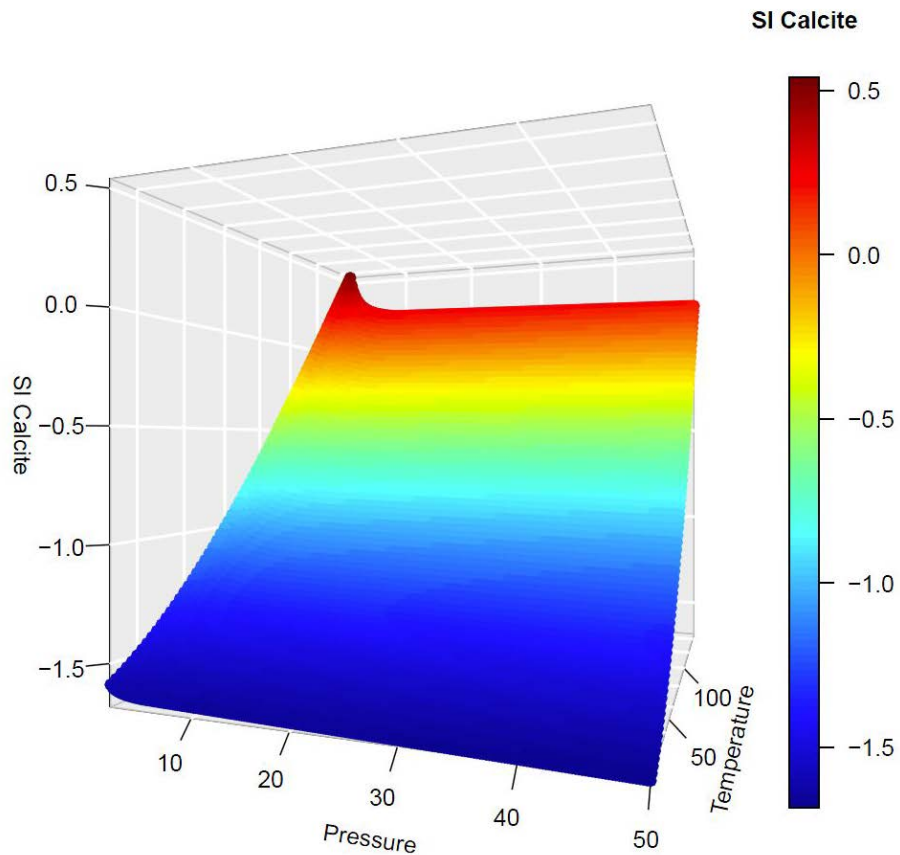
Abbildung 22: Sättigungsindex von Kalzit (Calcite) als Funktion von Druck und Temperatur für eine Anlage im Bayerischen Molassebecken.
