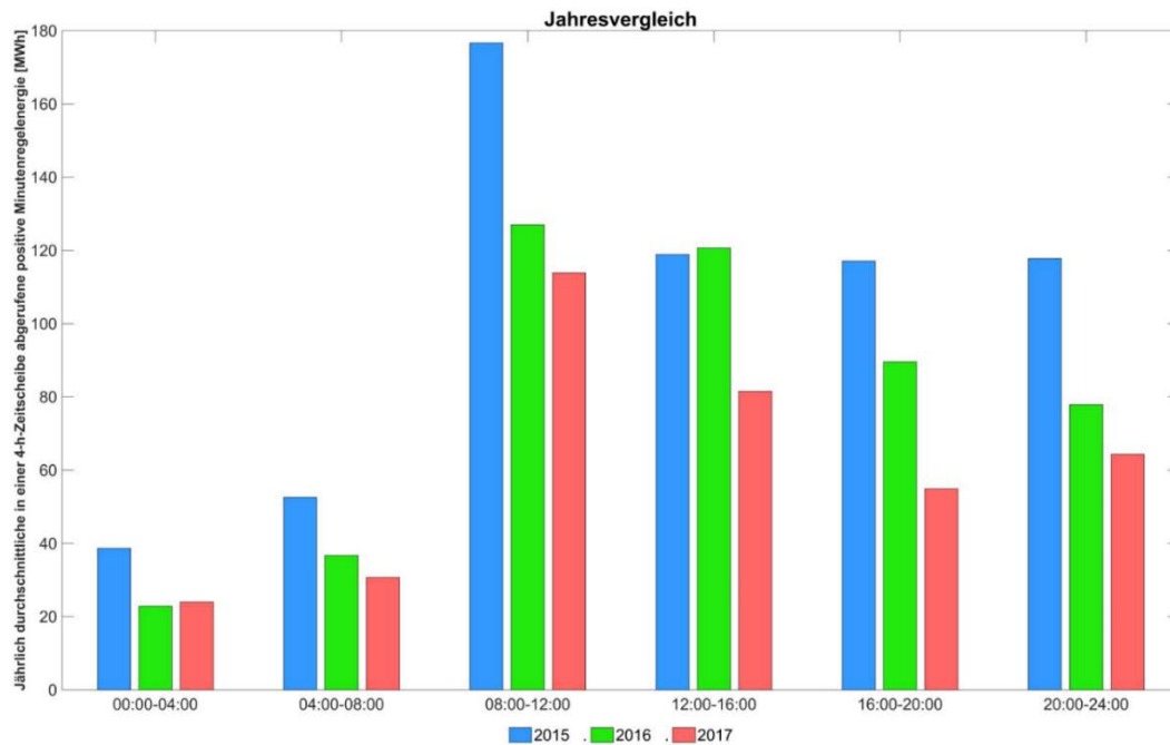
Abbildung 260: Jährlich durchschnittlich in einer 4h-Zeitscheibe abgerufene positive Minutenregelenergie.
