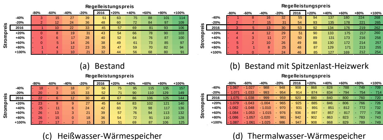
Abbildung 144: Sensitivität der Mehrgewinne (p.a.) in 10^3 EUR im wirtschaftlich optimalen Betrieb bei Marktpreisvergütung und Fernwärmenetz-Anschlussleistung von 67,5 MW.
