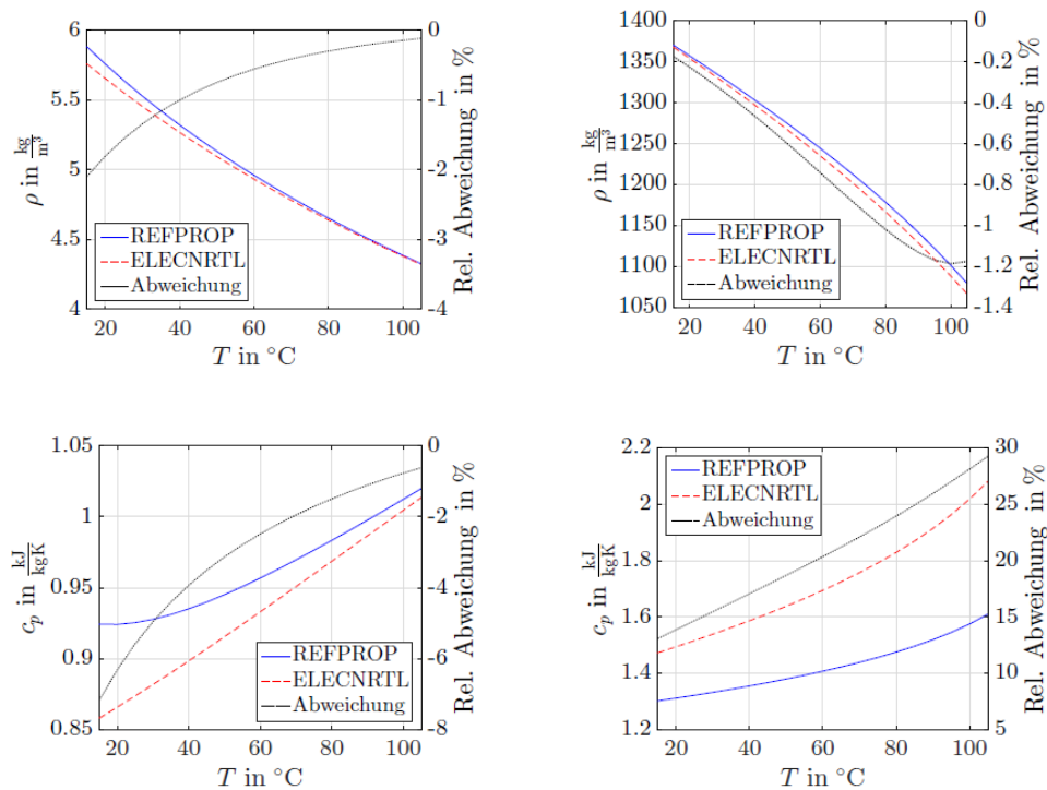
Abbildung 177: Vergleich der Stoffdatenmethoden REFPROP und ELECRTL anhand der Dichte (oben) und der spezifischen Wärmekapazität (unten) von R245fa bei 1 bar (gasförmig, links) und bei 20 bar (flüssig, rechts). Relative Abweichung ELECRTL von REFPROP.
