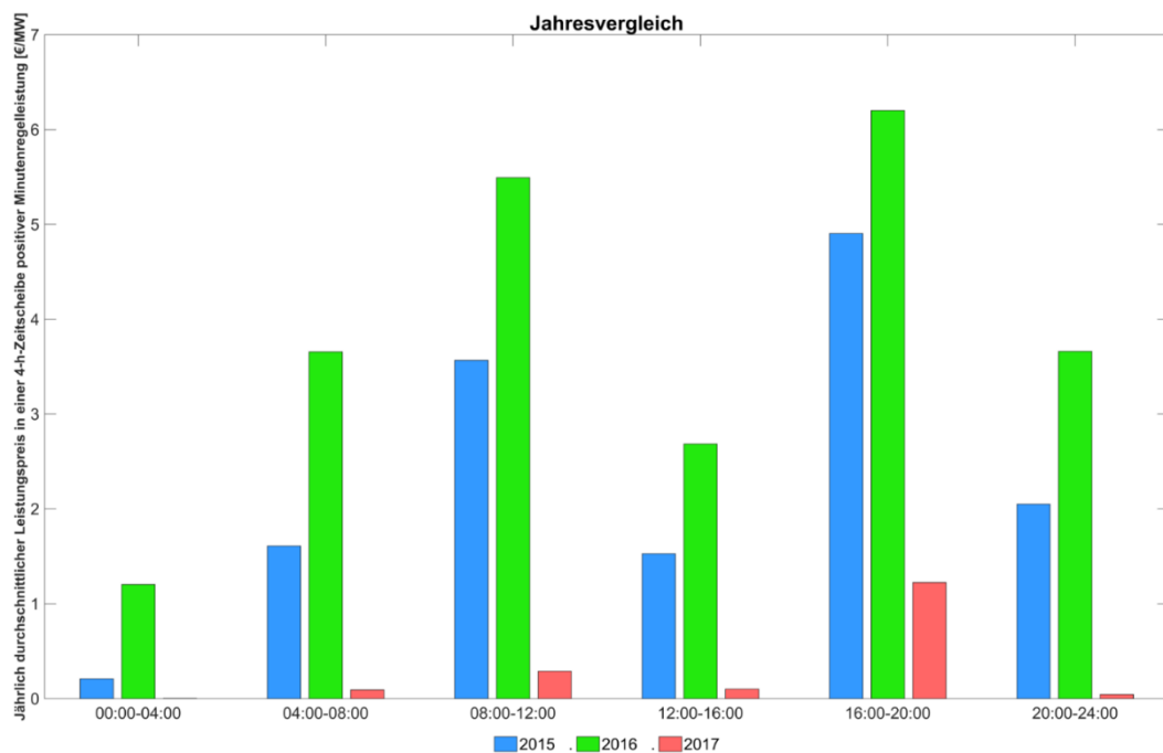
Abbildung 258: Jährlich durchschnittlicher Leistungspreis in einer 4h-Zeitscheibe positiver Minutenregelleistung.
