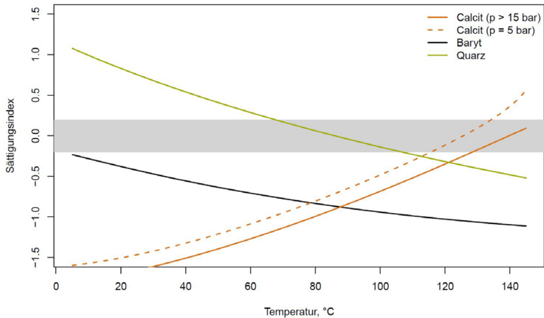
Abbildung 21: Sättigungsindex für Kalzit und Baryt als Funktion der Temperatur an einem Geothermiekraftwerk im Bayerischen Molassebecken.
