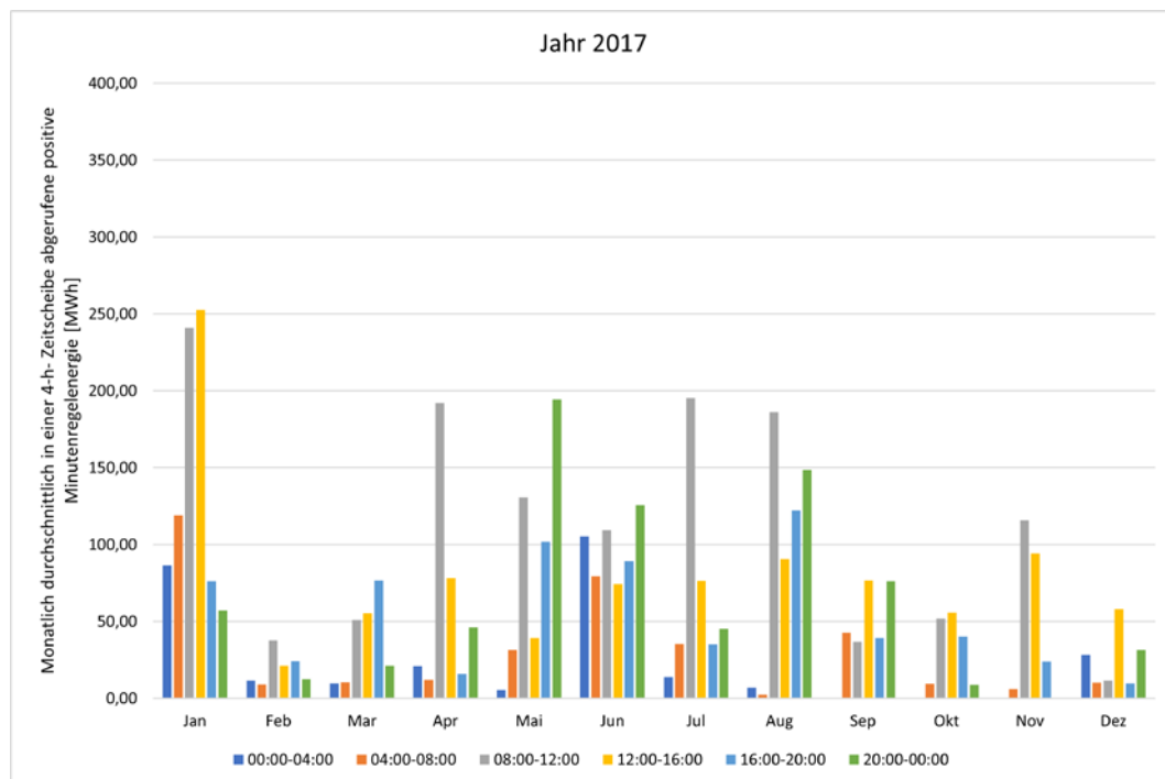
Abbildung 246: Monatlich durchschnittlich in einer 4h-Zeitscheibe abgerufene positive Minutenregelenergie 2017.
