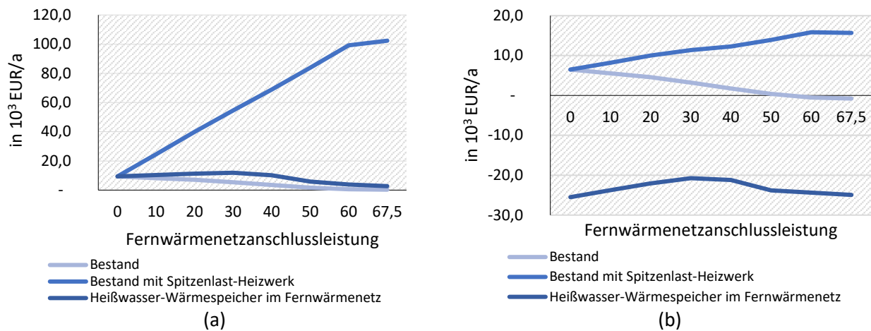
Abbildung 138: Abhängigkeit der (a) Mehrerlöse (p.a.) und (b) Zusatzgewinne (p.a.) von der Fernwärmenetzanschlussleistung (im optimalen Betrieb für das Referenzjahr 2016).
