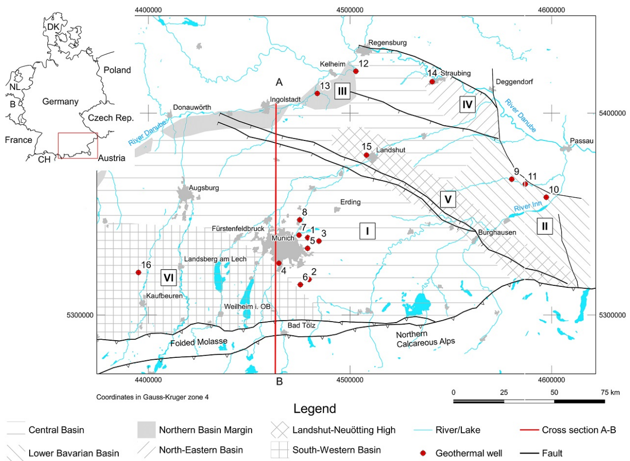
Abbildung 8: Übersicht über die hydrogeochemischen Regionen im Bayerischen Molassebecken [9].
