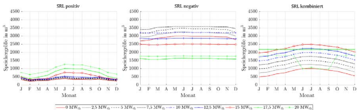
Abbildung 297: Benötigte Speichergrößen bei Angebot von positiver, negativer und kombinierter SRL des ORC-Referenz-Geothermie-Kraftwerks mit Einsatz eines Thermalwasserspeichers im Kraftwerk für Fernwärmenetzleistungen von 0 MW th bis 20 MW th bei drei 4h-Zeitscheiben Einspeicherung und zwei aufeinanderfolgenden Zeitscheiben Angebotszeitraum.
