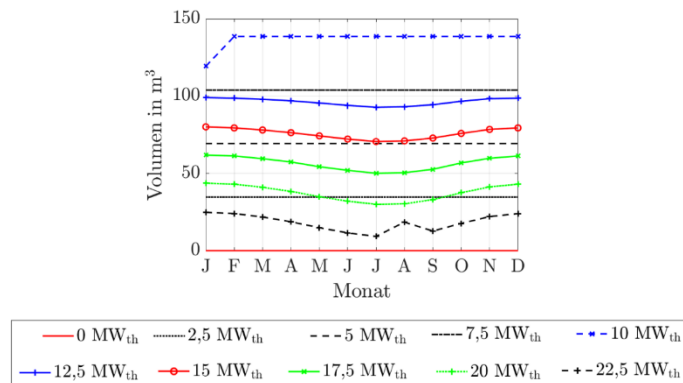
Abbildung 183: Benötigte Speichervolumina für die stationären Primärregelleistungen des Kalina-Referenz-Geothermie-Kraftwerks mit Einsatz eines Fernwärmenetzspeichers für Fernwärmenetzleistungen von 0 MW th bis 22,5 MW th .
