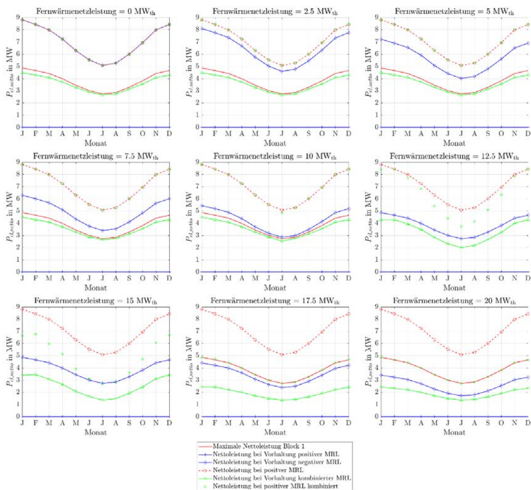
Abbildung 334: Stationäre Minutenregelleistungen des ORC-Referenz-Geothermie-Kraftwerks mit Einsatz eines Heißwasser-Wärmespeichers des Heiz- und Kraftwerks für Fernwärmenetzleistungen von 0 MW th bis 20 MW th bei drei 4h-Zeitscheiben Einspeicherung und drei aufeinanderfolgenden Zeitscheiben Angebotszeitraum.
