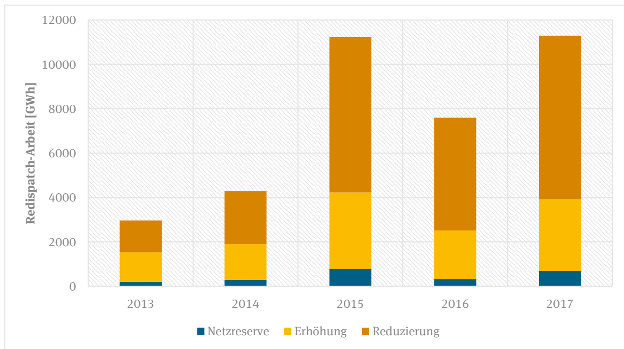
Abbildung 6: Verrichtete Redispatch-Arbeit für die Jahre 2013 bis 2017.
