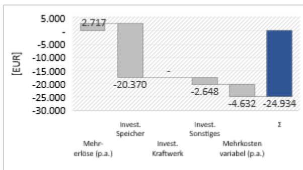
(c) Heißwasser-Wärmespeicher
