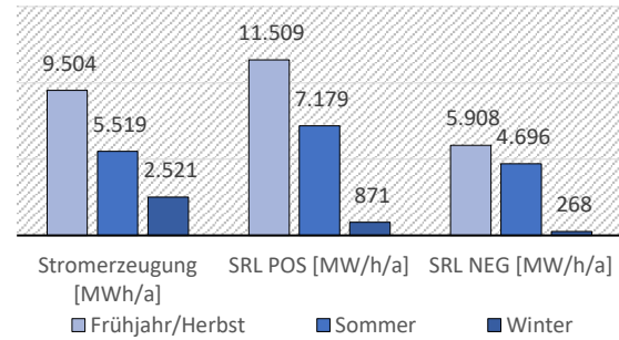
(d) Thermalwasser-Wärmespeicher
