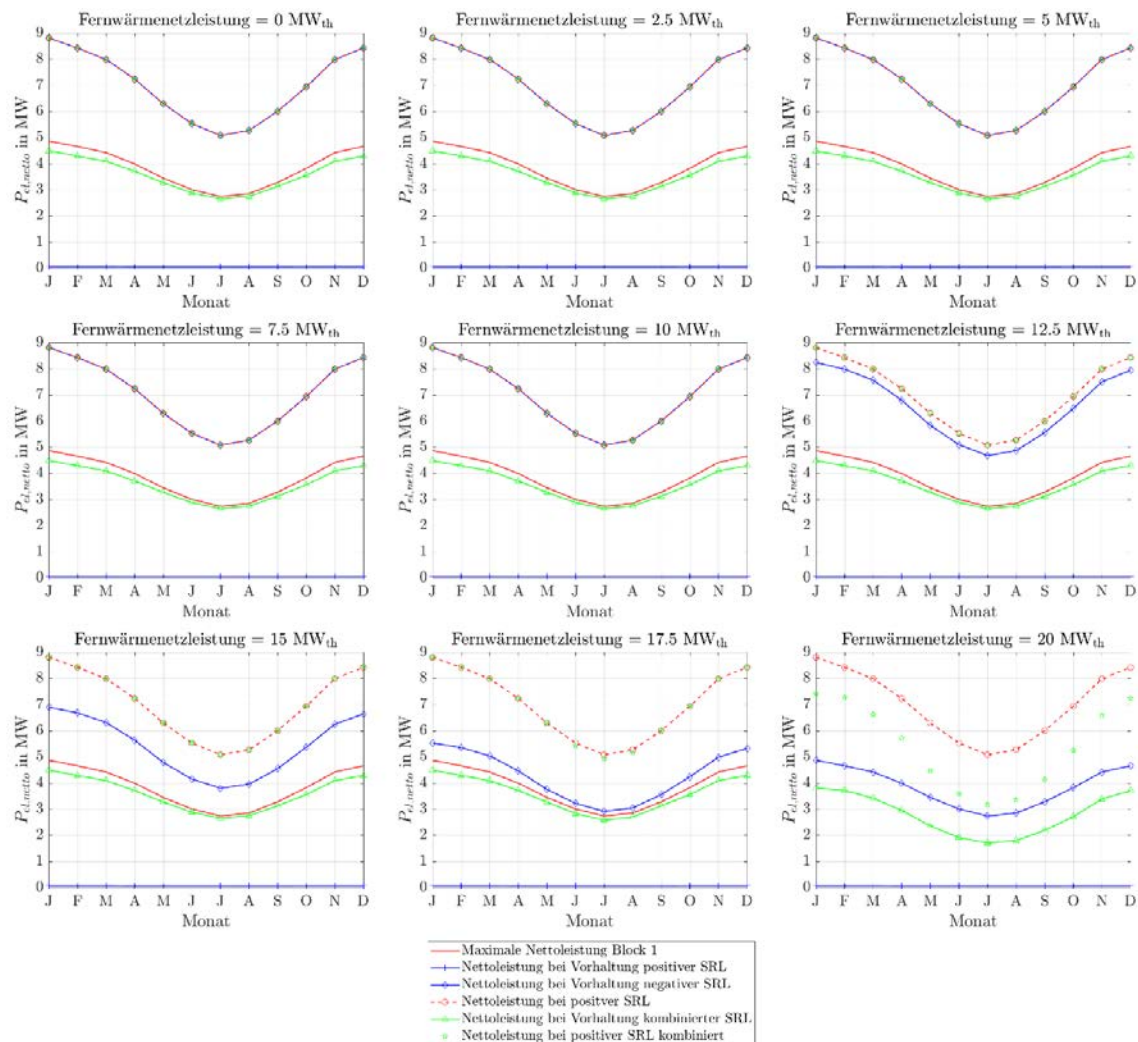
Abbildung 304: Stationäre Sekundärregelleistungen des Referenz-Geothermie-Kraftwerks mit Einsatz eines Heißwasser-Wärmespeichers des Heiz- und Kraftwerks für Fernwärmenetzleistungen von 0 MW th bis 20 MW th bei vier 4h-Zeitscheiben Einspeicherung und zwei aufeinanderfolgenden Zeitscheiben Angebotszeitraum.
