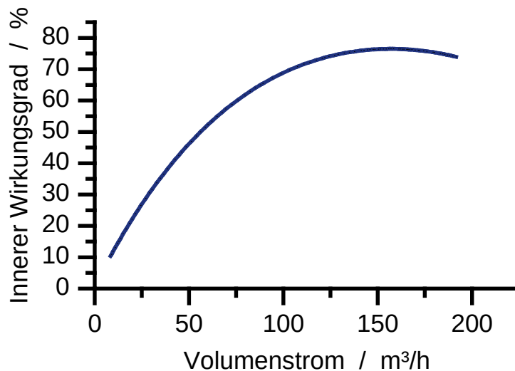
Abbildung 60: Innerer Wirkungsgrad der ORC-Speisepumpe in Abhängigkeit des Volumenstroms.
