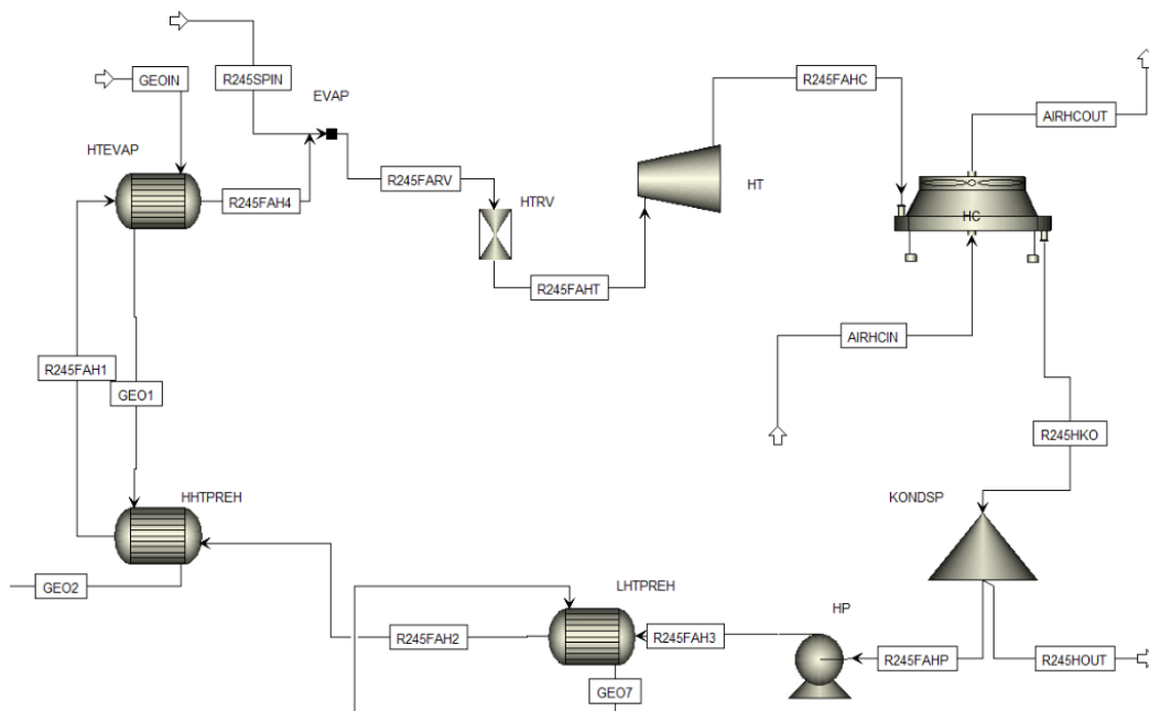
Abbildung 101: Stationäres Simulationsmodell des modifizierten Hochdruckkreises des ORC-Referenz-Geothermie-Kraftwerks für die Berechnung der Betriebszustände des Kraftwerks mit Einsatz eines Dampfspeichers [98, S. 52].
