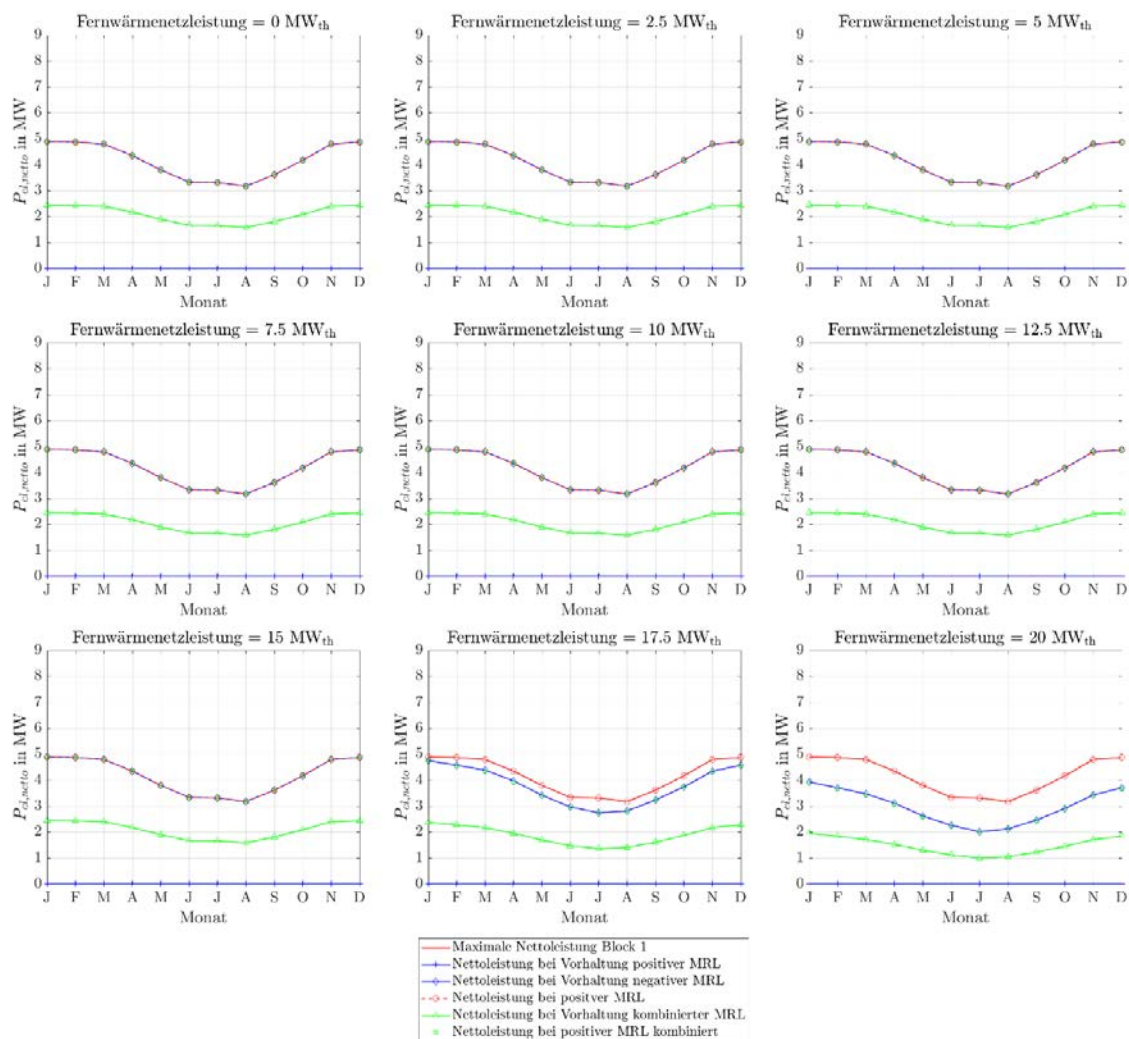
Abbildung 330: Stationäre Minutenregelleistungen des ORC-Referenz-Geothermie-Kraftwerks mit Einsatz eines Heißwasser-Wärmespeichers im Fernwärmenetz für Fernwärmenetzleistungen von 0 MW th bis 20 MW th bei drei 4h-Zeitscheiben Einspeicherung und drei aufeinanderfolgenden Zeitscheiben Angebotszeitraum.
