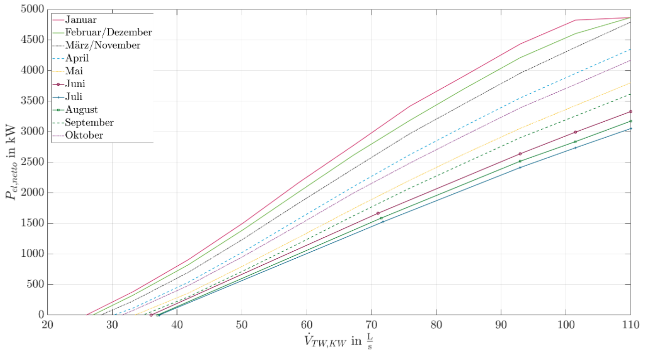
Abbildung 70: Nettoleistungs-Thermalwasservolumenstrom-Diagramm für das ORC-Referenz-Geothermie-Kraftwerk.
