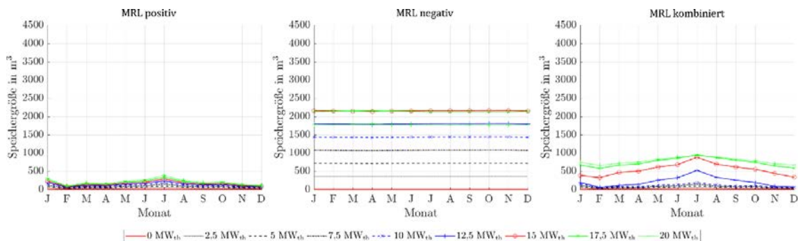
Abbildung 313: Benötigte Speichergrößen bei Angebot von positiver, negativer und kombinierter MRL des ORC-Referenz-Geothermie-Kraftwerks mit Einsatz eines Heißwasser-Wärmespeichers im Fernwärmenetz für Fernwärmenetzleistungen von 0 MW th bis 20 MW th bei zwei 4h-Zeitscheiben Einspeicherung und zwei aufeinanderfolgenden Zeitscheiben Angebotszeitraum.
