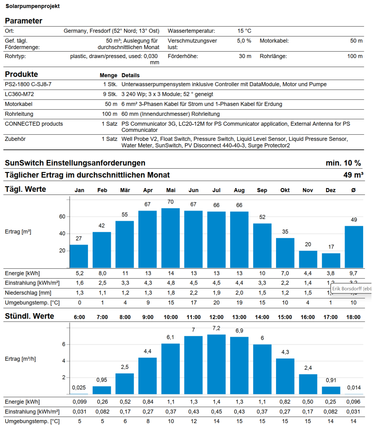
Abbildung 114: Solaranlagenauslegung für den Standort Fresdorf.
