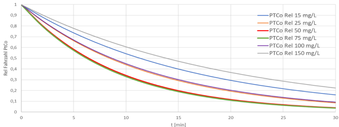
Abbildung 53: Vergleich der Reaktionsgeschwindigkeiten für unterschiedliche Wasserstoffperoxidkonzentrationen.
